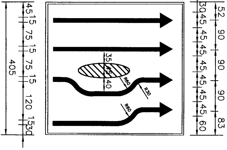
王田南向189K+076門架 圖示車輛改道告示牌 (B-B/W)
