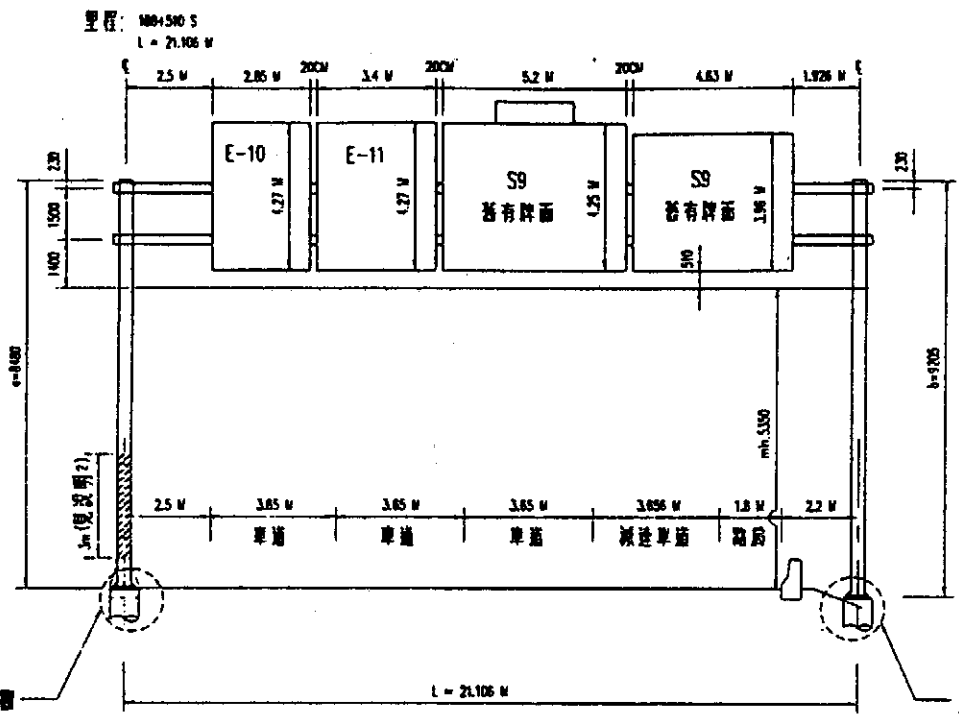
架空型標註 (一) 188+510 S
