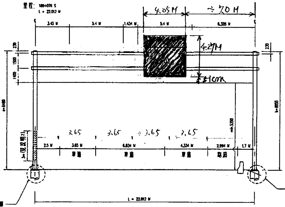
架空型標註 (二) 189+076 S
