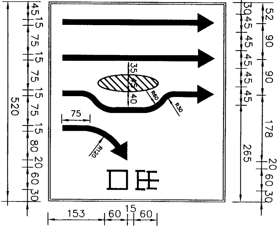
王田北向190K+695門架 圖示車輛改道告示牌 (B-B/W)
