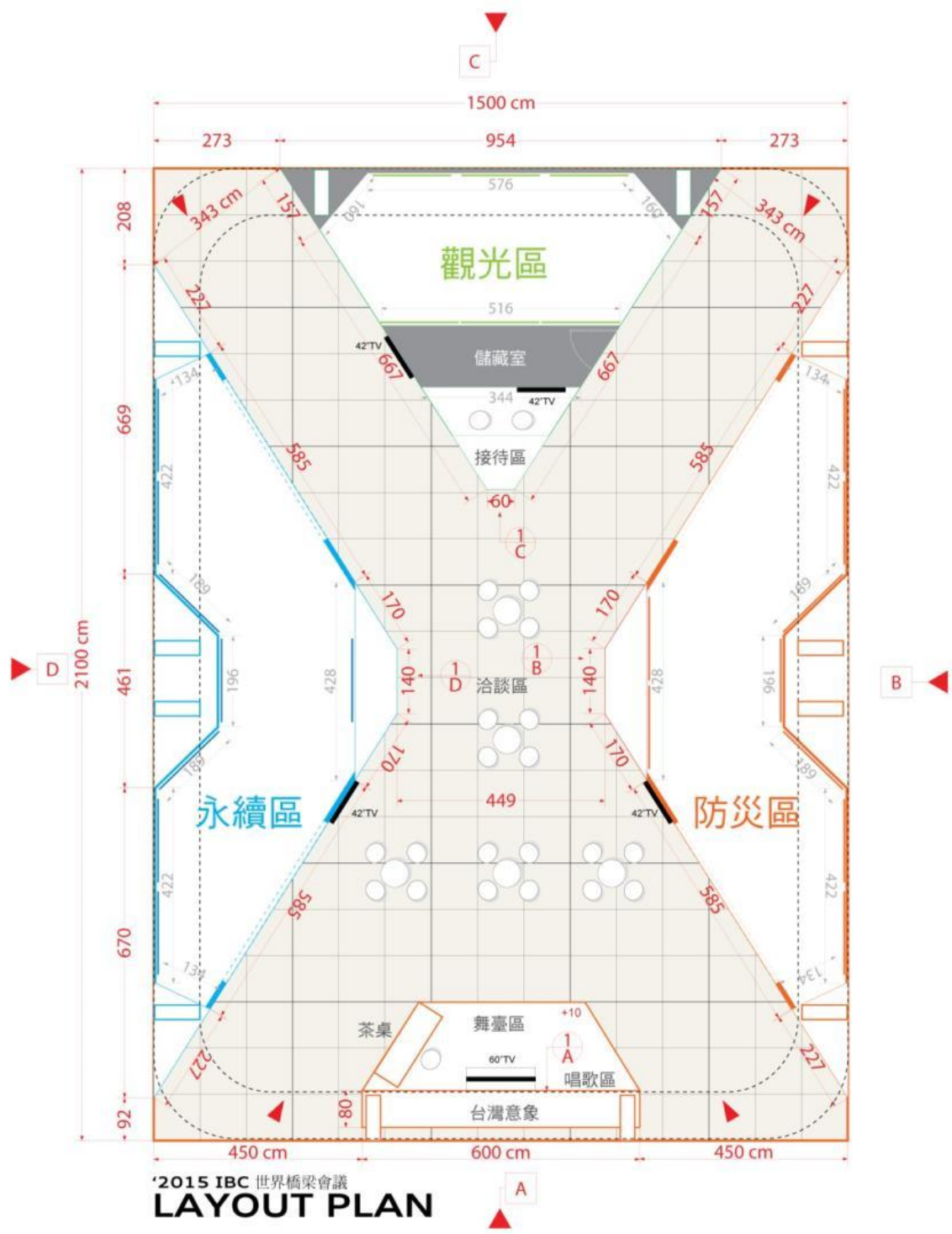
圖 2-2 臺灣主題館平面配置圖
