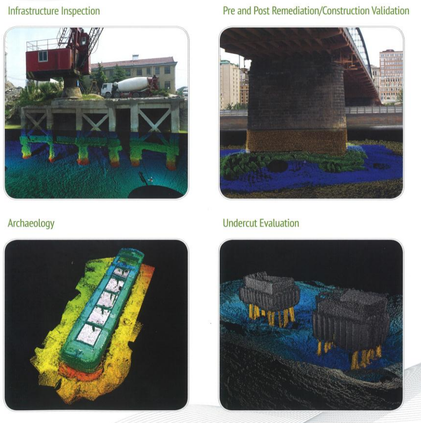
圖4-1 橋梁基礎水下檢測3D顯示的新科技
