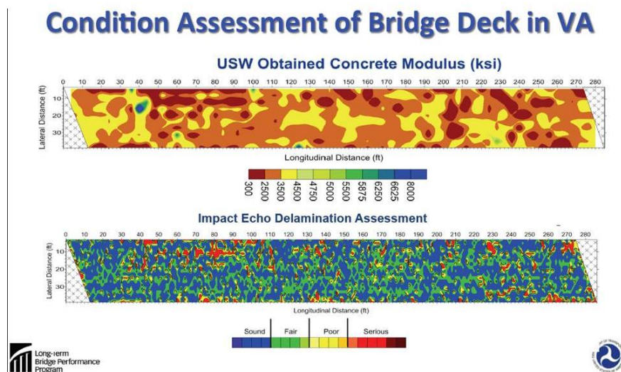
圖 4-4 敲擊聲波回音之劣化評估
