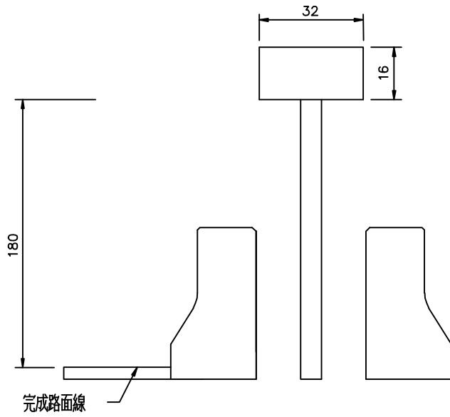
側百公尺里程牌 ( A 型, 適用於中央有植栽, 護欄僅為示意 )
