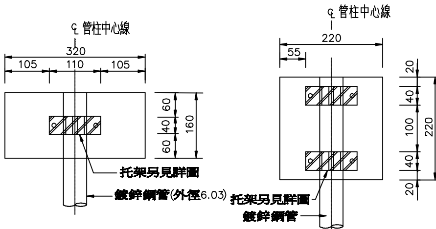
牌面安裝詳圖
