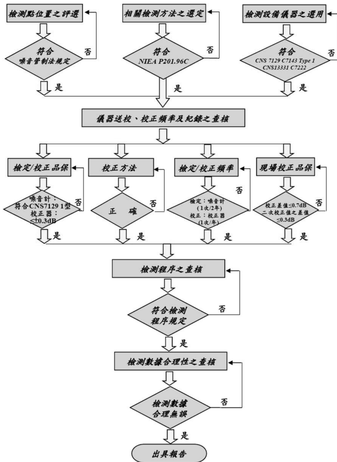
圖 1-3 噪音檢測品保/品管作業流程
