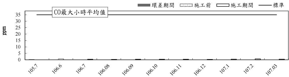
圖 2-1(2) 計畫區測站空氣品質監測結果
