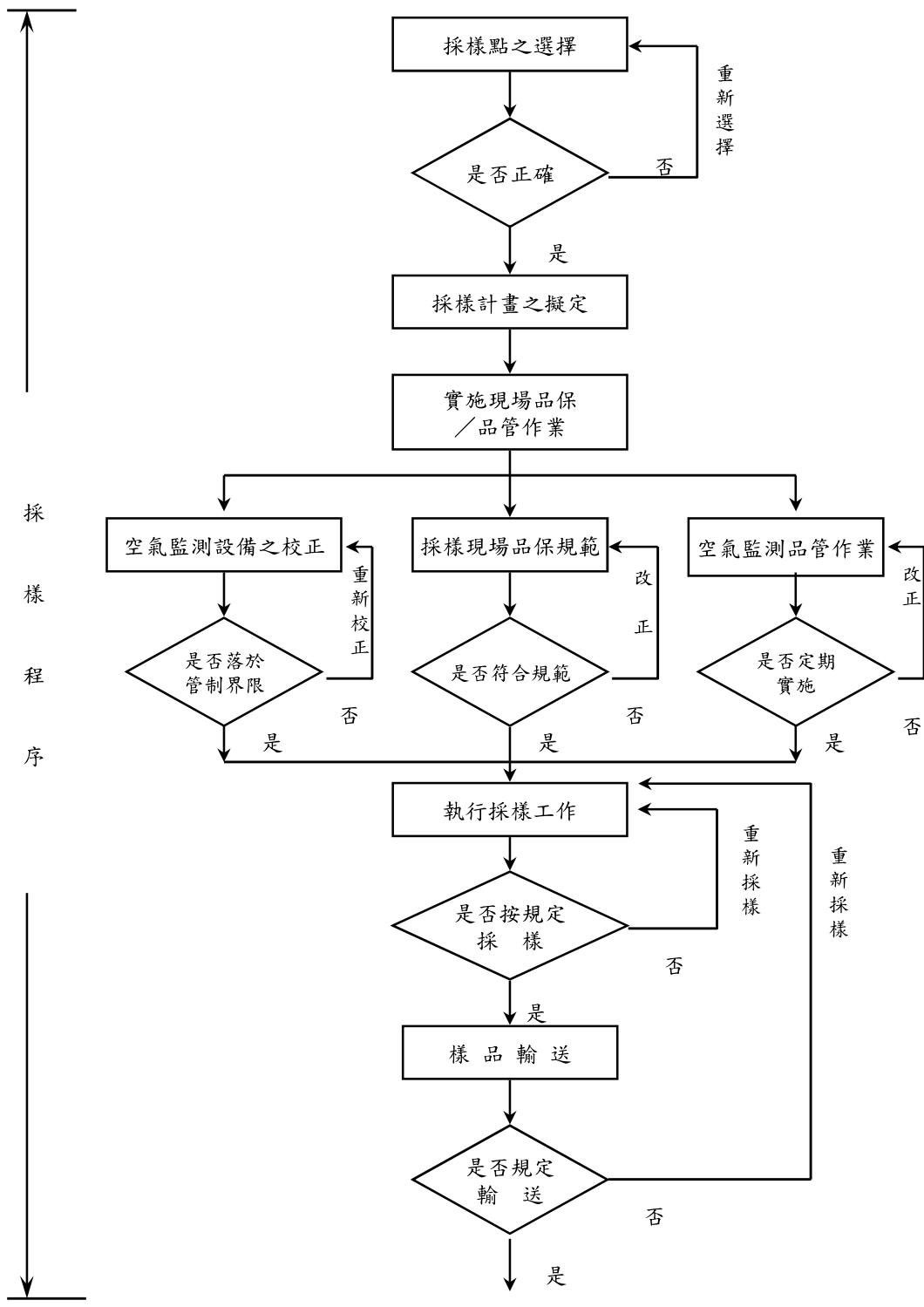
圖 1-2 空氣品質檢測品保/品管作業流程(1/2)
