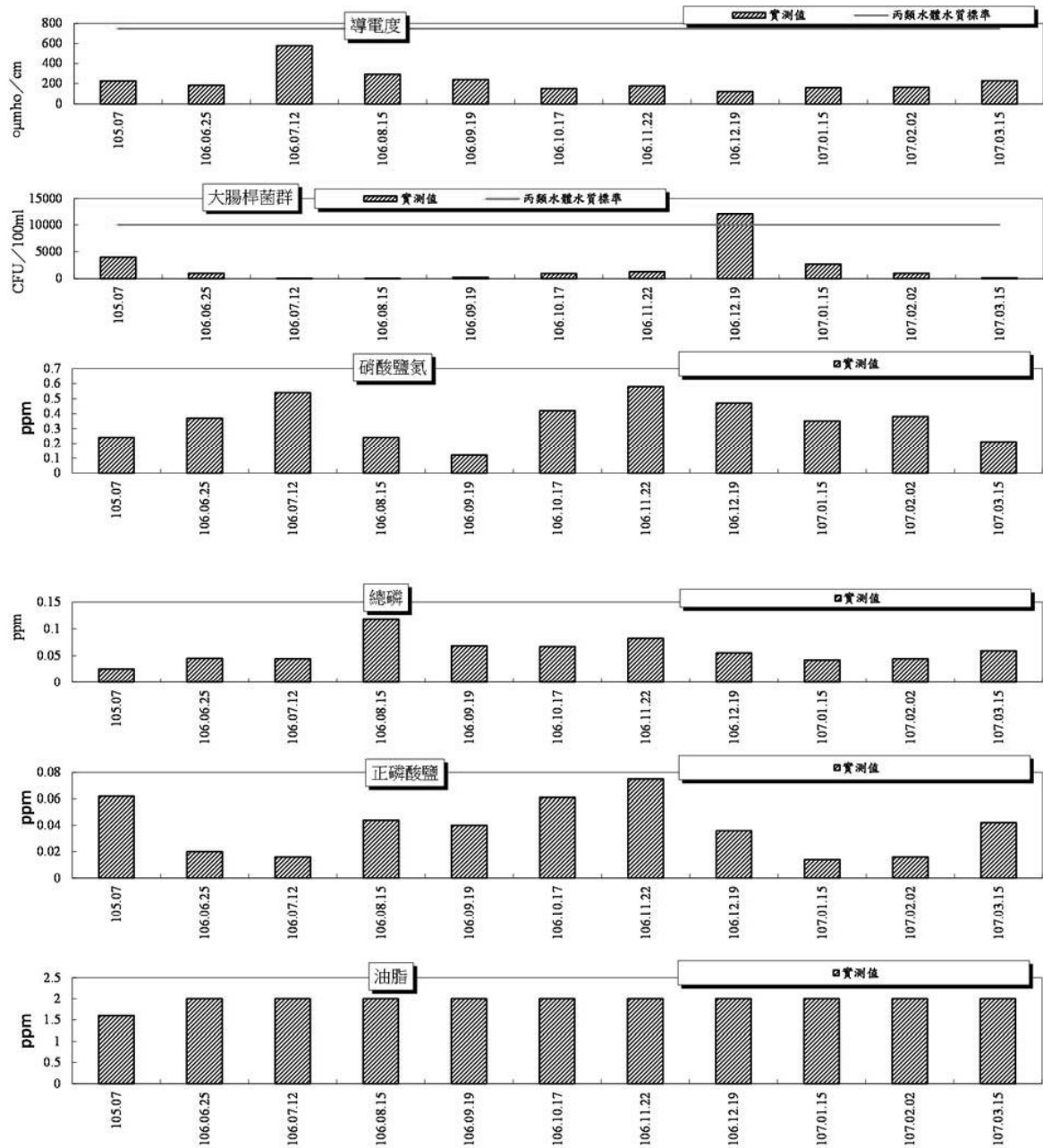
圖 2-8(2) 新城溪下游測站水質監測結果
