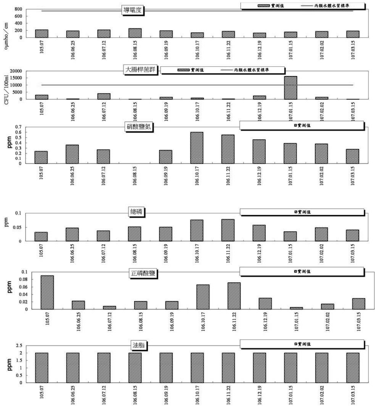
圖 2-7(2) 新城溪上游測站水質監測結果
