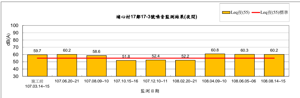
圖 2.2-3 埔心村 17 鄰 17-3 號環境噪音監測結果(夜間)
