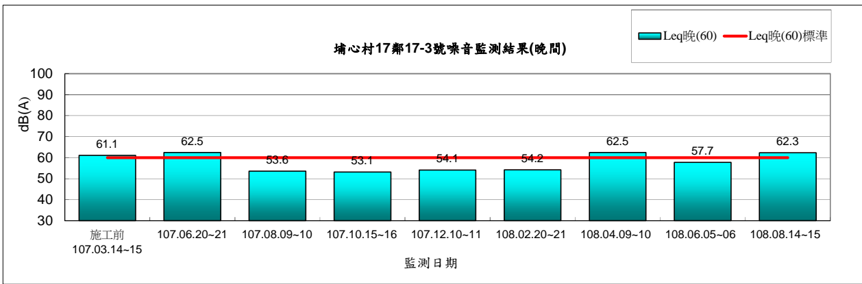
圖 2.2-2 埔心村 17 鄰 17-3 號環境噪音監測結果(晚間)
