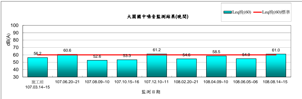
圖 2.2-5 大園國中環境噪音監測結果(晚間)
