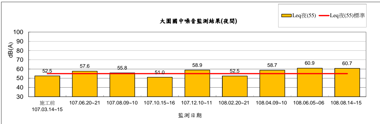
圖 2.2-6 大園國中環境噪音監測結果(夜間)
