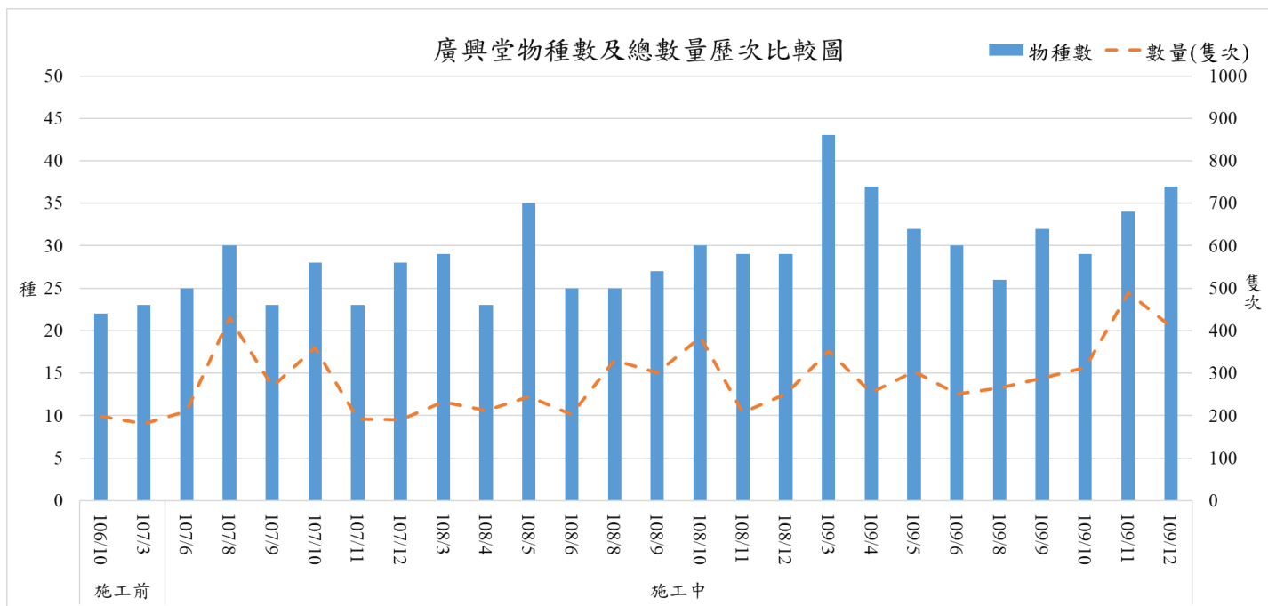
圖 2.7-8 物種數及總數量歷次比較(廣興堂)
