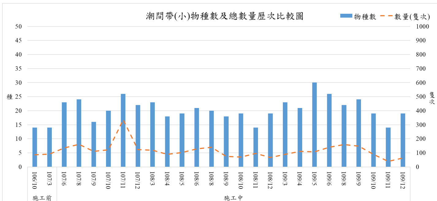
圖 2.7-10 物種數及總數量歷次比較(潮間帶-小)
