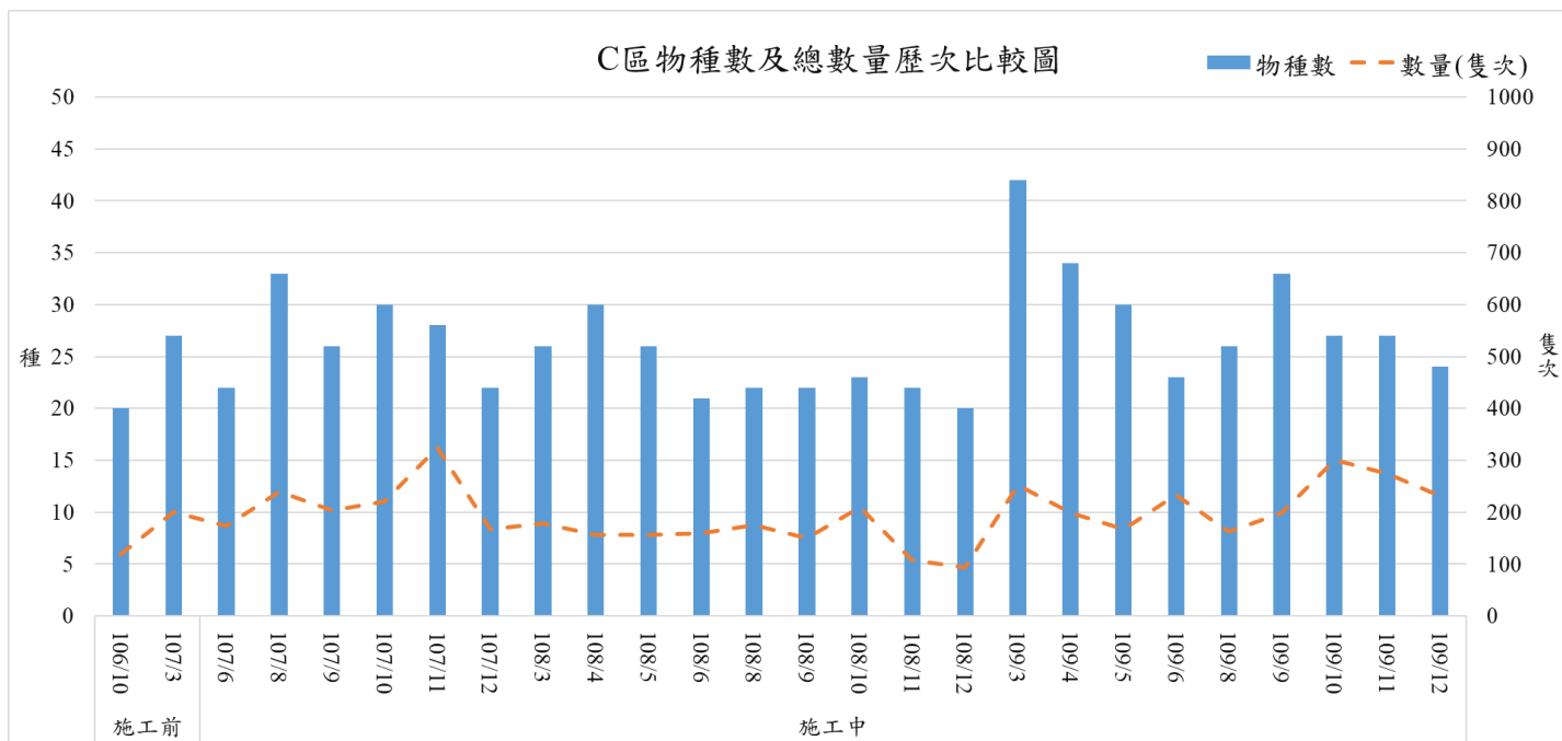
圖 2.7-7 物種數及總數量歷次比較(C區)
