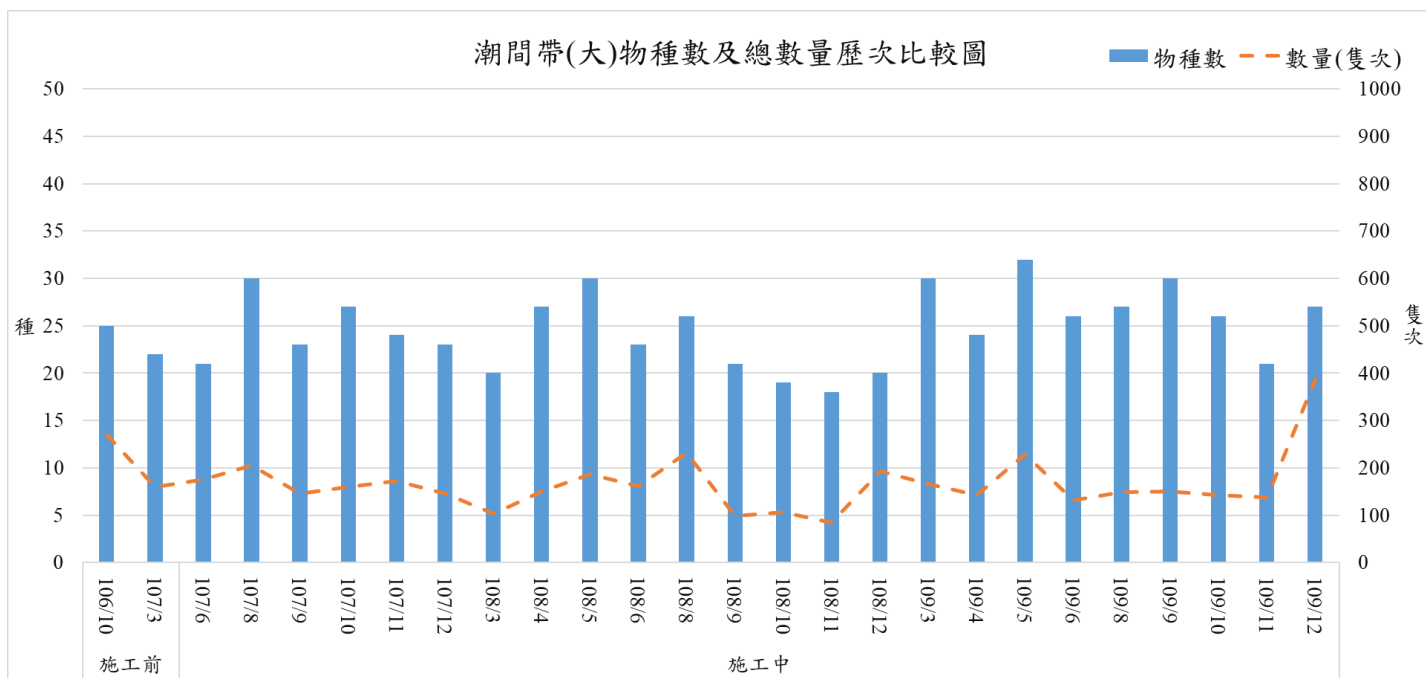
圖 2.7-9 物種數及總數量歷次比較(潮間帶-大)
