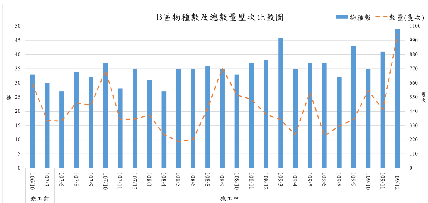
圖 2.7-6 物種數及總數量歷次比較(B 區)
