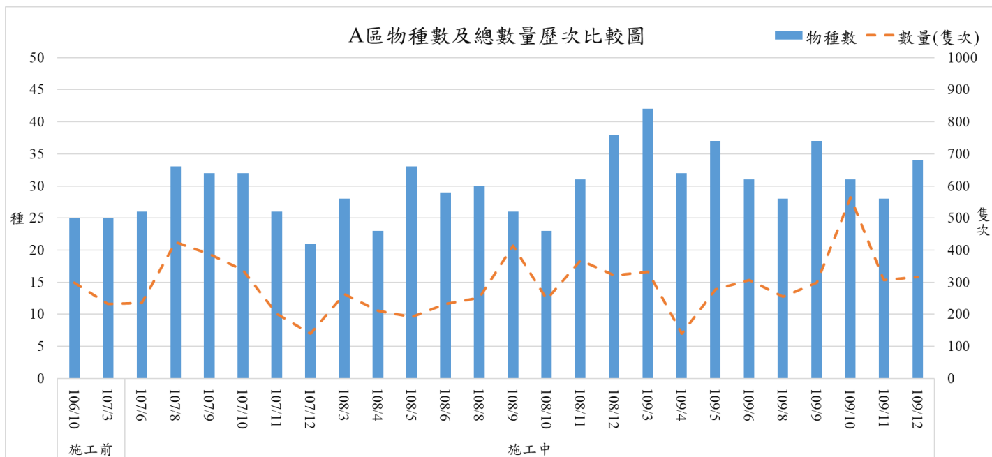
圖 2.7-5 物種數及總數量歷次比較(A 區)
