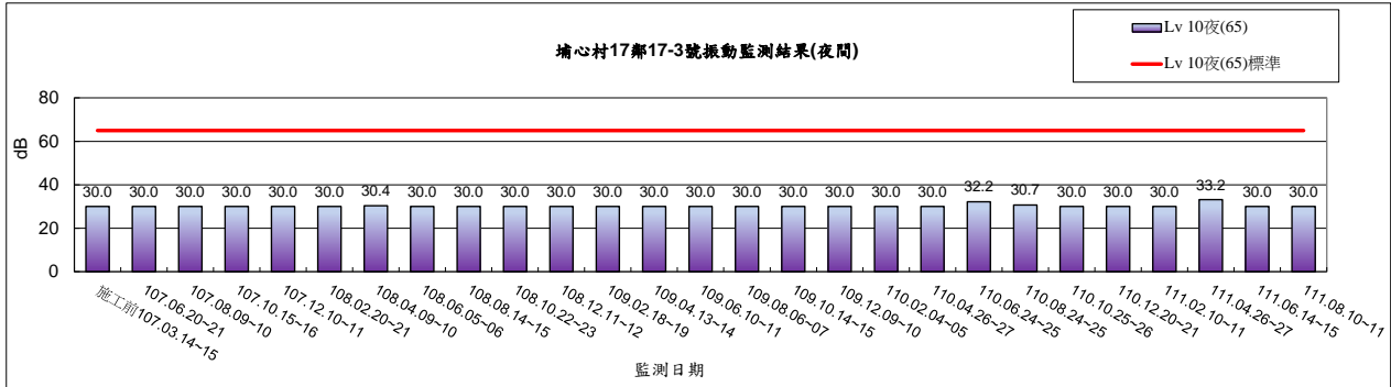
圖 2.2-8 埔心村 17 鄰 17-3 號環境振動監測結果(夜間)
