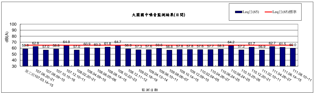
圖 2.2-4 大園國中環境噪音監測結果(日間)
