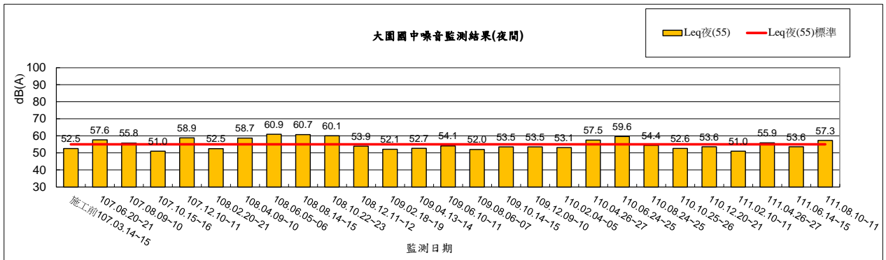
圖 2.2-6 大園國中環境噪音監測結果(夜間)
