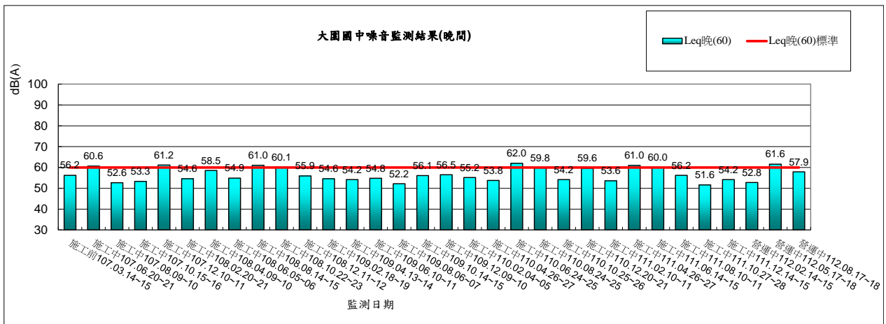
圖 2.2-5 大園國中環境噪音監測結果(晚間)
