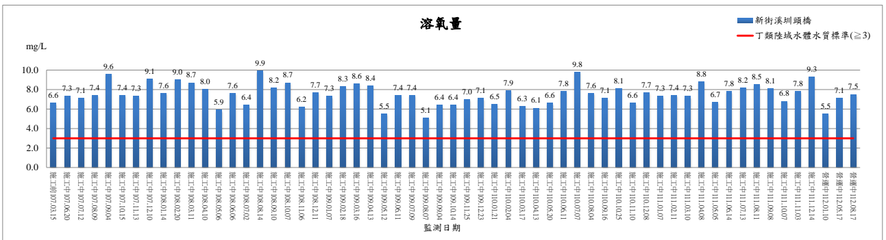
圖 2.3-3 河川水質之溶氧量監測結果趨勢圖
