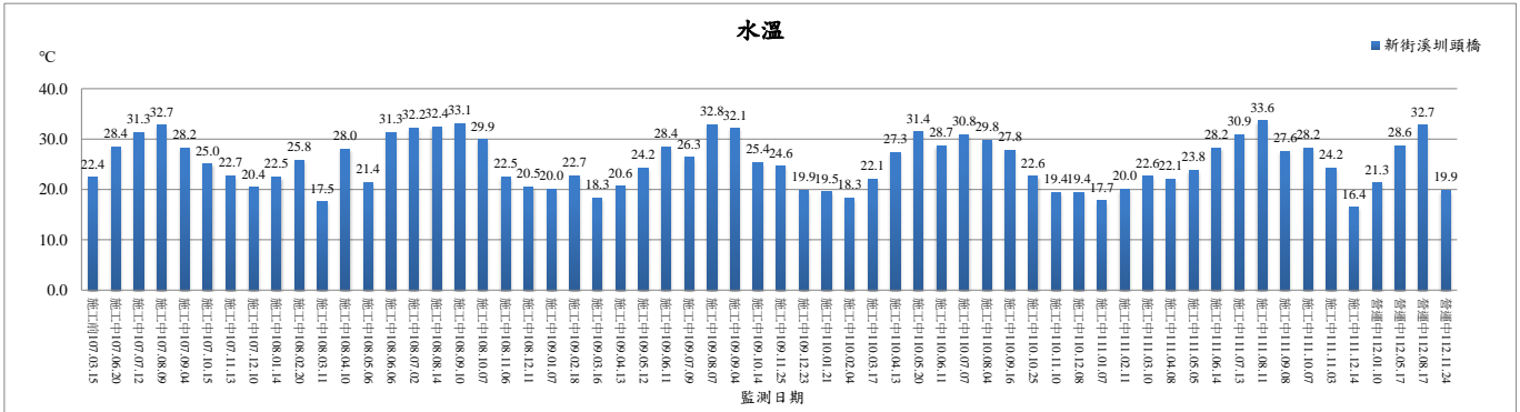
圖 2.3-2 河川水質之水溫監測結果趨勢圖
