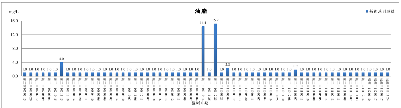
圖 2.3-7 河川水質之油脂監測結果趨勢圖
