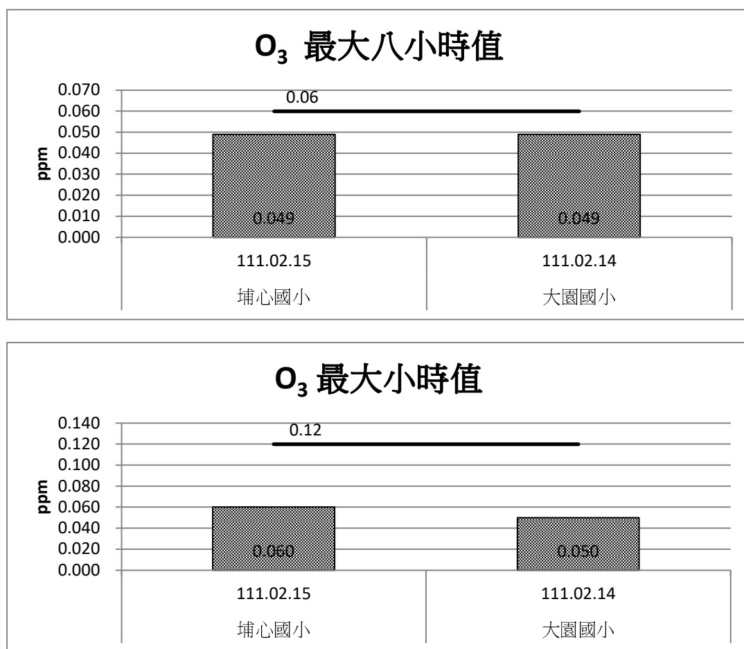
圖 2.1-6 施工期間空氣品質 O 3 監測成果比較圖(111 年 1 月~3 月)
