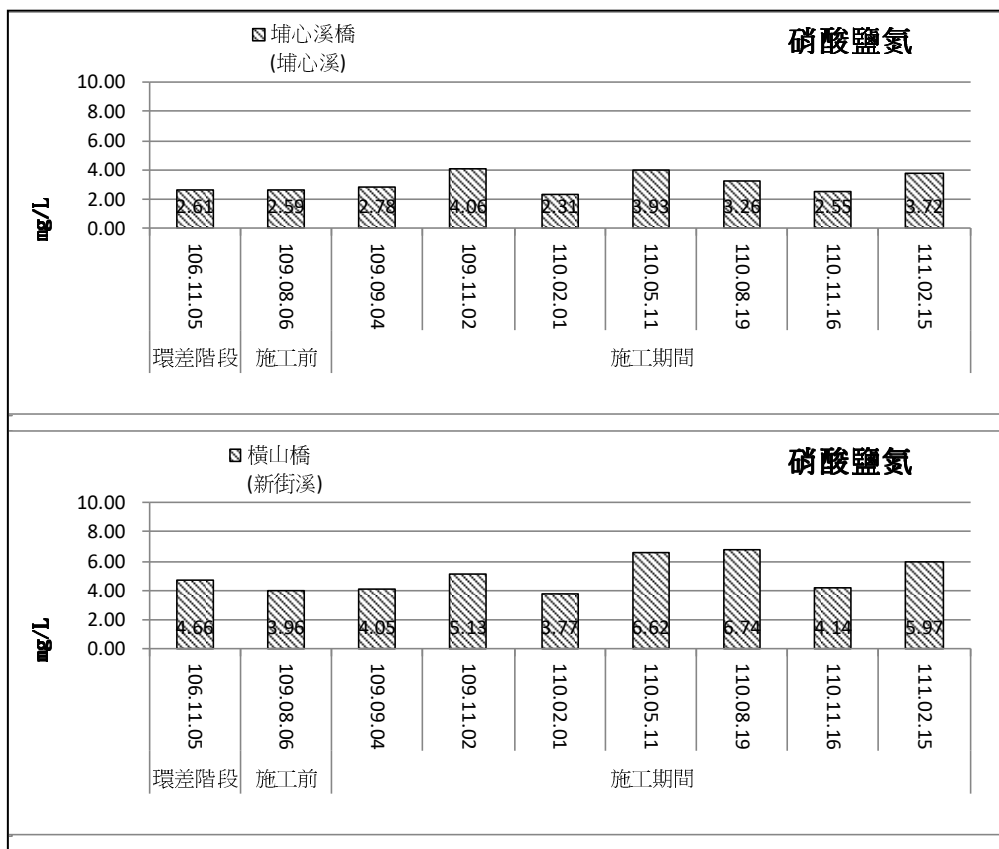
圖 3.1.6-7 計畫區周邊歷次河川水質硝酸鹽氮監測成果
