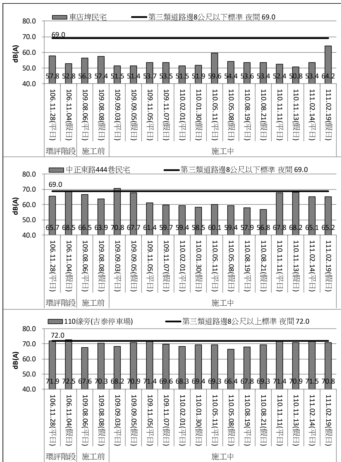
圖 3.1.3-3 計畫區周邊歷次環境噪音 L night 監測成果
