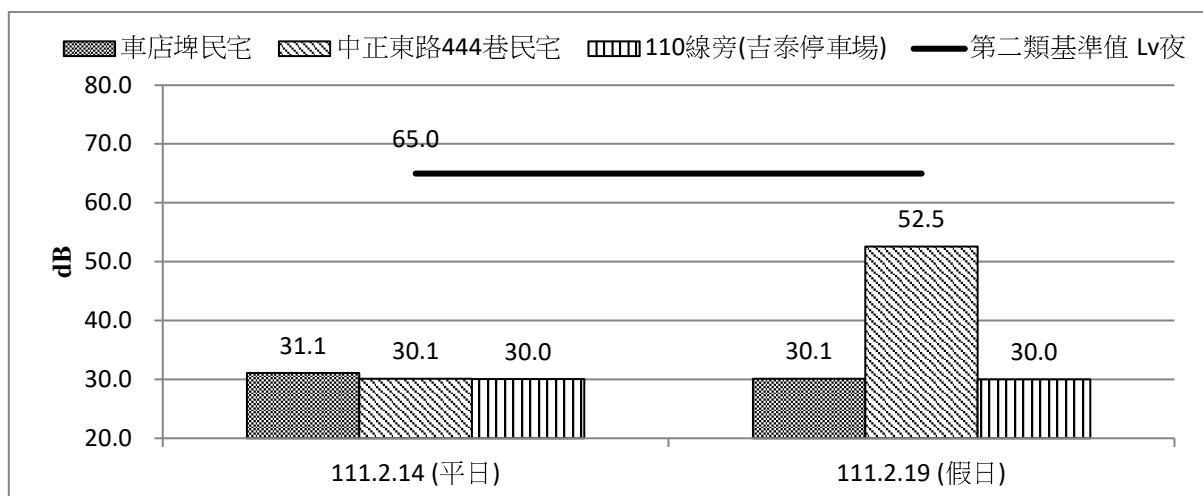
圖 2.2-5 施工期間環境振動 L_{v10夜} 監測成果比較圖(111 年 1 月~3 月)
