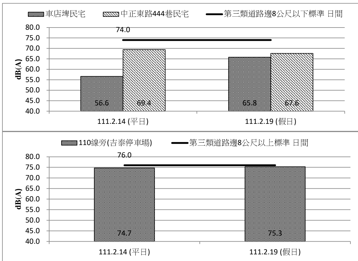
圖 2.2-1 施工期間環境噪音 L eq 監測成果比較圖(111 年 1 月~3 月)
