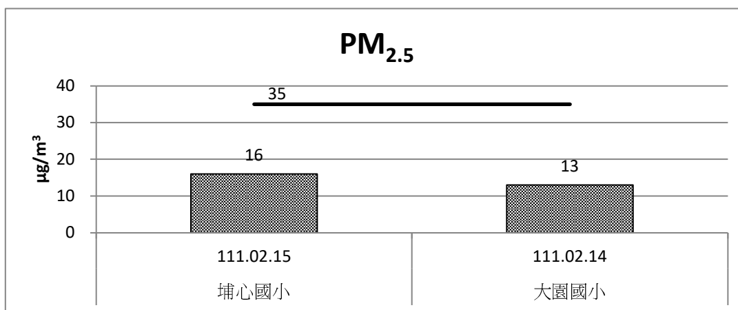
圖 2.1-3 施工期間空氣品質 PM 2.5 監測成果比較圖(111 年 1 月~3 月)
