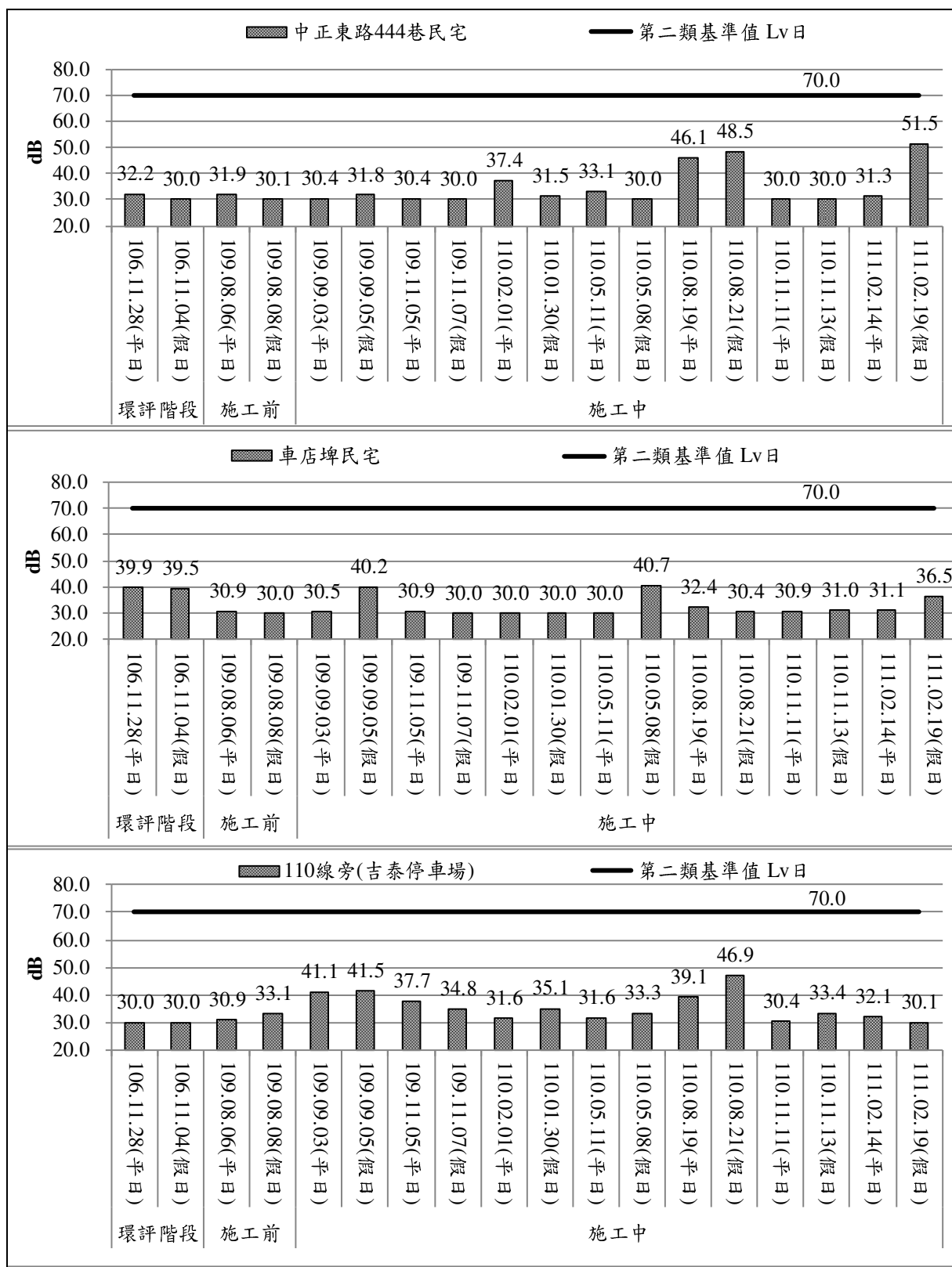
圖 3.1.3-4 計畫區周邊歷次環境振動 Lv10 日監測成果
