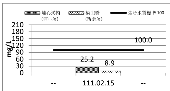
圖 2.5-6 施工期間第 7 期(111 年 1 月~3 月)河川水質懸浮固體監測成果圖
