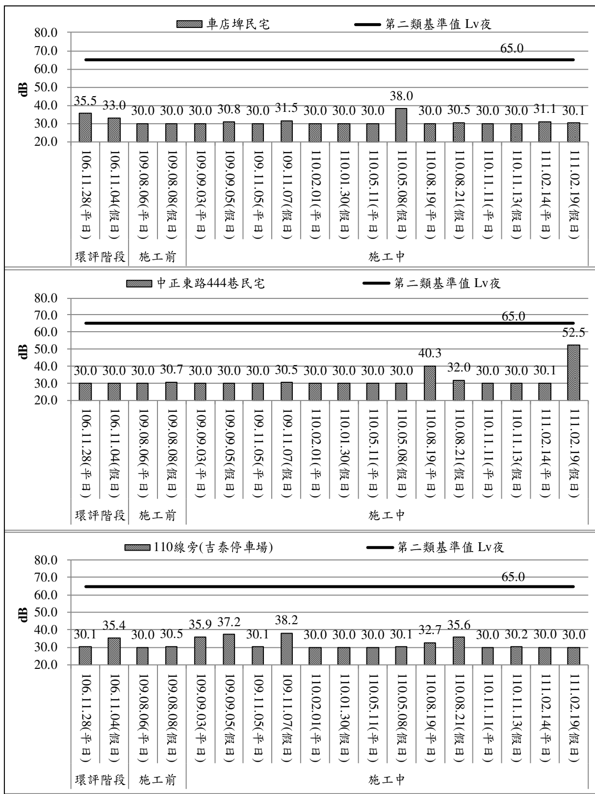
圖 3.1.3-5 計畫區周邊歷次環境振動 L v10 夜監測成果
