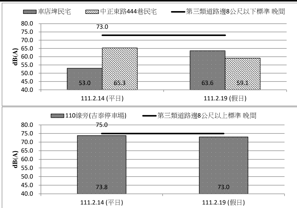
圖 2.2-2 施工期間環境噪音 L w 監測成果比較圖(111 年 1 月~3 月)
