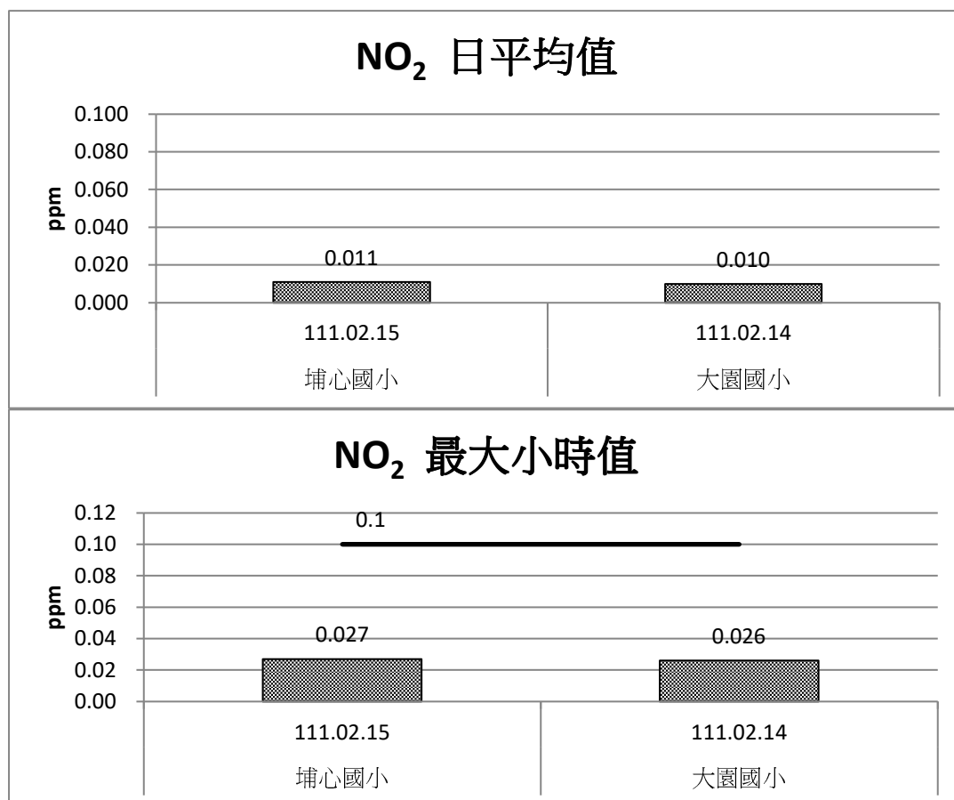
圖 2.1-7 施工期間空氣品質 NO 2 監測成果比較圖(111 年 1 月~3 月)
