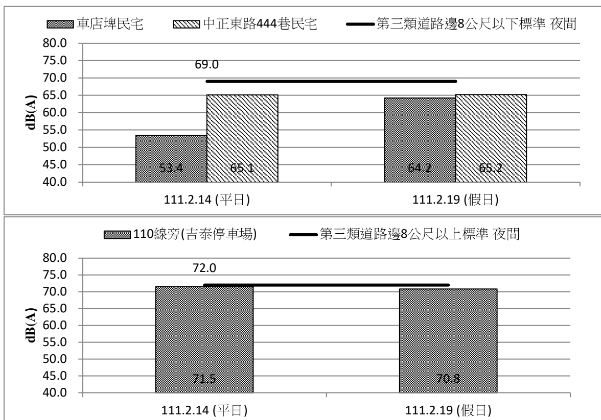
圖 2.2-3 施工期間環境噪音 L w 監測成果比較圖(111 年 1 月~3 月)
