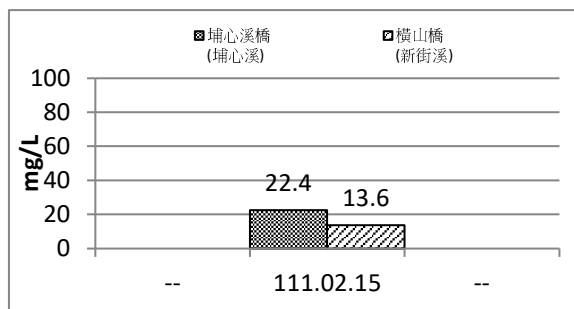
圖 2.5-10 施工期間第 7 期(111 年 1 月~3 月) 河川水質化學需氧量監測成果圖
