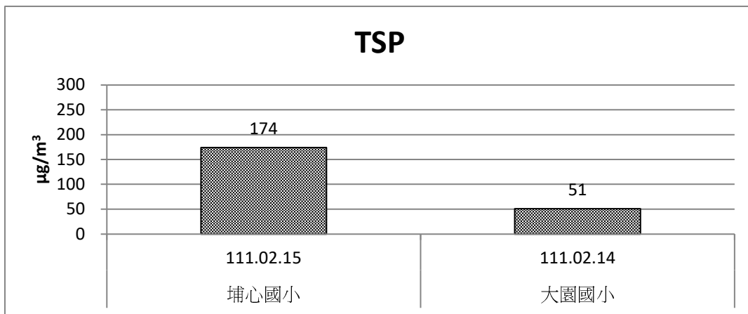
圖 2.1-1 施工期間空氣品質 TSP 監測成果比較圖(111 年 1 月~3 月)
