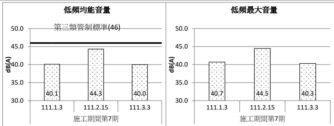
圖 2.3-1 施工期間第 7 期低頻噪音監測成果比較(111 年 1 月~3 月)
