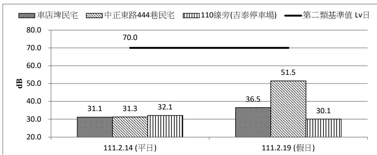
圖 2.2-4 施工期間環境振動 L_{v10日} 監測成果比較圖(111 年 1 月~3 月)
