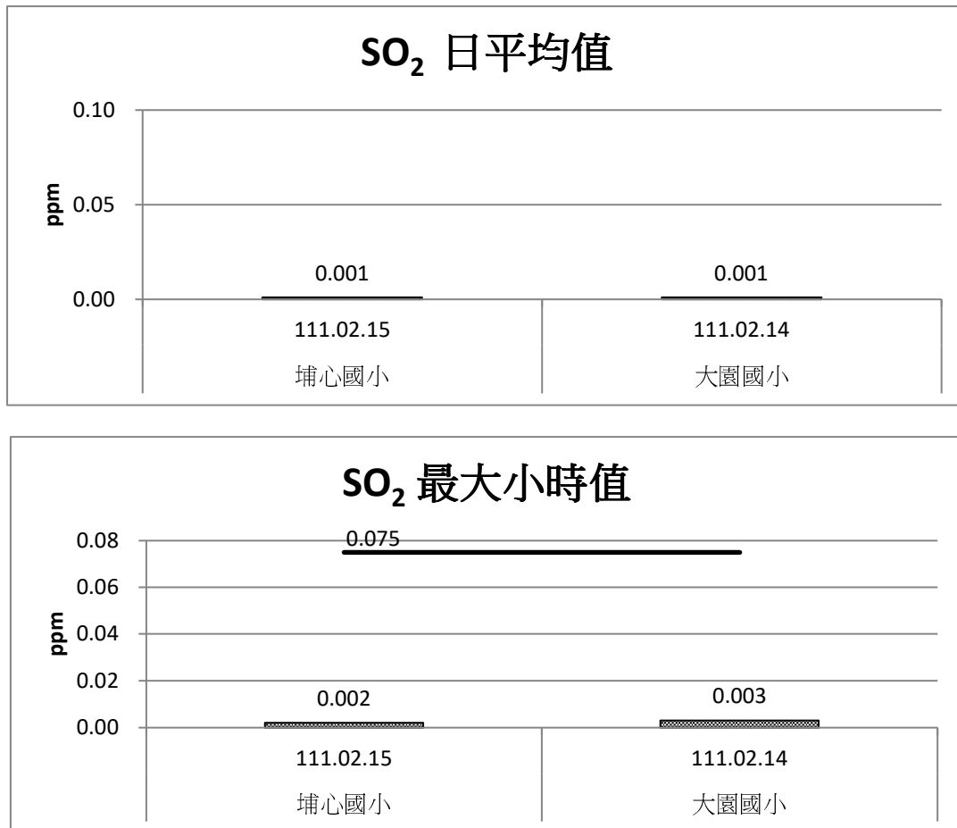
圖 2.1-4 施工期間空氣品質 SO 2 監測成果比較圖(111 年 1 月~3 月)
