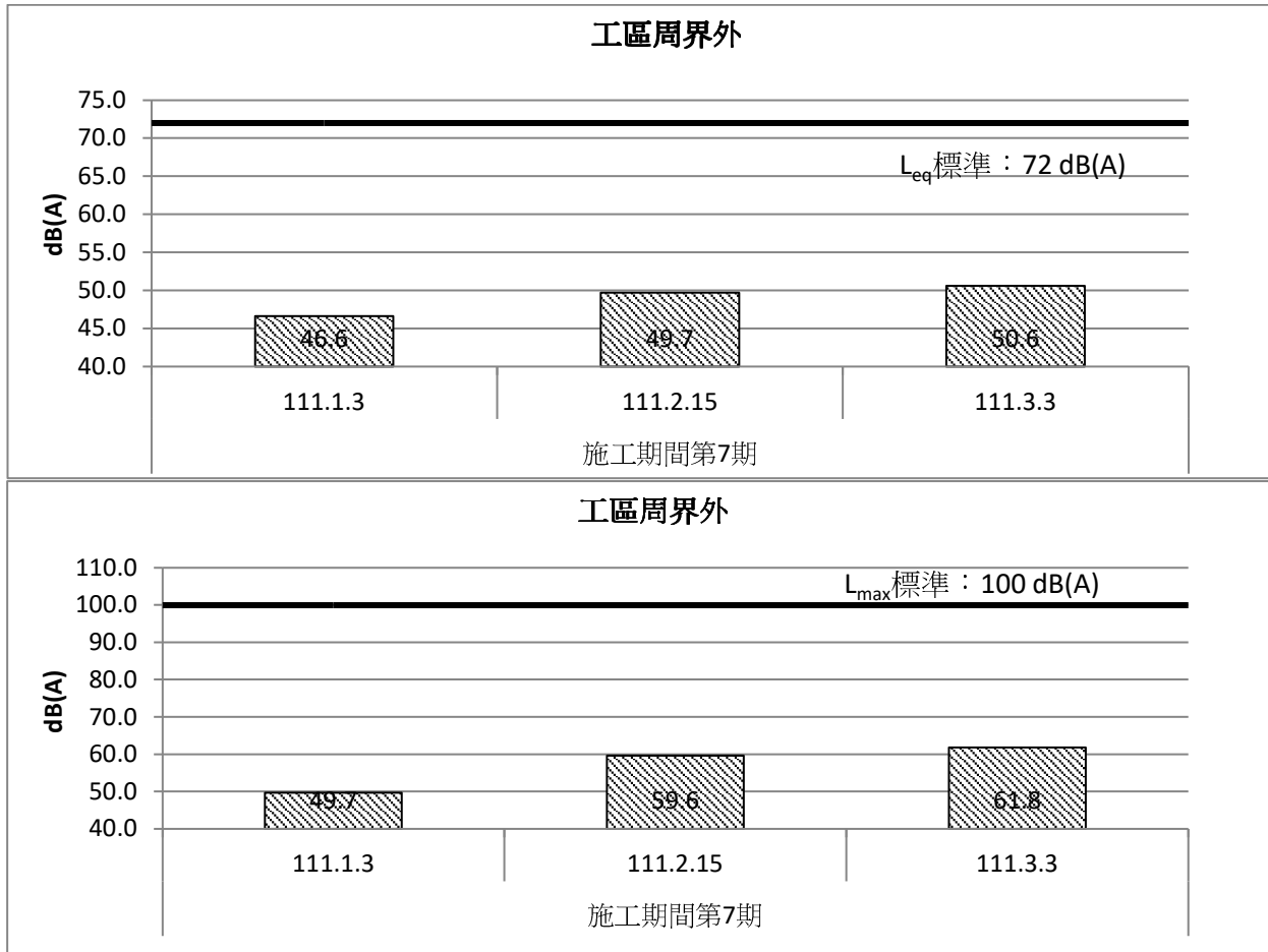
圖 2.4-1 施工期間第7期營建噪音監測成果比較圖(111年1月~3月)
