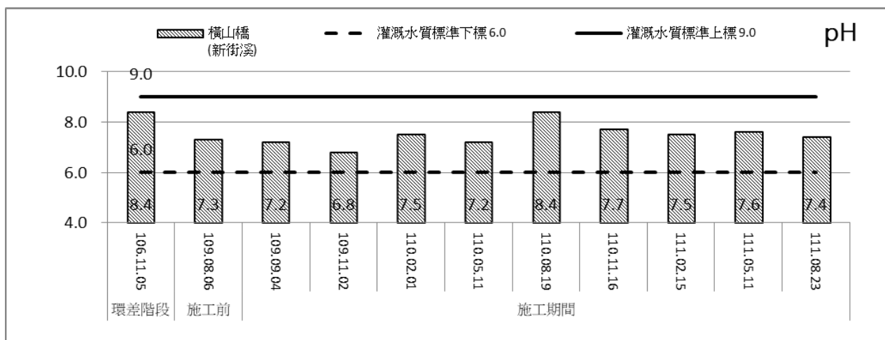
圖 3.1.6-1 計畫區周邊歷次河川水質 pH 監測成果
