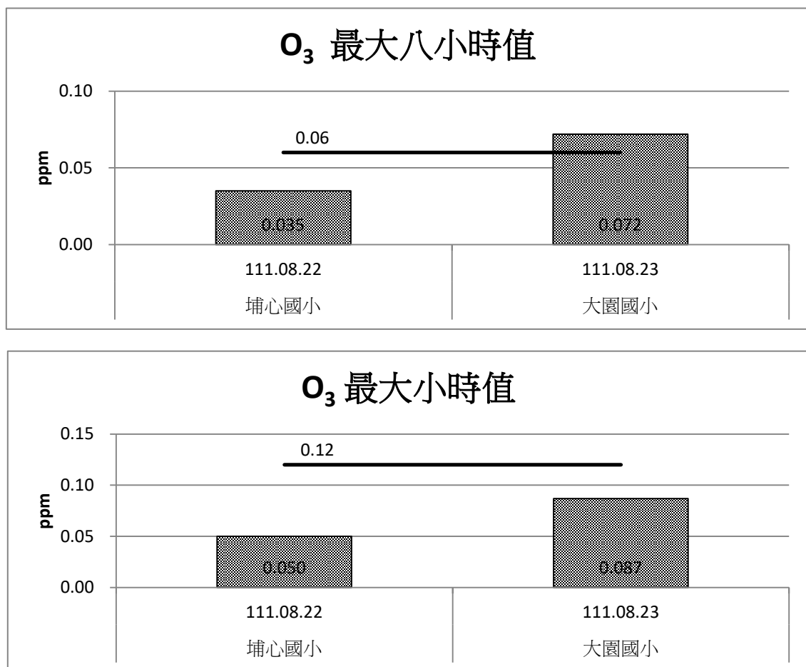
圖 2.1-6 施工期間空氣品質 O 3 監測成果比較圖(111 年 7 月~9 月)
