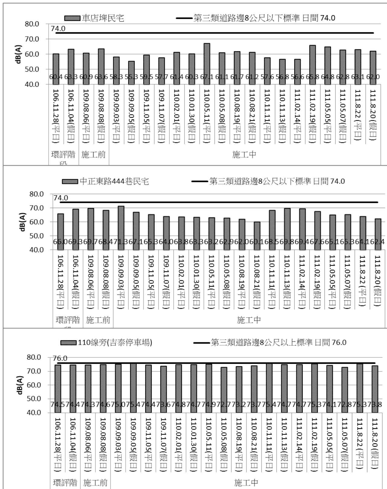
圖 3.1.3-1 計畫區周邊歷次環境噪音 L d 監測成果
