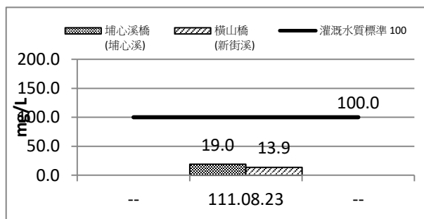
圖 2.5-6 施工期間第 9 期(111 年 7 月~9 月)河川水質懸浮固體監測成果圖
