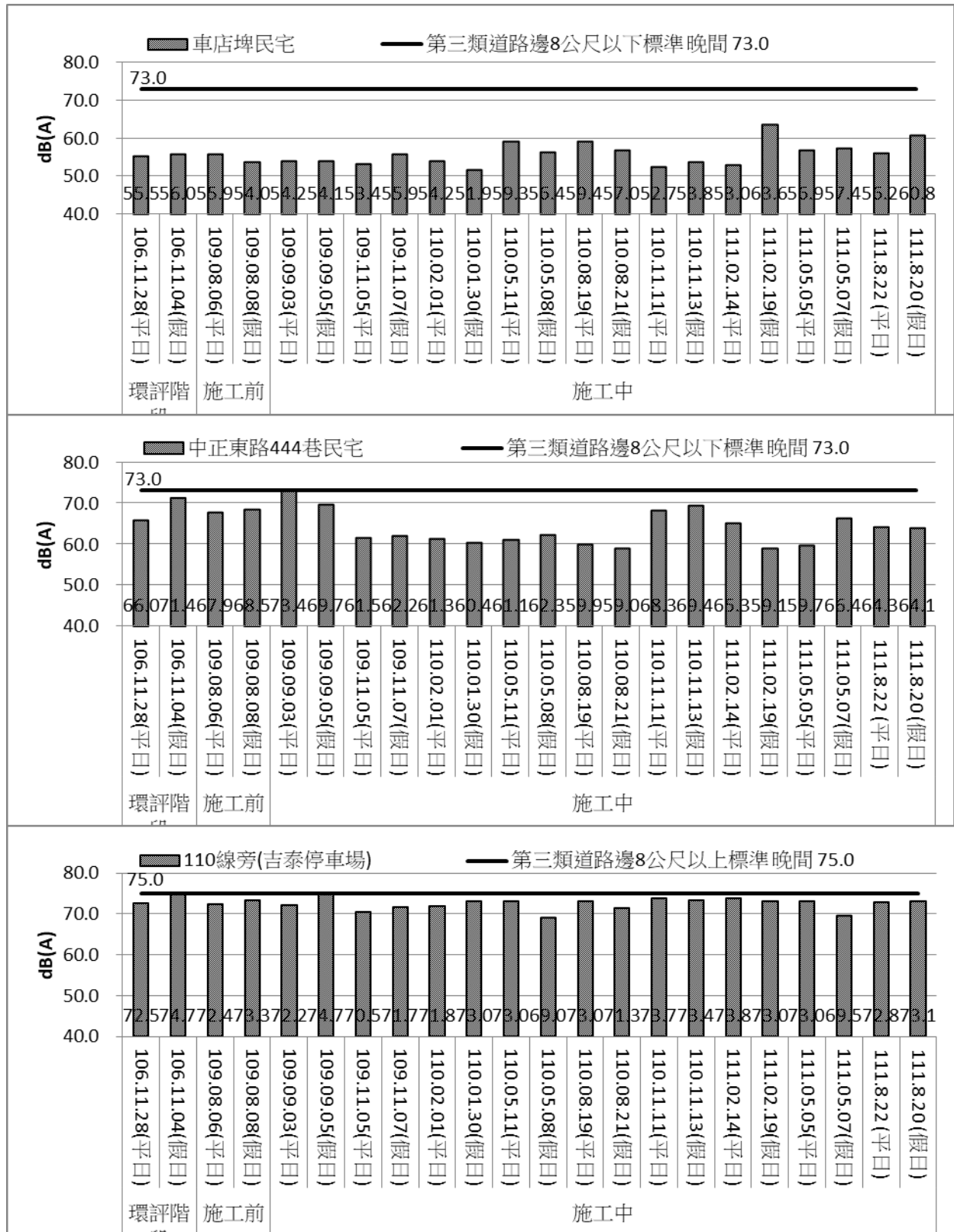
圖 3.1.3-2 計畫區周邊歷次環境噪音 L w 監測成果
