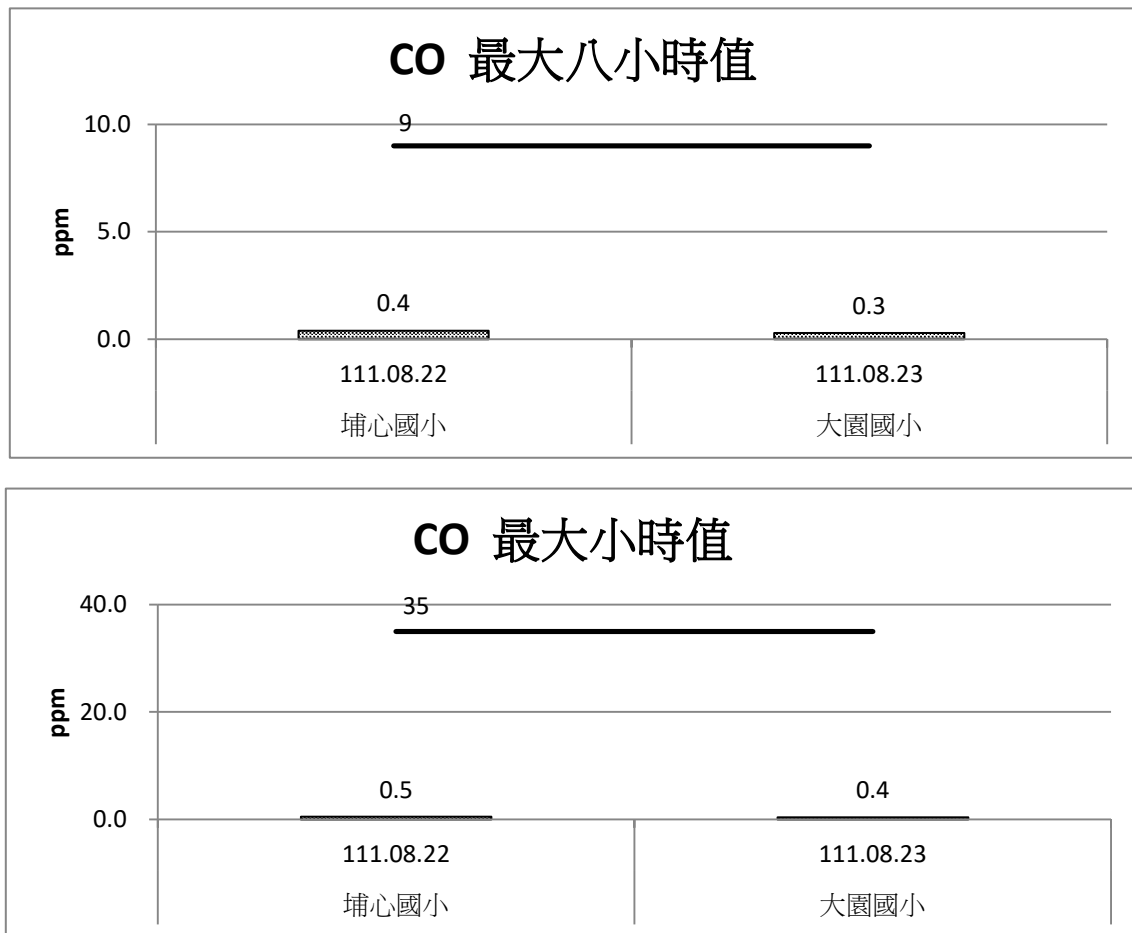
圖 2.1-5 施工期間空氣品質 CO 監測成果比較圖(111 年 7 月~9 月)
