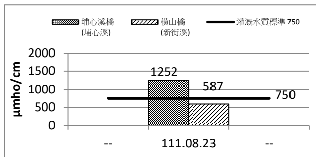
圖 2.5-3 施工期間第 9 期(111 年 7 月~9 月) 河川水質導電度監測成果圖
