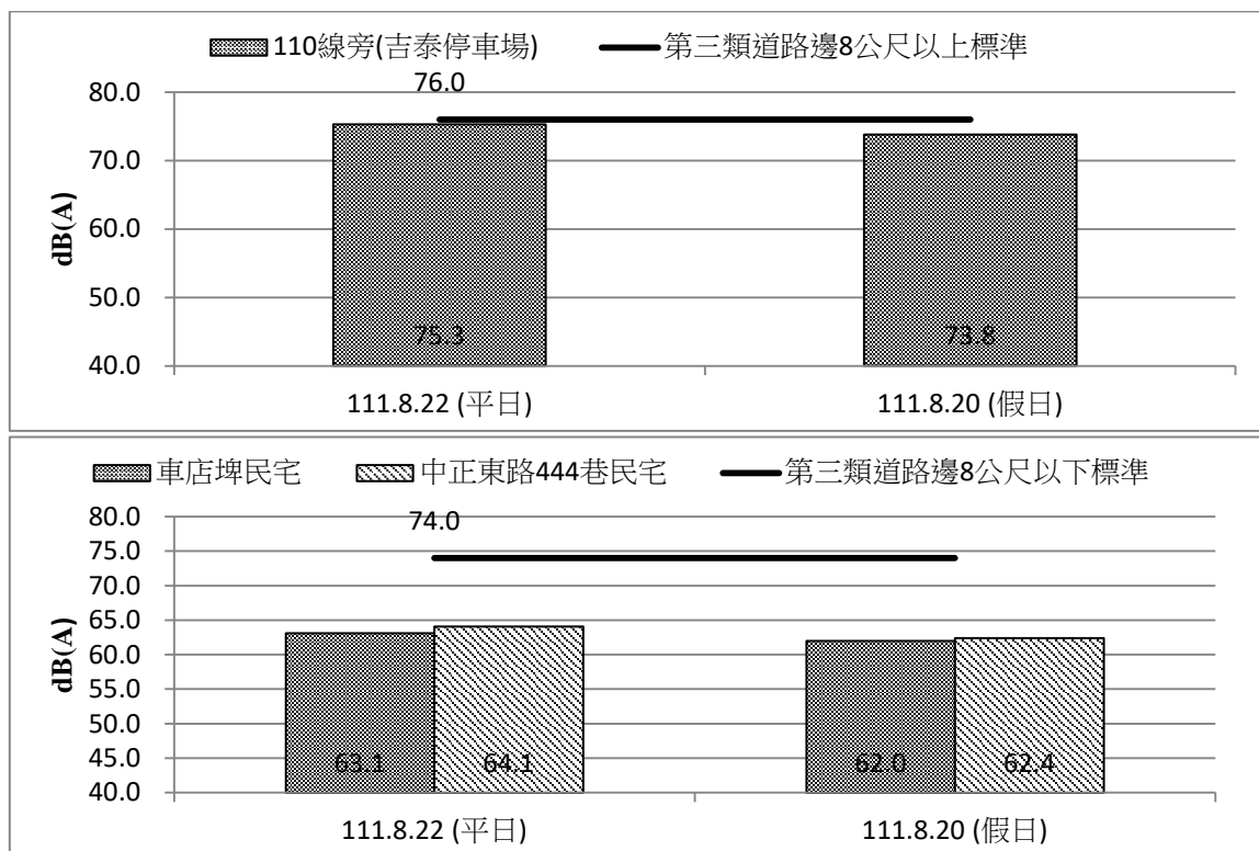
圖 2.2-1 施工期間環境噪音 L_{eq} 監測成果比較圖(111 年 7 月~9 月)
