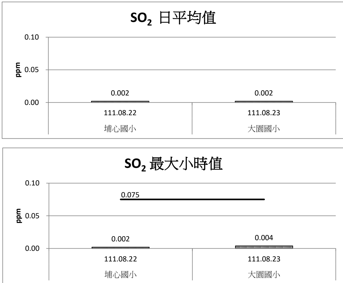
圖 2.1-4 施工期間空氣品質 SO 2 監測成果比較圖(111 年 7 月~9 月)
