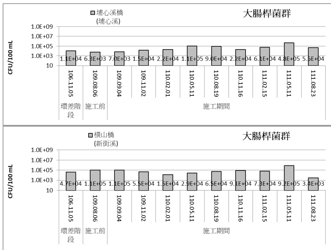
圖 3.1.6-11 計畫區周邊歷次河川水質大腸桿菌群監測成果
