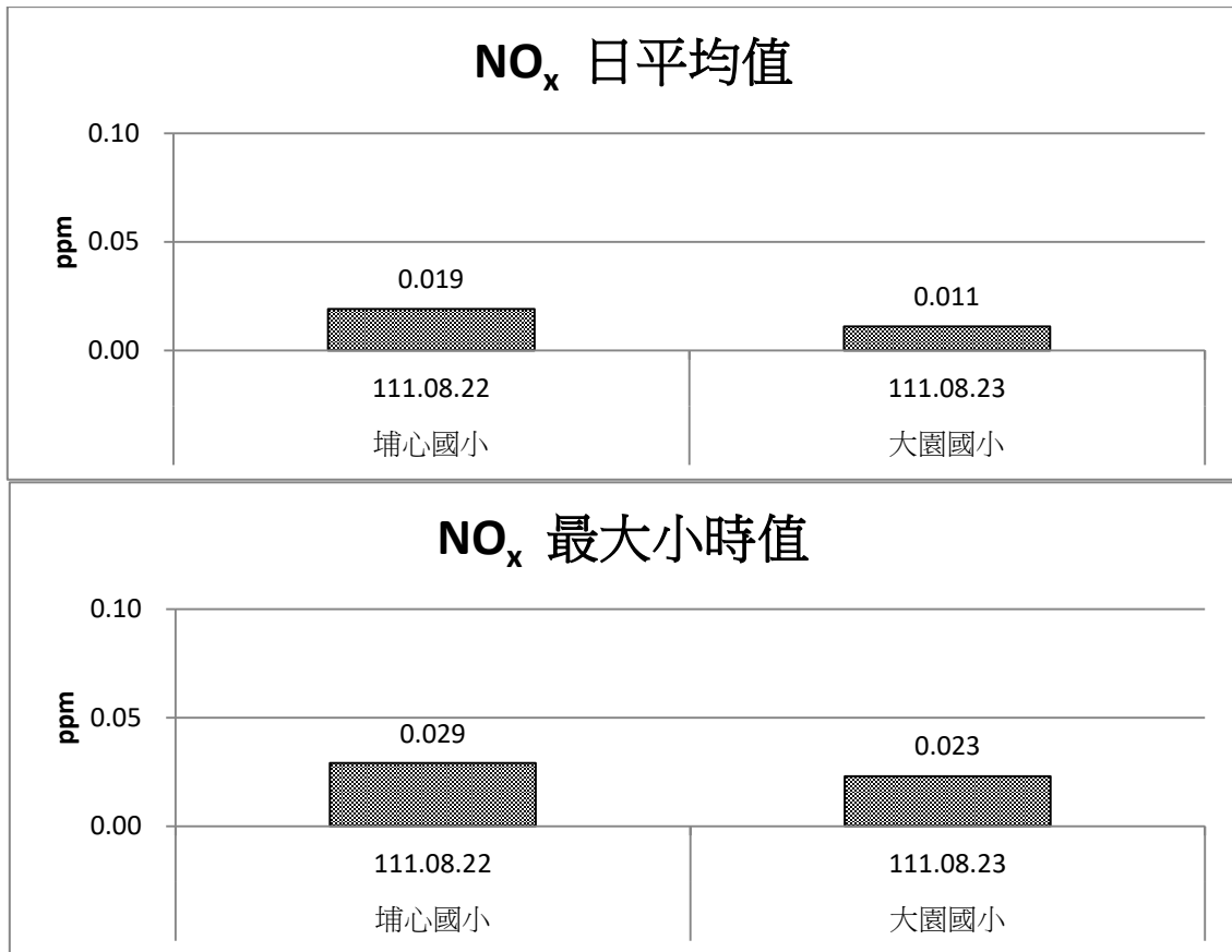
圖 2.1-10 施工期間空氣品質 NO x 監測成果比較圖(111 年 7 月~9 月)
