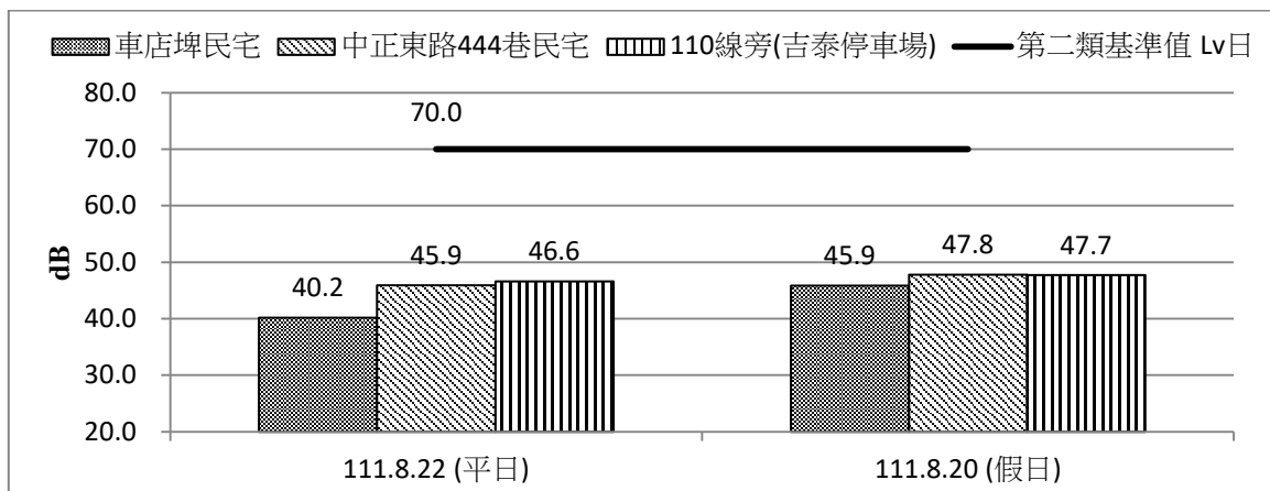
圖 2.2-4 施工期間環境振動 L_{v10日} 監測成果比較圖(111 年 7 月~9 月)
