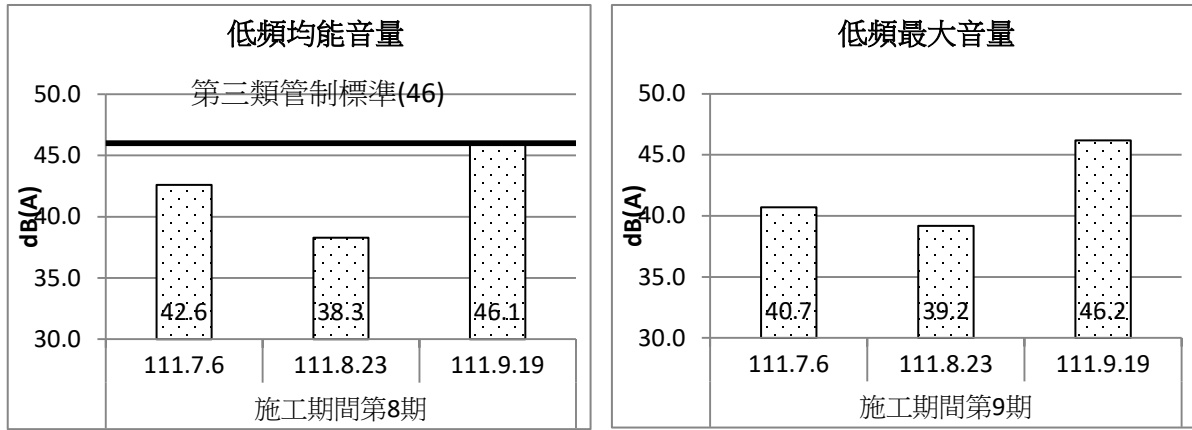
圖 2.3-1 施工期間第 9 期低頻噪音監測成果比較(111 年 7 月~9 月)
