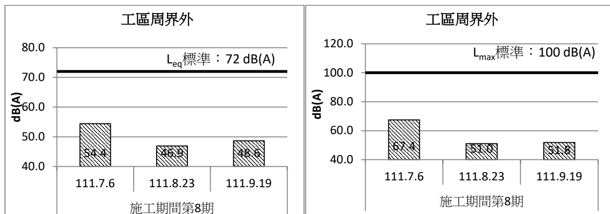
圖 2.4-1 施工期間第 9 期營建噪音監測成果比較圖(111 年 7 月~9 月)
