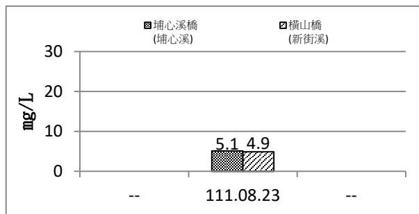
圖 2.5-8 施工期間第 9 期(111 年 7 月~9 月) 河川水質 BOD 5 監測成果圖
