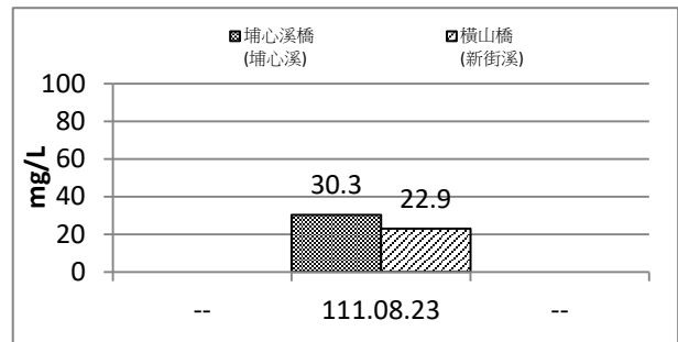
圖 2.5-10 施工期間第 9 期(111 年 7 月~9 月) 河川水質化學需氧量監測成果圖
