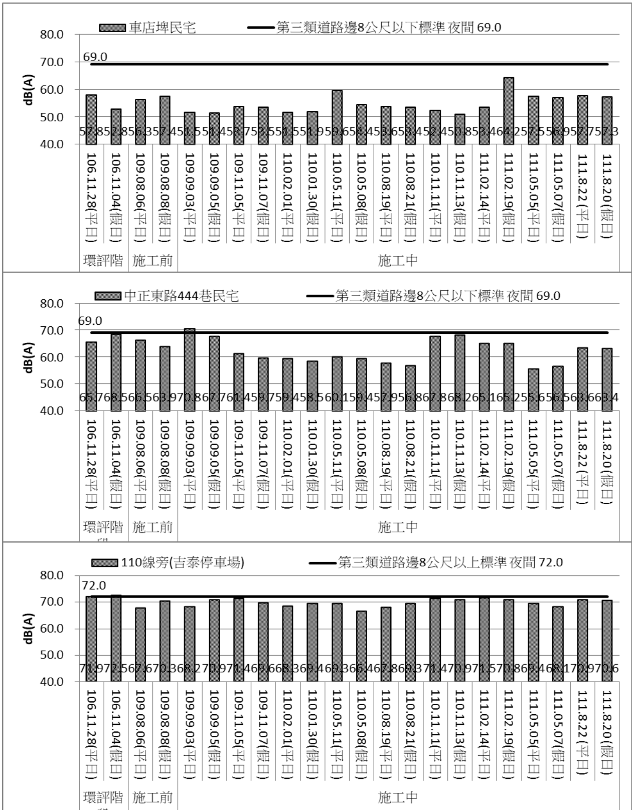
圖 3.1.3-3 計畫區周邊歷次環境噪音 L max 監測成果
