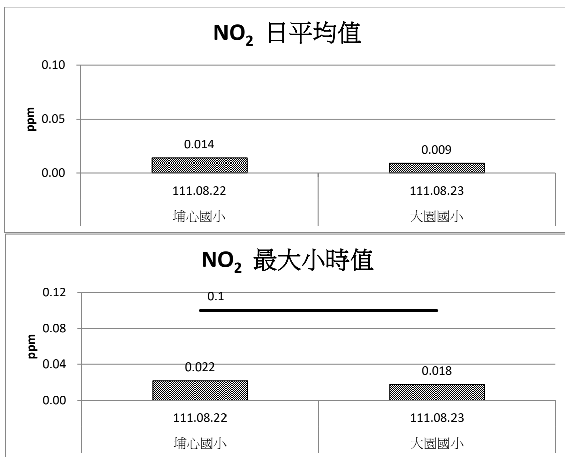
圖 2.1-8 施工期間空氣品質 NO 2 監測成果比較圖(111 年 7 月~9 月)
