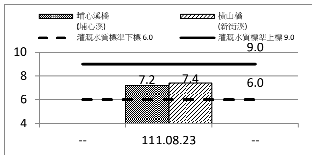
圖 2.5-1 施工期間第 9 期(111 年 7 月~9 月) 河川水質 pH 監測成果圖
