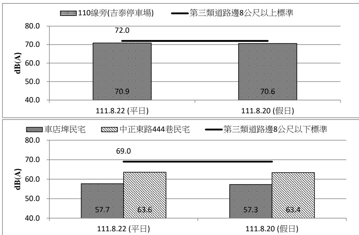
圖 2.2-3 施工期間環境噪音 L eq 監測成果比較圖(111 年 7 月~9 月)
