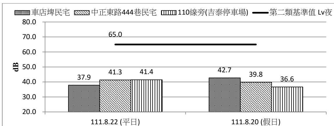
圖 2.2-5 施工期間環境振動 L_{v10夜} 監測成果比較圖(111 年 7 月~9 月)
