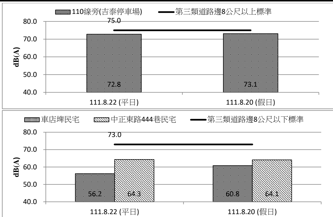
圖 2.2-2 施工期間環境噪音 L eq 監測成果比較圖(111 年 7 月~9 月)
