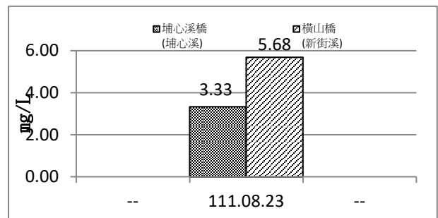
圖 2.5-7 施工期間第 9 期(111 年 7 月~9 月) 河川水質硝酸鹽氮監測成果圖
