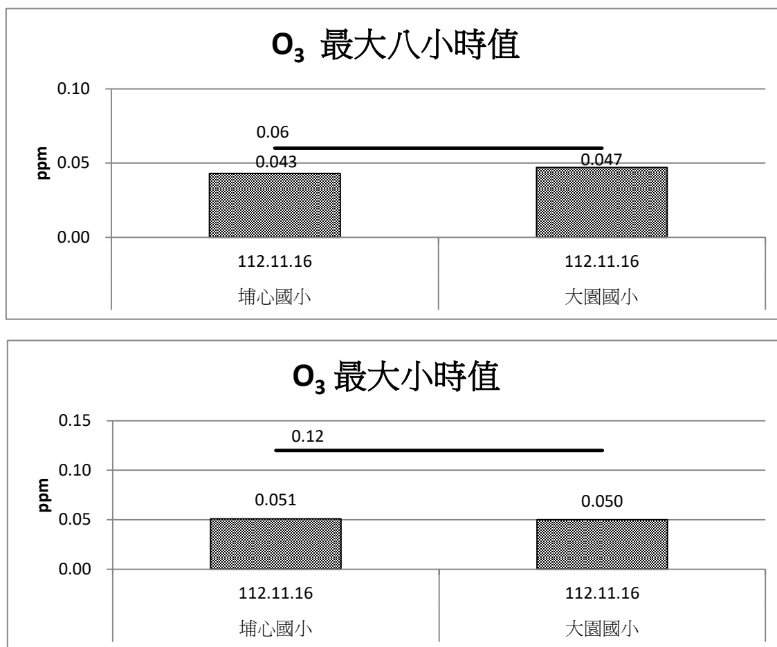
圖 2.1-6 營運期間空氣品質 O 3 監測成果比較圖(112 年 10 月~12 月)
