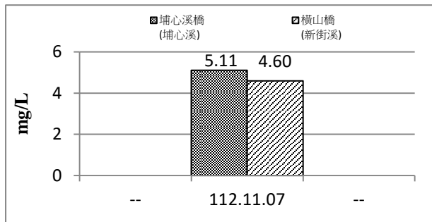
圖 2.3-9 營運期間第 4 期(112 年 10 月~12 月)河川水質氨氮監測成果圖
