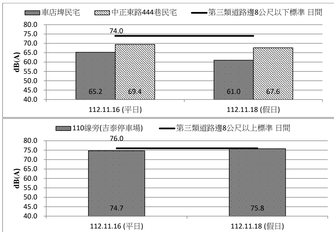
圖 2.2-1 營運期間環境噪音 L_{eq} 監測成果比較圖(112 年 10 月~12 月)
