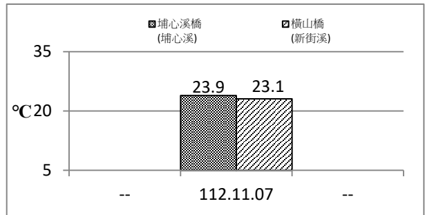
圖 2.3-2 營運期間第 4 期(112 年 10 月~12 月)河川水質水溫監測成果圖
