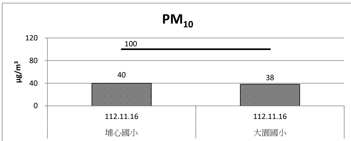
圖 2.1-2 營運期間空氣品質 PM 10 監測成果比較圖(112 年 10 月~12 月)
