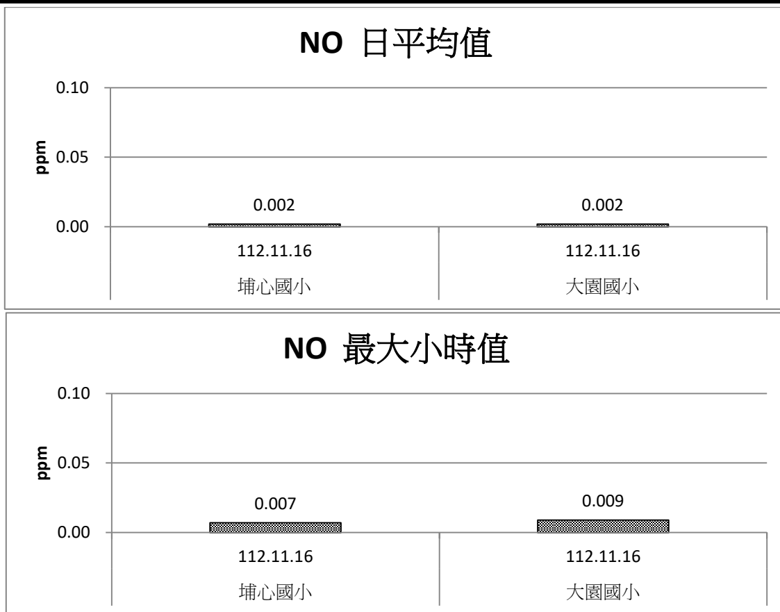
圖 2.1-8 營運期間空氣品質 NO 監測成果比較圖(112 年 10 月~12 月)
