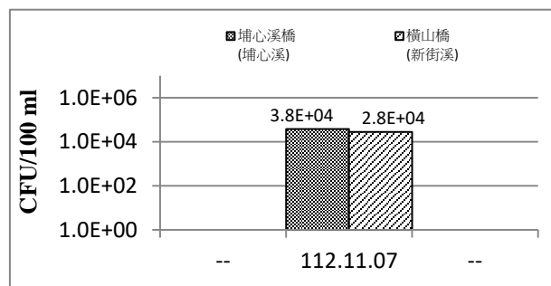
圖 2.3-11 營運期間第 4 期(112 年 10 月~12 月)河川水質大腸桿菌群監測成果圖
