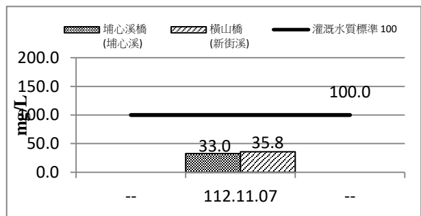
圖 2.3-6 營運期間第 4 期(112 年 10 月~12 月)河川水質懸浮固體監測成果圖
