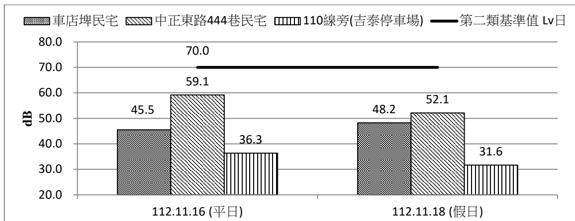
圖 2.2-4 營運期間環境振動 L_{v10日} 監測成果比較圖(112 年 10 月~12 月)
