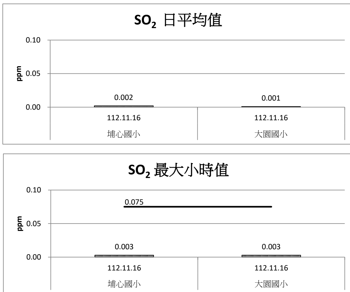
圖 2.1-4 營運期間空氣品質 SO 2 監測成果比較圖(112 年 10 月~12 月)
