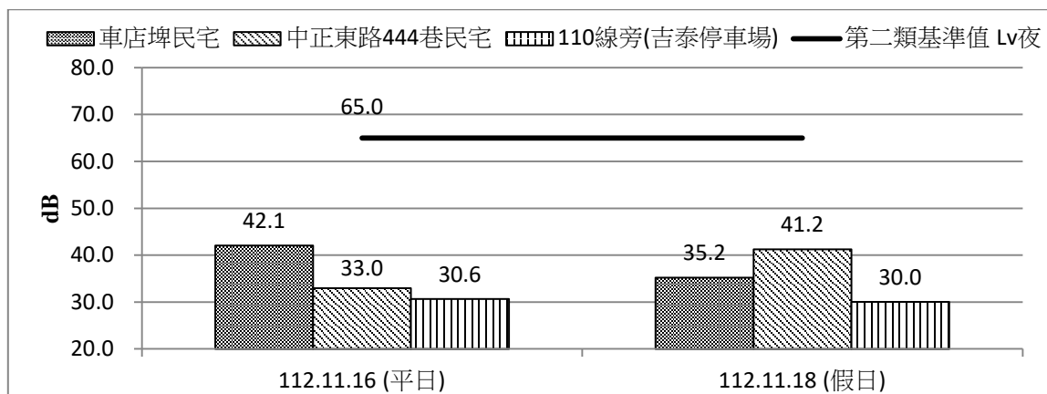
圖 2.2-5 營運期間環境振動 L_{v10夜} 監測成果比較圖(112 年 10 月~12 月)
