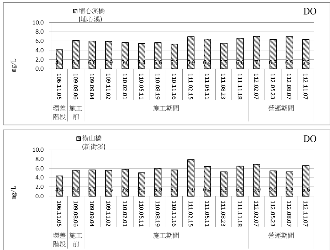
圖 3.1.4-4 計畫區周邊歷次河川水質 DO 監測成果
