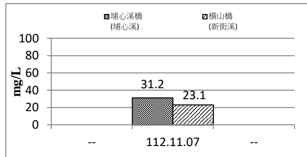
圖 2.3-10 營運期間第 4 期(112 年 10 月~12 月)河川水質化學需氧量監測成果圖
