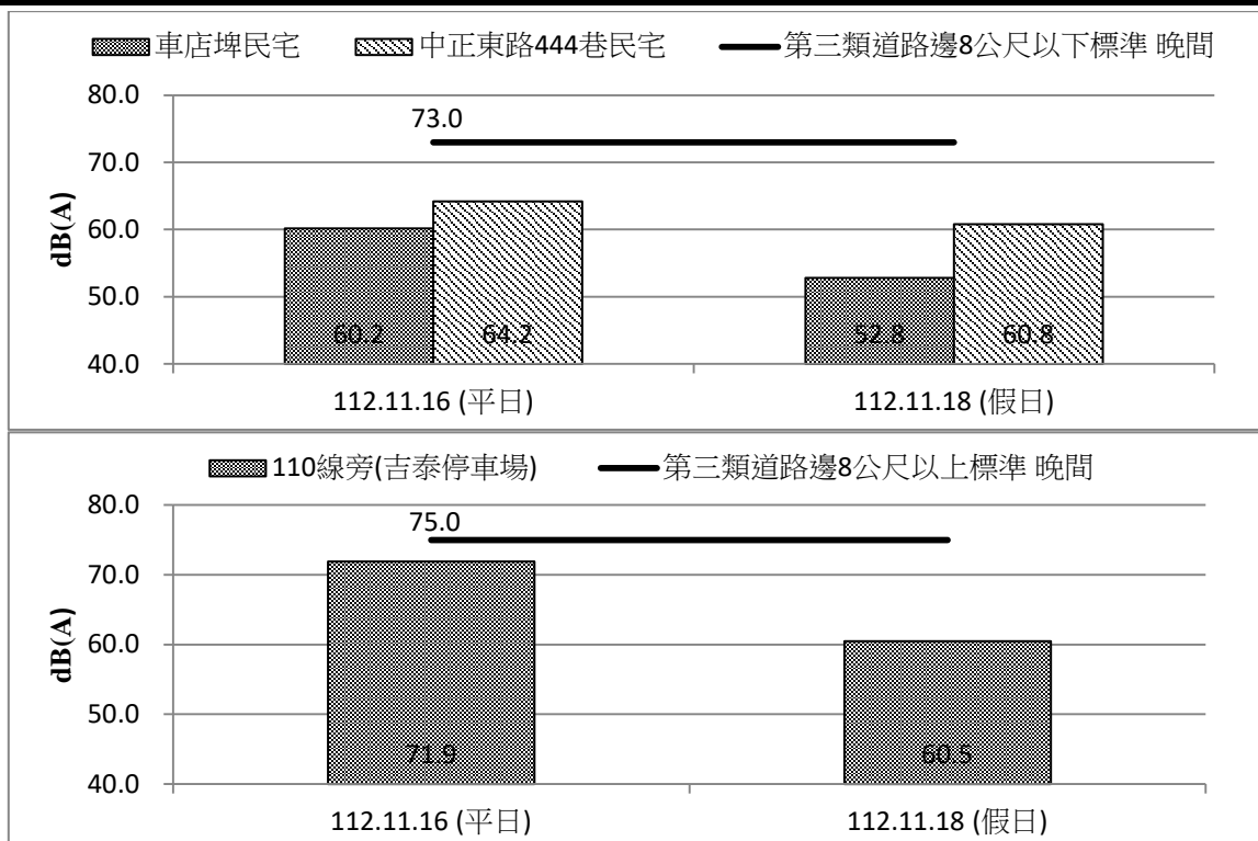
圖 2.2-2 營運期間環境噪音 L w 監測成果比較圖(112 年 10 月~12 月)
