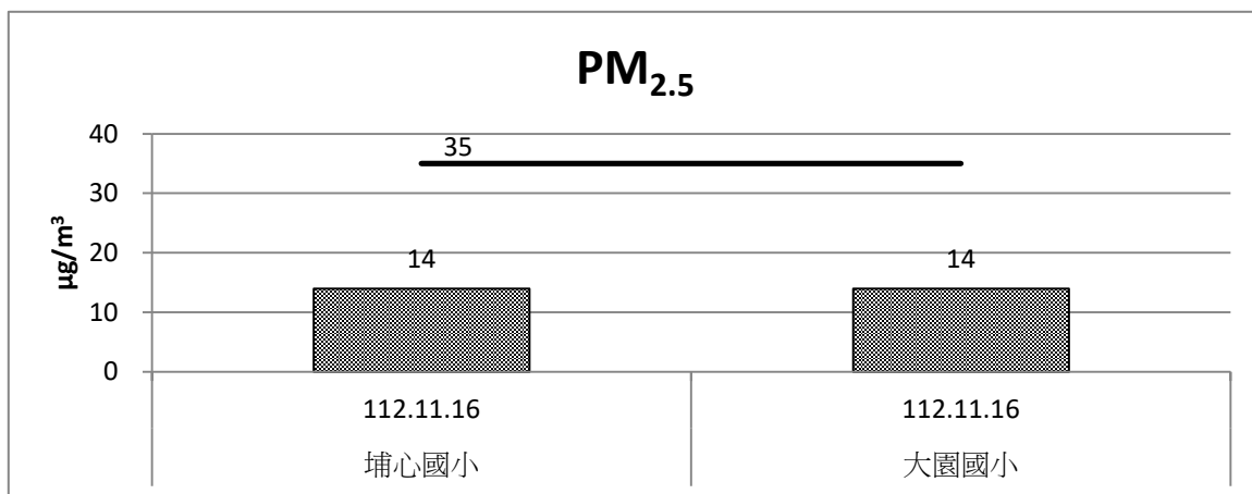
圖 2.1-3 營運期間空氣品質 PM 2.5 監測成果比較圖(112 年 10 月~12 月)
