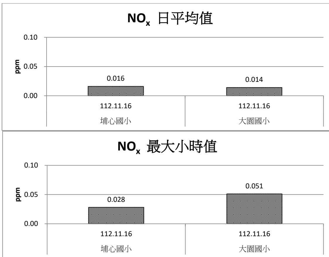
圖 2.1-9 營運期間空氣品質 NO x 監測成果比較圖(112 年 10 月~12 月)
