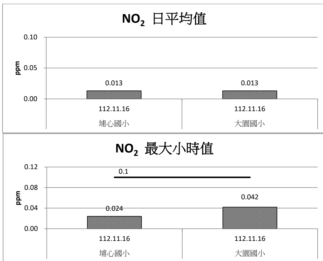
圖 2.1-7 營運期間空氣品質 NO 2 監測成果比較圖(112 年 10 月~12 月)
