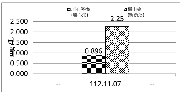
圖 2.3-5 營運期間第 4 期(112 年 10 月~12 月)河川水質總磷監測成果圖
