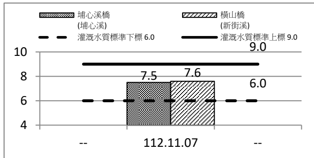
圖 2.3-1 營運期間第 4 期(112 年 10 月~12 月)河川水質 pH 監測成果圖
