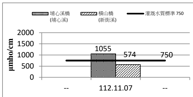
圖 2.3-3 營運期間第 4 期(112 年 10 月~12 月)河川水質導電度監測成果圖
