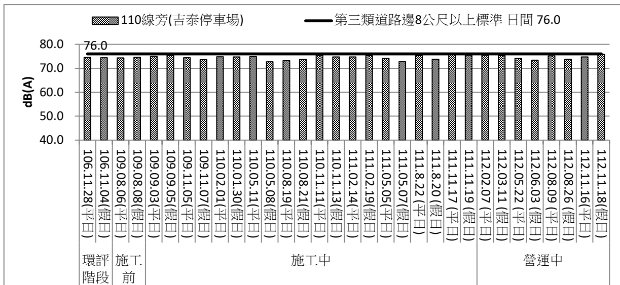
圖 3.1.3-1 計畫區周邊歷次環境噪音 L d 監測成果
