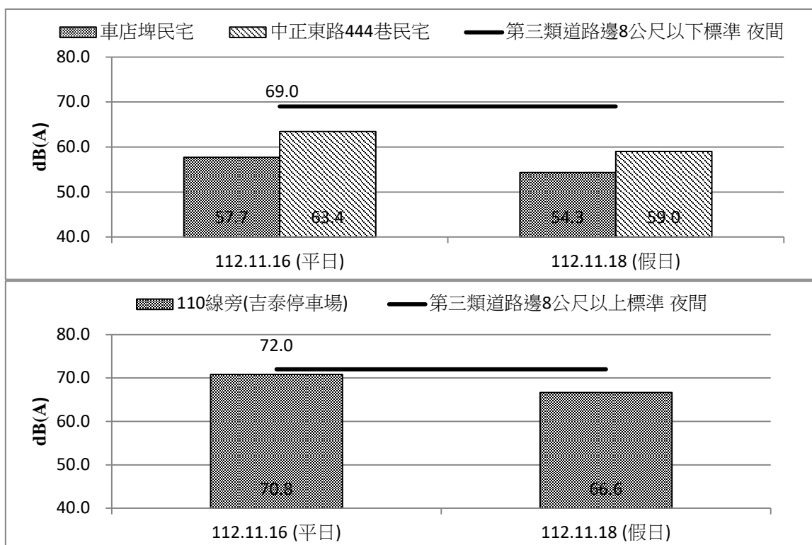
圖 2.2-3 營運期間環境噪音 L w 監測成果比較圖(112 年 10 月~12 月)
