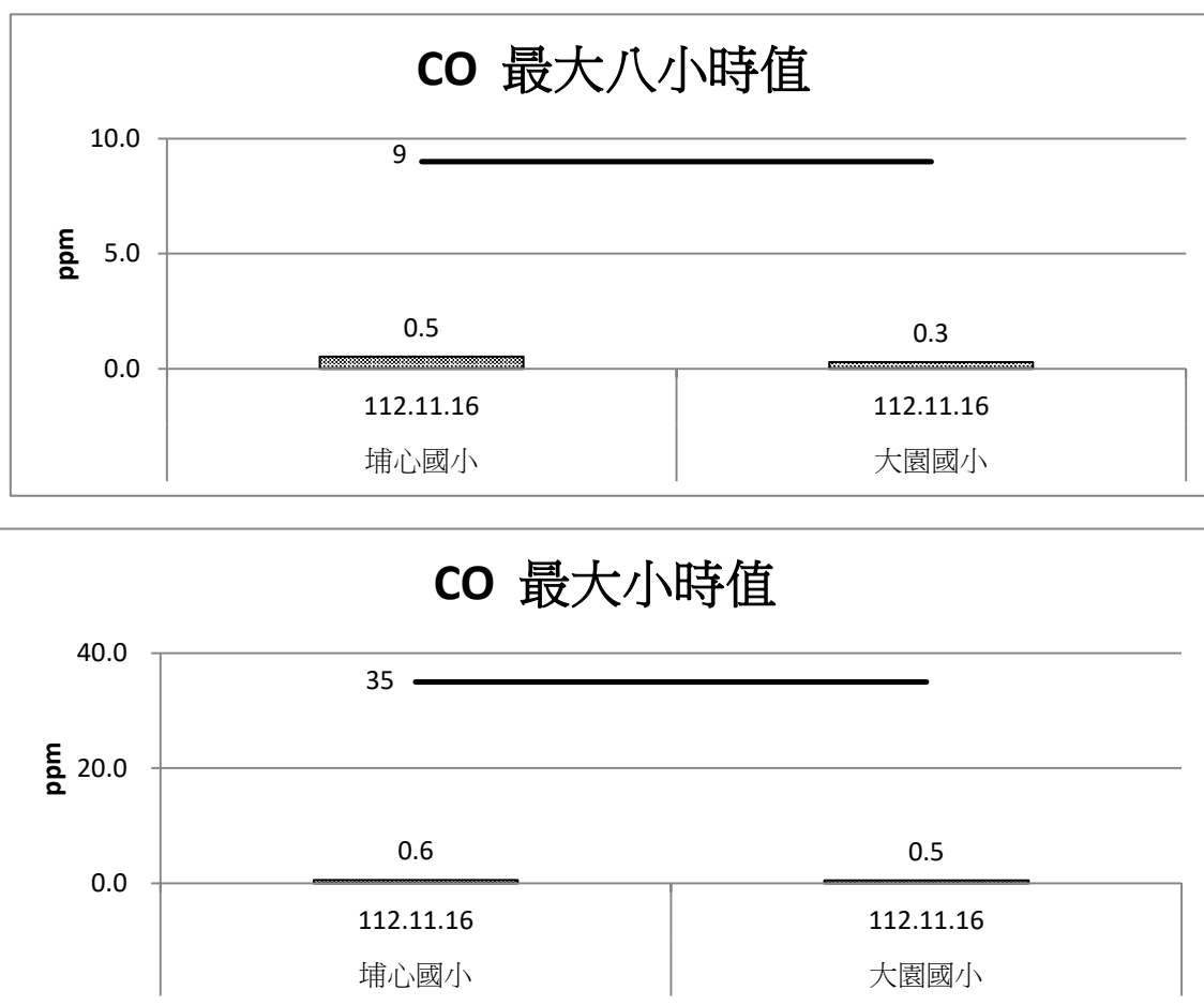
圖 2.1-5 營運期間空氣品質 CO 監測成果比較圖(112 年 10 月~12 月)
