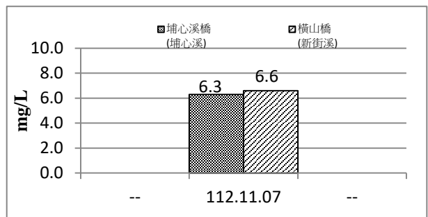
圖 2.3-4 營運期間第 4 期(112 年 10 月~12 月)河川水質溶氧監測成果圖
