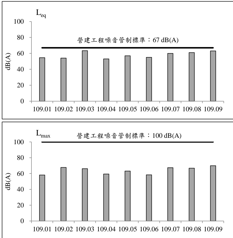
圖 2.6-1 歷次營建噪音監測之各項測值變化圖
