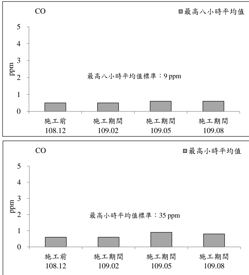
圖 2.1-3 南興路二段 52 巷測站歷次空氣品質監測之各項測值變化圖 (續 2)
