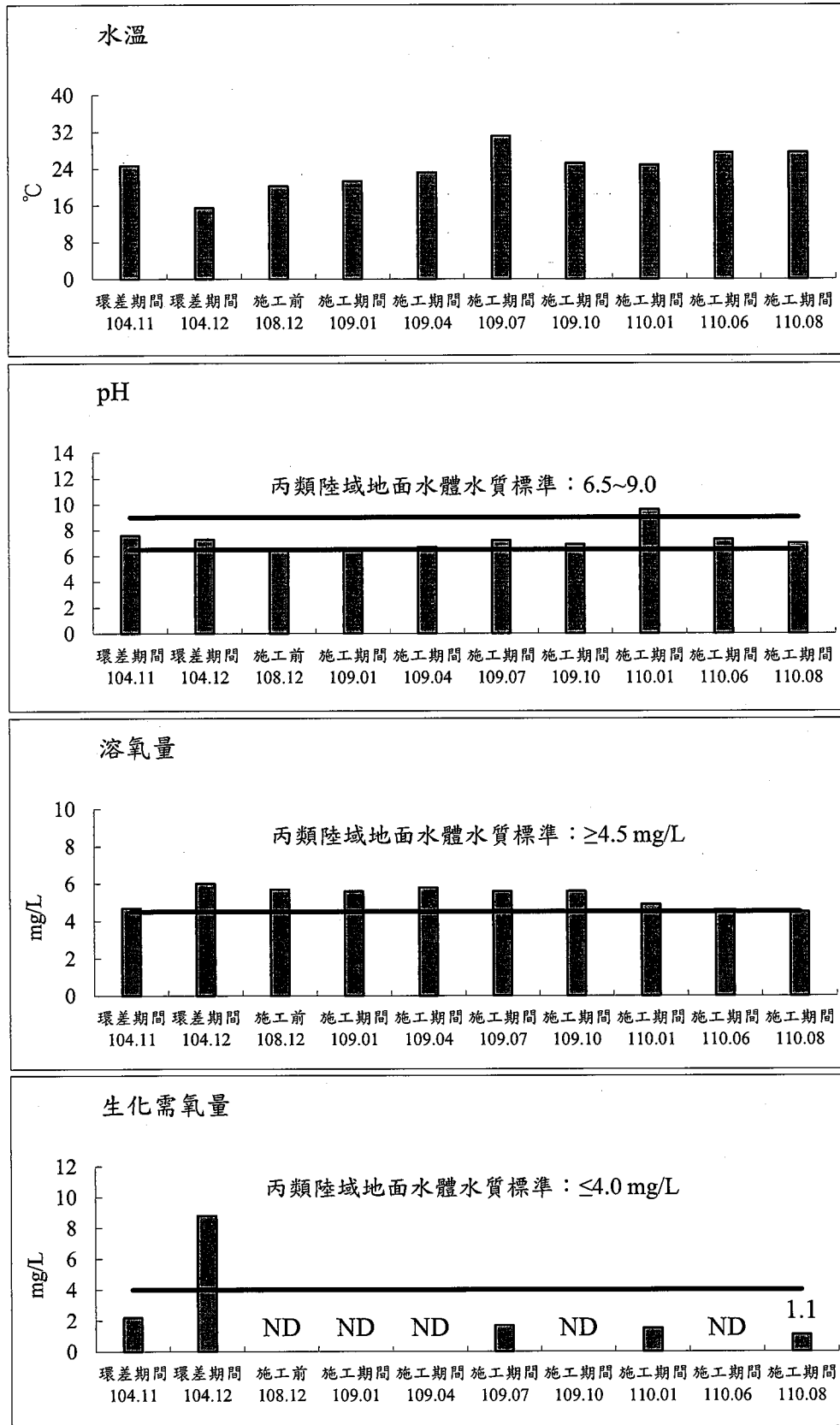
圖 2.3-1 茄苳溪測站歷次地面水體水質監測之各項測值變化圖
