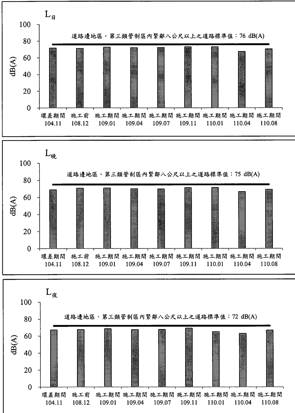
圖 2.2-5 市112線與市112甲線交會口測站歷次噪音監測之各項測值變化圖(假日)
