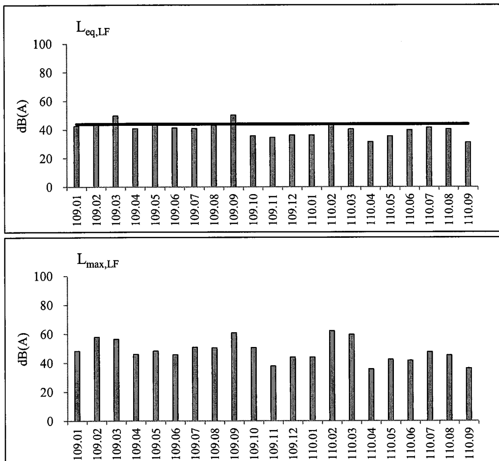
圖 2.6-2 歷次營建低頻噪音監測之各項測值變化圖
