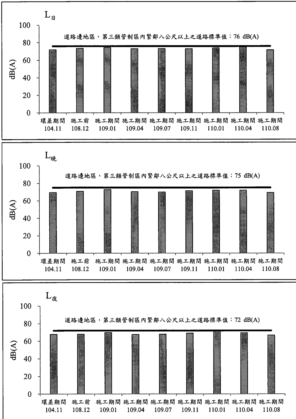
圖 2.2-6 市112線與市112甲線交會口測站歷次噪音監測之各項測值變化圖(平日)
