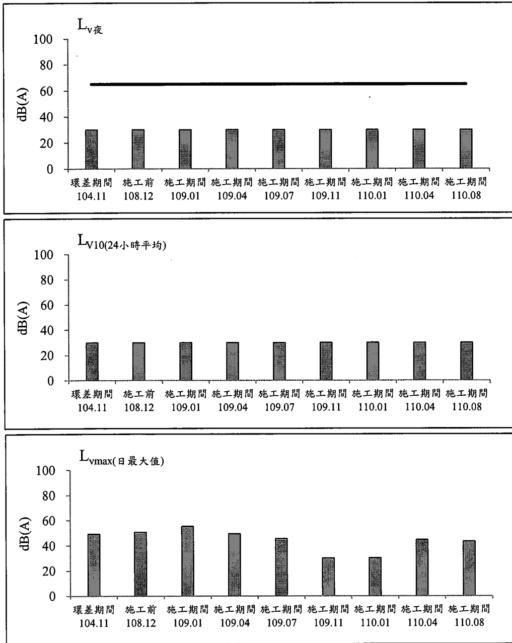
圖 2.2-10 台66線與市112甲線交會口測站歷次振動監測之各項測值變化圖(平日)
