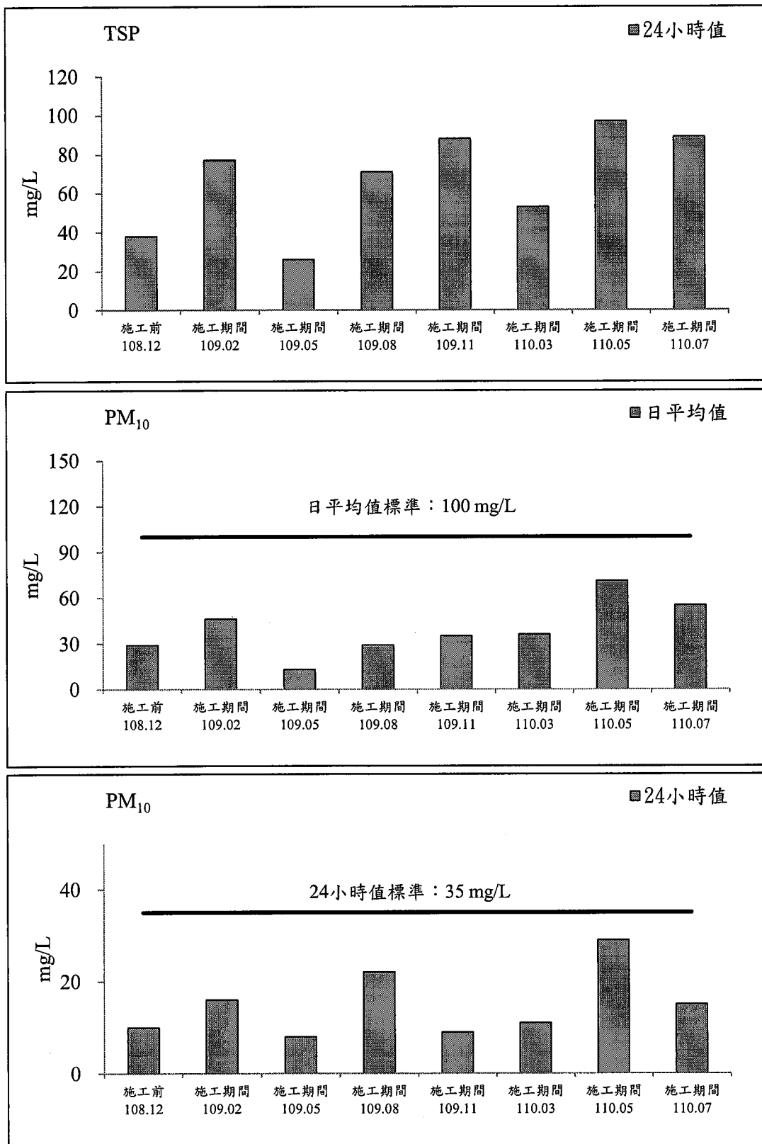
圖 2.1-3 南興路二段 52 巷測站歷次空氣品質監測之各項測值變化圖
