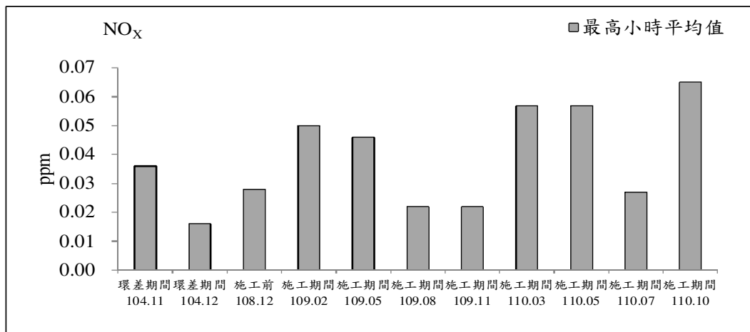
圖 2.1-2 永昌宮測站歷次空氣品質監測之各項測值變化圖
