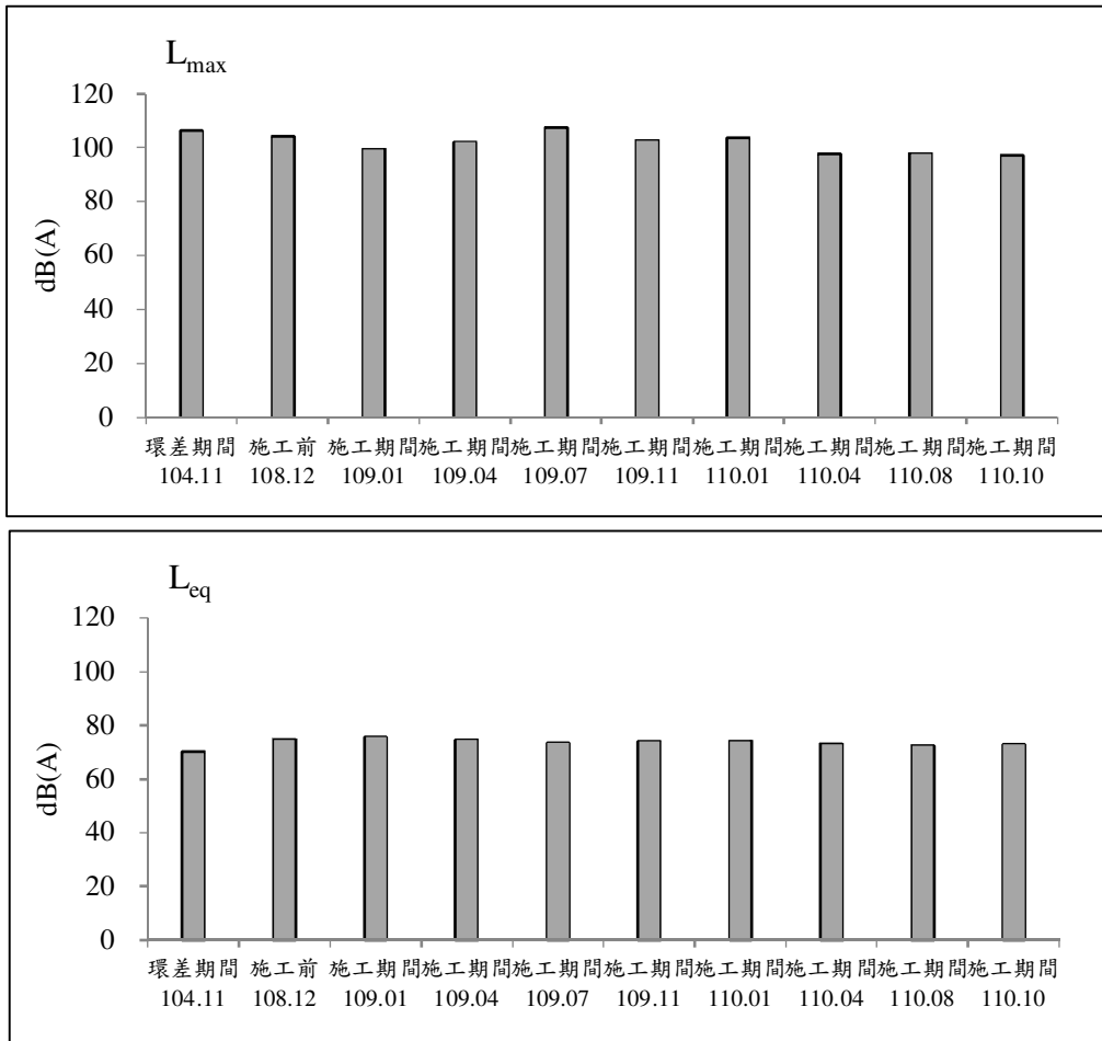
圖 2.2-4 台66線與市112甲線交會口測站歷次噪音監測之各項測值變化圖(平日)(續)
