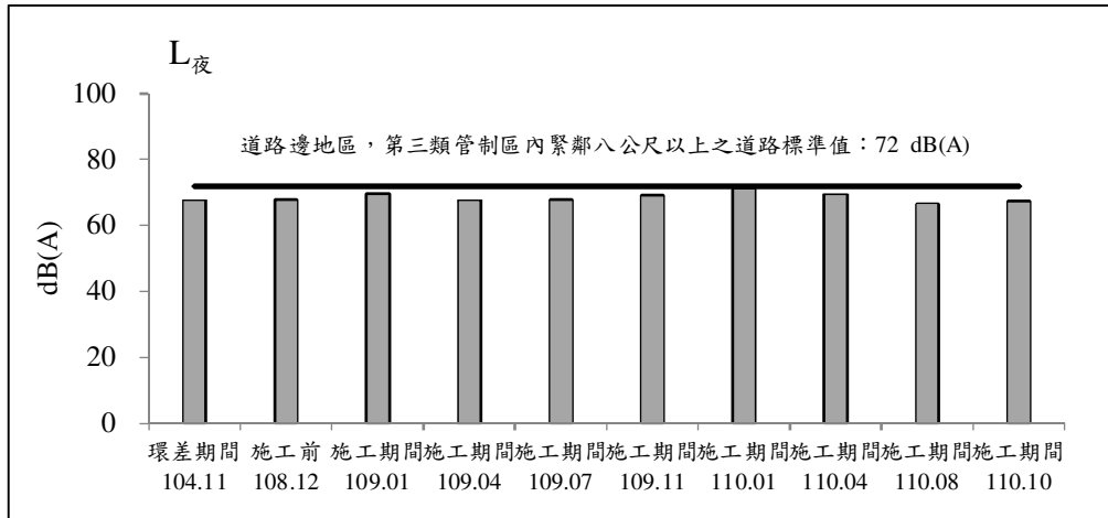
圖 2.2-6 市112線與市112甲線交會口測站歷次噪音監測之各項測值變化圖(平日)
