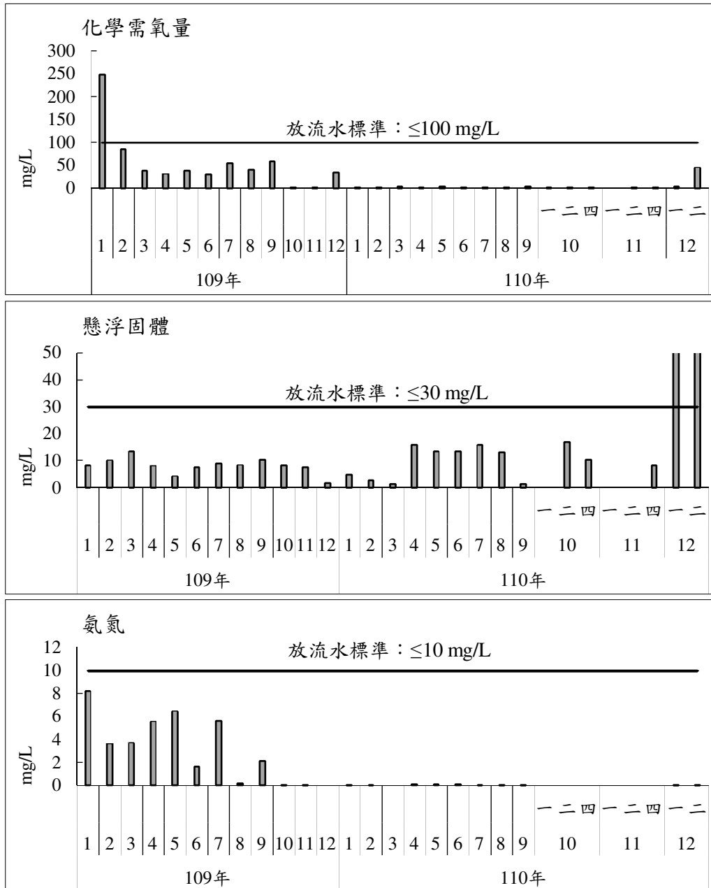
圖 2.7-2 歷次工區放流水監測之各項測值變化圖(續)
