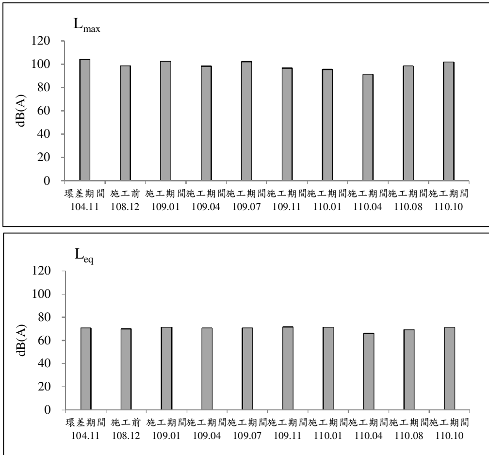
圖 2.2-5 市112線與市112甲線交會口測站歷次噪音監測之各項測值變化圖(假日)(續)
