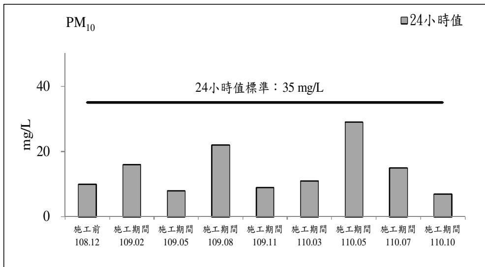
圖 2.1-3 南興路二段 52 巷測站歷次空氣品質監測之各項測值變化圖 (續 3)
