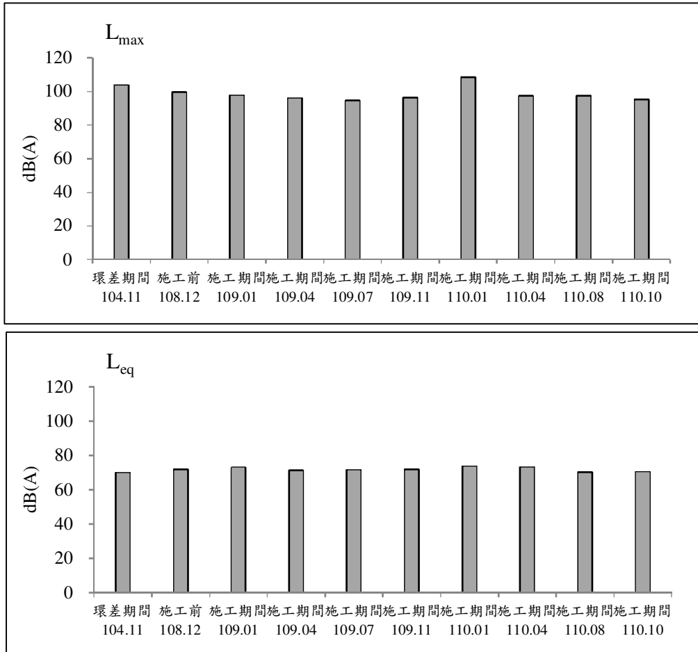
圖 2.2-6 市112線與市112甲線交會口測站歷次噪音監測之各項測值變化圖(平日)(續)
