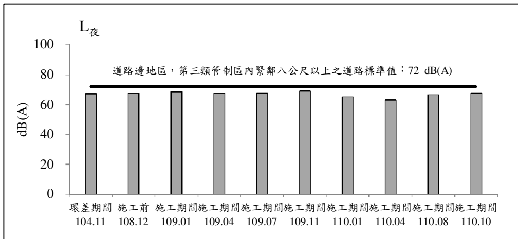
圖 2.2-5 市112線與市112甲線交會口測站歷次噪音監測之各項測值變化圖(假日)
