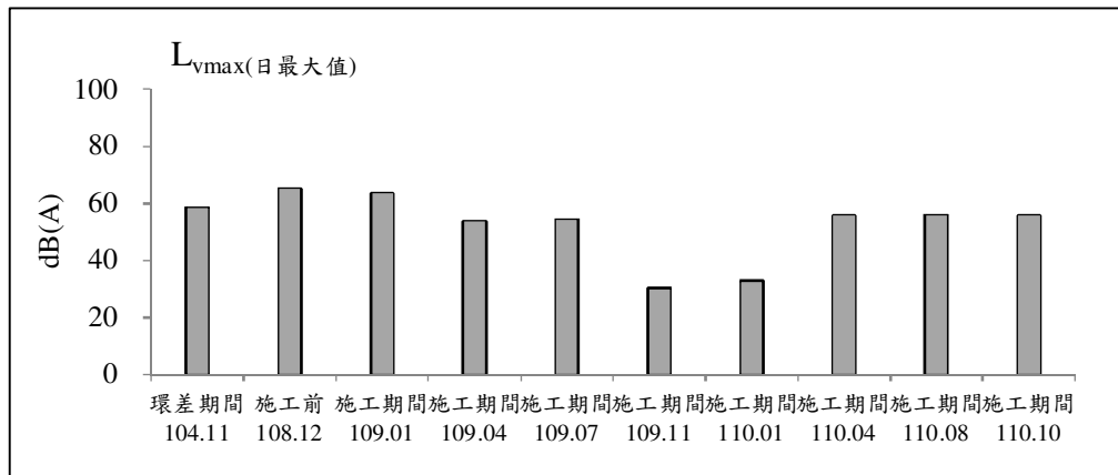
圖 2.2-12 市112線與市112甲線交會口測站歷次振動監測之各項測值變化圖(平日)
