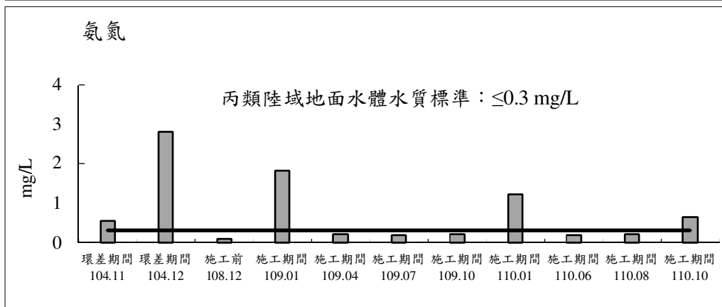
圖 2.3-1 茄苳溪測站歷次地面水體水質監測之各項測值變化圖(續 1)
