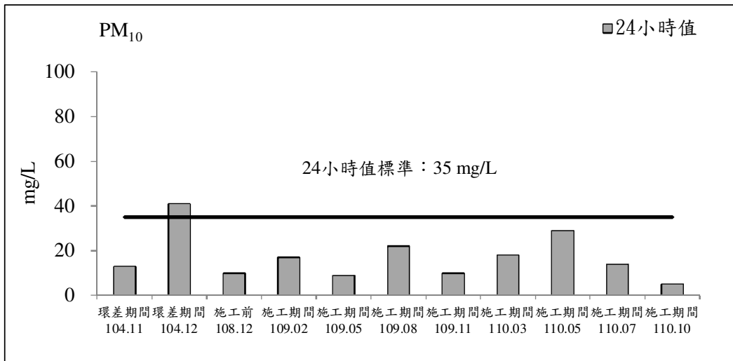
圖 2.1-2 永昌宮測站歷次空氣品質監測之各項測值變化圖(續 3)
