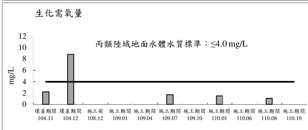
圖 2.3-1 茄苳溪測站歷次地面水體水質監測之各項測值變化圖
