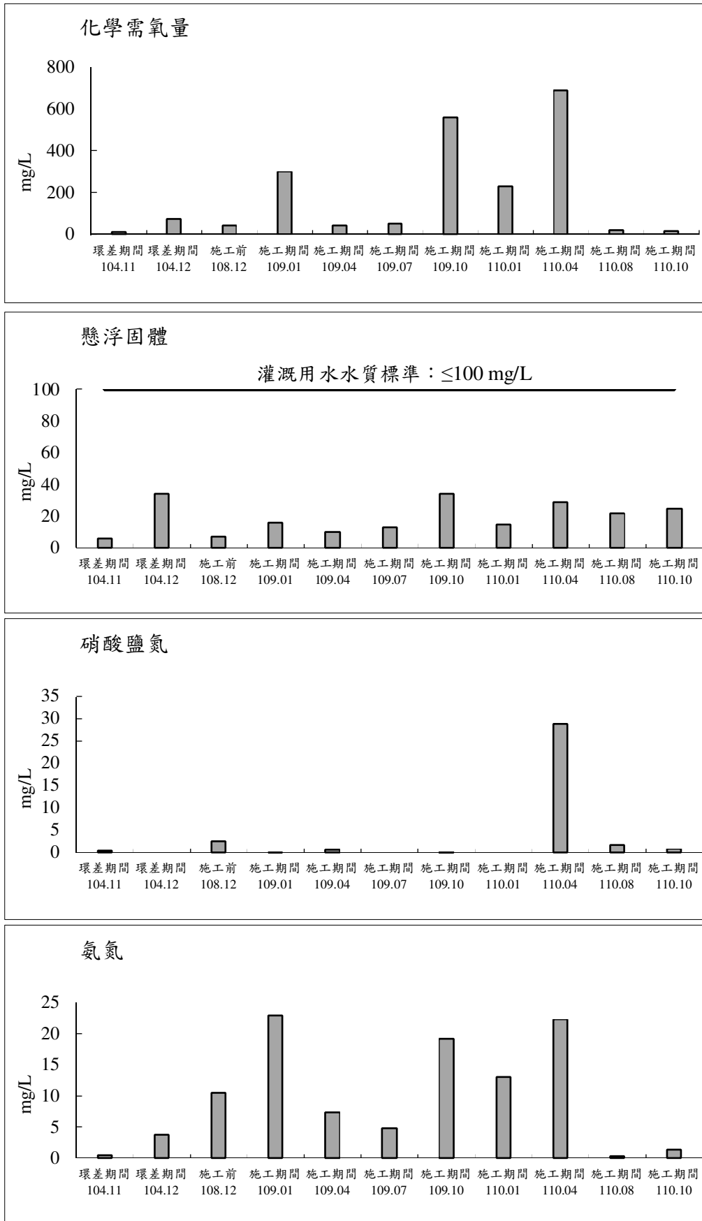
圖 2.3-2 八德分渠(工區上游)測站歷次地面水體水質監測之各項測值變化圖(續 1)
