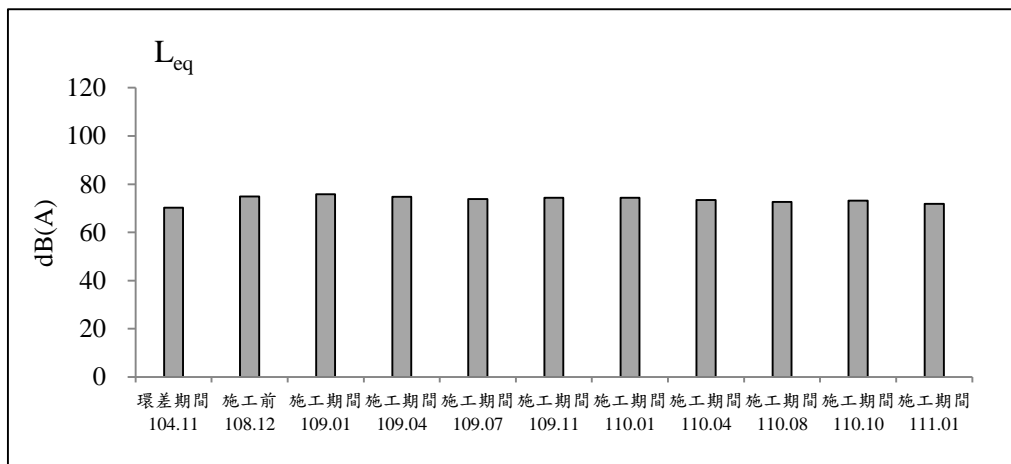
圖 2.2-4 台66線與縣112甲線交會口測站歷次噪音監測之各項測值變化圖(平日)(續)
