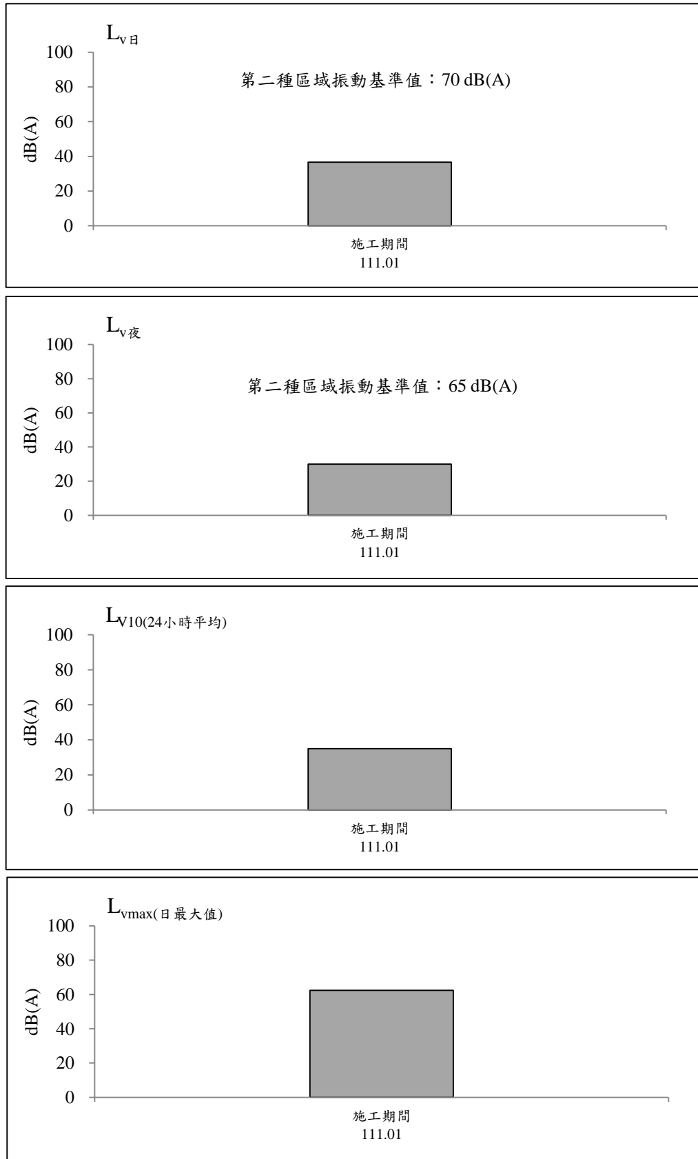
圖 2.2-16 保留戶(南興路二段230號民宅)測站歷次振動監測之各項測值變化圖(假日)
