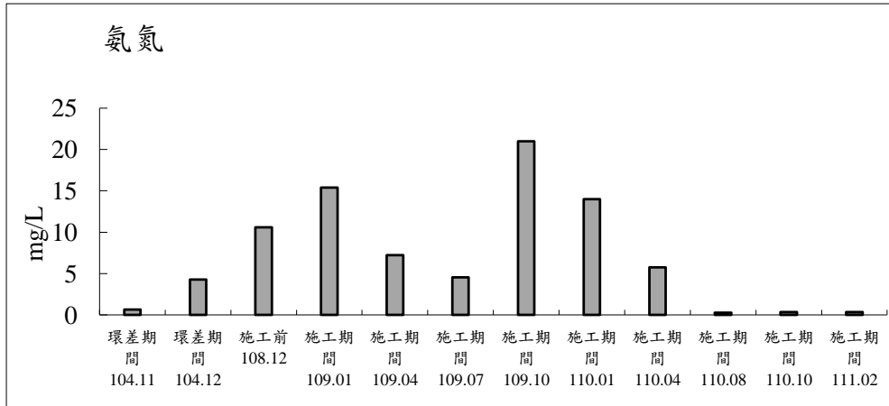
圖 2.3-3 八德分渠(工區下游)測站歷次地面水體水質監測之各項測值變化圖(續 1)
