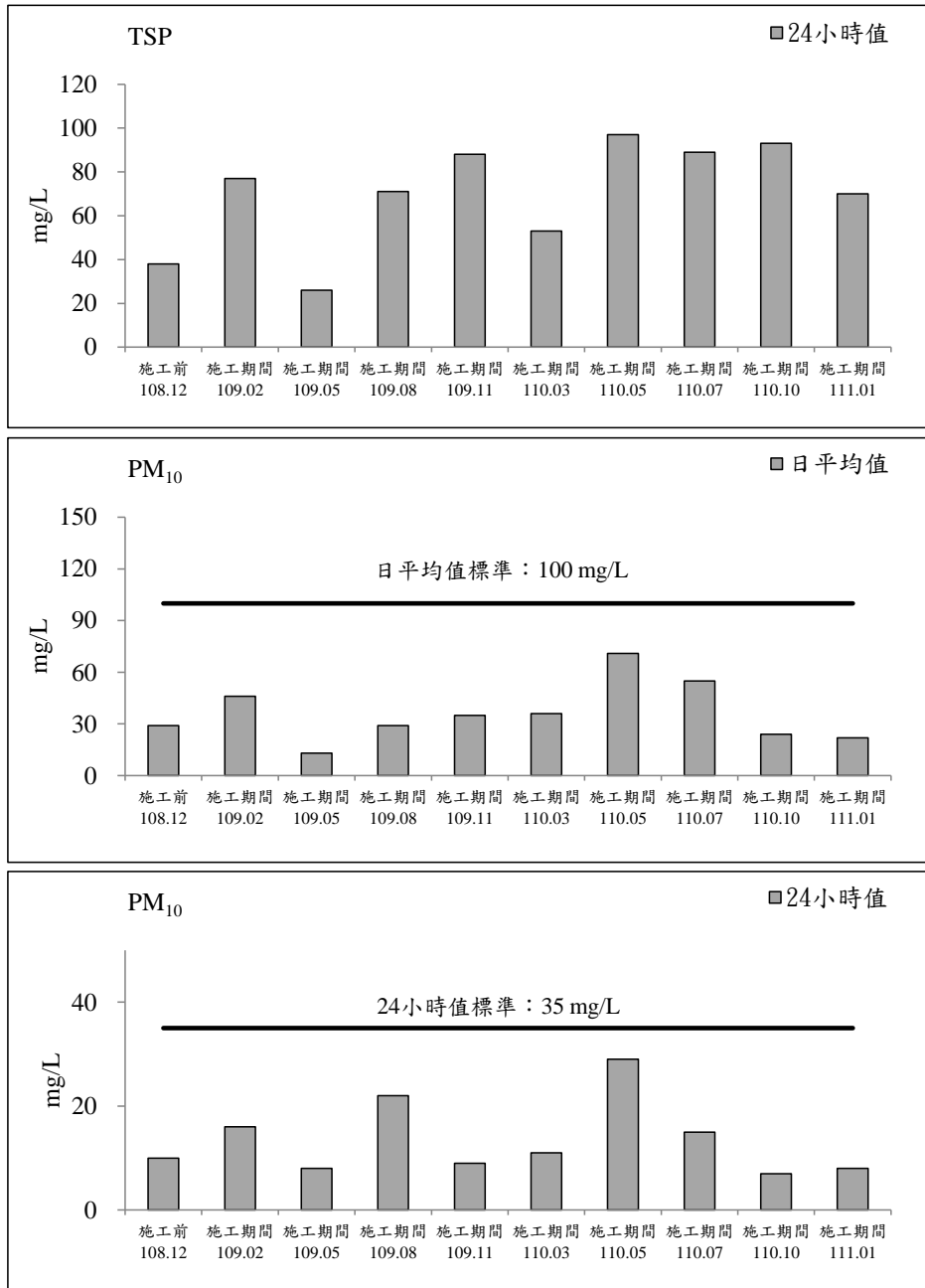
圖 2.1-3 南興路二段 52 巷測站歷次空氣品質監測之各項測值變化圖 (續 3)
