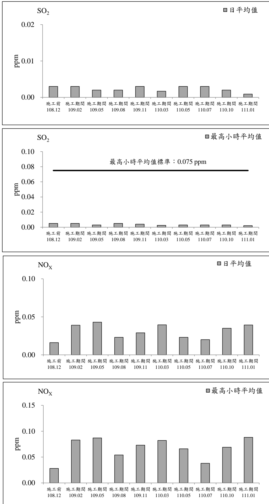
圖 2.1-3 南興路二段 52 巷測站歷次空氣品質監測之各項測值變化圖
