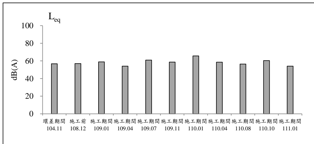
圖 2.2-2 鴻喜鎮社區測站歷次噪音監測之各項測值變化圖(平日)(續)
