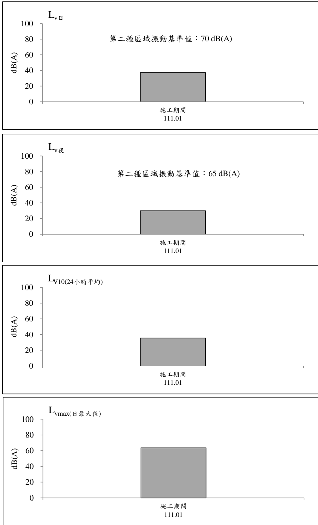
圖 2.2-15 保留戶(南興路二段230號民宅)測站歷次振動監測之各項測值變化圖(假日)
