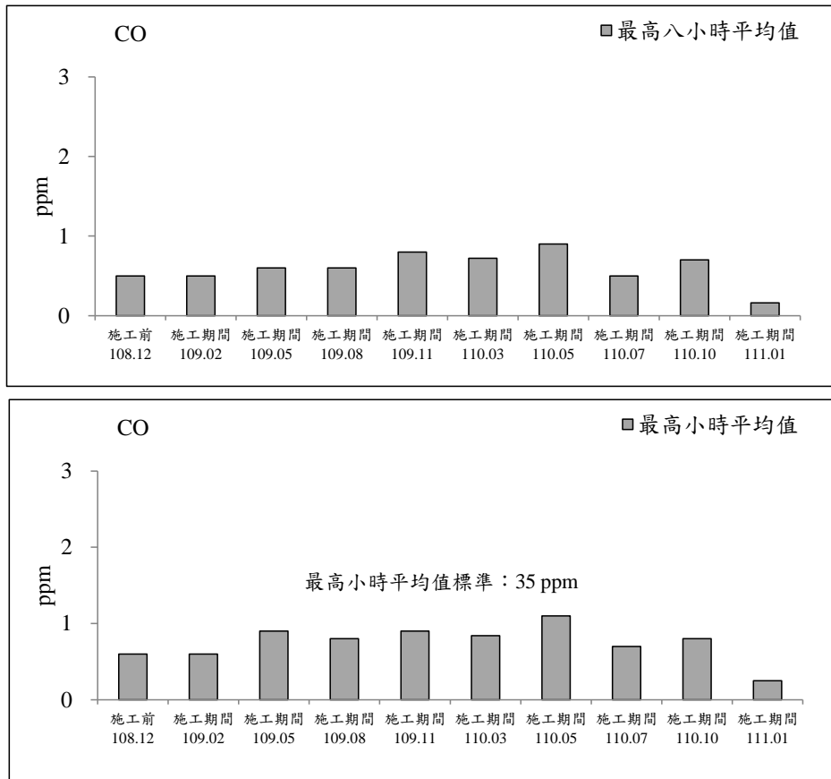
圖 2.1-3 南興路二段 52 巷測站歷次空氣品質監測之各項測值變化圖 (續 2)
