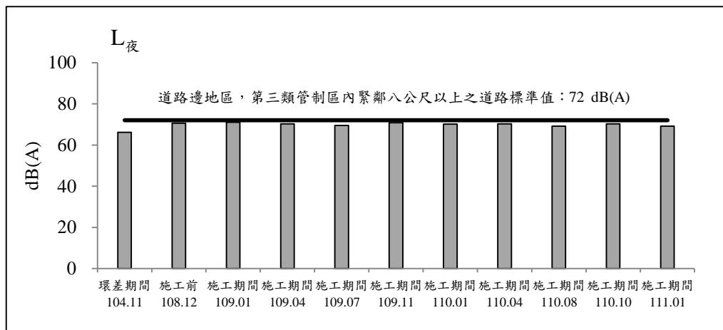
圖 2.2-3 台66線與縣112甲線交會口測站歷次噪音監測之各項測值變化圖(假日)
