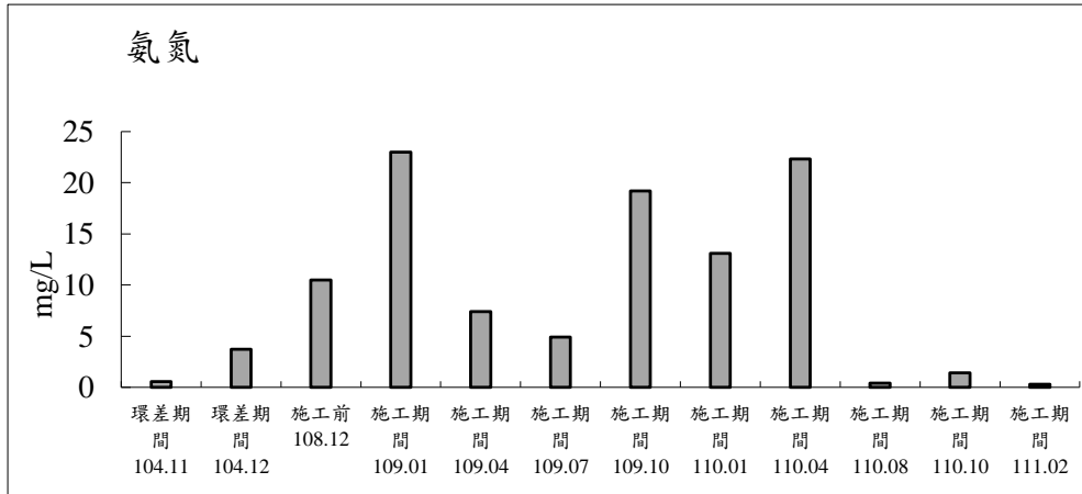
圖 2.3-2 八德分渠(工區上游)測站歷次地面水體水質監測之各項測值變化圖(續 1)
