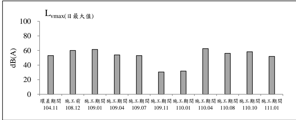
圖 2.2-13 縣112線與縣112甲線交會口測站歷次振動監測之各項測值變化圖(假日)
