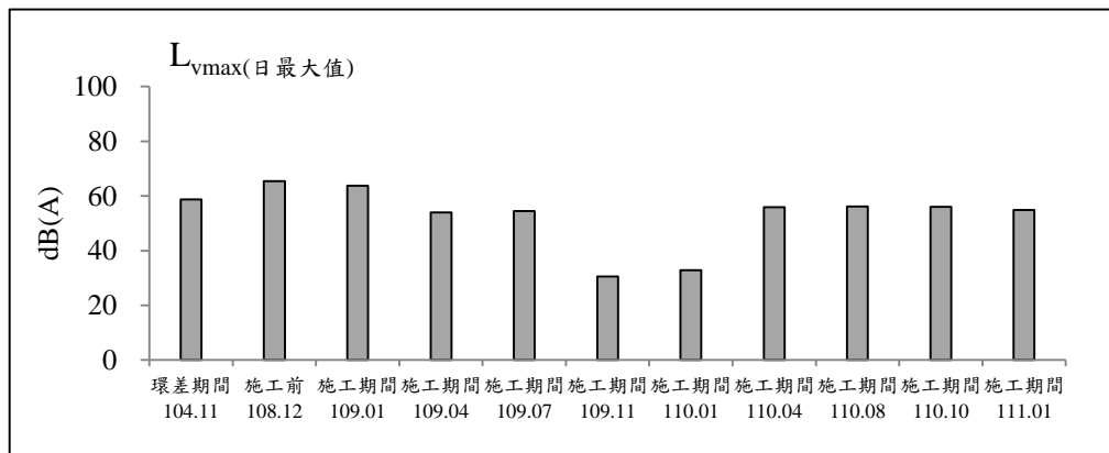
圖 2.2-14 縣112線與縣112甲線交會口測站歷次振動監測之各項測值變化圖(平日)
