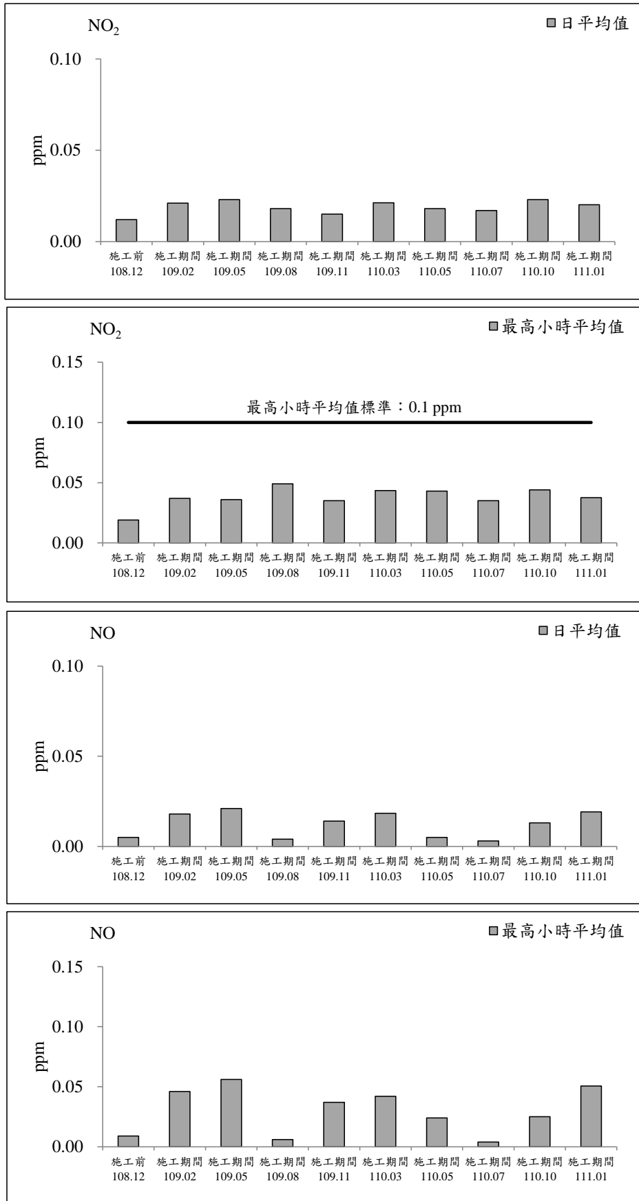
圖 2.1-3 南興路二段 52 巷測站歷次空氣品質監測之各項測值變化圖 (續 1)
