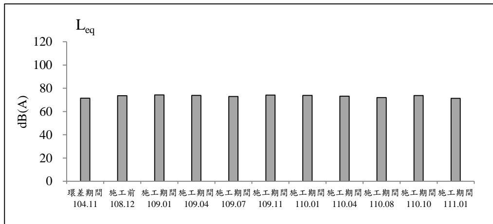
圖 2.2-3 台66線與縣112甲線交會口測站歷次噪音監測之各項測值變化圖(假日)(續)
