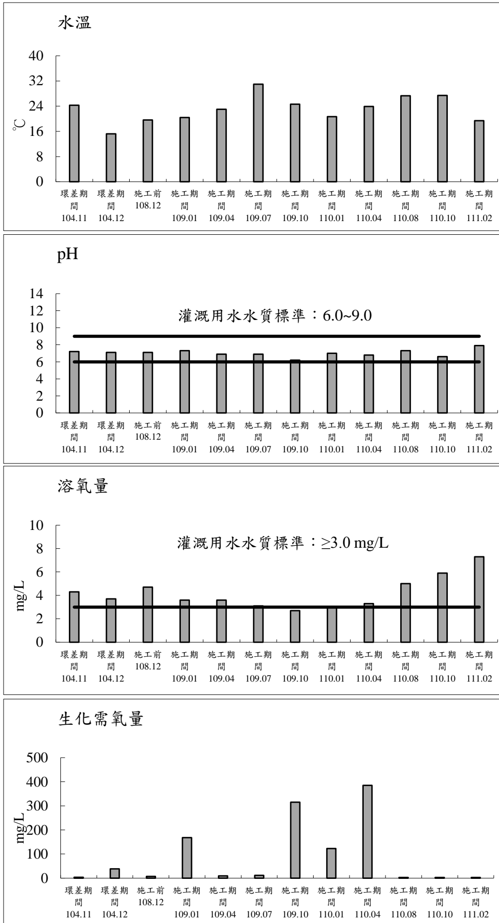
圖 2.3-2 八德分渠(工區上游)測站歷次地面水體水質監測之各項測值變化圖
