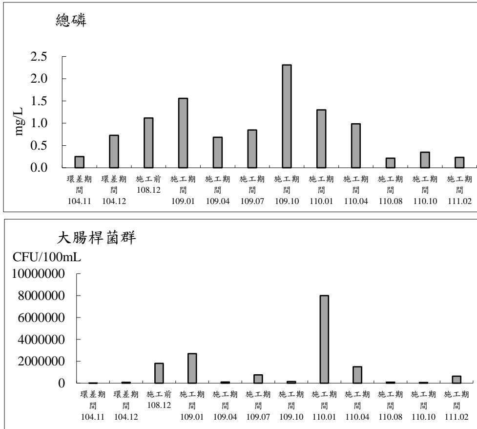
圖 2.3-3 八德分渠(工區下游)測站歷次地面水體水質監測之各項測值變化圖(續 2)
