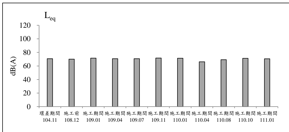
圖 2.2-5 縣112線與縣112甲線交會口測站歷次噪音監測之各項測值變化圖(假日)(續)
