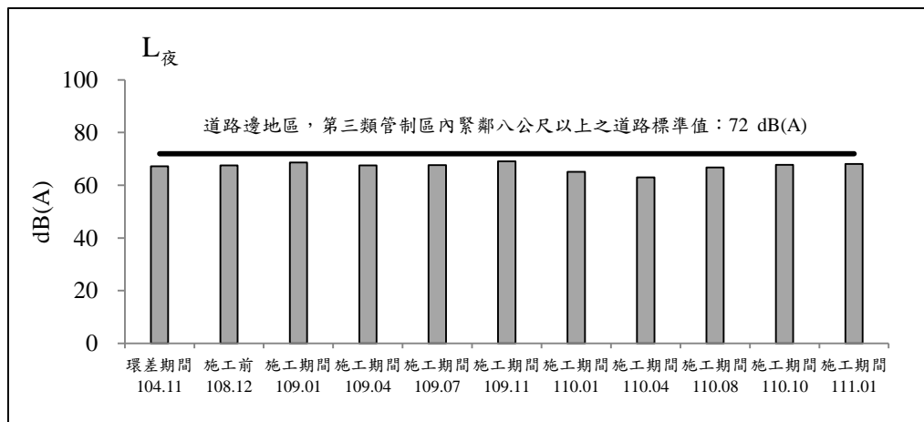
圖 2.2-5 縣112線與縣112甲線交會口測站歷次噪音監測之各項測值變化圖(假日)
