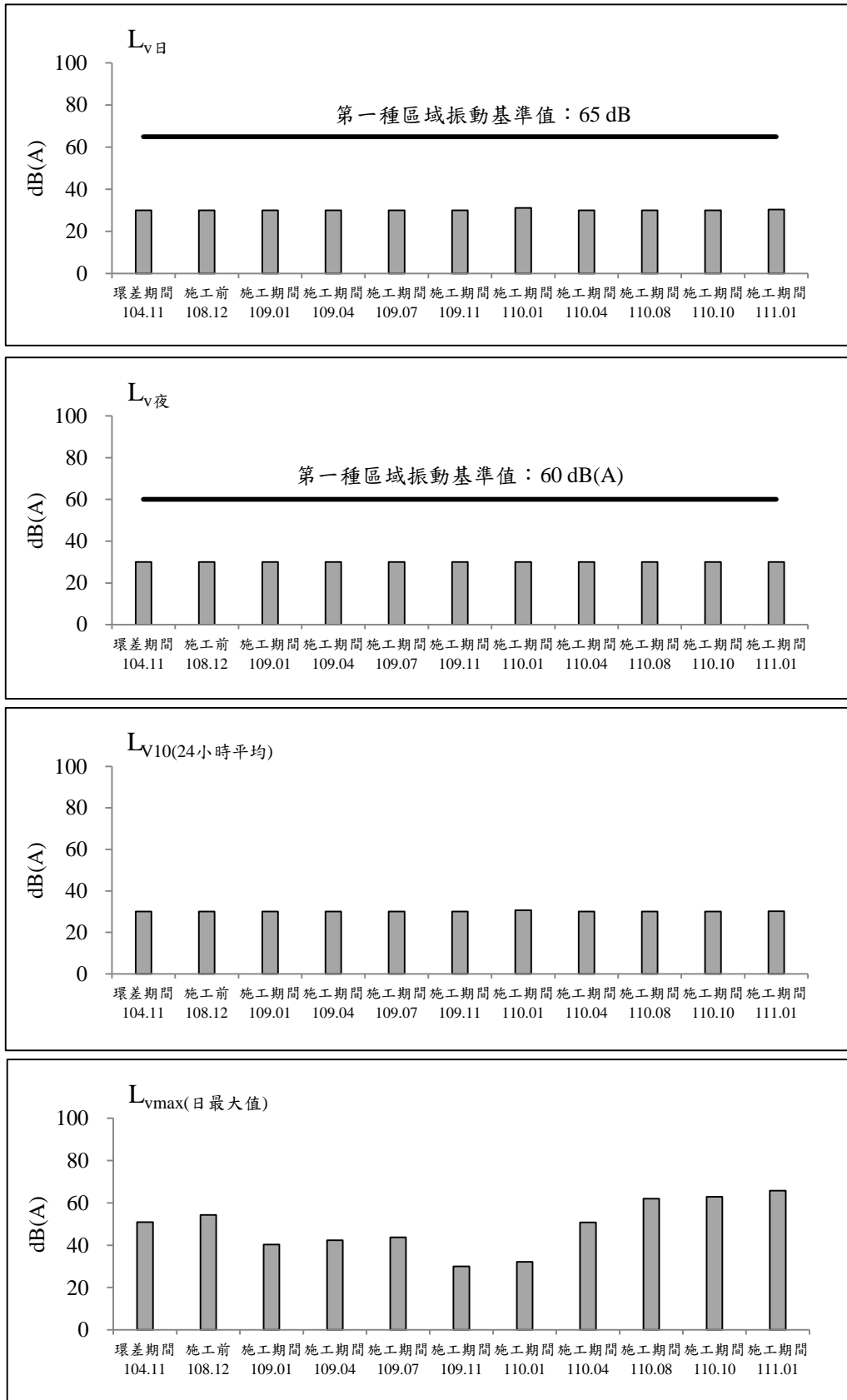
圖 2.2-9 鴻喜鎮社區測站歷次振動監測之各項測值變化圖(假日)
