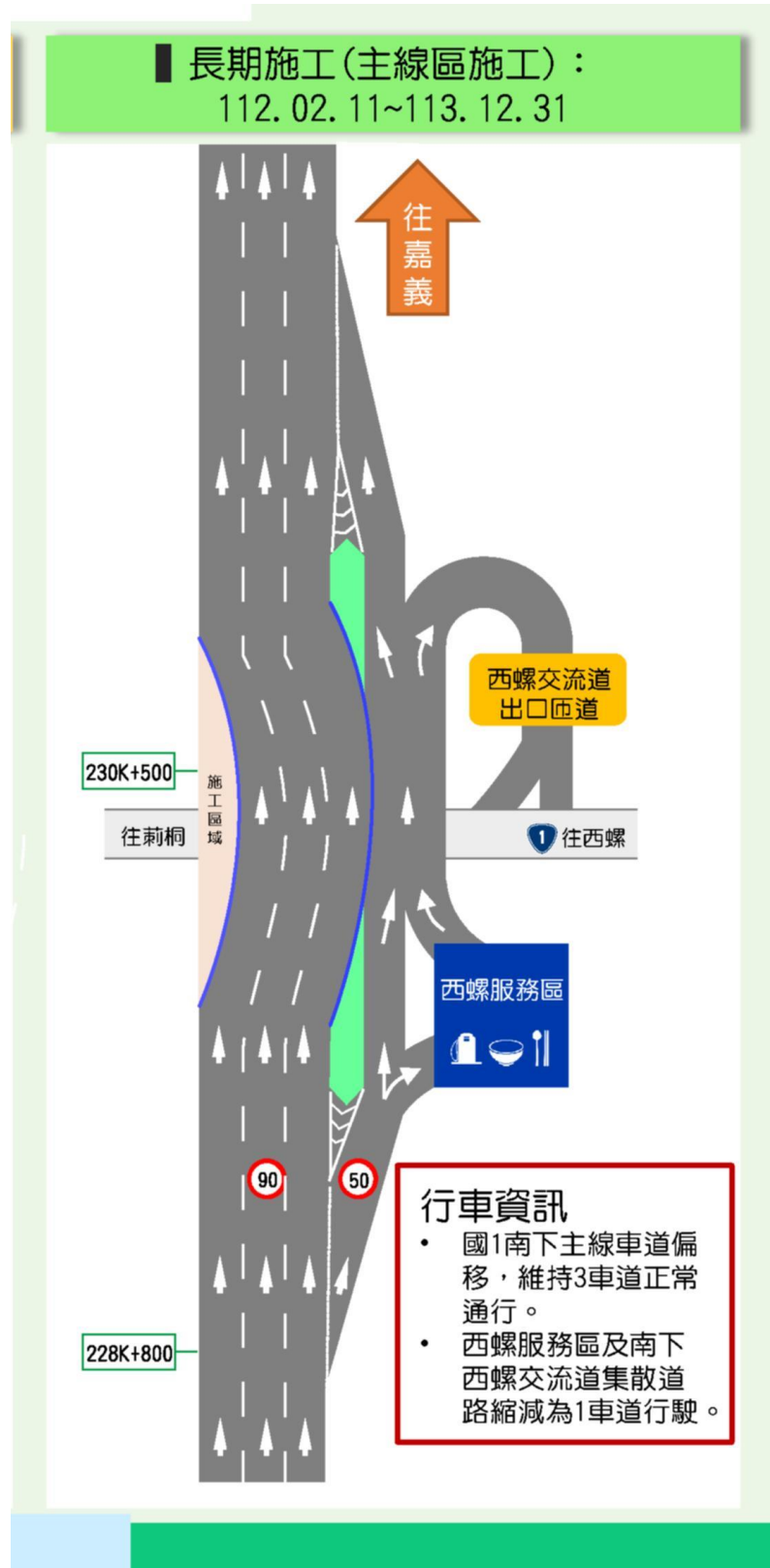
附圖 1 施工路段車道配置調整
