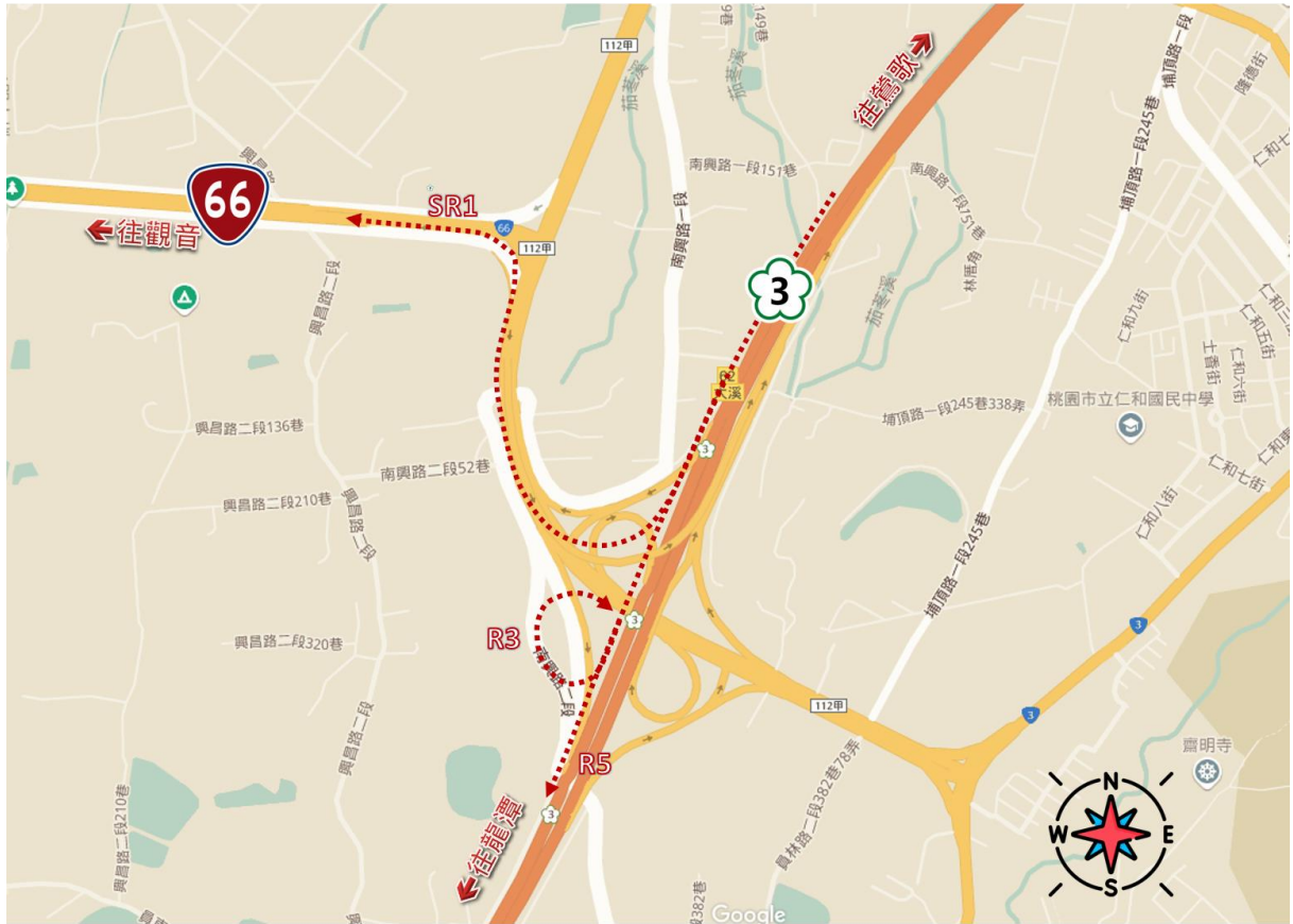
國道 3 號銜接台 66 線增設系統交流道工程位置
