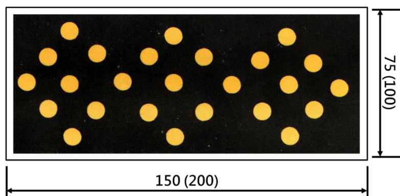
預告警示箭頭標誌牌面 (單位：公分)
