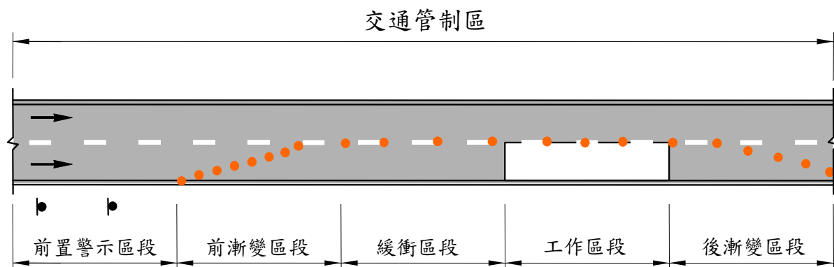
圖 3.1 交通管制區
