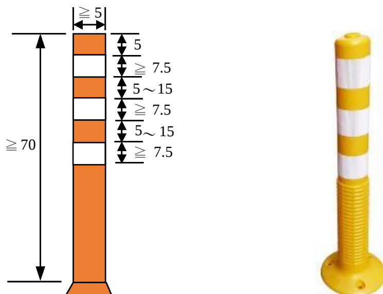
交通桿圖例及相片例 (註：水平環繞之反光材料數量依需要設置，至少 3 條)
