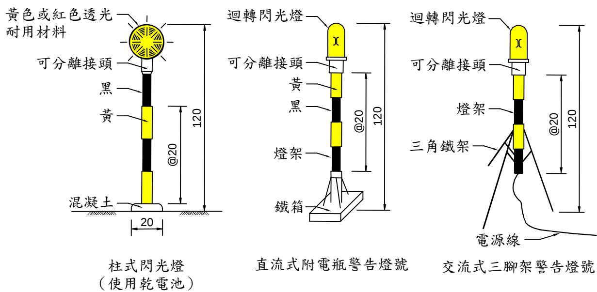
施工警告燈號裝設於獨立活動支架上
