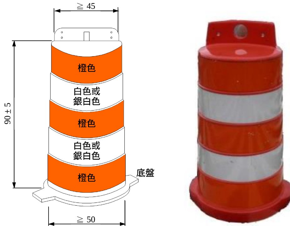
交通筒圖例及相片例 附圖二、(二) 交通筒
