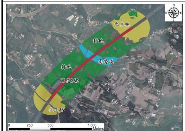
通霄四號高架橋(南北向)
