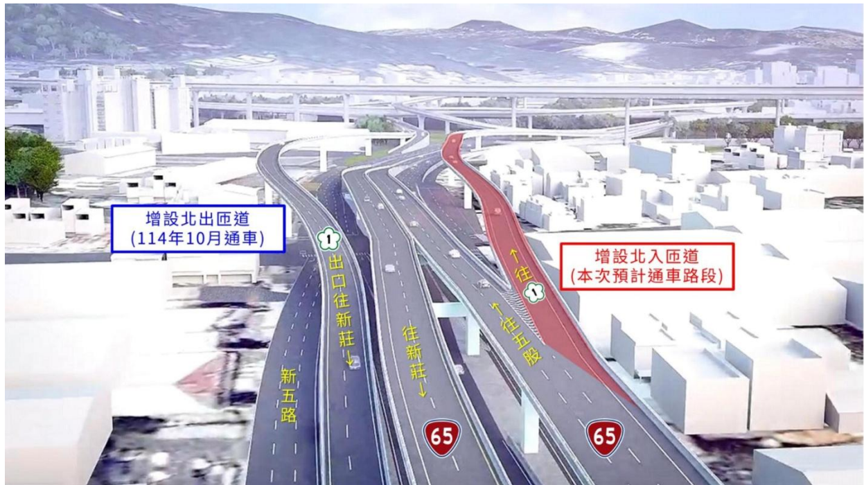
附圖 1 國道 1 號五股交流道增設北入及北出匝道改善工程示意圖
