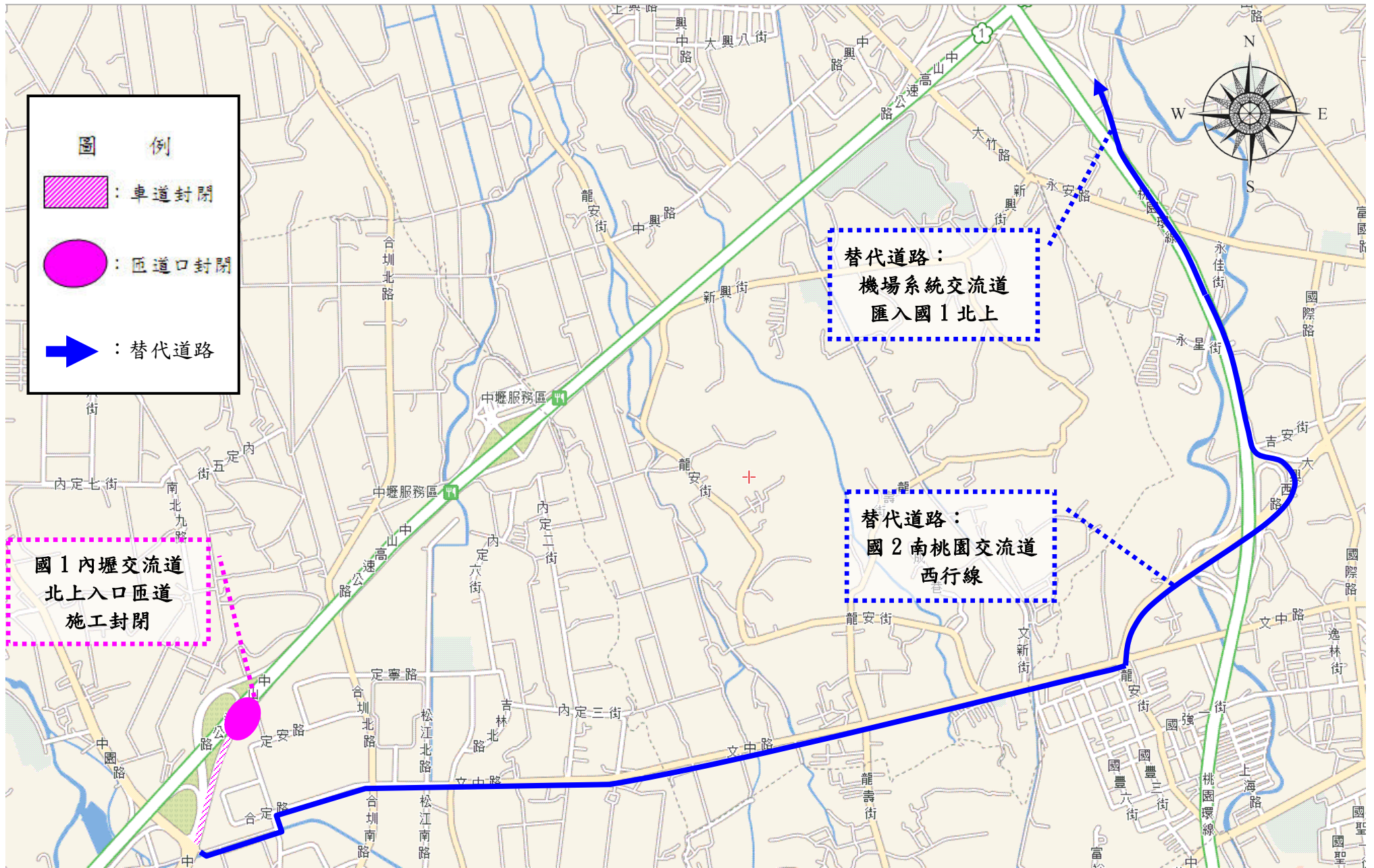
國道1號北上里程56K+700內壢交流道入口匝道施工封閉範圍暨改道路線示意圖
