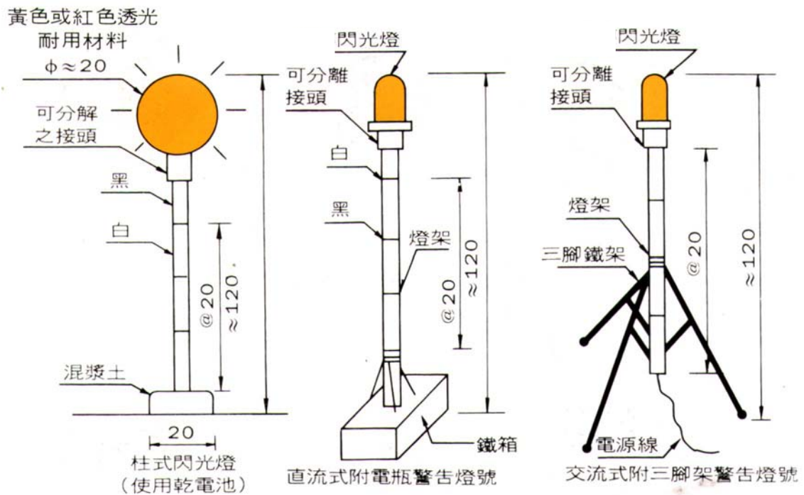
施工警告燈號裝設於獨立活動支架上 (單位：公分)
