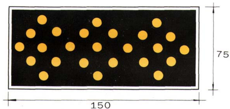
預告警示箭頭標誌牌面
