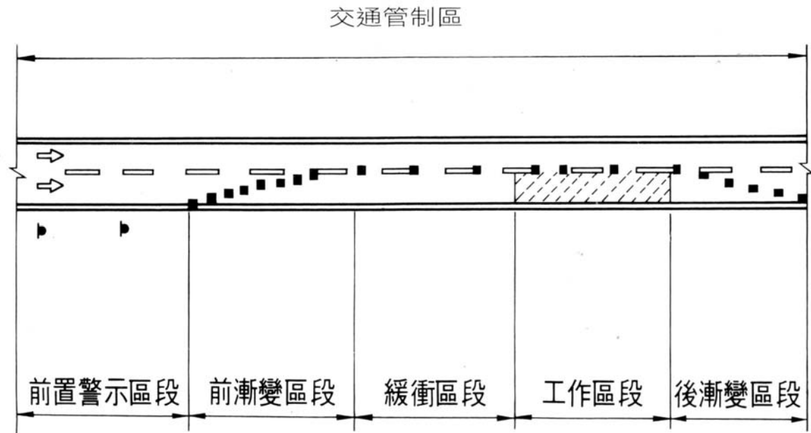
圖 3.1 交通管制區
