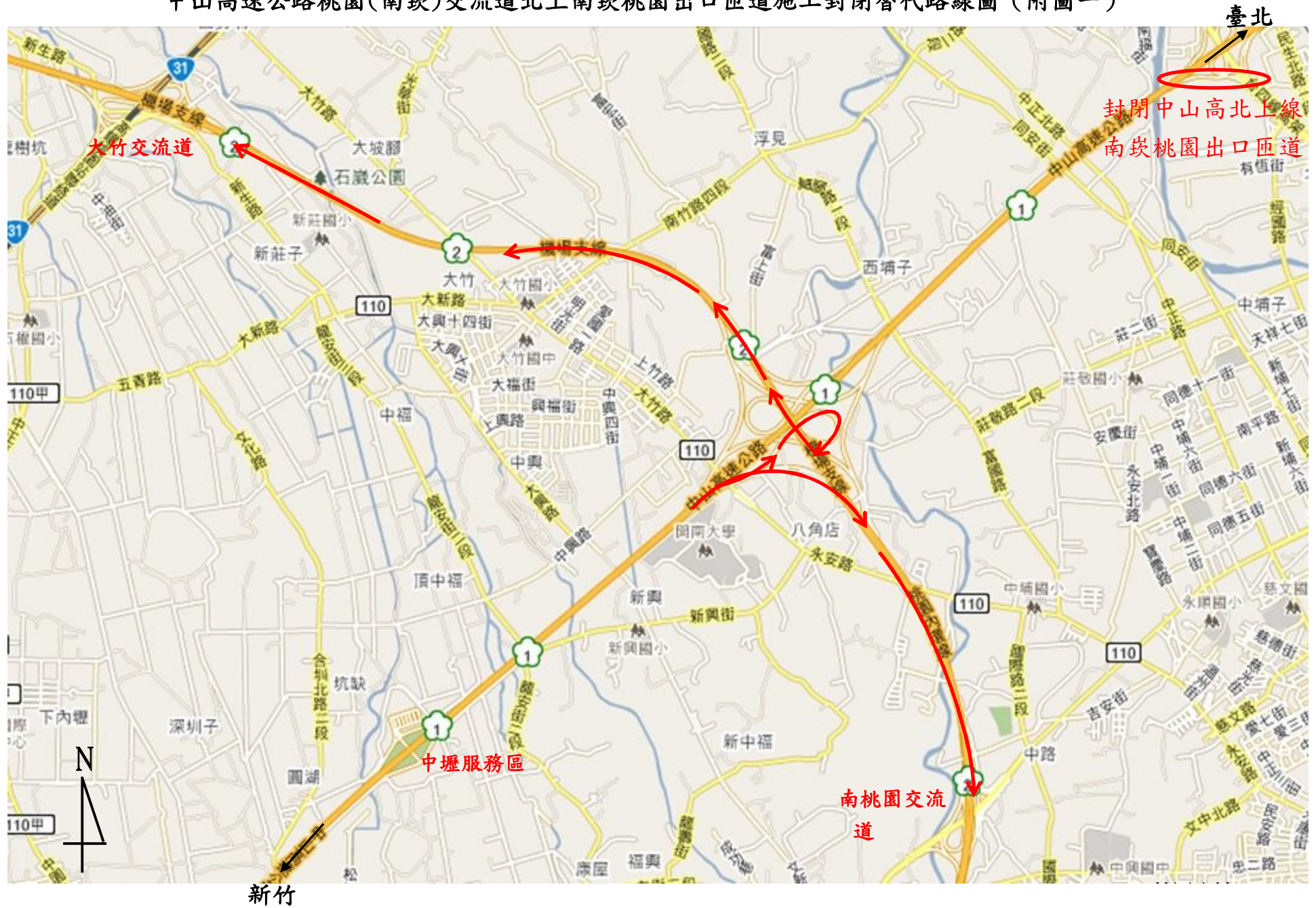
中山高速公路桃園(南崁)交流道北上南崁桃園出口匝道施工封閉替代路線圖 (附圖一)
