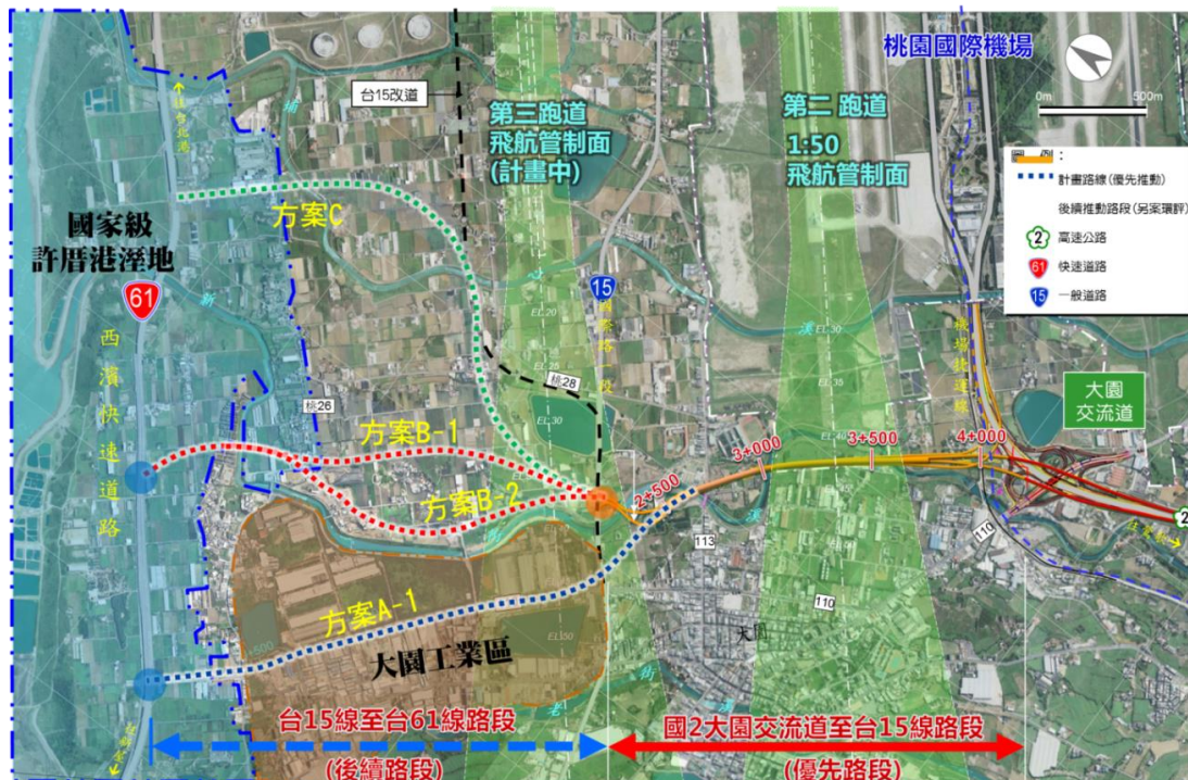
圖 1-2 國 2 大園交流道至台 61 線可行性研究路廊
