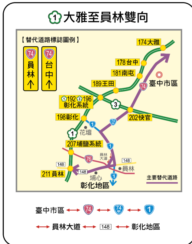
附圖 6 國 1 大雅至員林雙向替代道路路線圖
