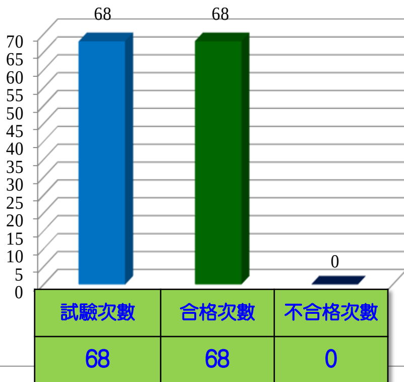
鋼纖噴凝土材料抗彎強度試驗次數統計
