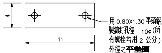
托架詳圖
