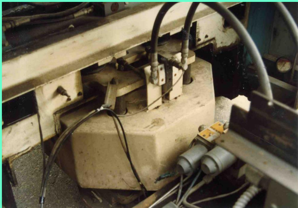
ROAD RTER MASE 震動體
