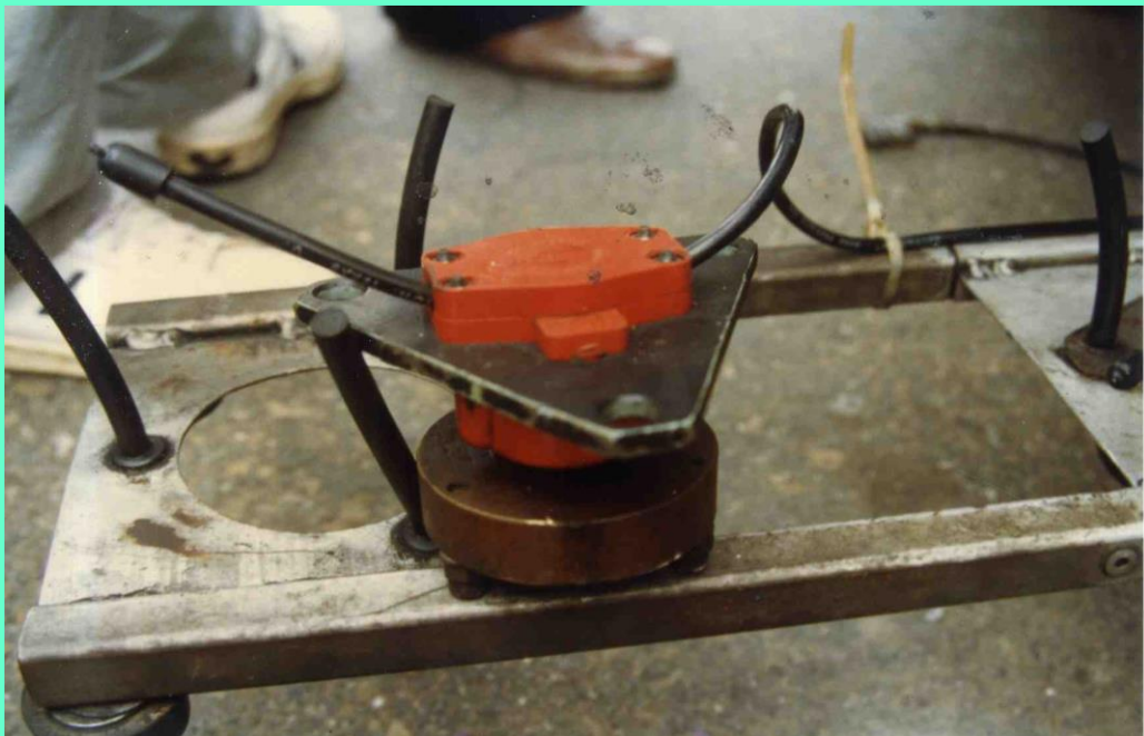
ROAD RATER 感應器
