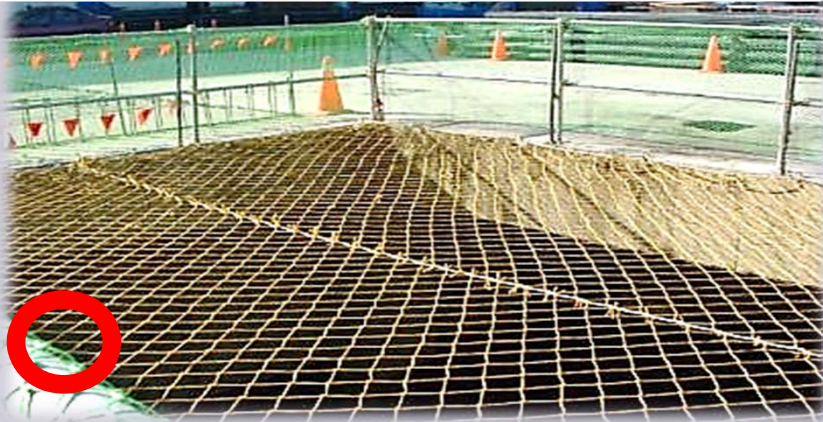
樓版開口應設護欄、安全網
