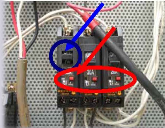
漏電斷路器押下測試鈕 紅色箭頭所指之處)後跳 脫情形。
