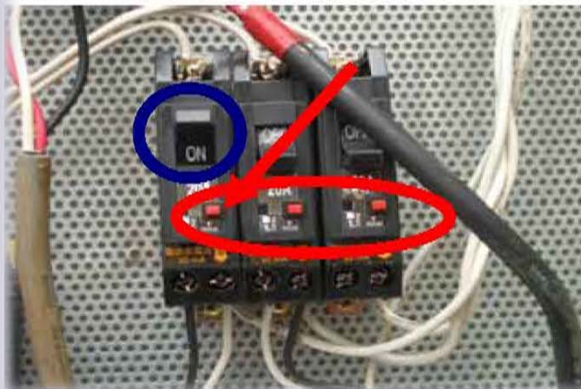
漏電斷路器測試前
