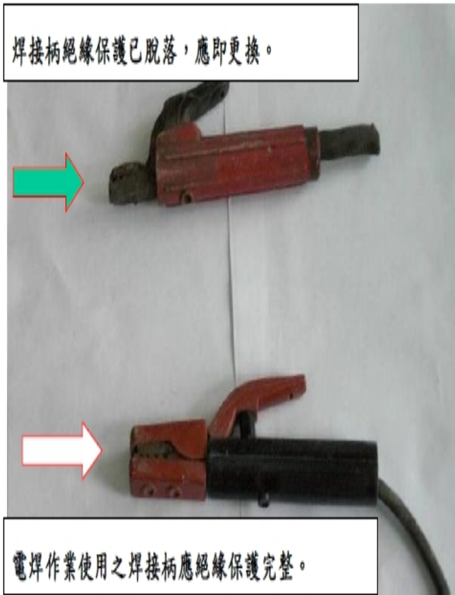
電焊作業使用之焊接柄應有相當之絕緣耐力及耐熱性。
