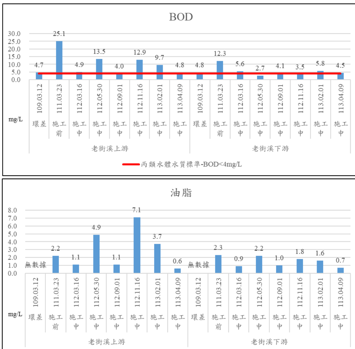
圖 2-7 河川水質結果趨勢圖(續 2)
