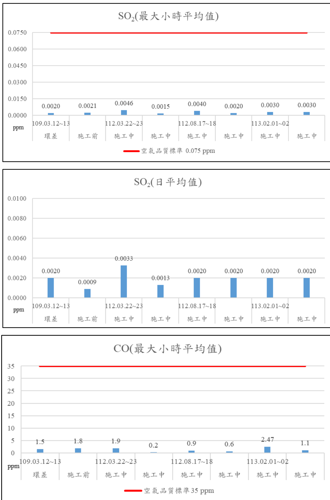
圖 2- 1 空氣品質監測結果趨勢圖(續 3)
