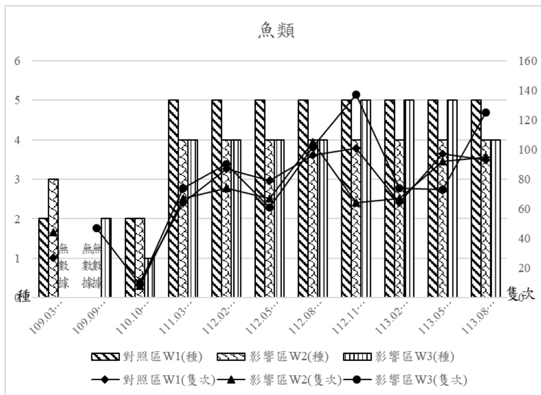
圖 2- 11 魚類調查趨勢圖
