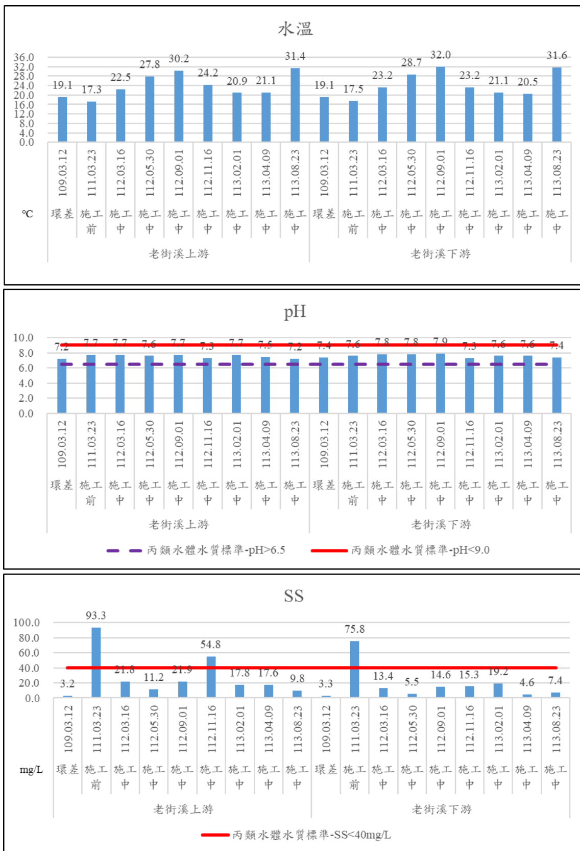
圖 2-7 河川水質結果趨勢圖
