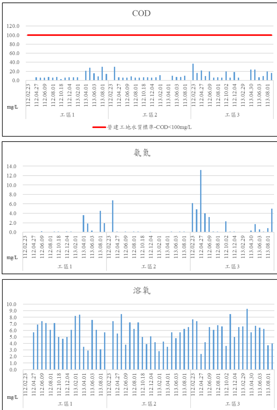
圖 2-6 工區放流水水質結果趨勢圖(續 1)
