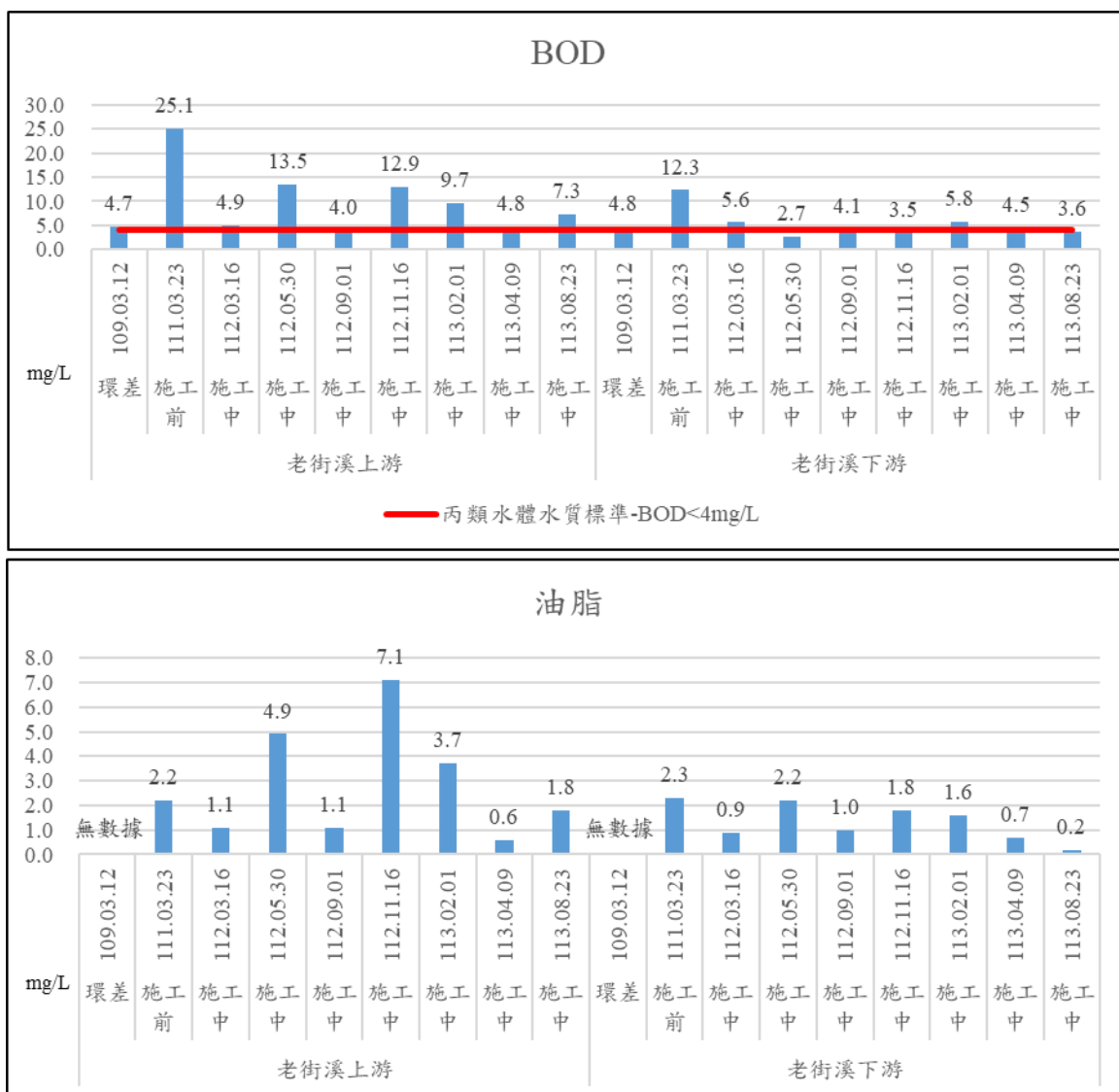
圖 2-7 河川水質結果趨勢圖(續 2)
