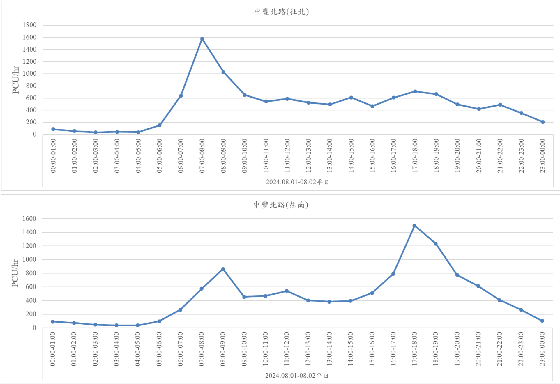
圖 2- 8 本期交通逐時變化圖
