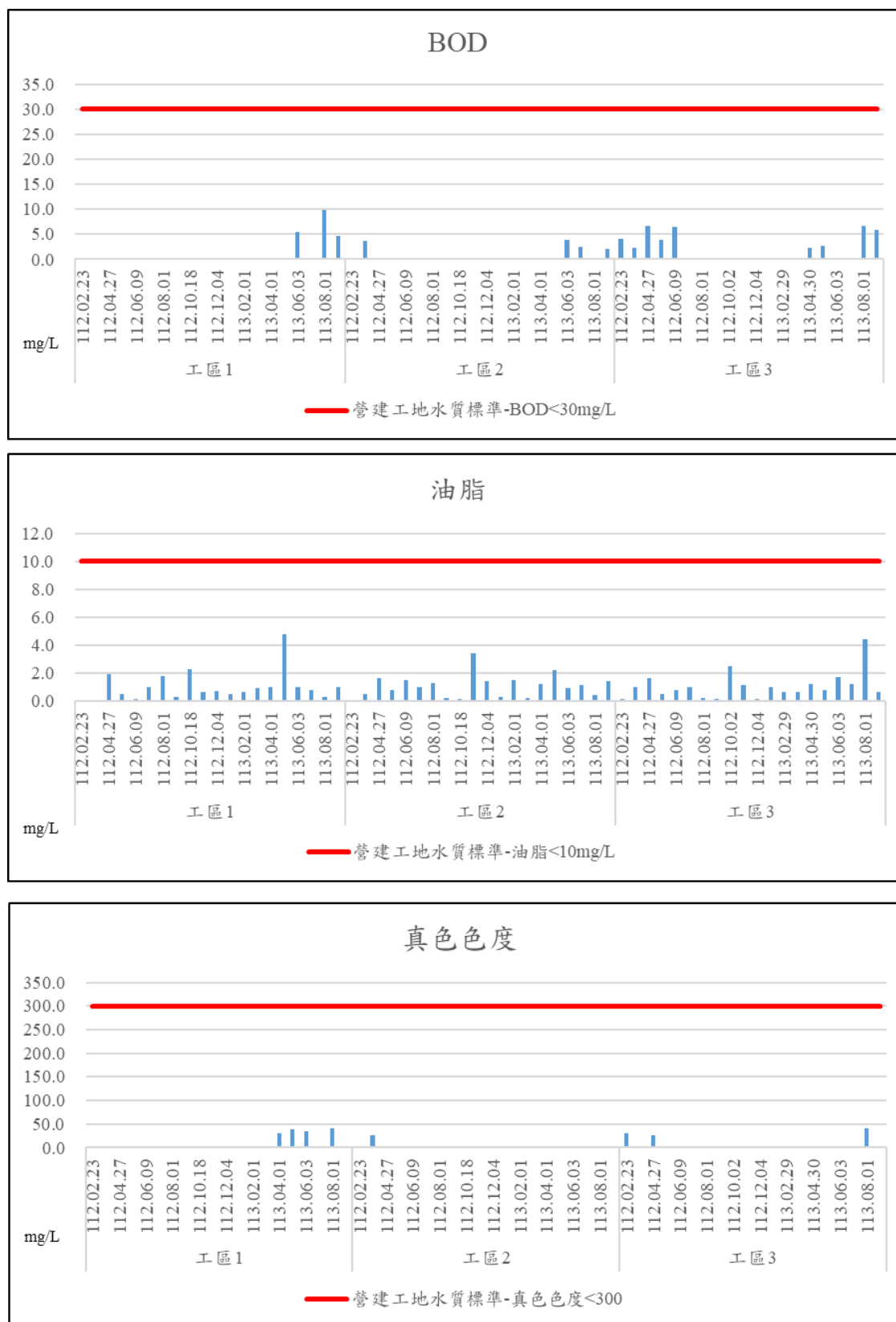
圖 2-6 工區放流水水質結果趨勢圖(續 2)
