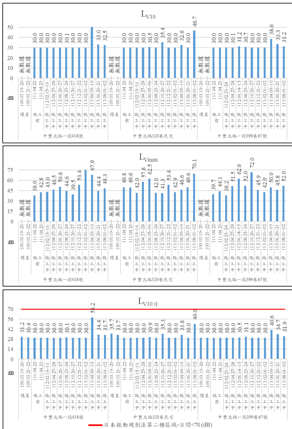
圖 2-3 振動結果趨勢圖
