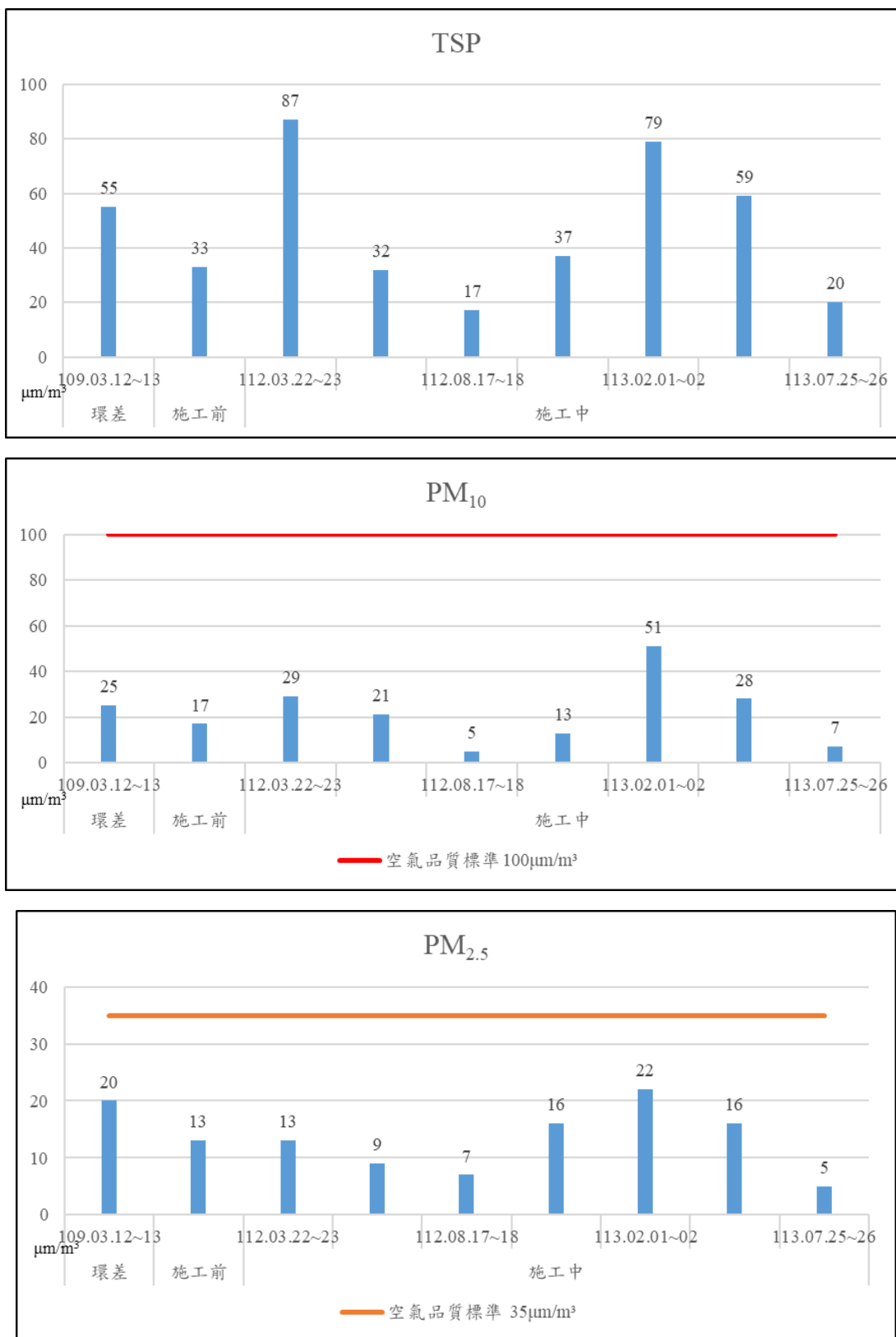
圖 2- 1 空氣品質監測結果趨勢圖
