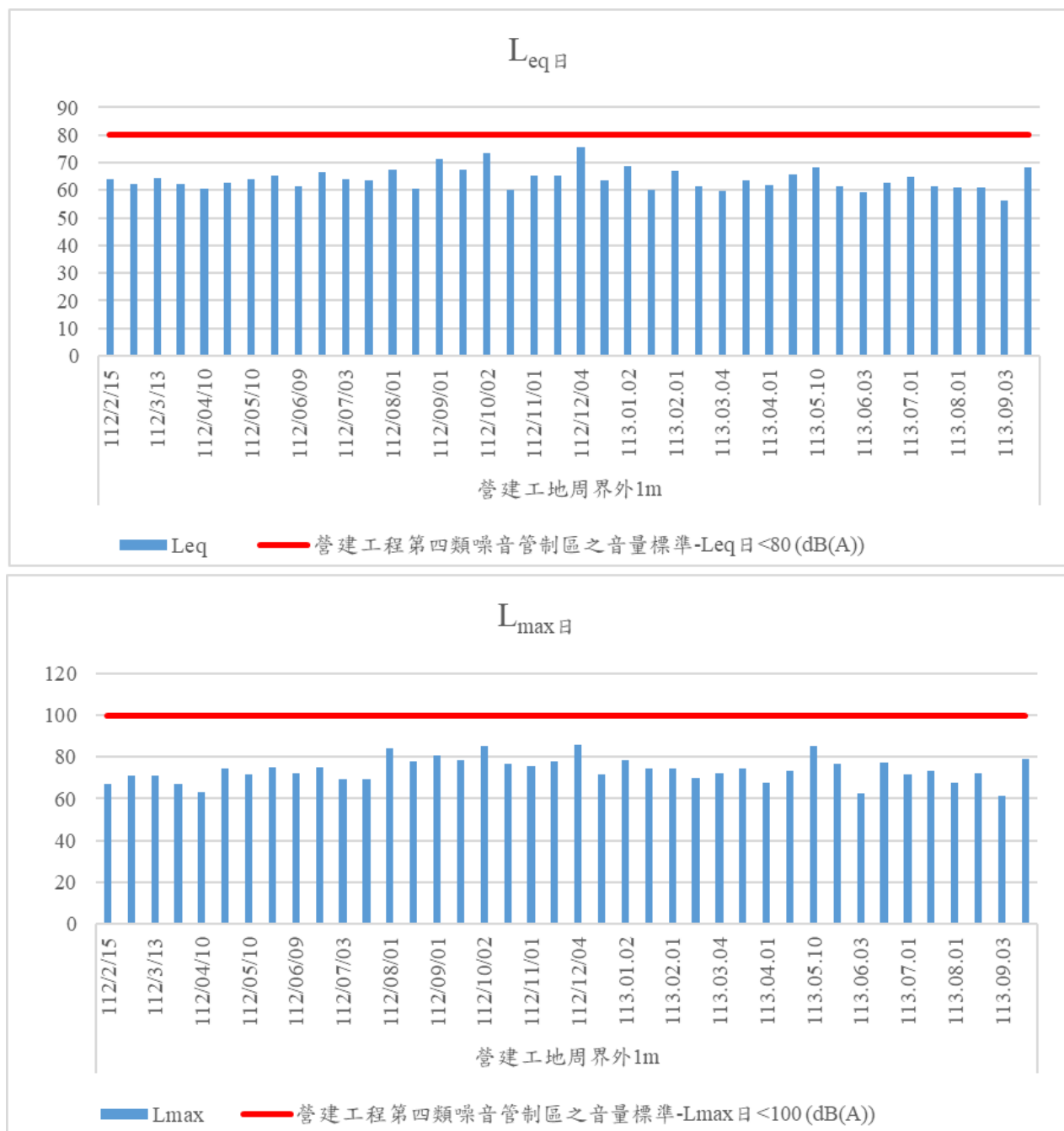
圖 2-4 營建噪音結果趨勢圖
