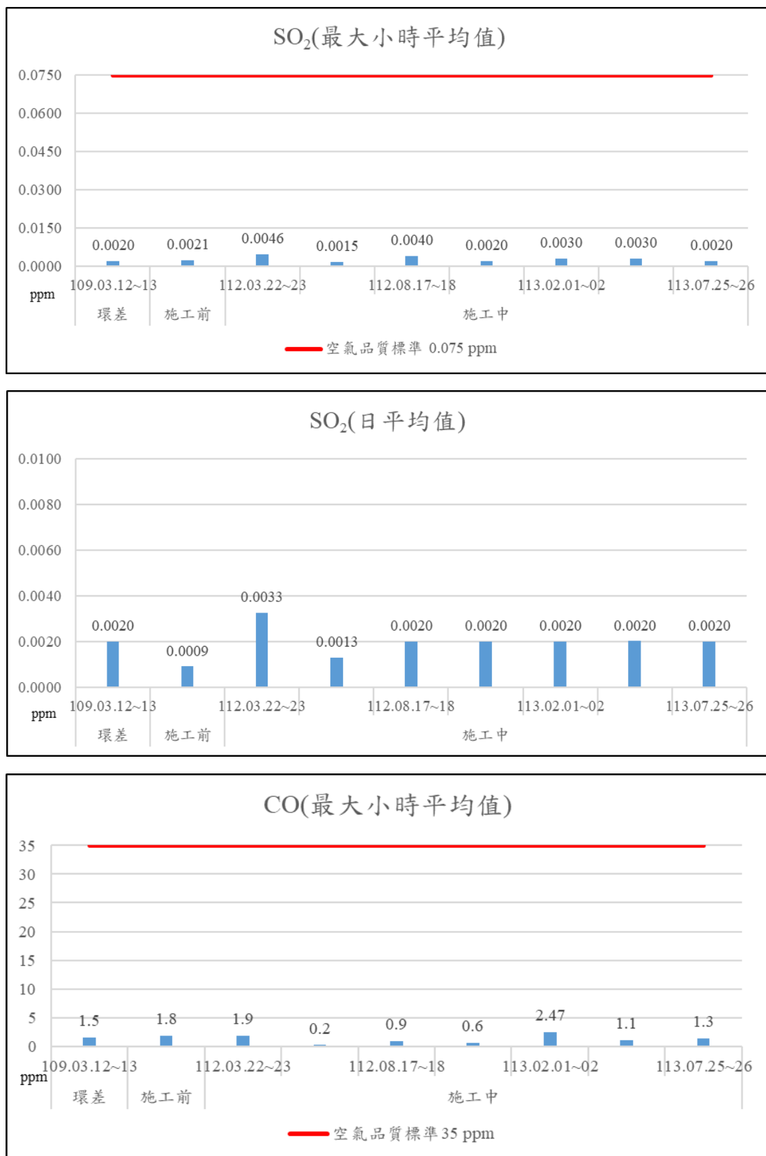
圖 2- 1 空氣品質監測結果趨勢圖(續 3)
