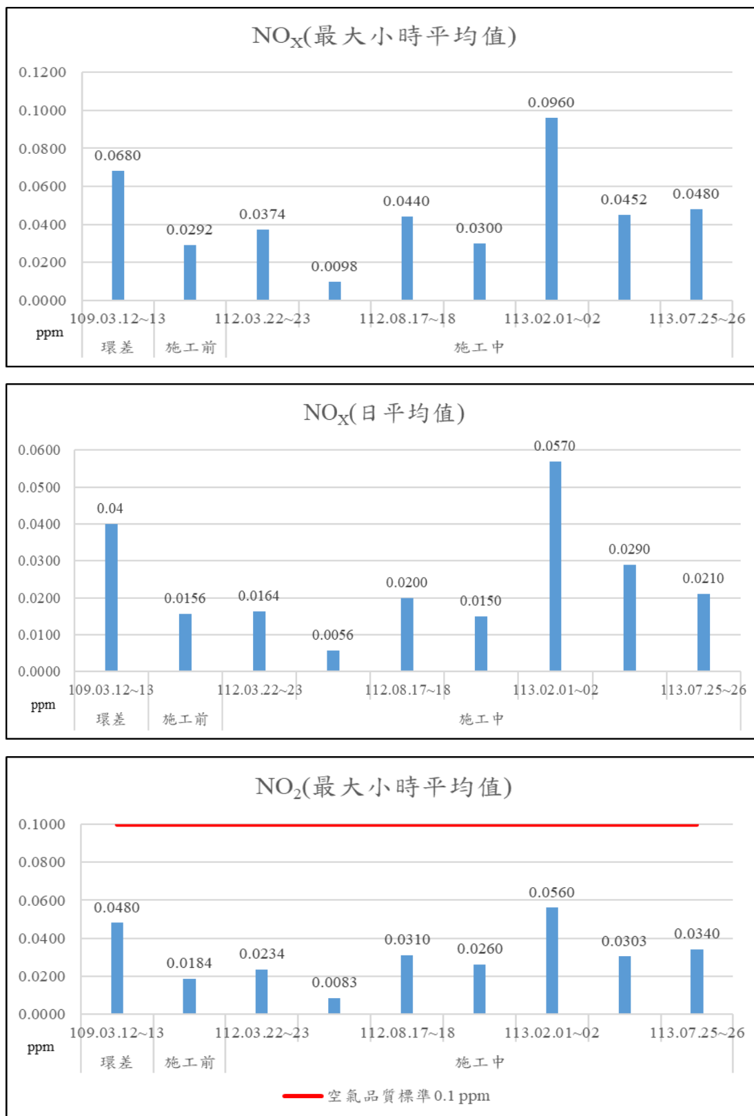
圖 2-1 空氣品質監測結果趨勢圖(續 1)
