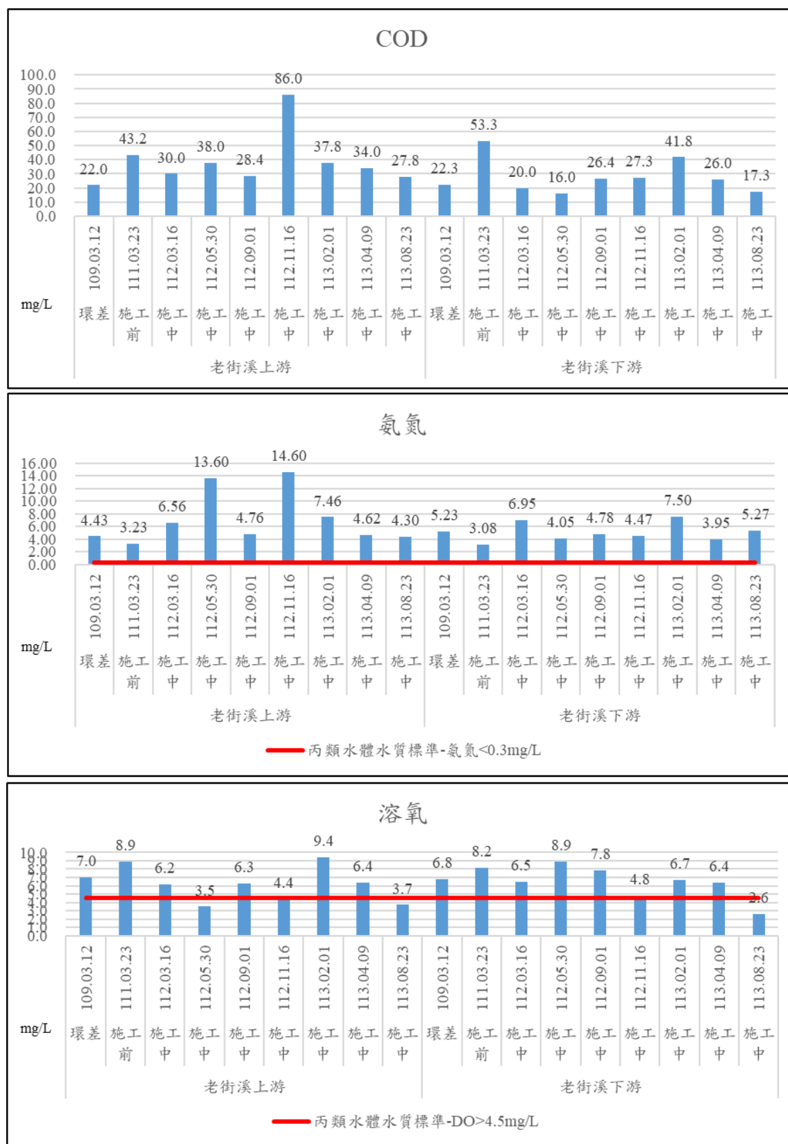
圖 2-7 河川水質結果趨勢圖(續 1)
