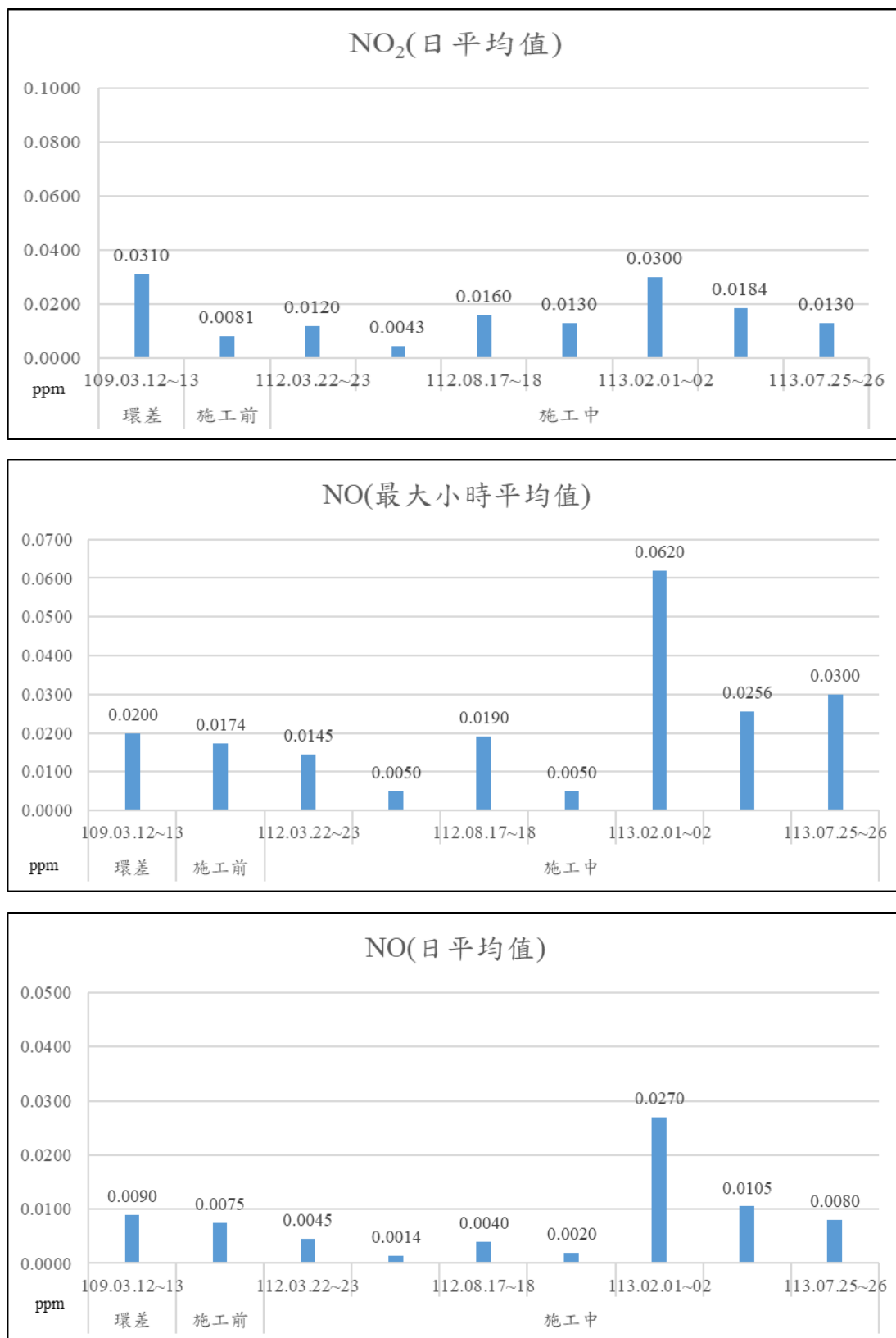
圖 2- 1 空氣品質監測結果趨勢圖(續 2)
