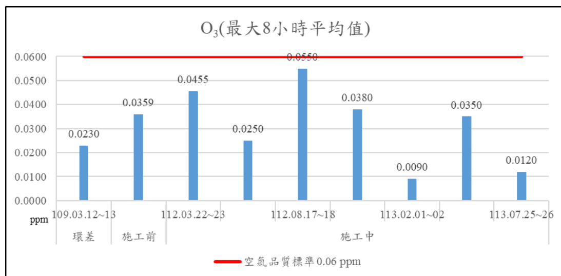
圖 2- 1 空氣品質監測結果趨勢圖 (續 4)
