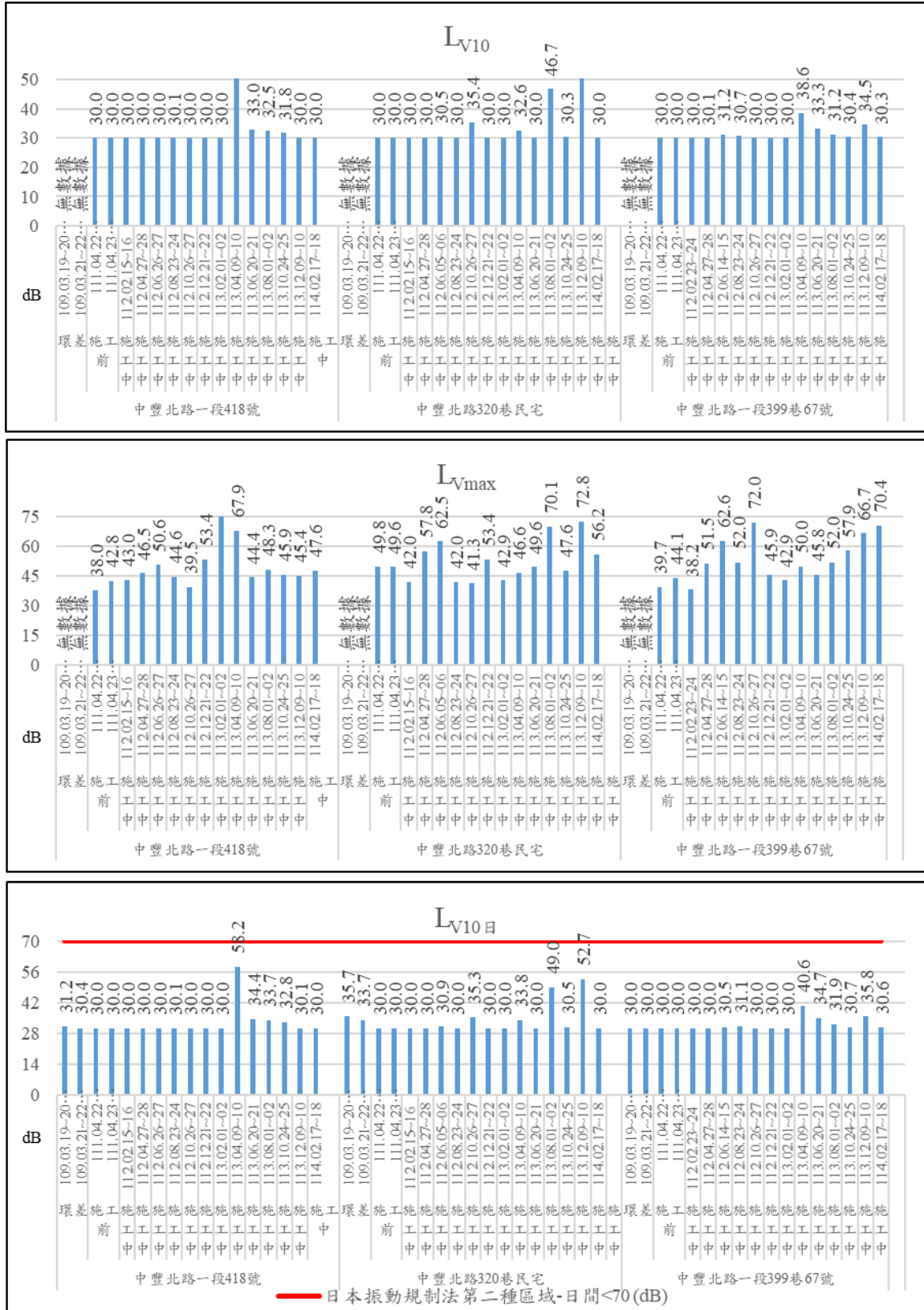
圖 2-4 振動結果趨勢圖
