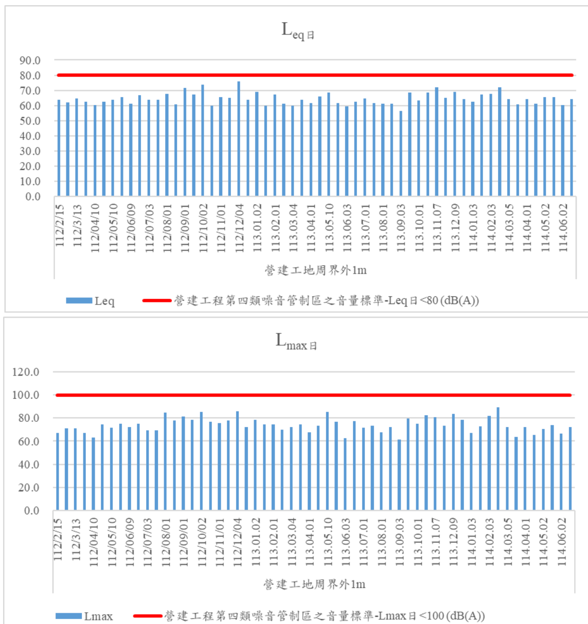
圖 2-4 營建噪音結果趨勢圖
