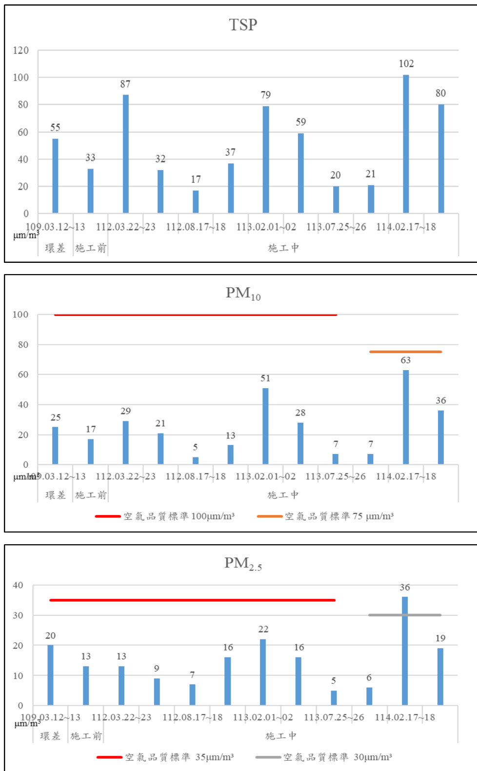
圖 2- 1 空氣品質監測結果趨勢圖
