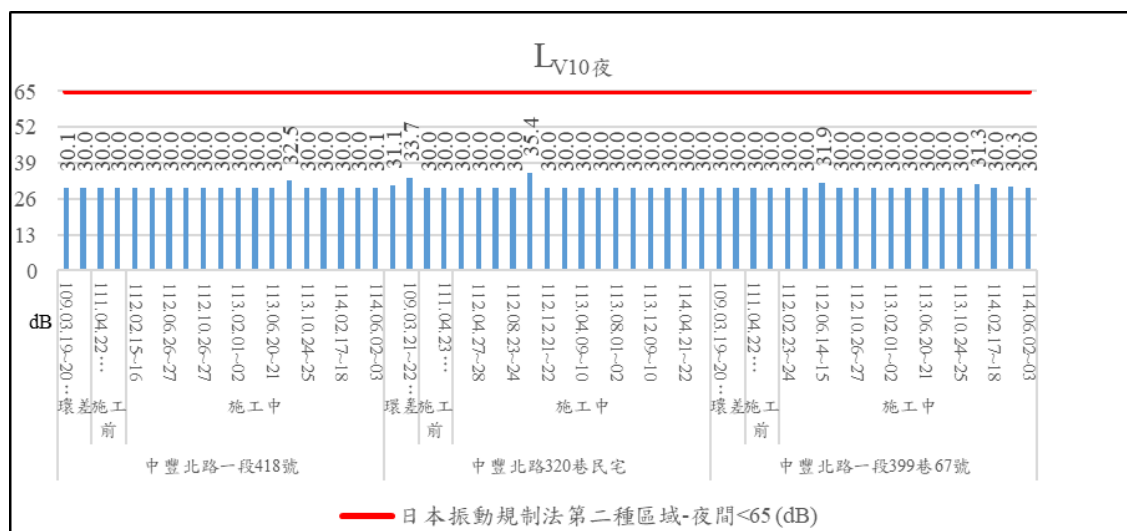
圖 2- 4 振動結果趨勢圖 (續 1)
