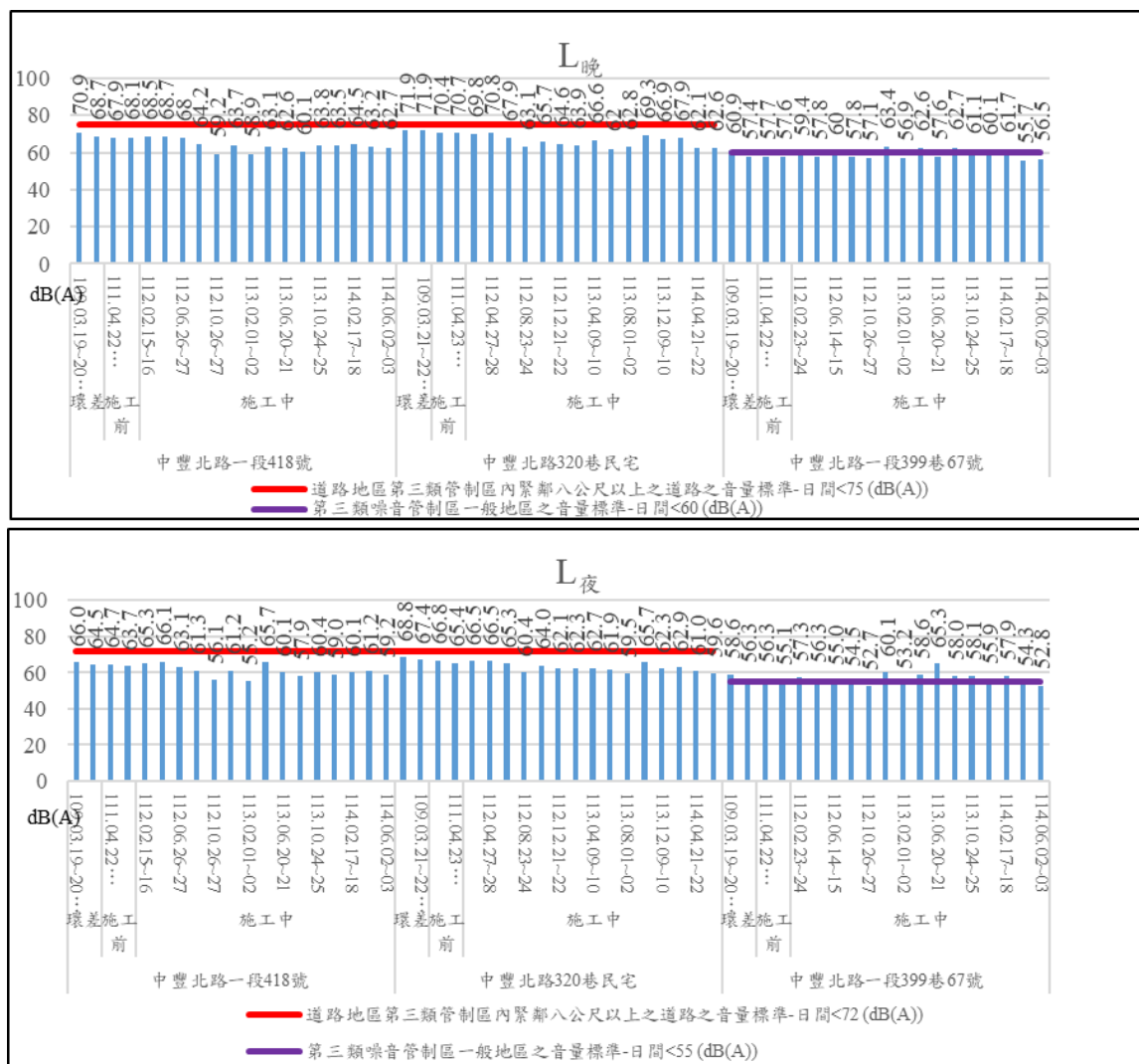
圖 2-3 噪音監測結果趨勢圖(續)
