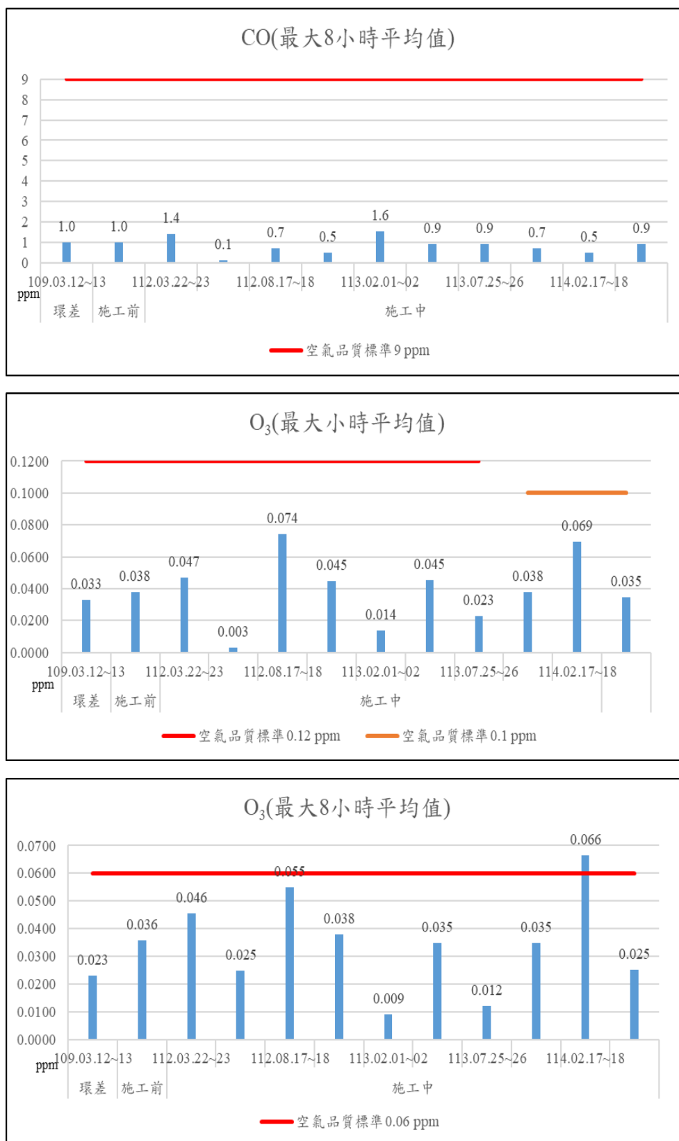
圖 2- 1 空氣品質監測結果趨勢圖 (續 4)
