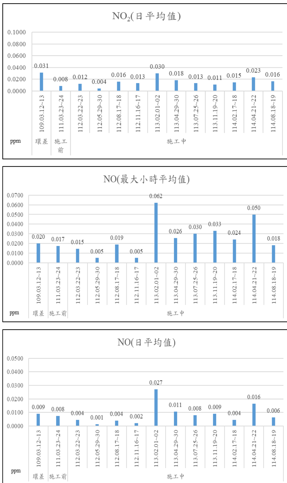
圖 2-1 空氣品質監測結果趨勢圖(續 2)
