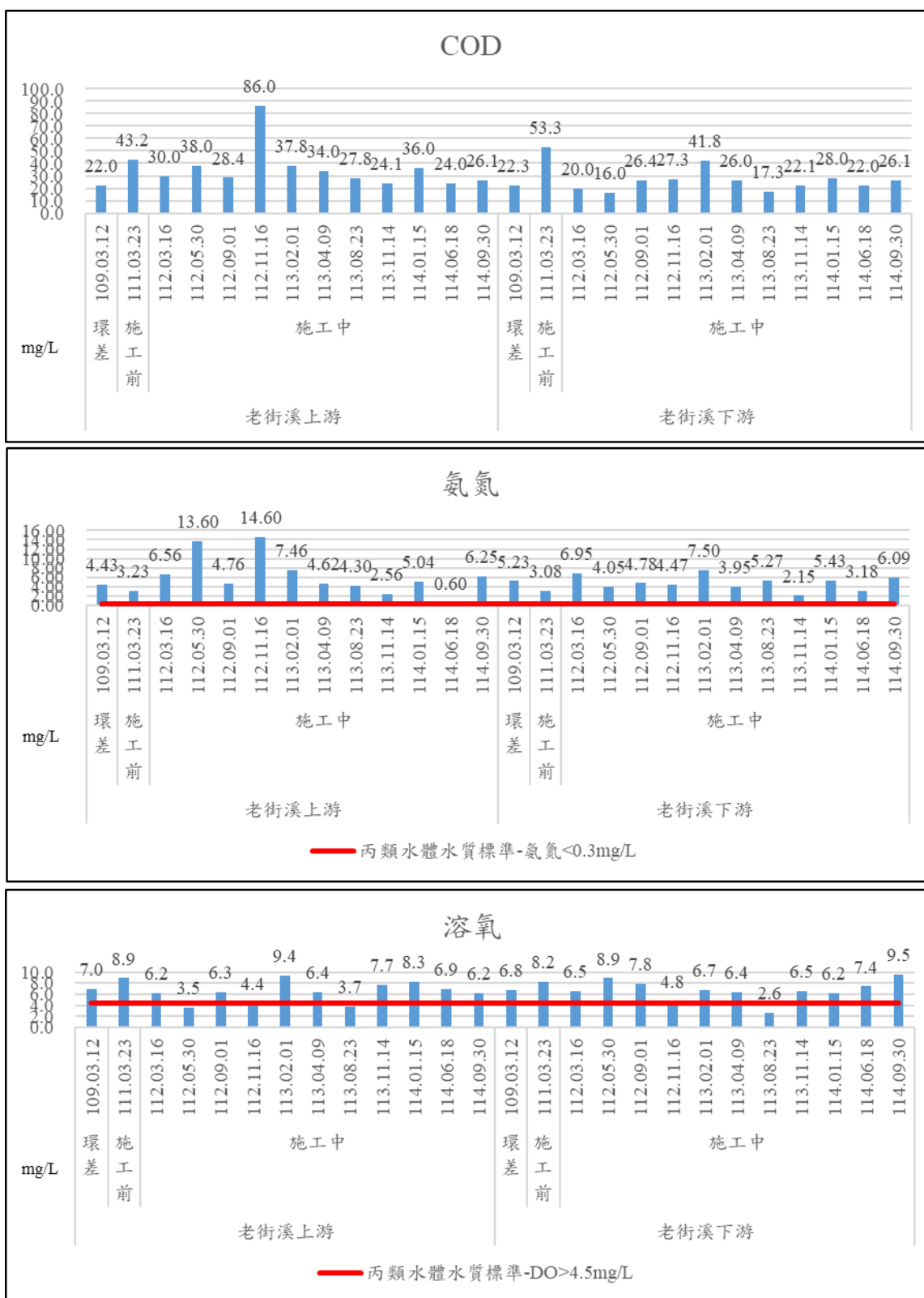
圖 2-8 河川水質結果趨勢圖(續 1)
