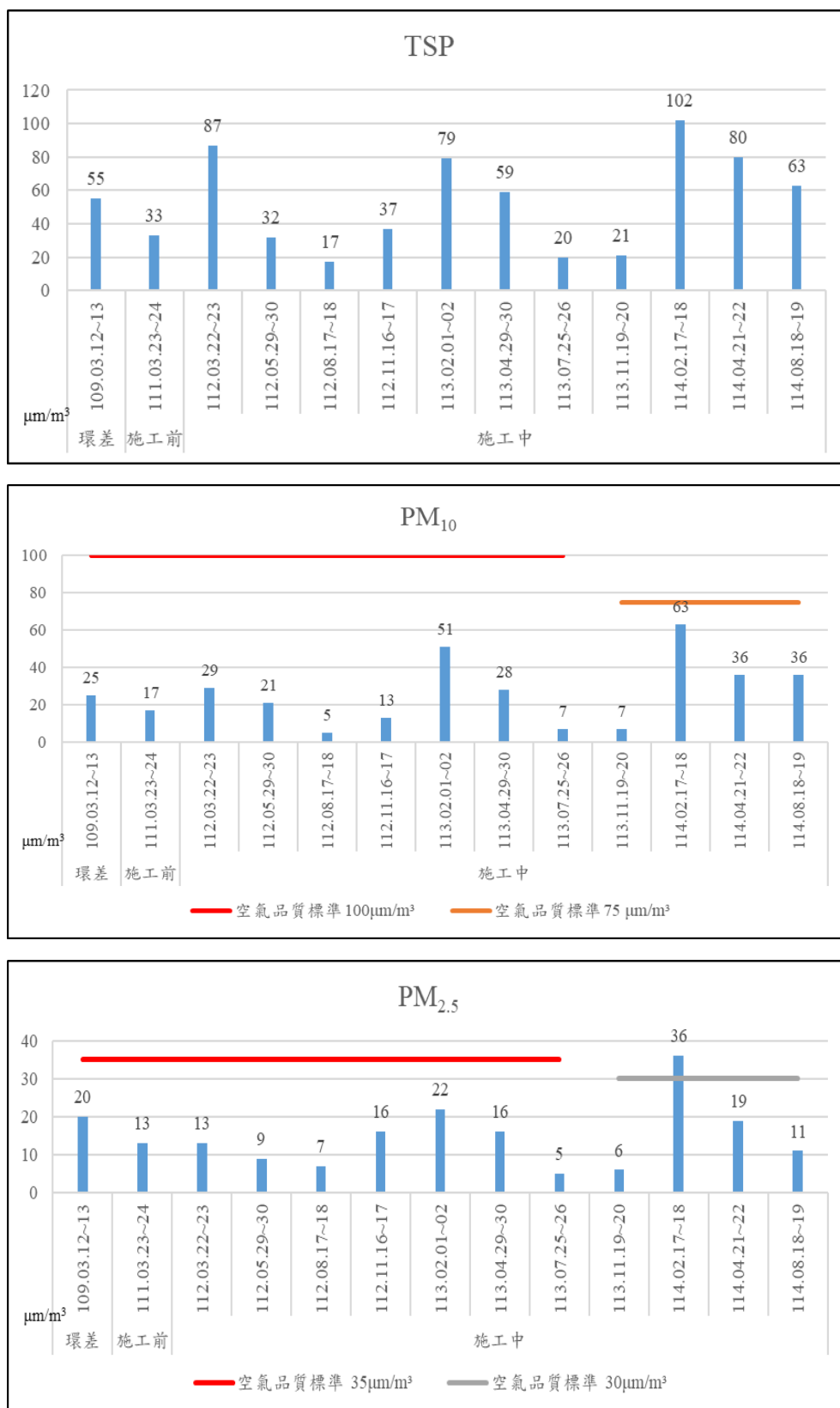
圖 2- 1 空氣品質監測結果趨勢圖
