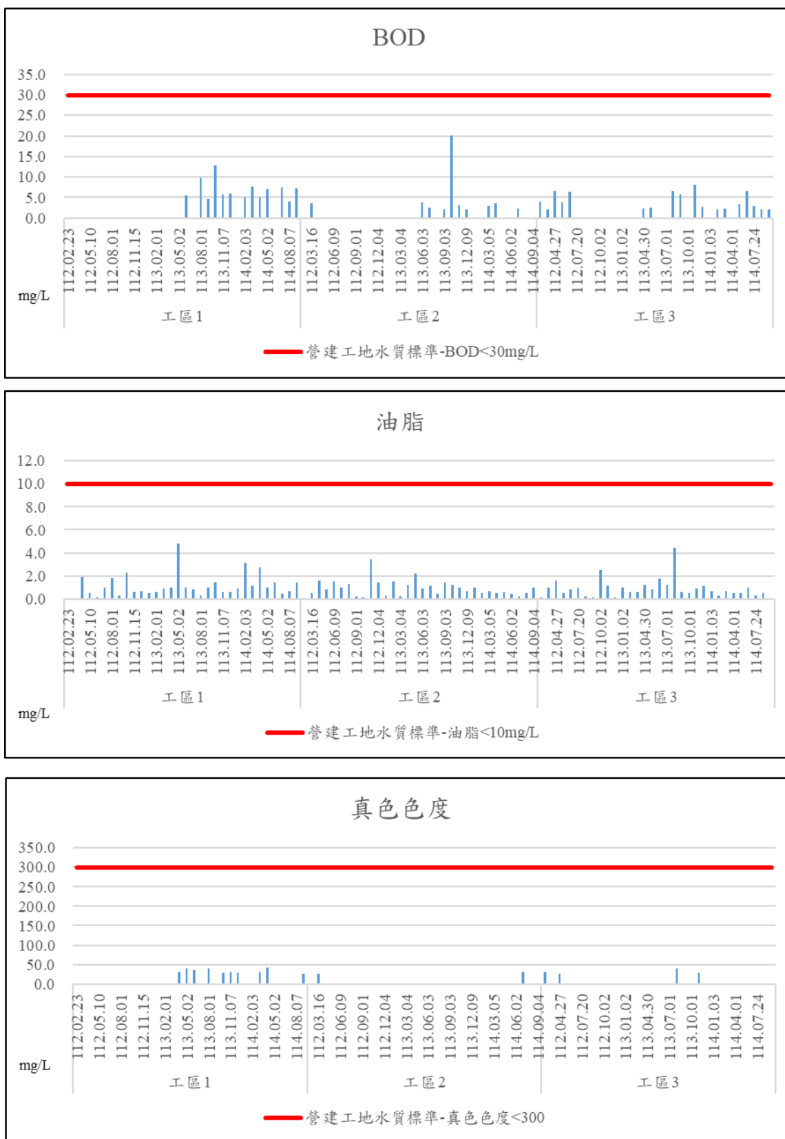
圖 2-7 工區放流水水質結果趨勢圖(續 2)
