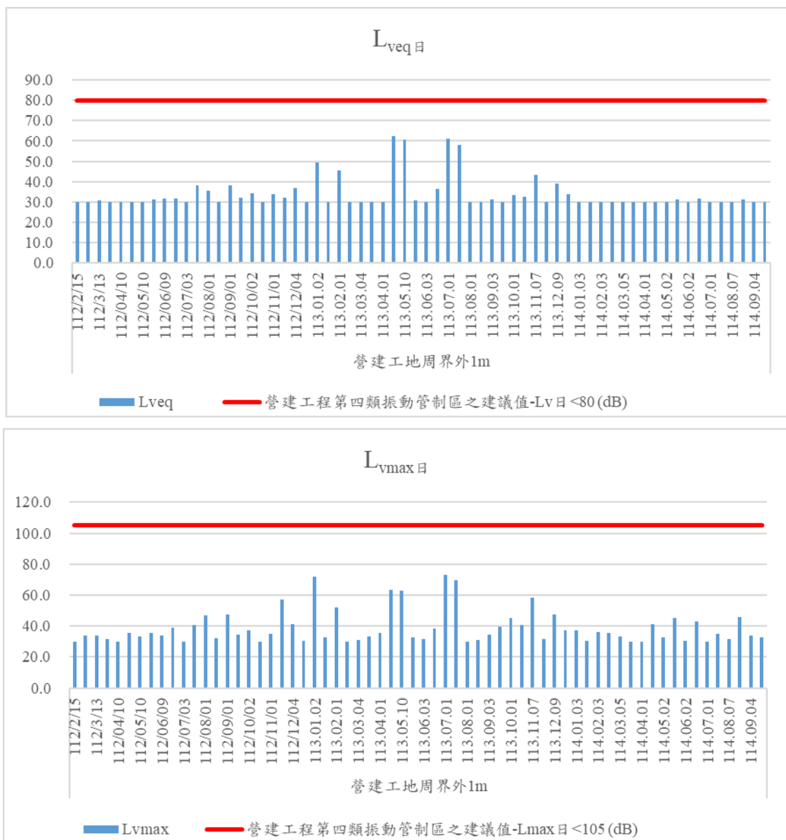
圖 2-5 營建振動結果趨勢圖
