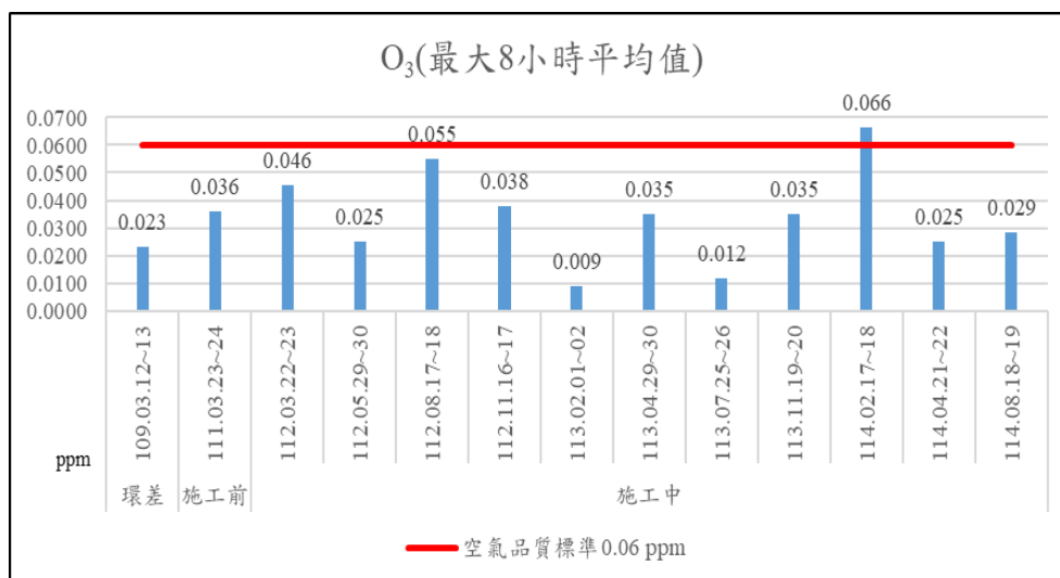
圖 2- 1 空氣品質監測結果趨勢圖 (續 4)
