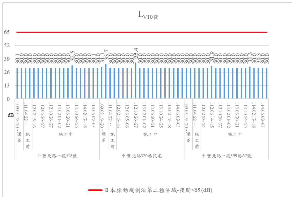
圖 2-4 振動結果趨勢圖 (續 1)
