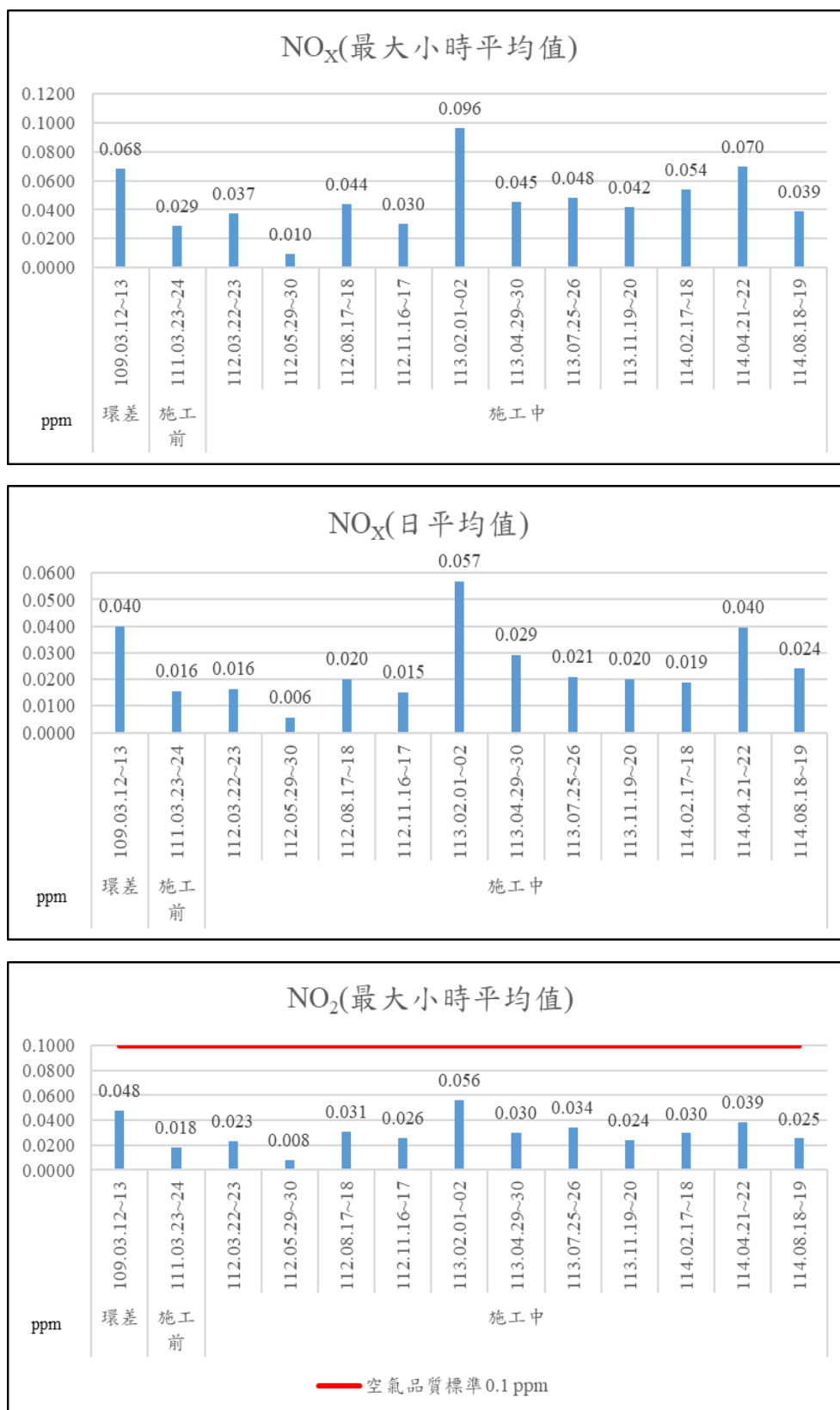
圖 2-1 空氣品質監測結果趨勢圖(續 1)
