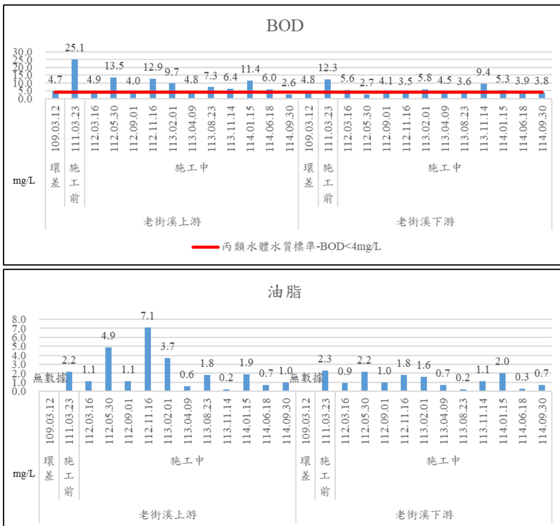
圖 2-8 河川水質結果趨勢圖(續 2)
