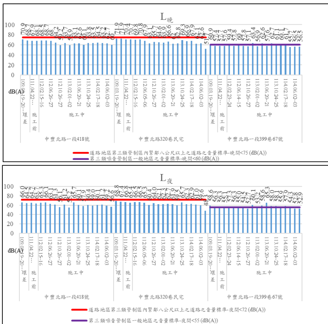
圖 2- 3 噪音監測結果趨勢圖(續)
