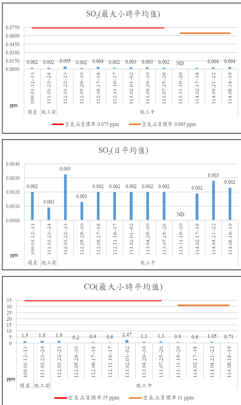
圖 2-1 空氣品質監測結果趨勢圖(續 3)
