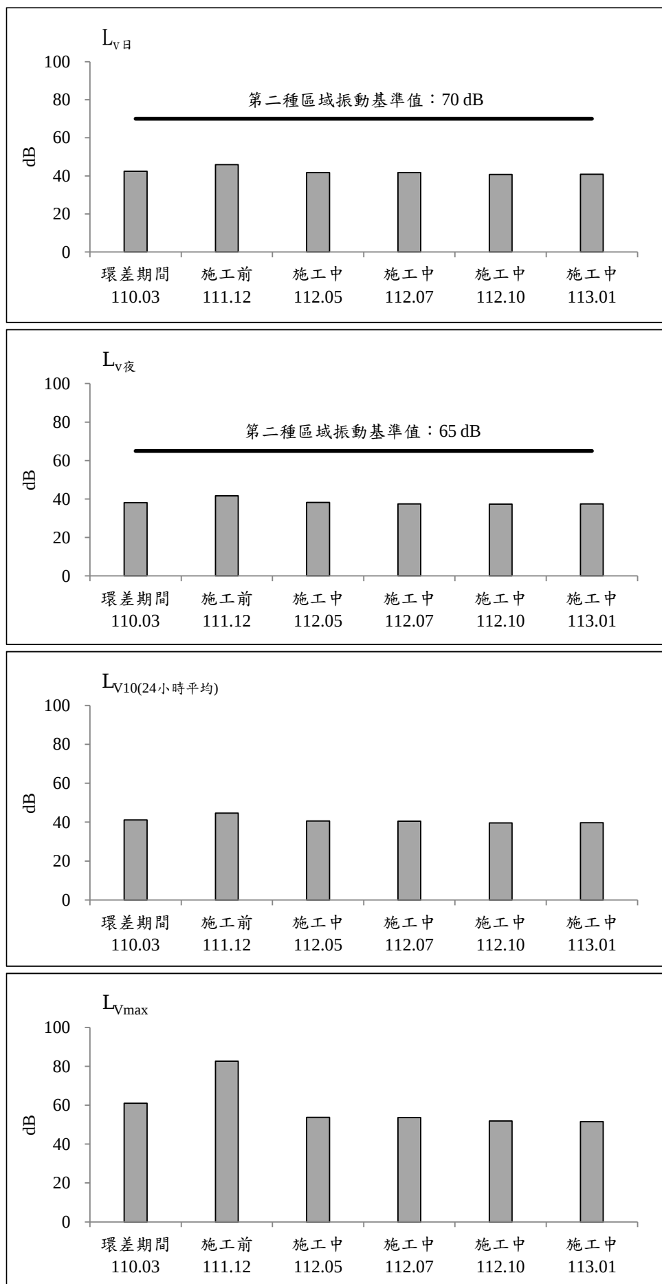
圖 2.2-6 德音國民小學測站歷次振動監測之各項測值變化圖(平日)
