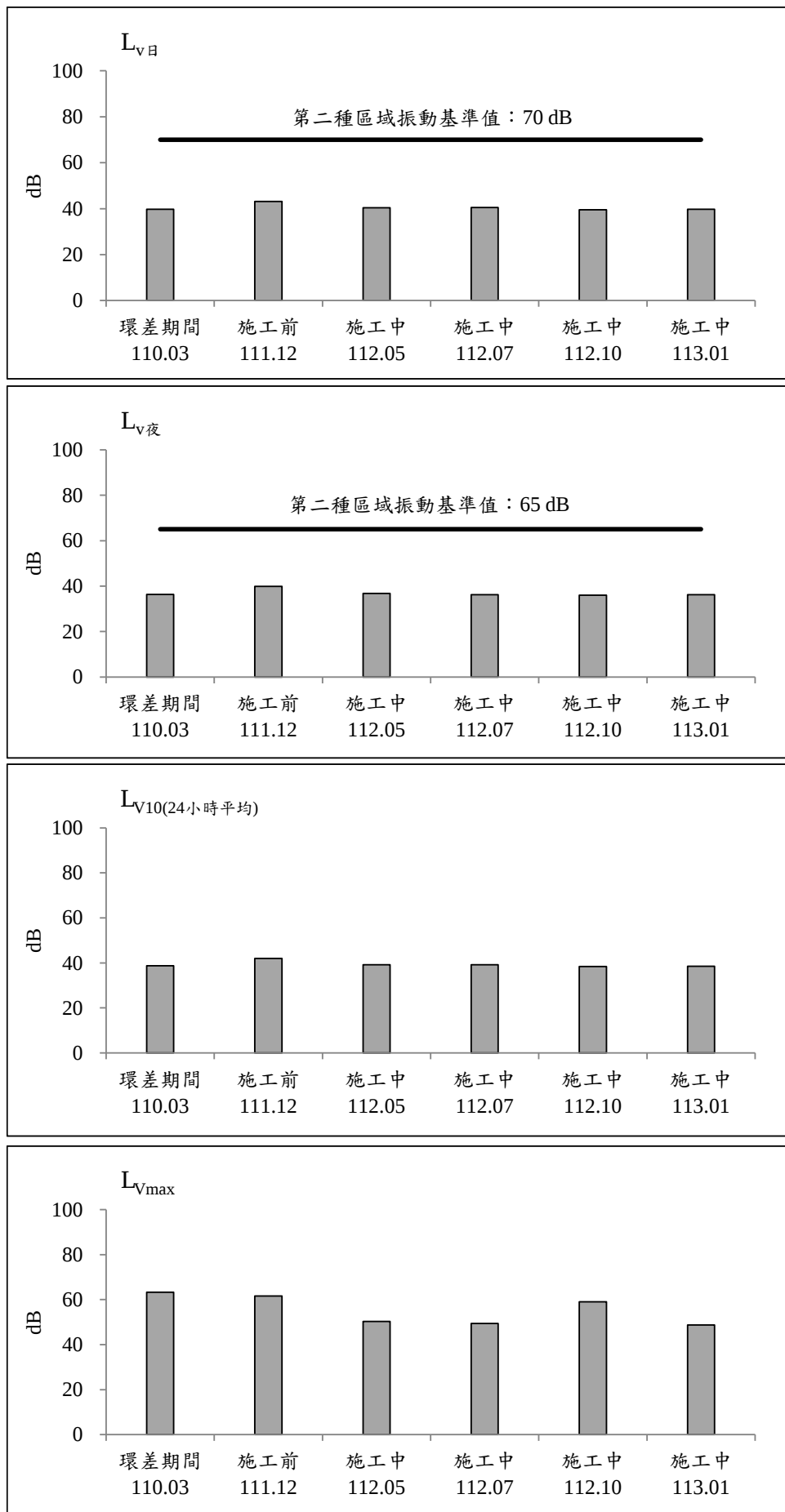
圖 2.2-5 德音國民小學測站歷次振動監測之各項測值變化圖(假日)
