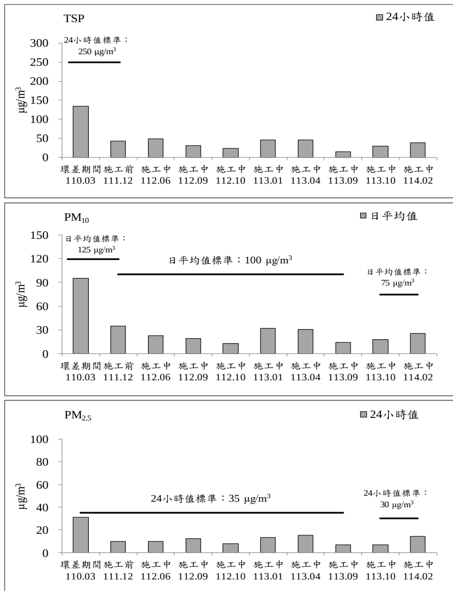
圖 2.1-2 準休閒農場測站歷次空氣品質監測之各項測值變化圖(續 3)
