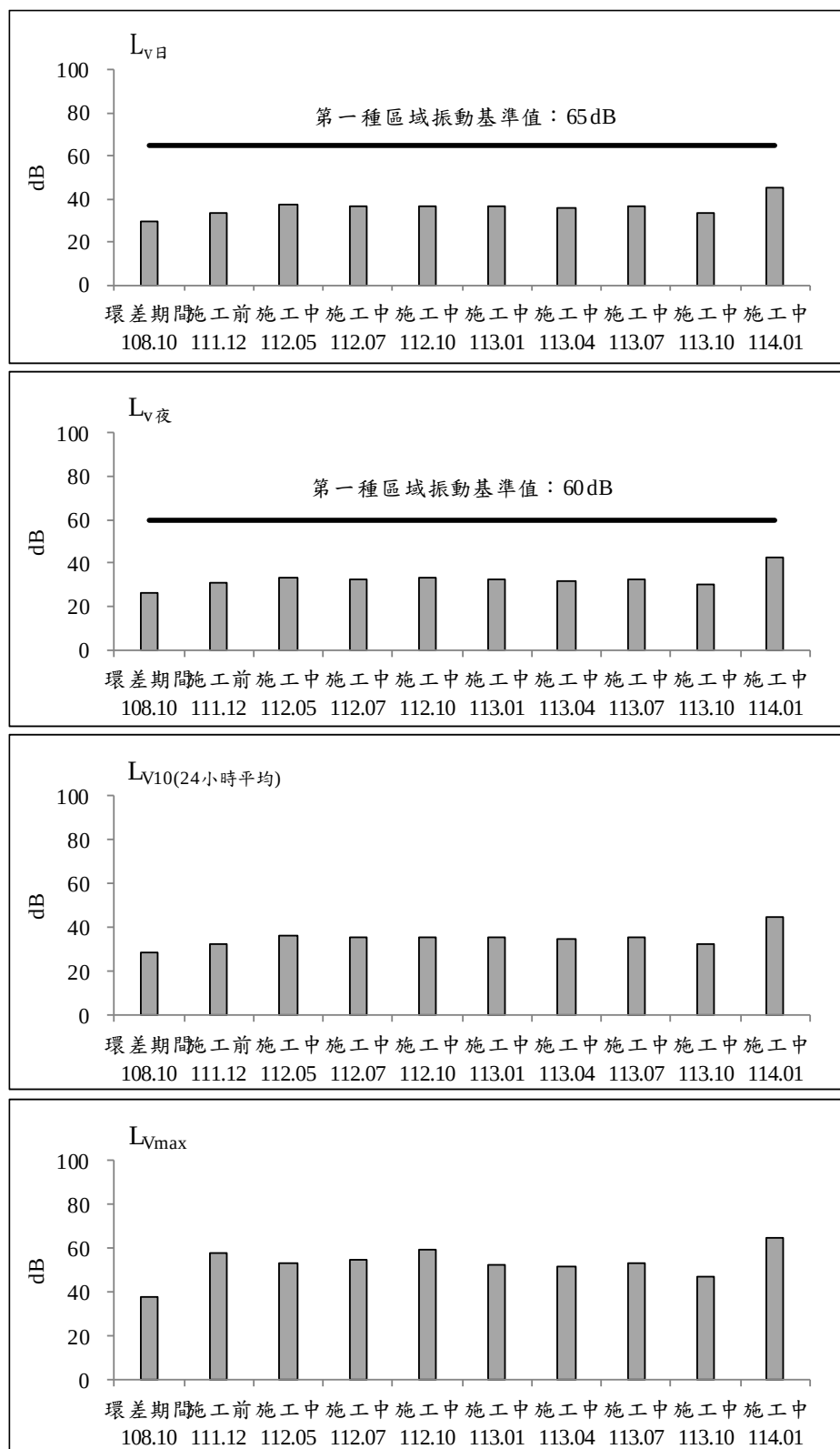
圖 2.2-8 台北星州社區測站歷次振動監測之各項測值變化圖(平日)
