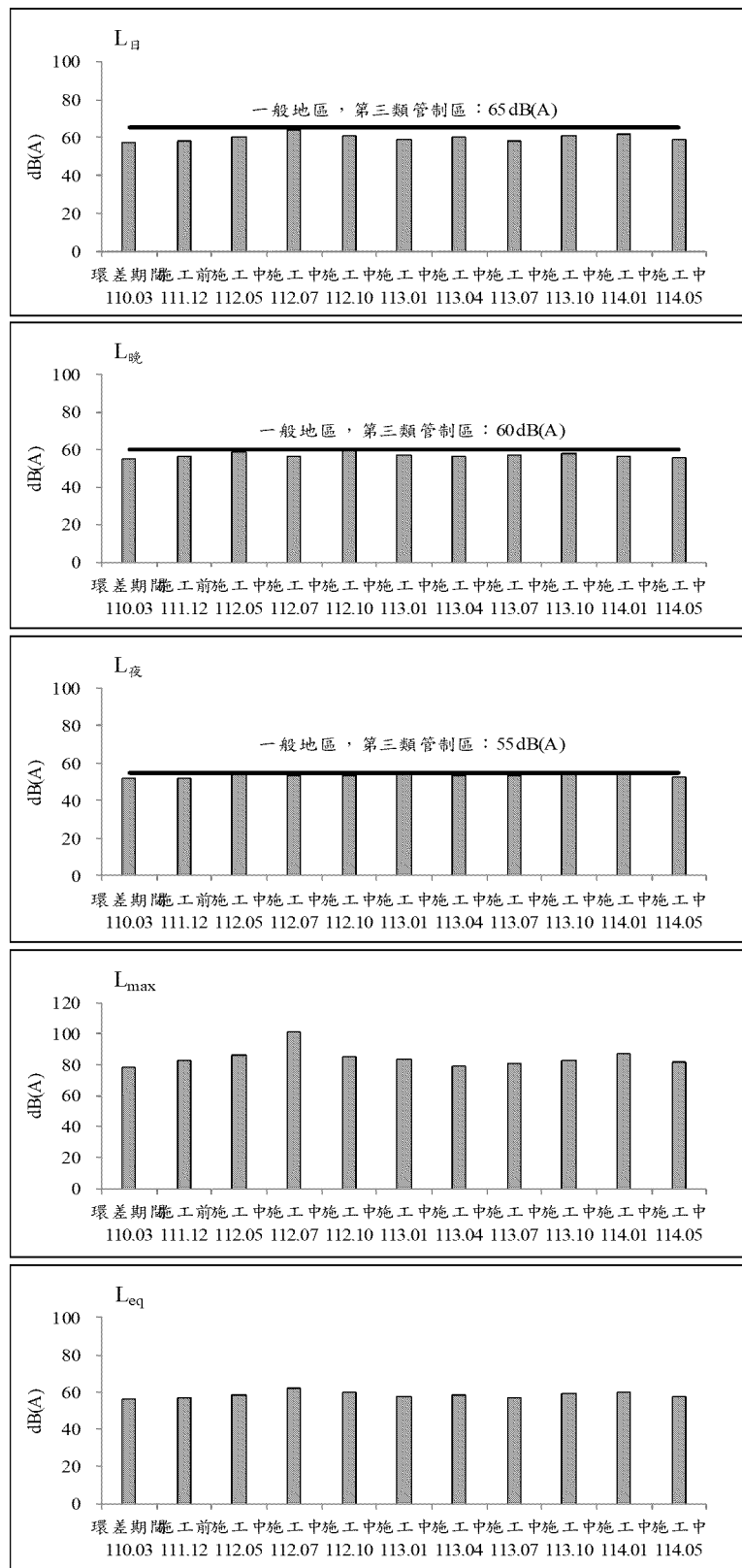
圖 2.2-1 德音國民小學測站歷次噪音監測之各項測值變化圖(假日)
