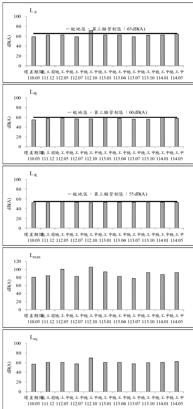
圖 2.2-2 德音國民小學測站歷次噪音監測之各項測值變化圖(平日)
