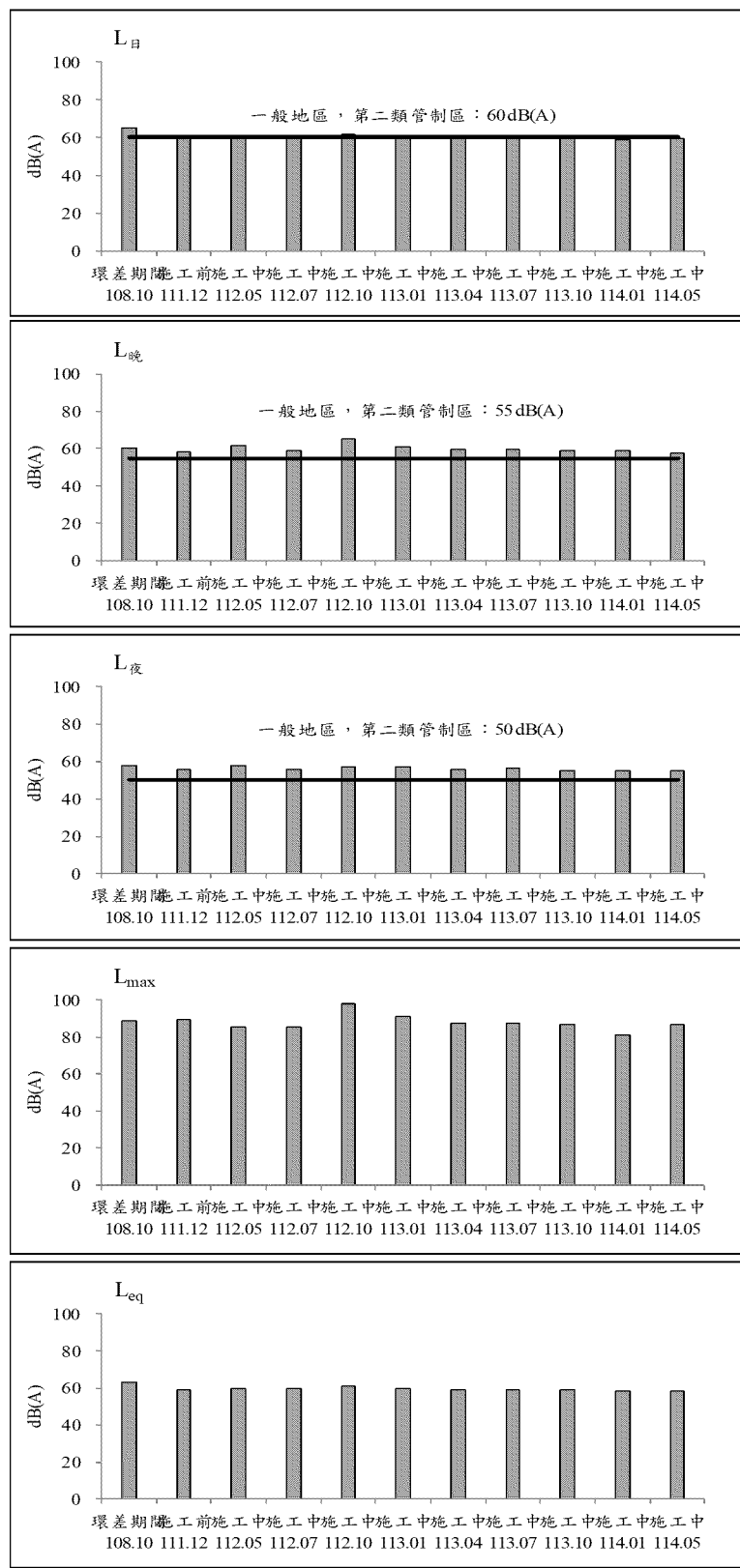
圖 2.2-3 台北星州社區測站歷次噪音監測之各項測值變化圖(假日)
