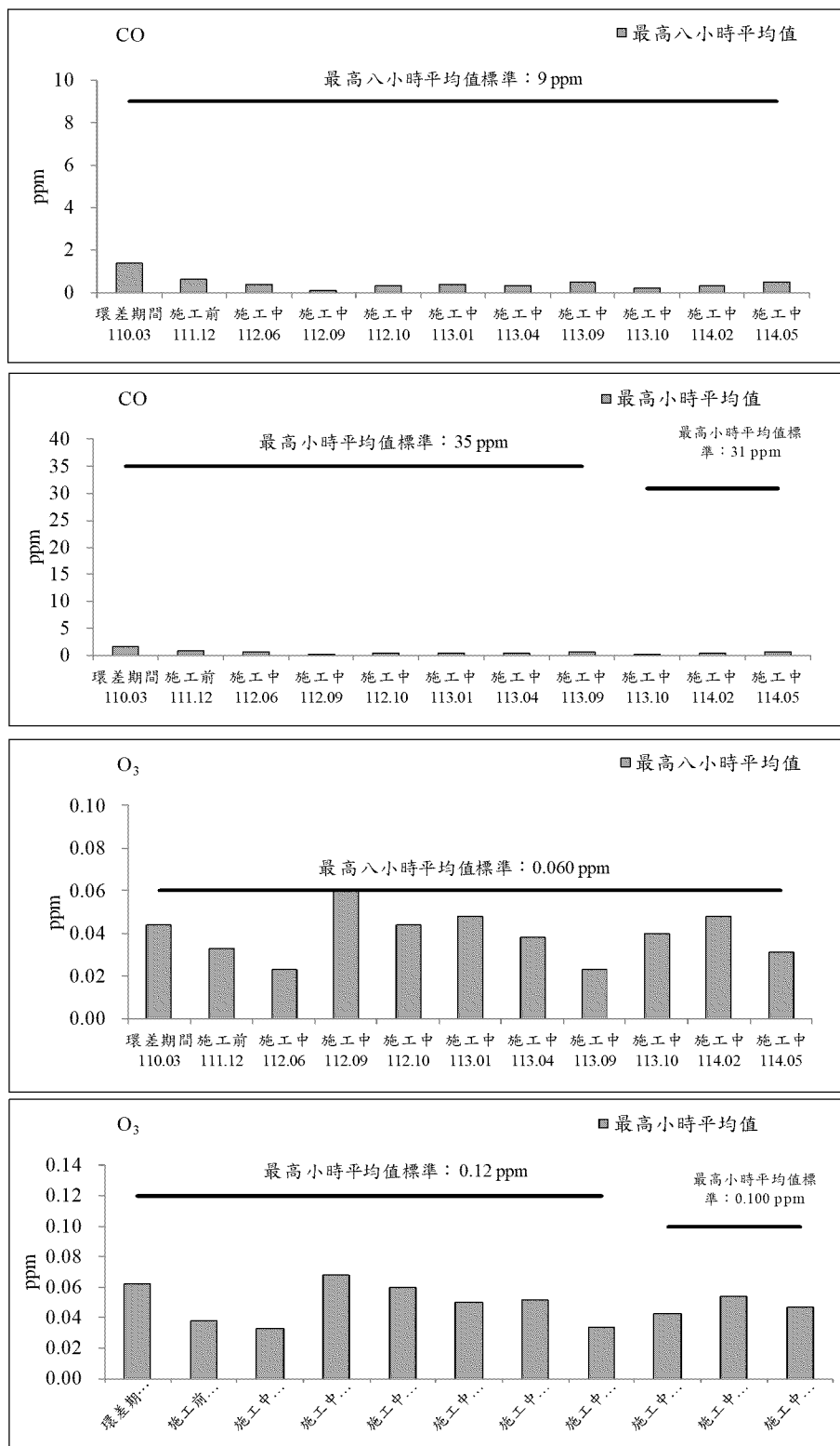
圖 2.1-2 準休閒農場測站歷次空氣品質監測之各項測值變化圖(續 2)
