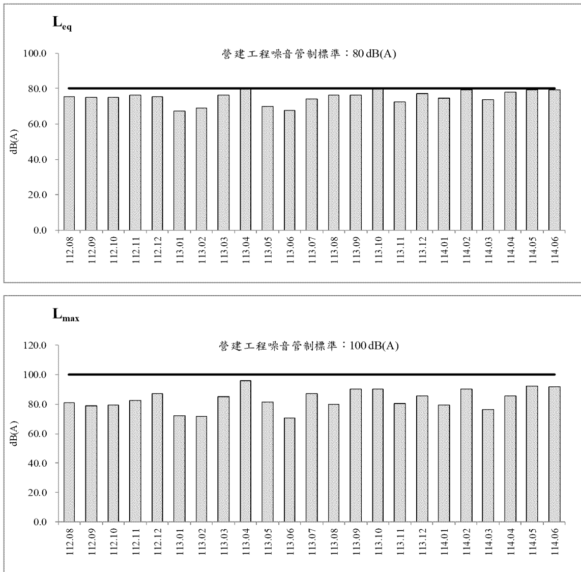
圖 2.4-1 歷次營建工程噪音監測之各項測值變化圖
