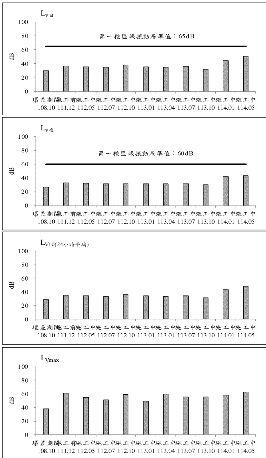
圖 2.2-7 台北星州社區測站歷次振動監測之各項測值變化圖(假日)
