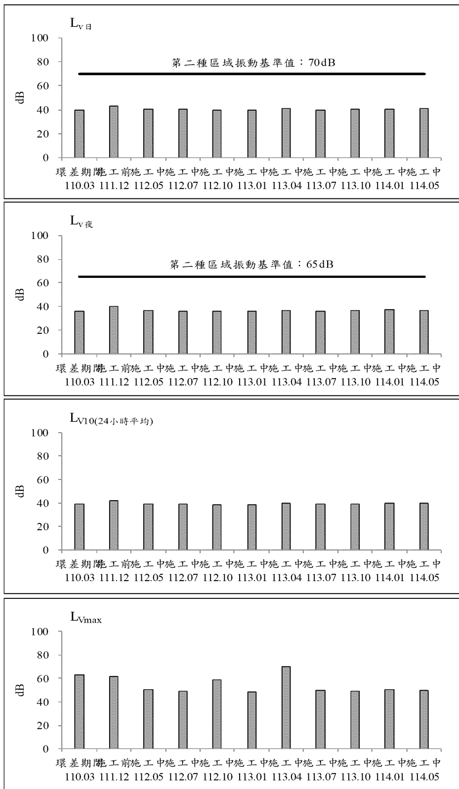
圖 2.2-5 德音國民小學測站歷次振動監測之各項測值變化圖(假日)
