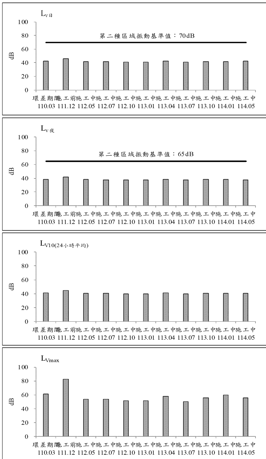
圖 2.2-6 德音國民小學測站歷次振動監測之各項測值變化圖(平日)
