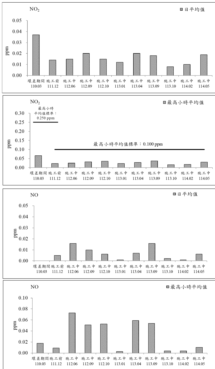
圖 2.1-2 準休閒農場測站歷次空氣品質監測之各項測值變化圖(續 1)
