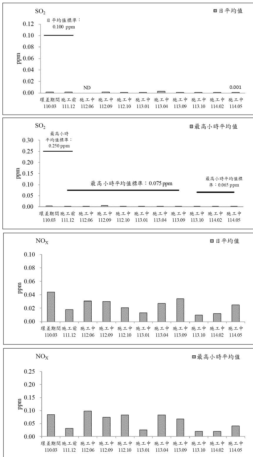
圖 2.1-2 準休閒農場測站歷次空氣品質監測之各項測值變化圖
