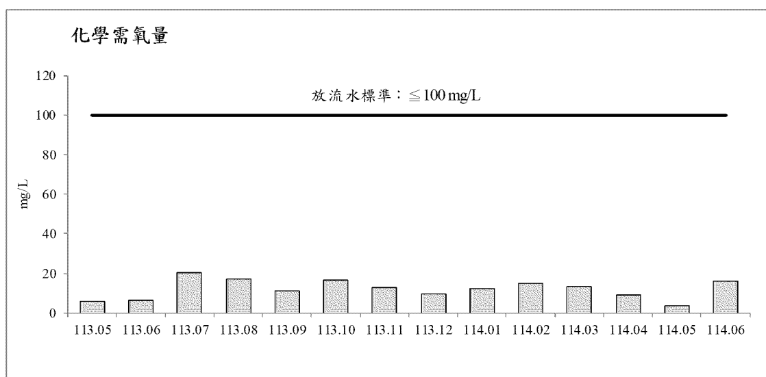
圖 2.5-1 工區放流水監測之各項測值變化圖(續)
