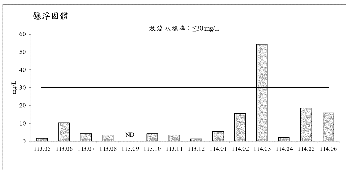
圖 2.5-1 工區放流水監測之各項測值變化圖
