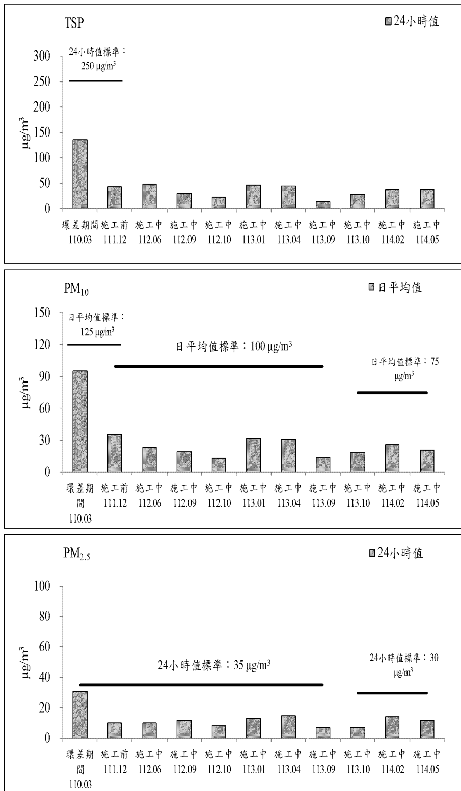
圖 2.1-2 準休閒農場測站歷次空氣品質監測之各項測值變化圖(續 3)
