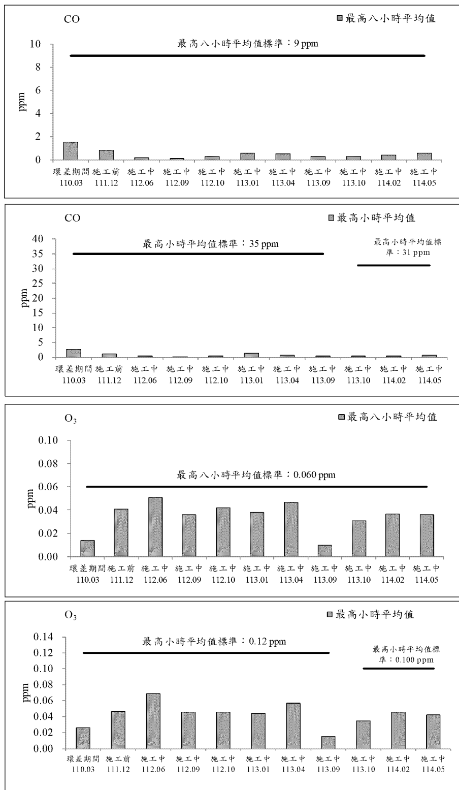
圖 2.1-1 德音國民小學測站歷次空氣品質監測之各項測值變化圖(續 2)
