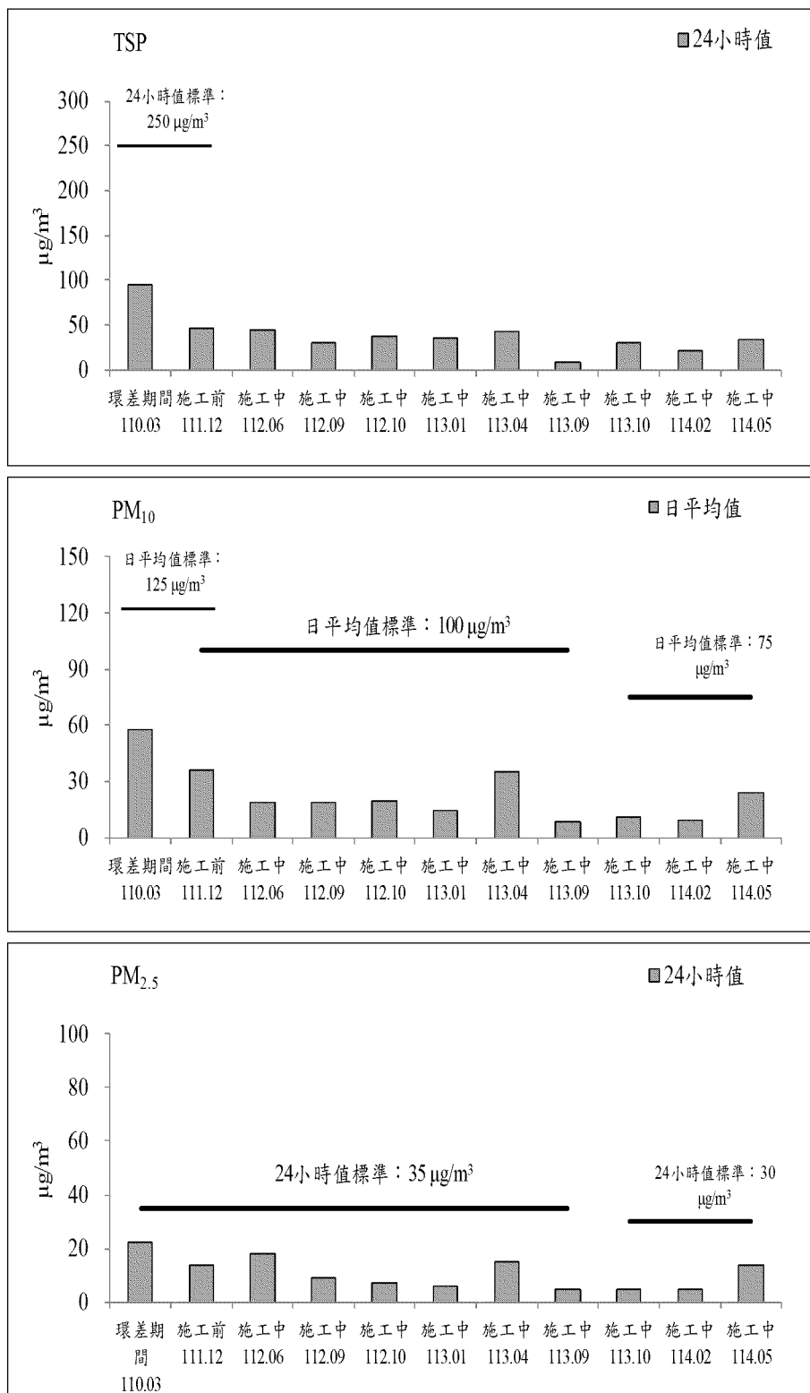
圖 2.1-1 德音國民小學測站歷次空氣品質監測之各項測值變化圖(續 3)
