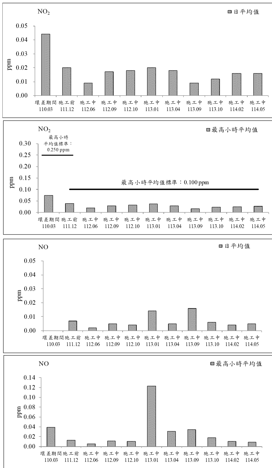
圖 2.1-1 德音國民小學測站歷次空氣品質監測之各項測值變化圖(續 1)
