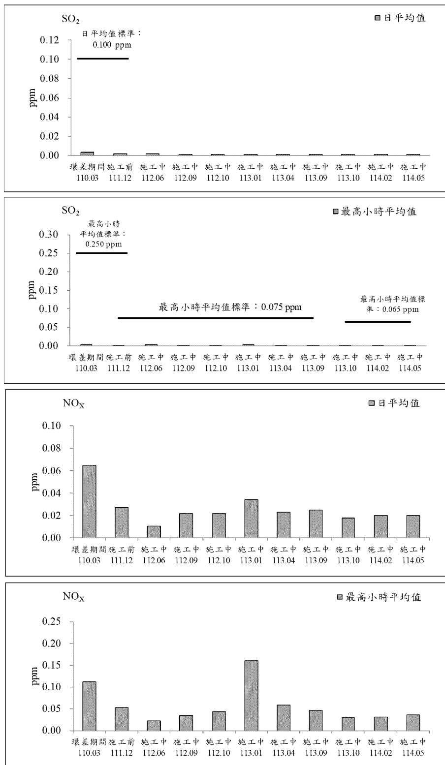
圖 2.1-1 德音國民小學測站歷次空氣品質監測之各項測值變化圖
