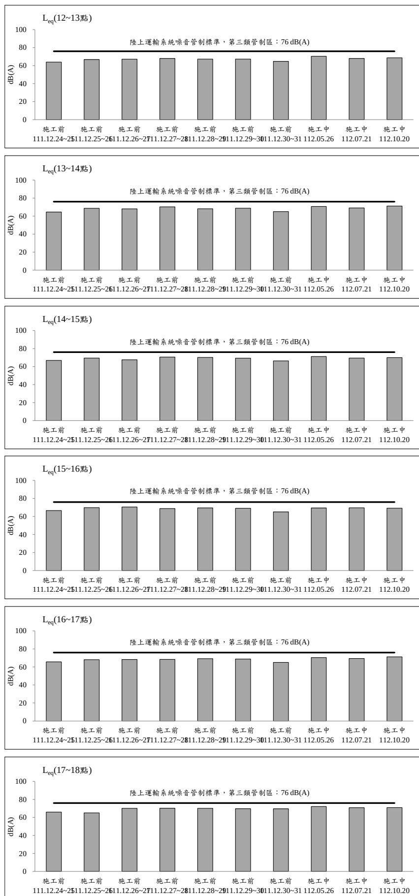
圖 2.2-6 金鑽公寓大廈測站歷次交通噪音監測之各項測值變化圖(平日) (續 2)
