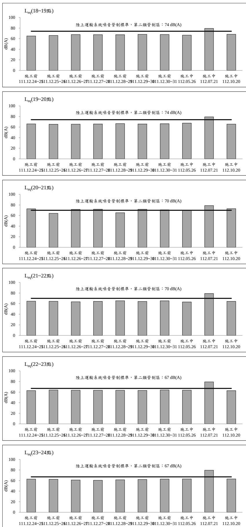
圖 2.2-2 成泰路台北星州社區聚落測站歷次交通噪音監測之各項測值 變化圖(平日)(續 3)
