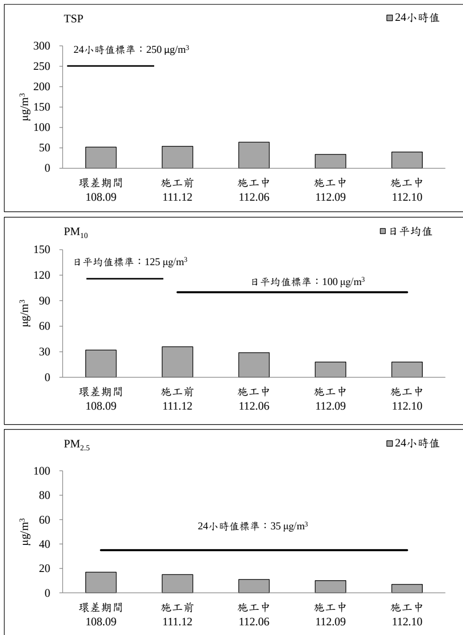
圖 2.1-1 成泰路台北星州社區聚落測站歷次空氣品質監測之各項測值變化圖(續 3)
