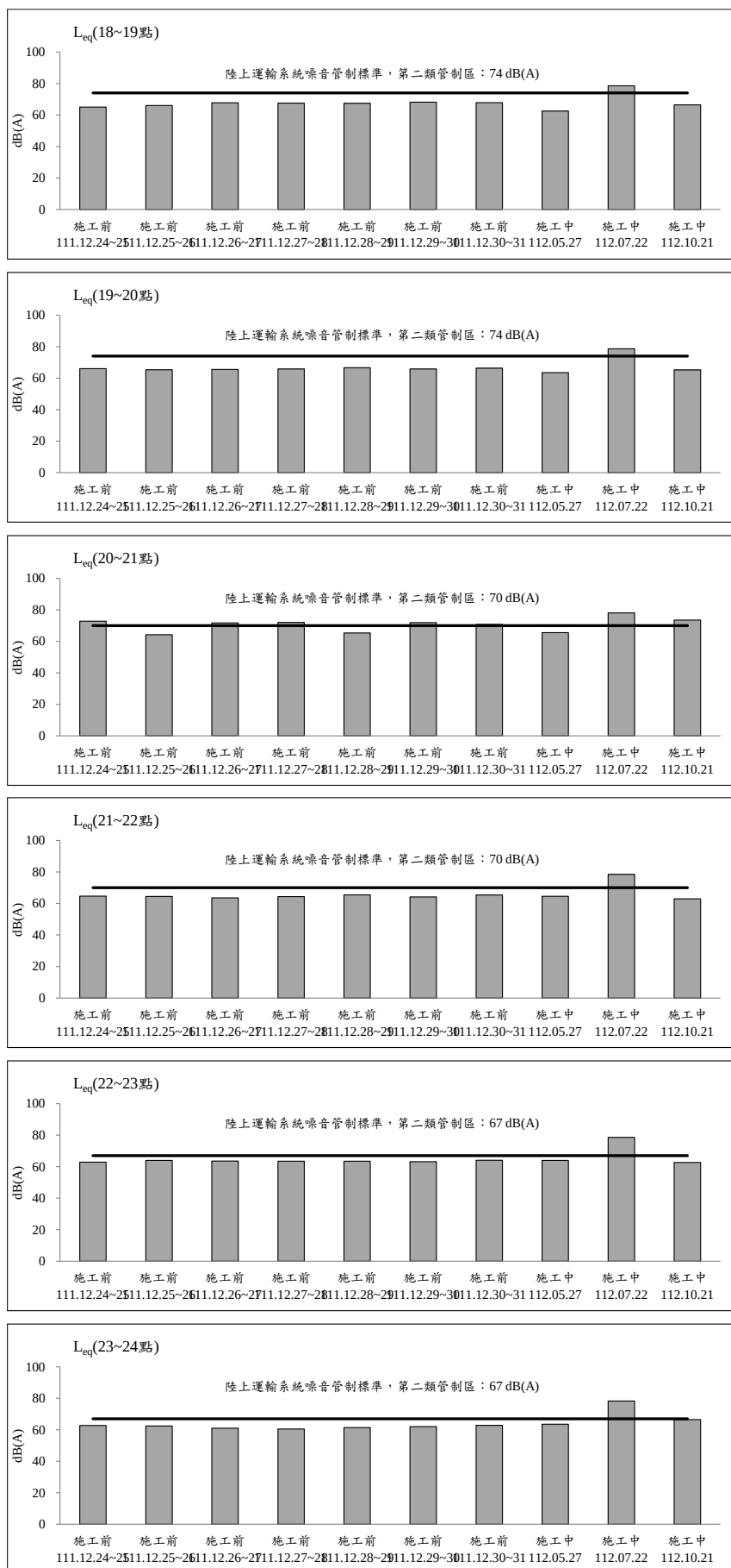
圖 2.2-1 成泰路台北星州社區聚落測站歷次交通噪音監測之各項測值變化圖(假日)(續 3)
