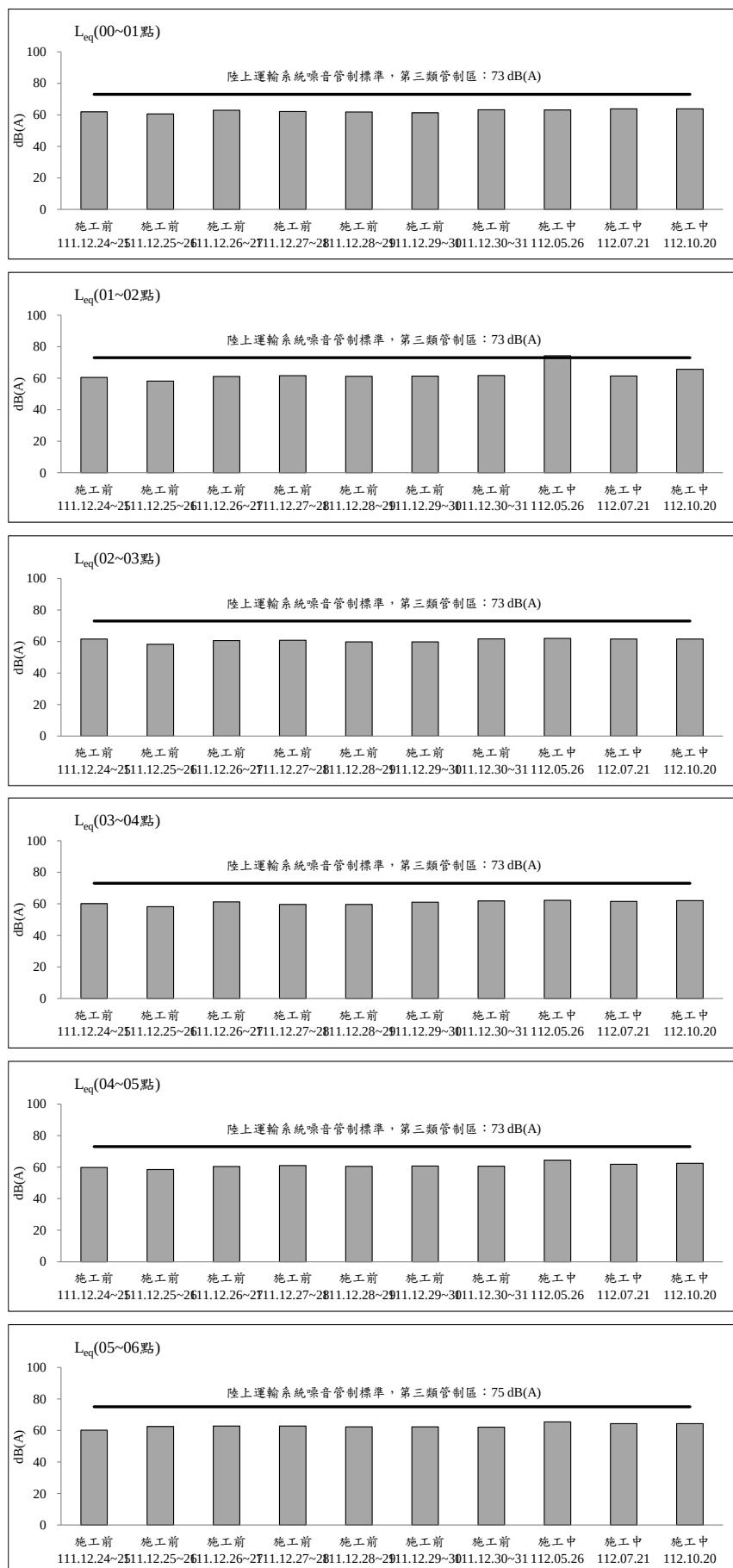
圖 2.2-6 金鑽公寓大廈測站歷次交通噪音監測之各項測值變化圖(平日)
