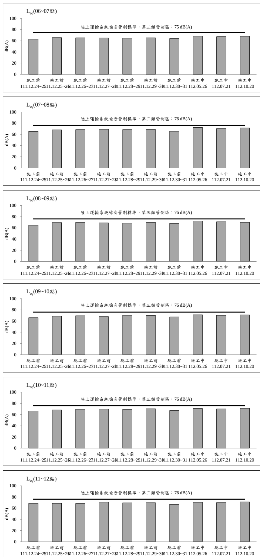
圖 2.2-6 金鑽公寓大廈測站歷次交通噪音監測之各項測值變化圖(平日) (續 1)
