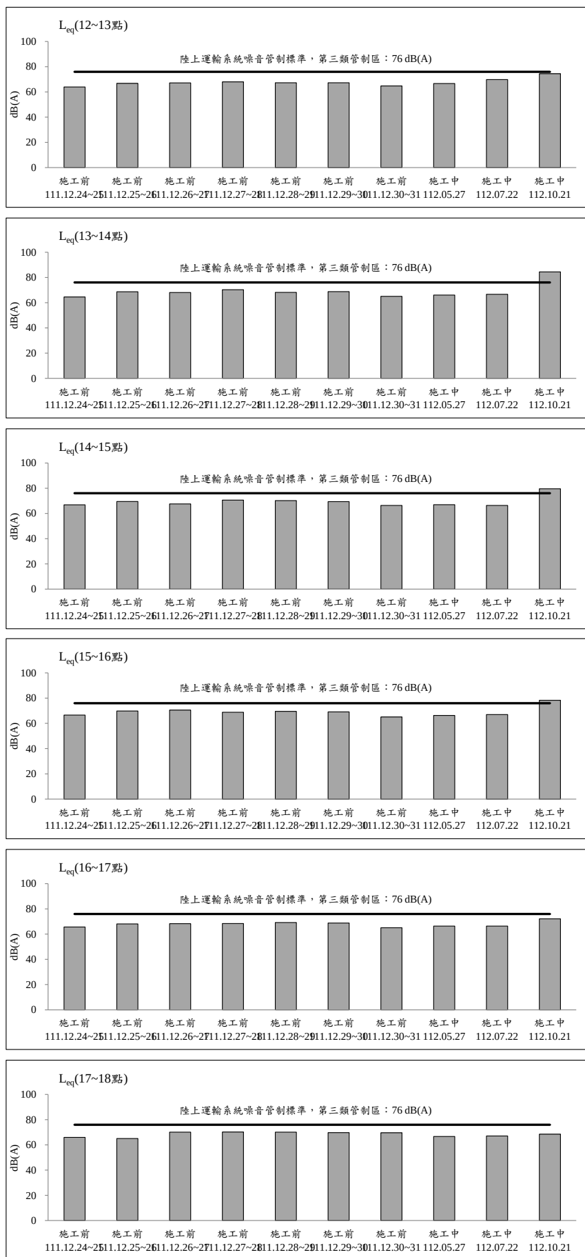
圖 2.2-5 金鑽公寓大廈測站歷次交通噪音監測之各項測值變化圖(假日) (續 2)
