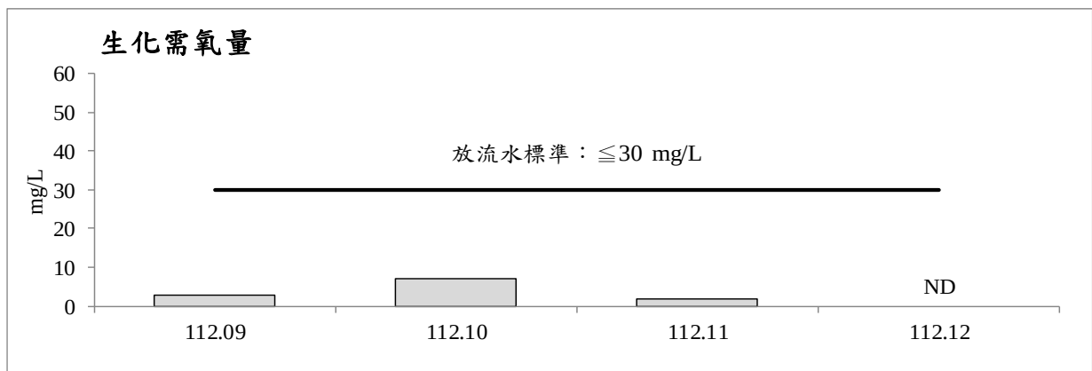
圖 2.5-1 工區放流水監測之各項測值變化圖
