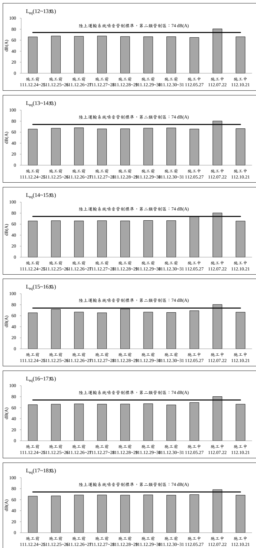
圖 2.2-1 成泰路台北星州社區聚落測站歷次交通噪音監測之各項測值 變化圖(假日)(續 2)
