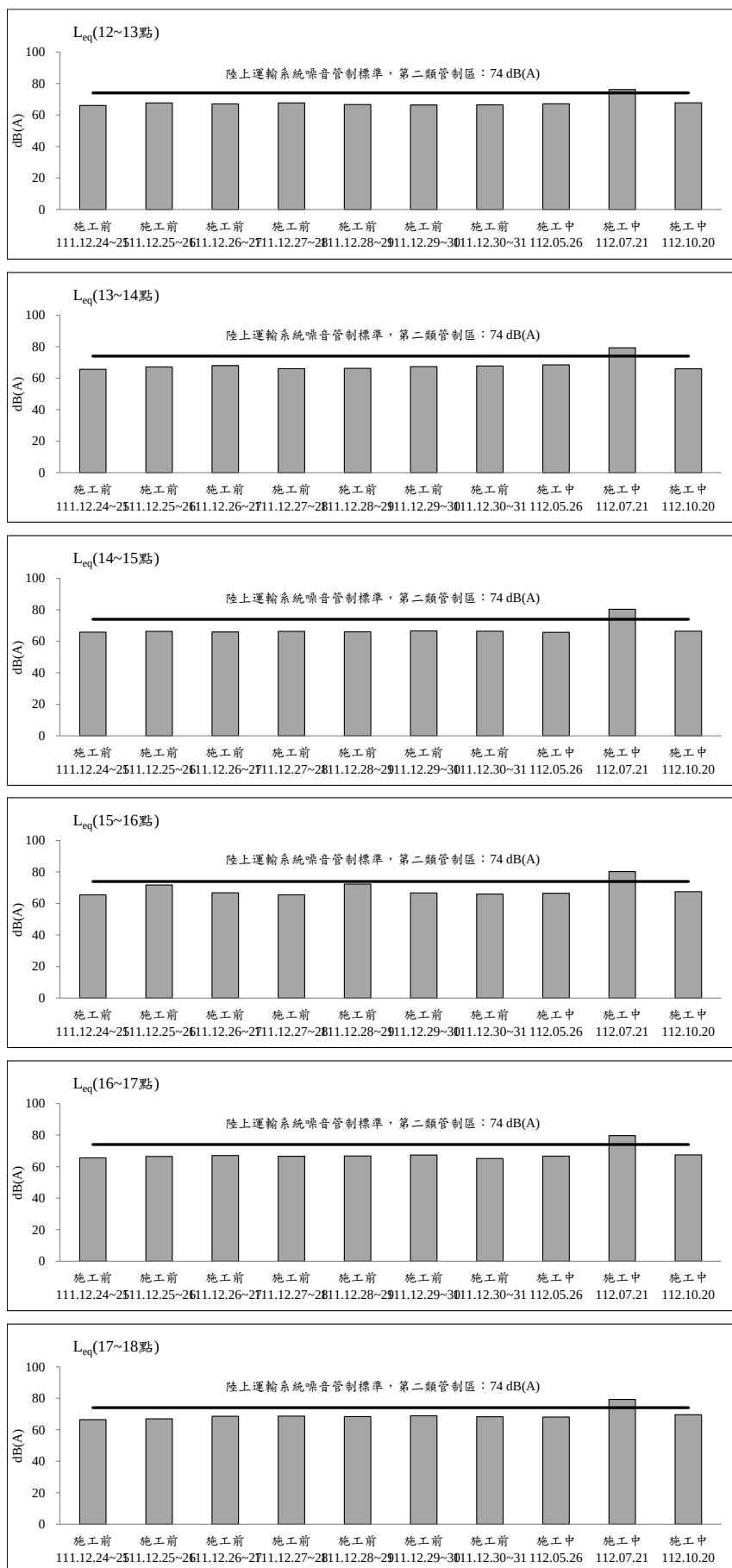
圖 2.2-2 成泰路台北星州社區聚落測站歷次交通噪音監測之各項測值變化圖(平日)(續 2)
