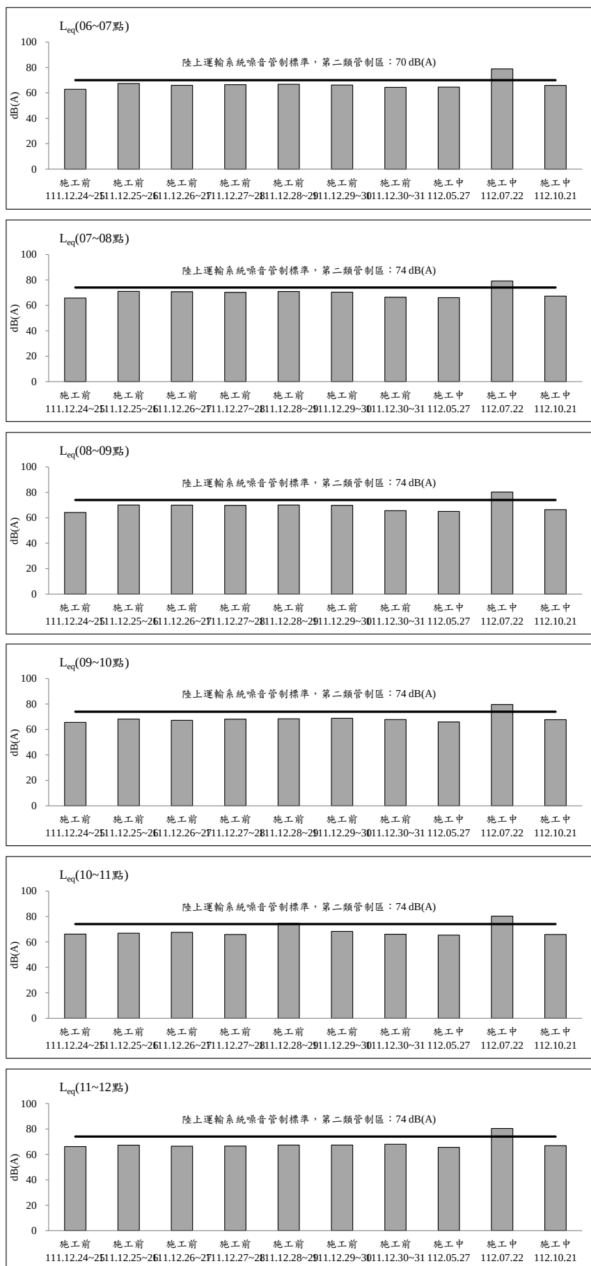
圖 2.2-1 成泰路台北星州社區聚落測站歷次交通噪音監測之各項測值變化圖(假日)(續 1)
