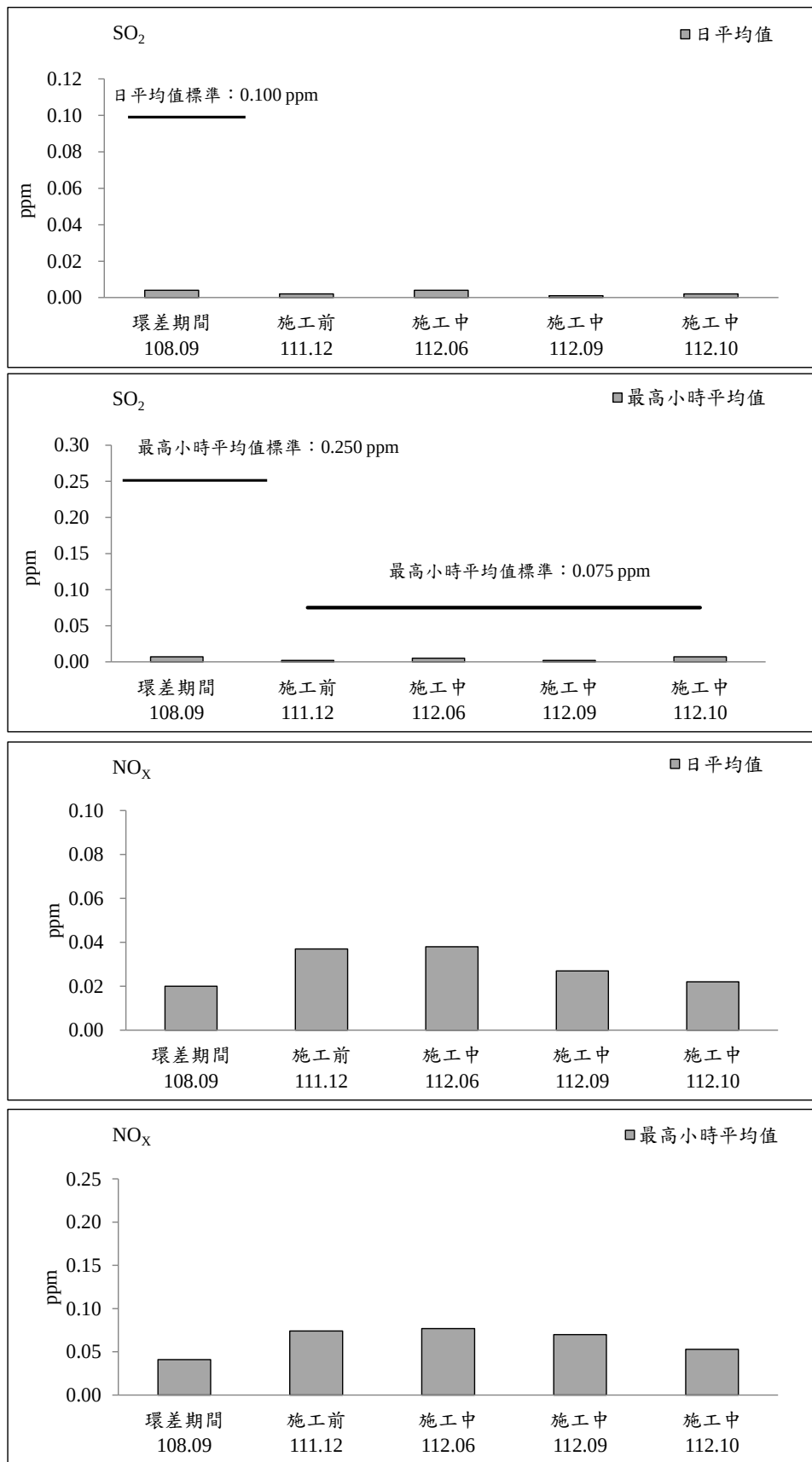
圖 2.1-1 成泰路台北星州社區聚落測站歷次空氣品質監測之各項測值變化圖
