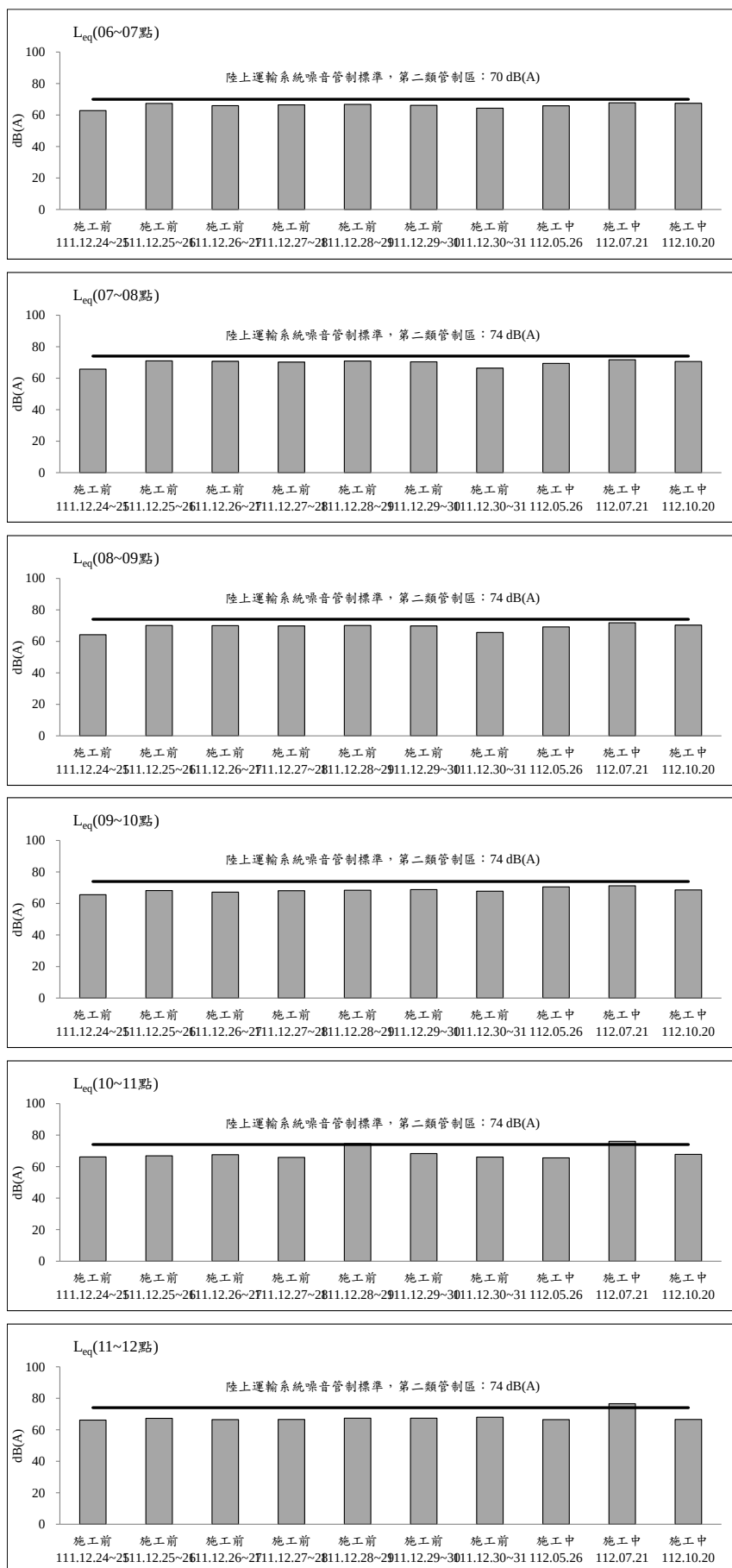
圖 2.2-2 成泰路台北星州社區聚落測站歷次交通噪音監測之各項測值 變化圖(平日)(續 1)
