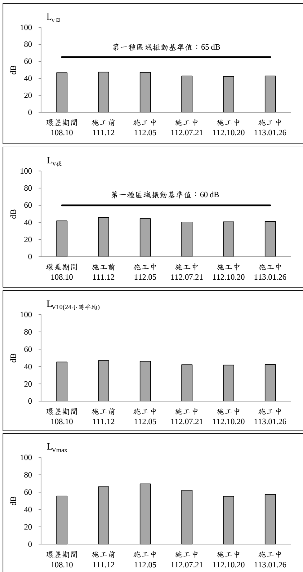
圖 2.2-10 新五路側商家測站歷次振動監測之各項測值變化圖(平日)
