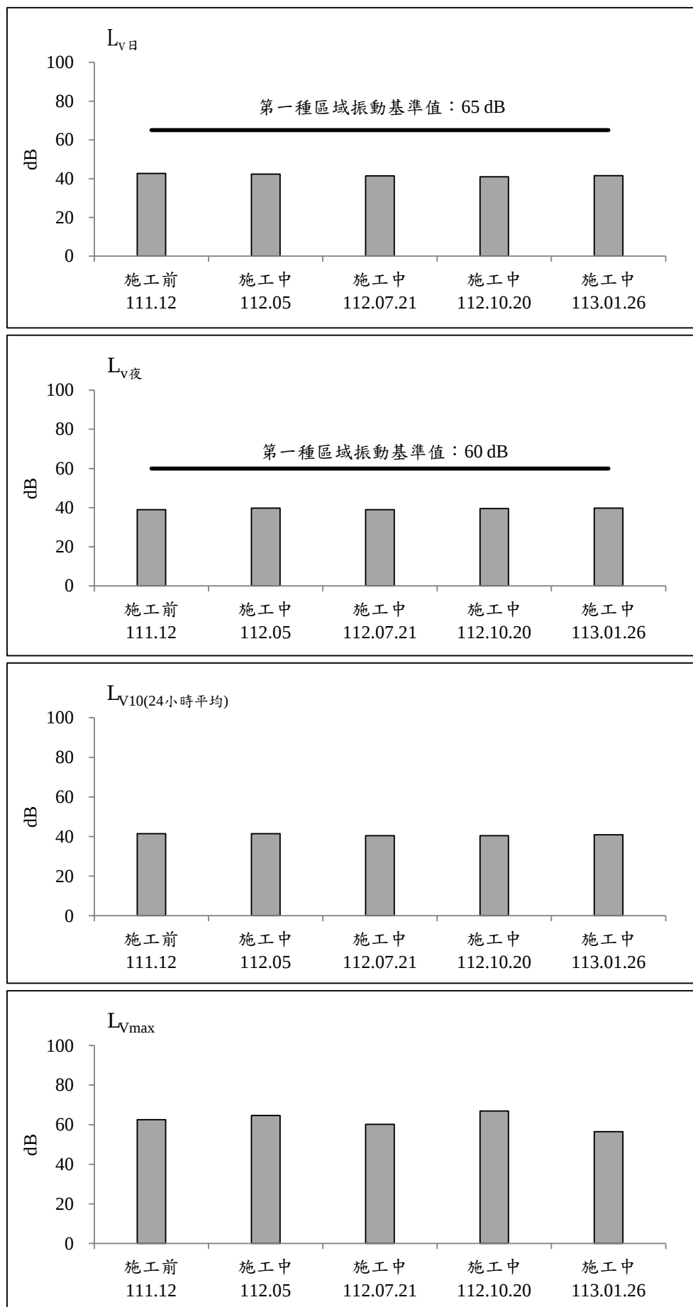
圖 2.2-12 金鑽公寓大廈測站歷次振動監測之各項測值變化圖(平日)
