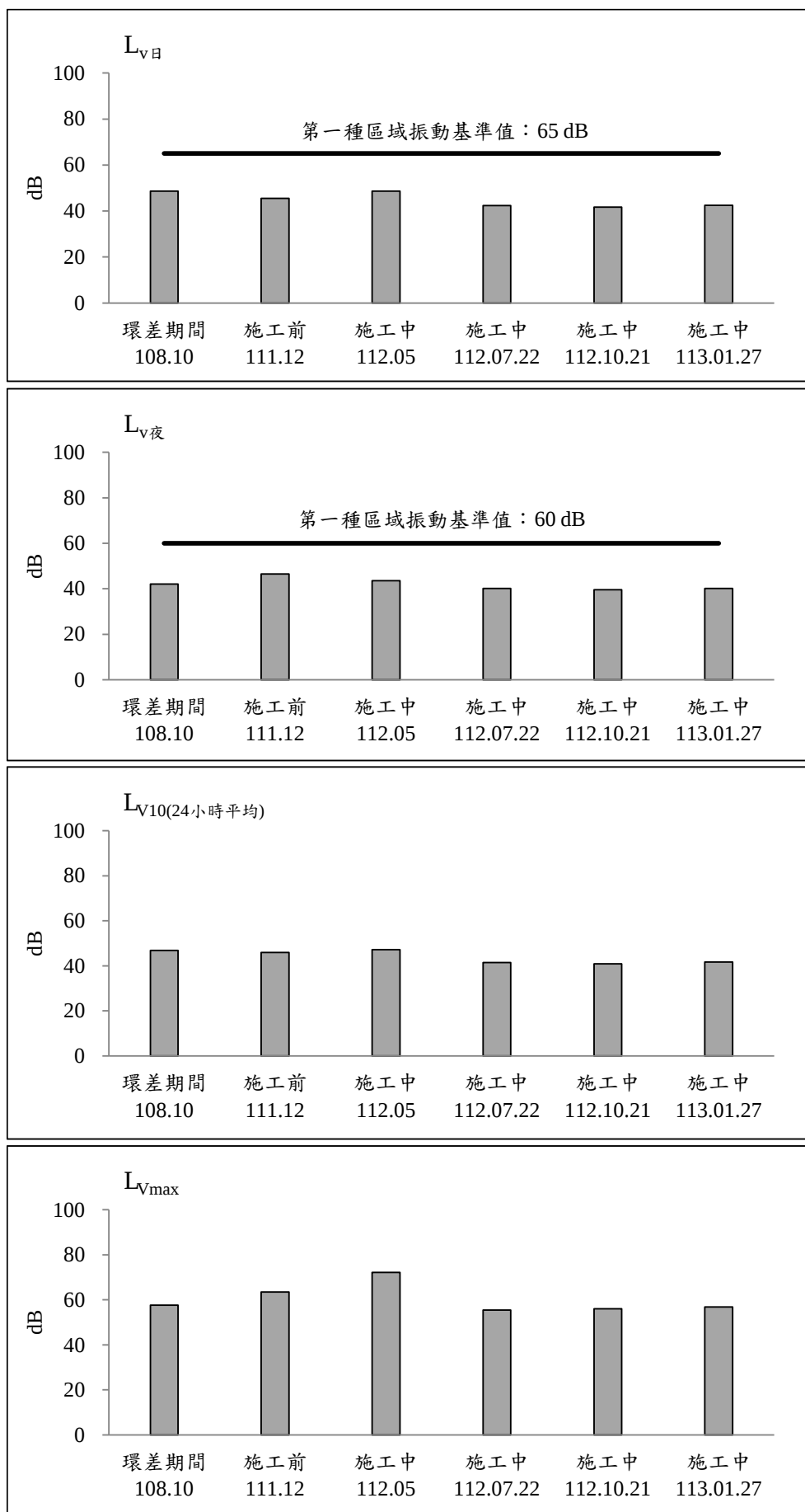
圖 2.2-9 新五路側商家測站歷次振動監測之各項測值變化圖(假日)
