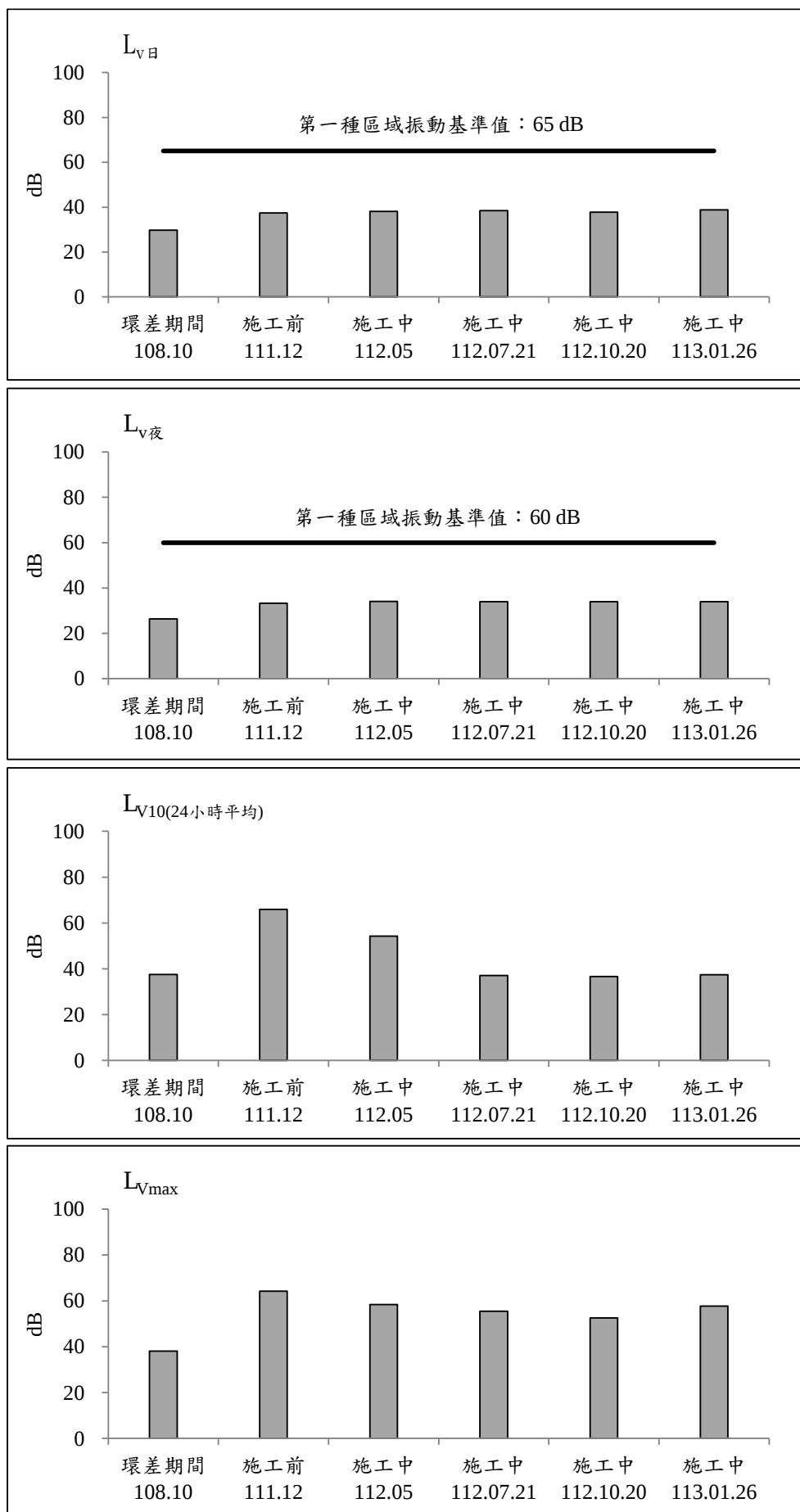
圖 2.2-8 成泰路台北星州社區測站歷次振動監測之各項測值變化圖(平日)
