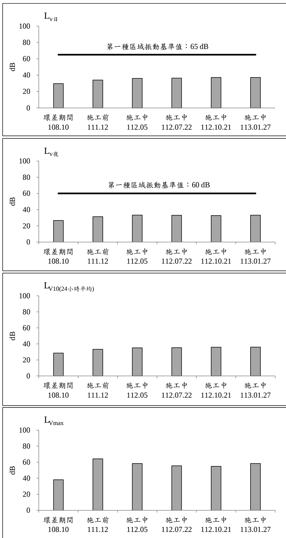
圖 2.2-7 成泰路台北星州社區測站歷次振動監測之各項測值變化圖(假日)
