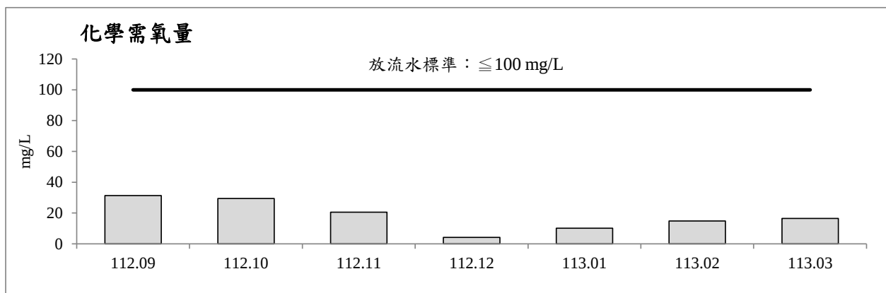
圖 2.5-1 工區放流水監測之各項測值變化圖(續)
