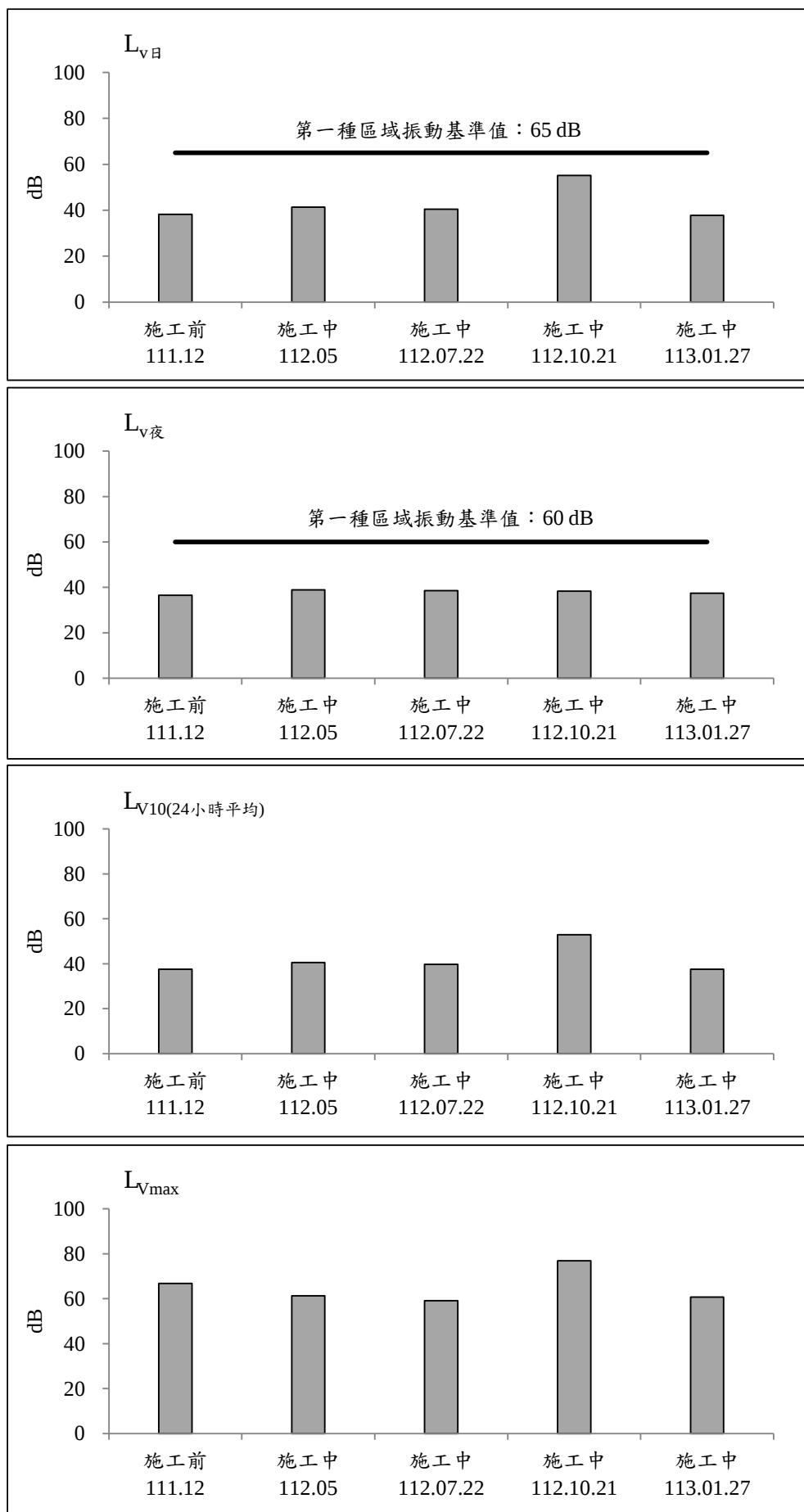
圖 2.2-11 金鑽公寓大廈測站歷次振動監測之各項測值變化圖(假日)
