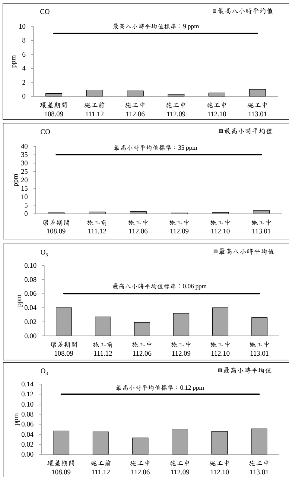
圖 2.1-1 成泰路台北星州社區聚落測站歷次空氣品質監測之各項測值變化圖(續 2)
