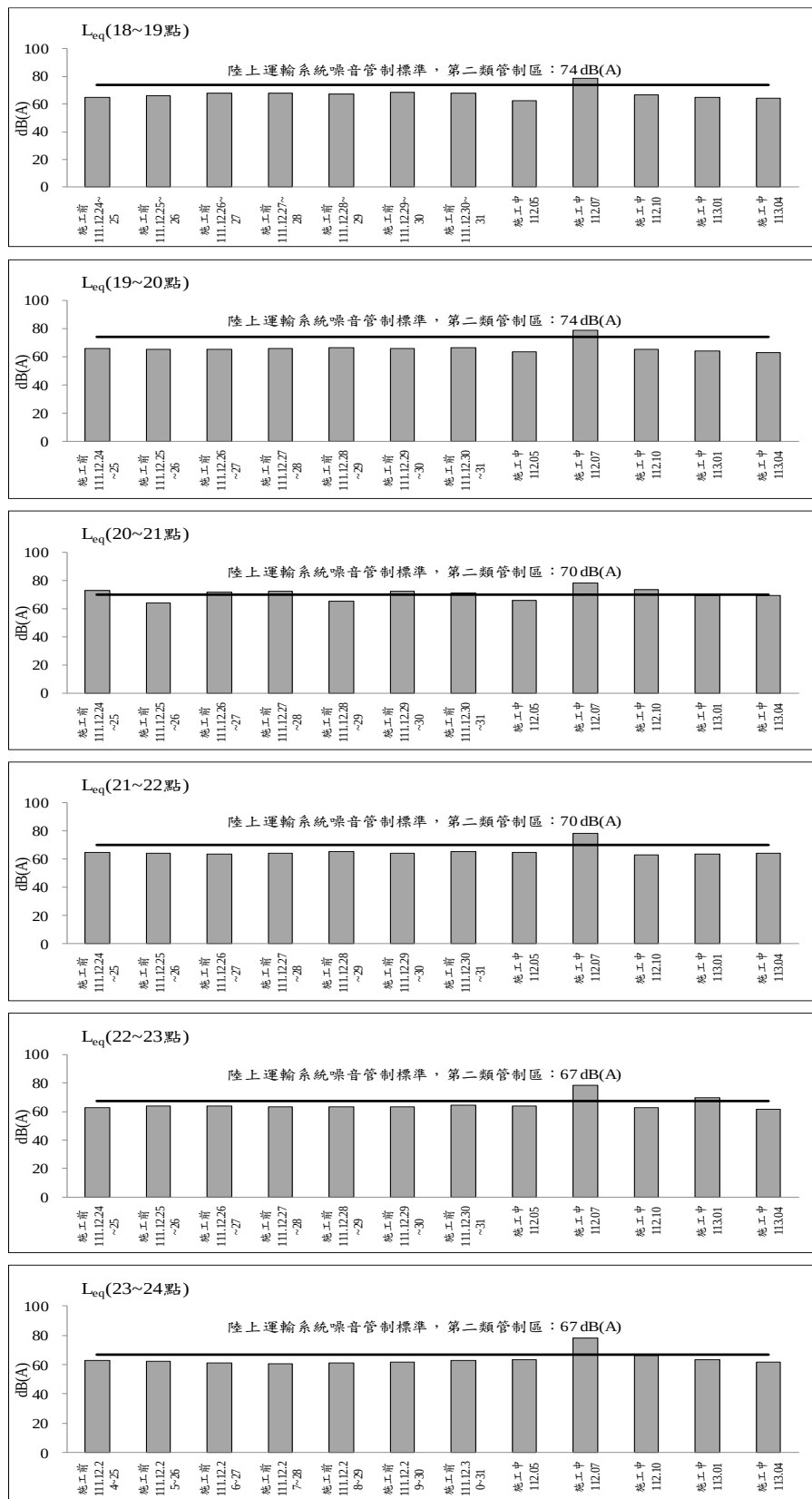
圖 2.2-1 成泰路台北星州社區聚落測站歷次交通噪音監測之各項測值變化圖(假日)(續 3)
