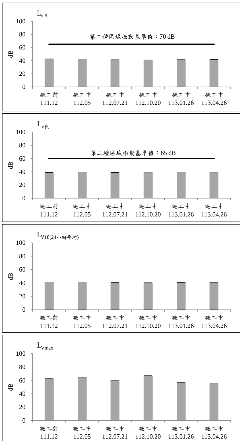
圖 2.2-12 金鑽公寓大廈測站歷次振動監測之各項測值變化圖(平日)
