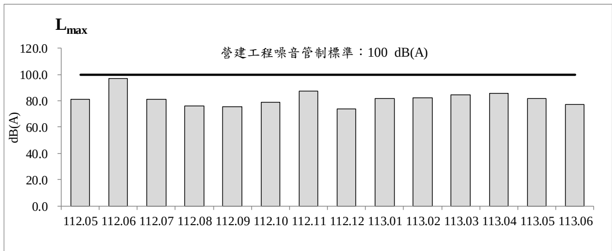
圖 2.4-1 歷次營建工程噪音監測之各項測值變化圖
