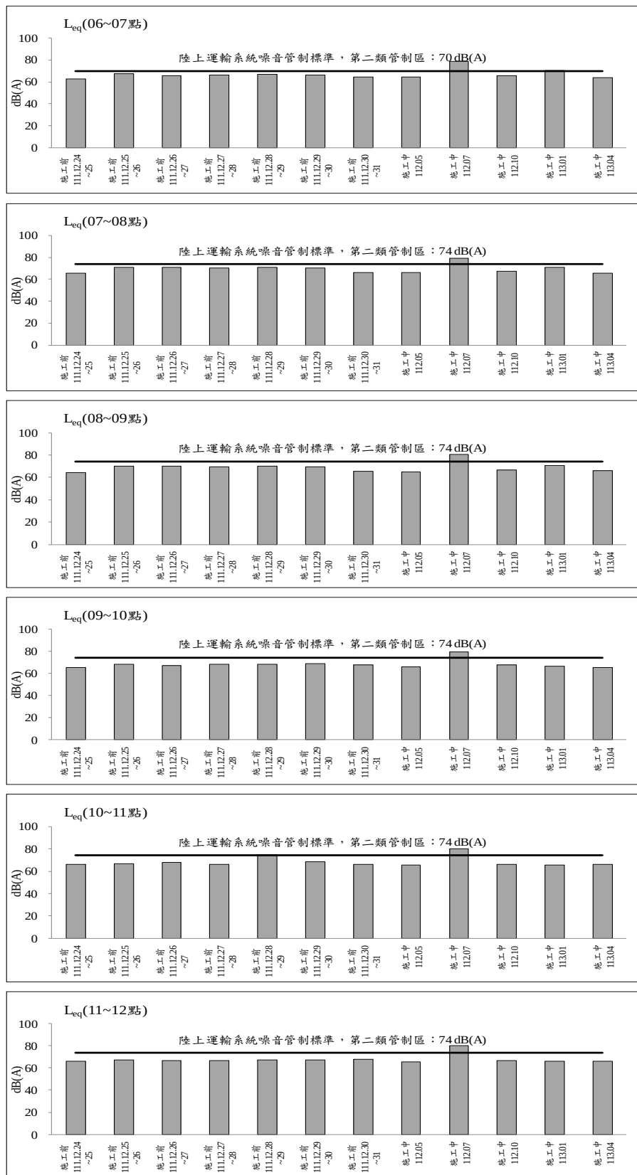
圖 2.2-1 成泰路台北星州社區聚落測站歷次交通噪音監測之各項測值變化圖(假日)(續 1)
