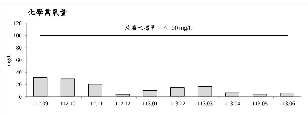
圖 2.5-1 工區放流水監測之各項測值變化圖(續)
