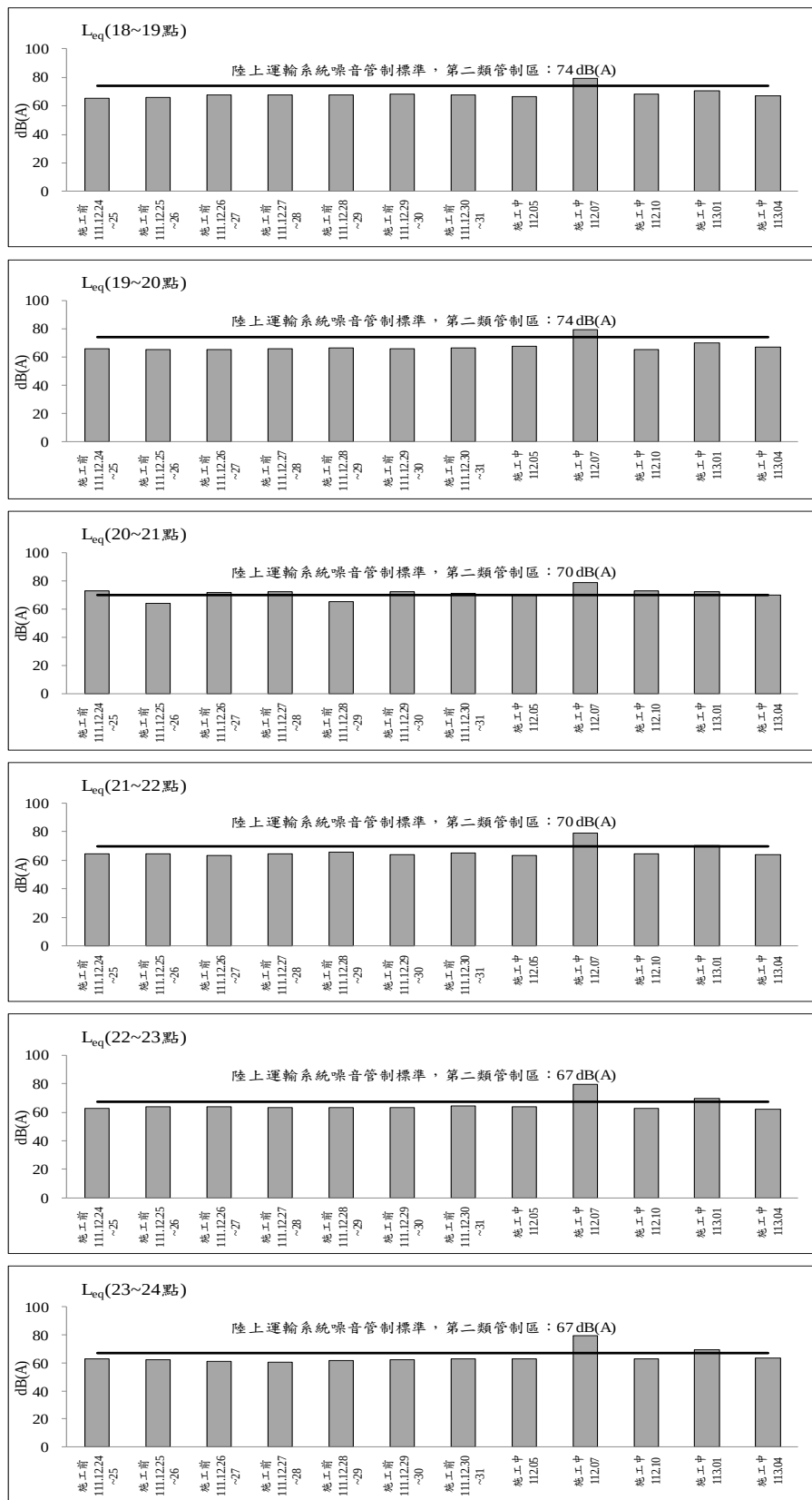
圖 2.2-2 成泰路台北星州社區聚落測站歷次交通噪音監測之各項測值變化圖(平日)(續 3)
