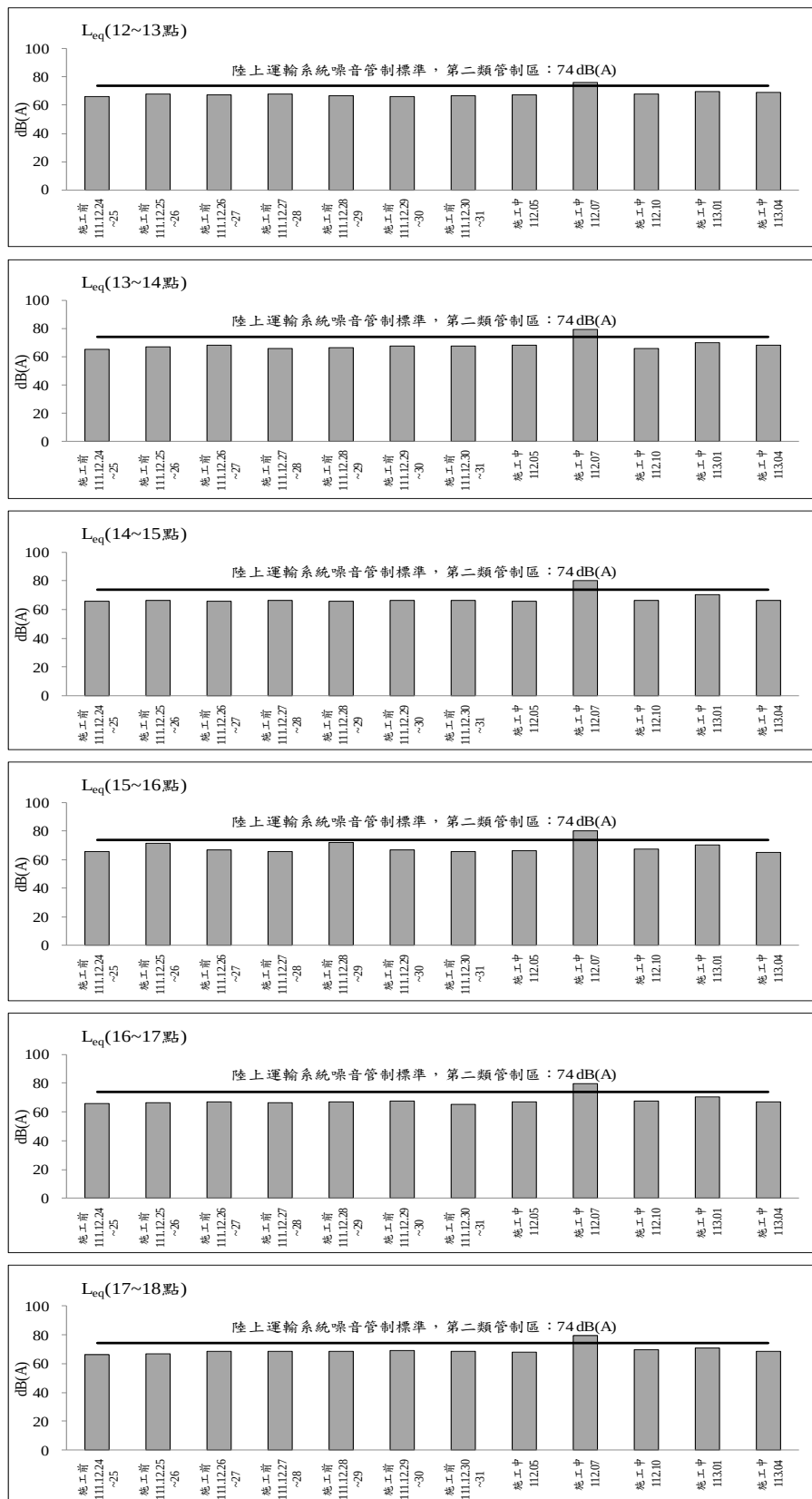
圖 2.2-2 成泰路台北星州社區聚落測站歷次交通噪音監測之各項測值變化圖(平日)(續 2)
