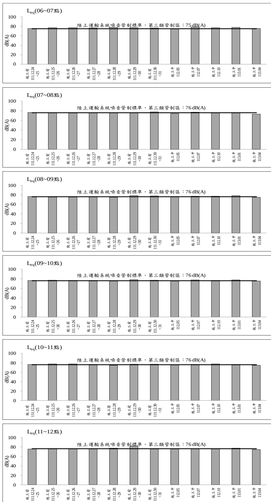
圖 2.2-4 新五路側商家測站歷次交通噪音監測之各項測值變化圖(平日)
