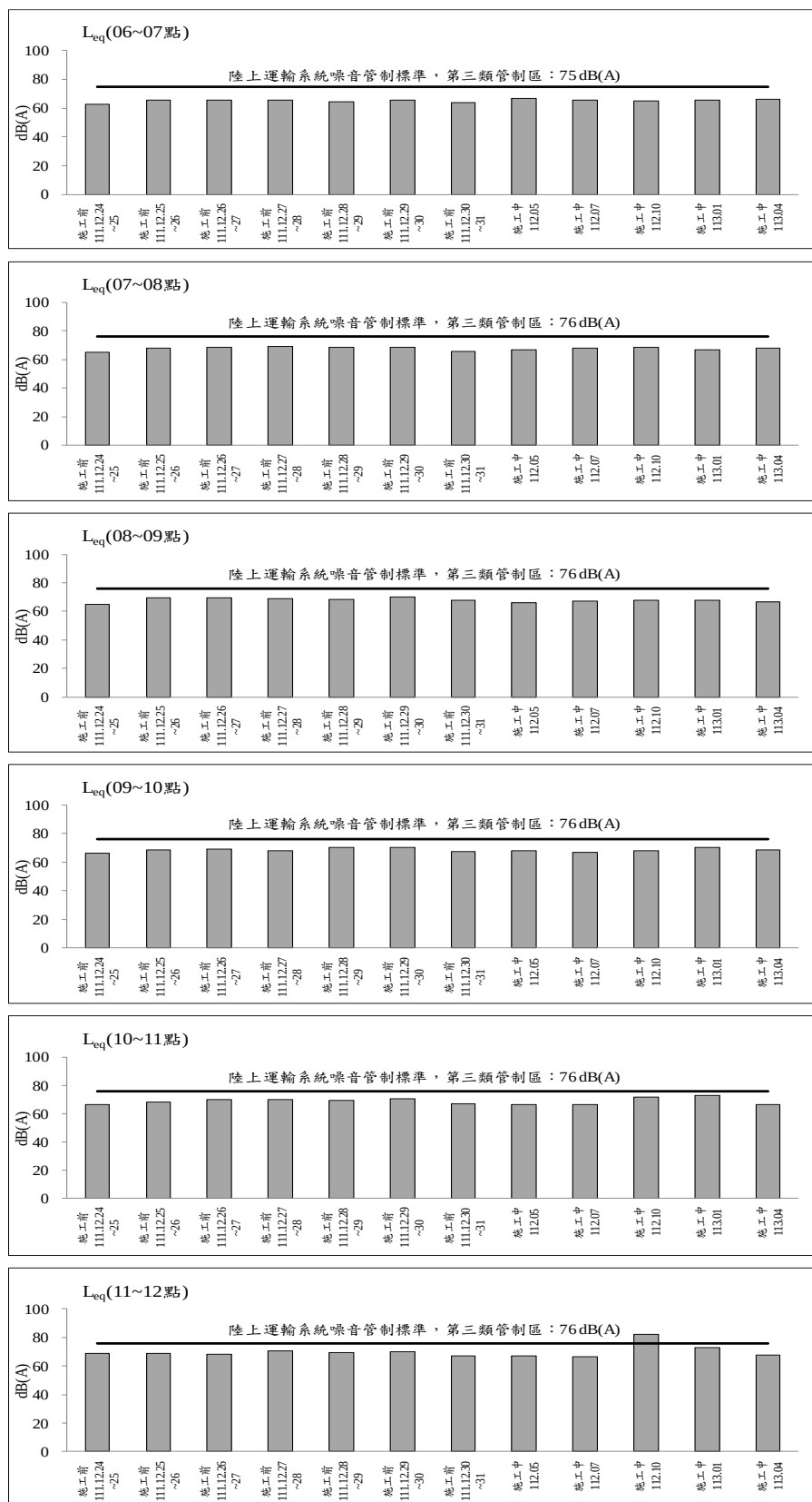
圖 2.2-5 金鑽公寓大廈測站歷次交通噪音監測之各項測值變化圖(假日)
