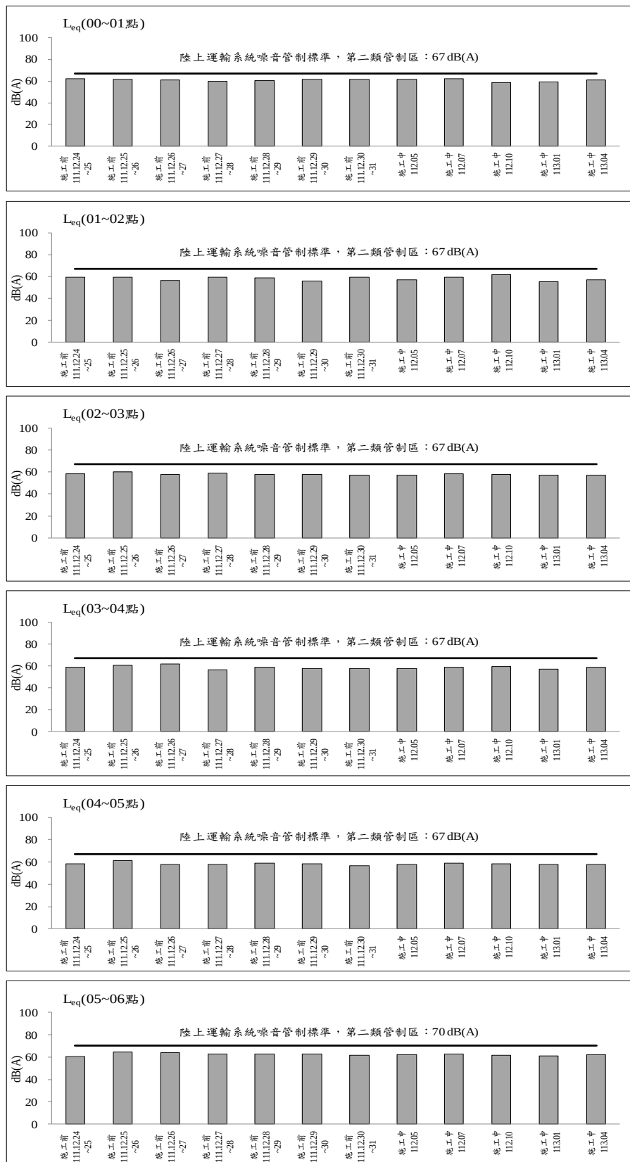
圖 2.2-2 成泰路台北星州社區聚落測站歷次交通噪音監測之各項測值變化圖(平日)
