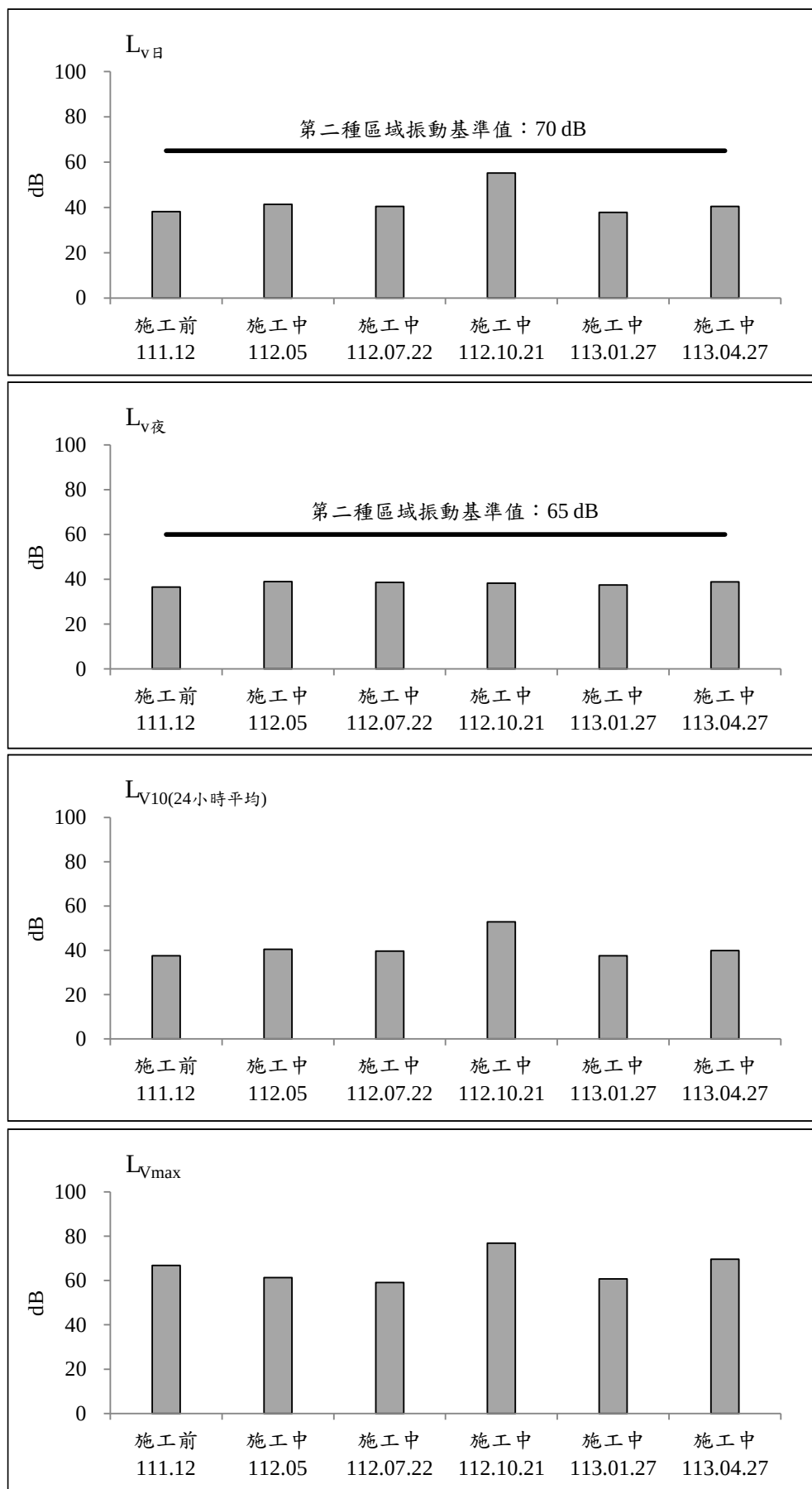
圖 2.2-11 金鑽公寓大廈測站歷次振動監測之各項測值變化圖(假日)
