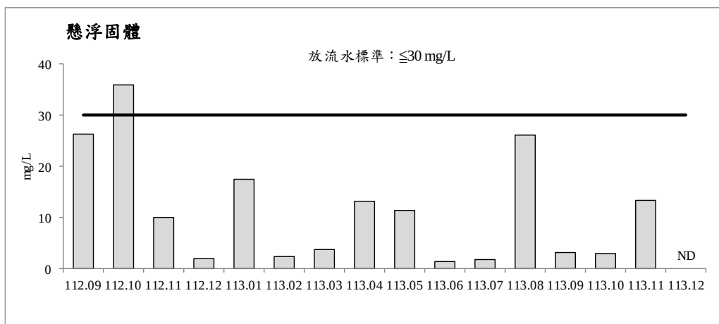
圖 2.5-1 工區放流水監測之各項測值變化圖
