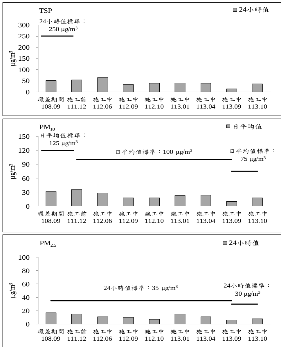
圖 2.1-1 成泰路台北星州社區聚落測站歷次空氣品質監測之各項測值變化圖(續 3)
