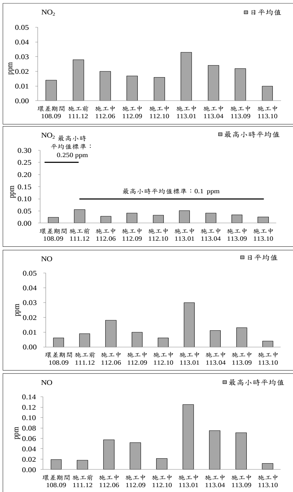
圖 2.1-1 成泰路台北星州社區聚落測站歷次空氣品質監測之各項測值變化圖(續 1)
