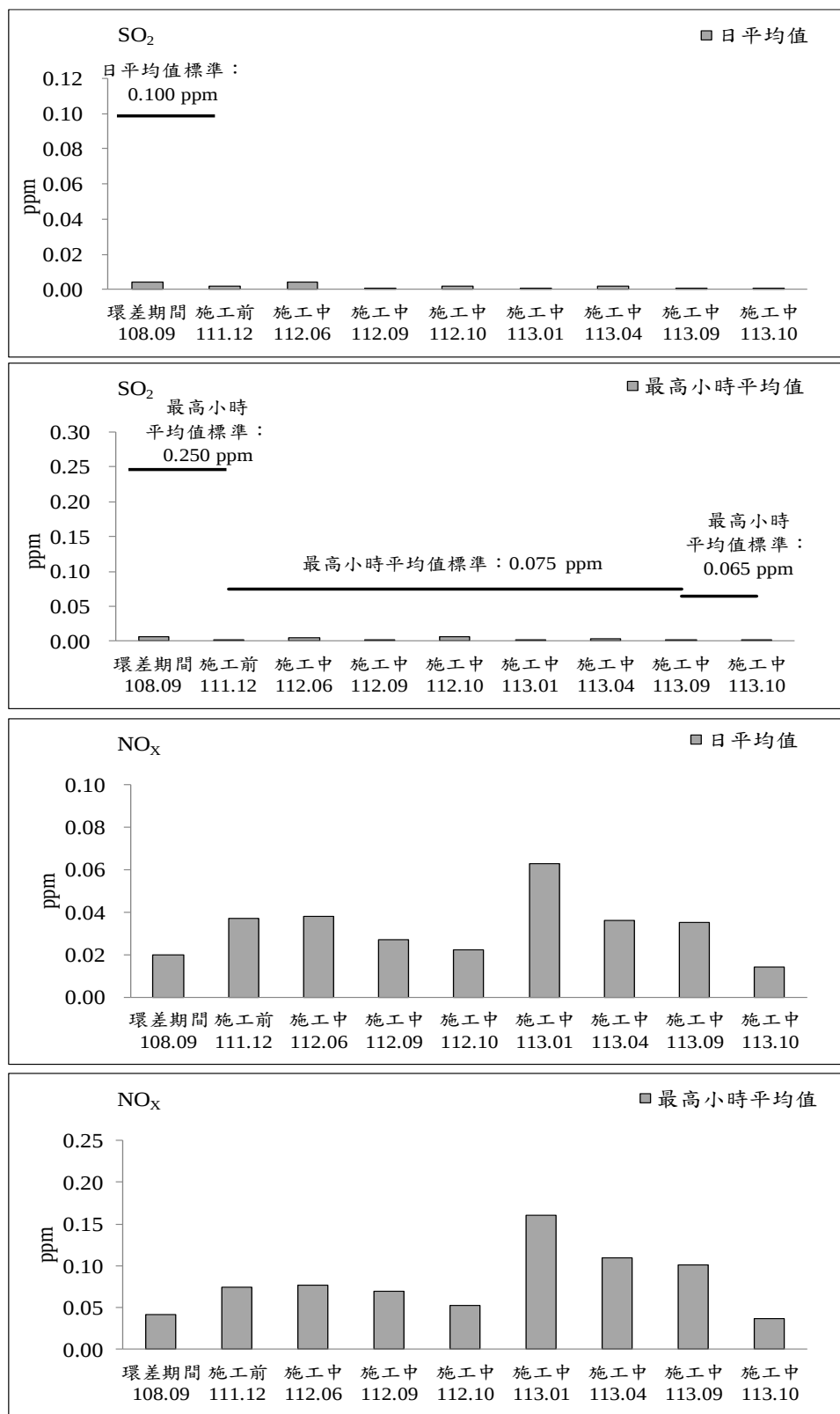
圖 2.1-1 成泰路台北星州社區聚落測站歷次空氣品質監測之各項測值變化圖
