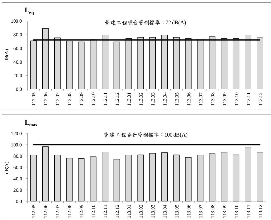
圖 2.4-1 歷次營建工程噪音監測之各項測值變化圖
