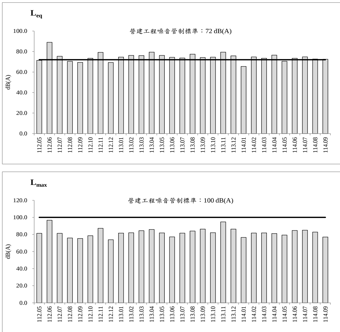
圖 2.4-1 歷次營建工程噪音監測之各項測值變化圖
