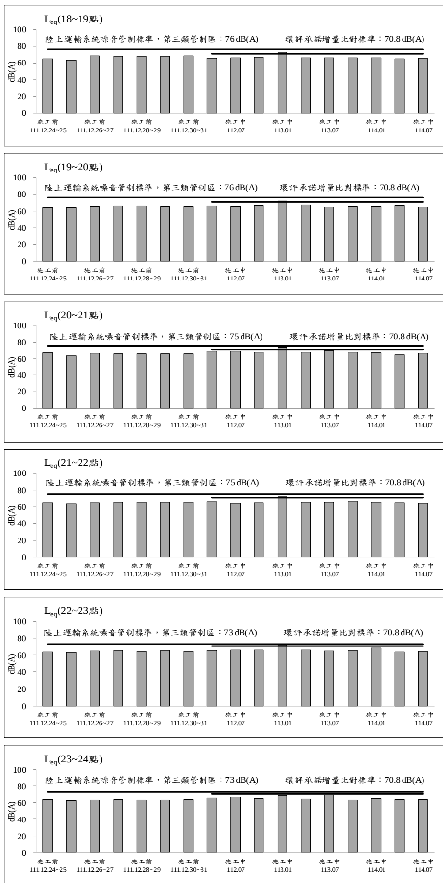
圖 2.2-5 金鑽公寓大廈測站歷次交通噪音監測之各項測值變化圖(假日)
