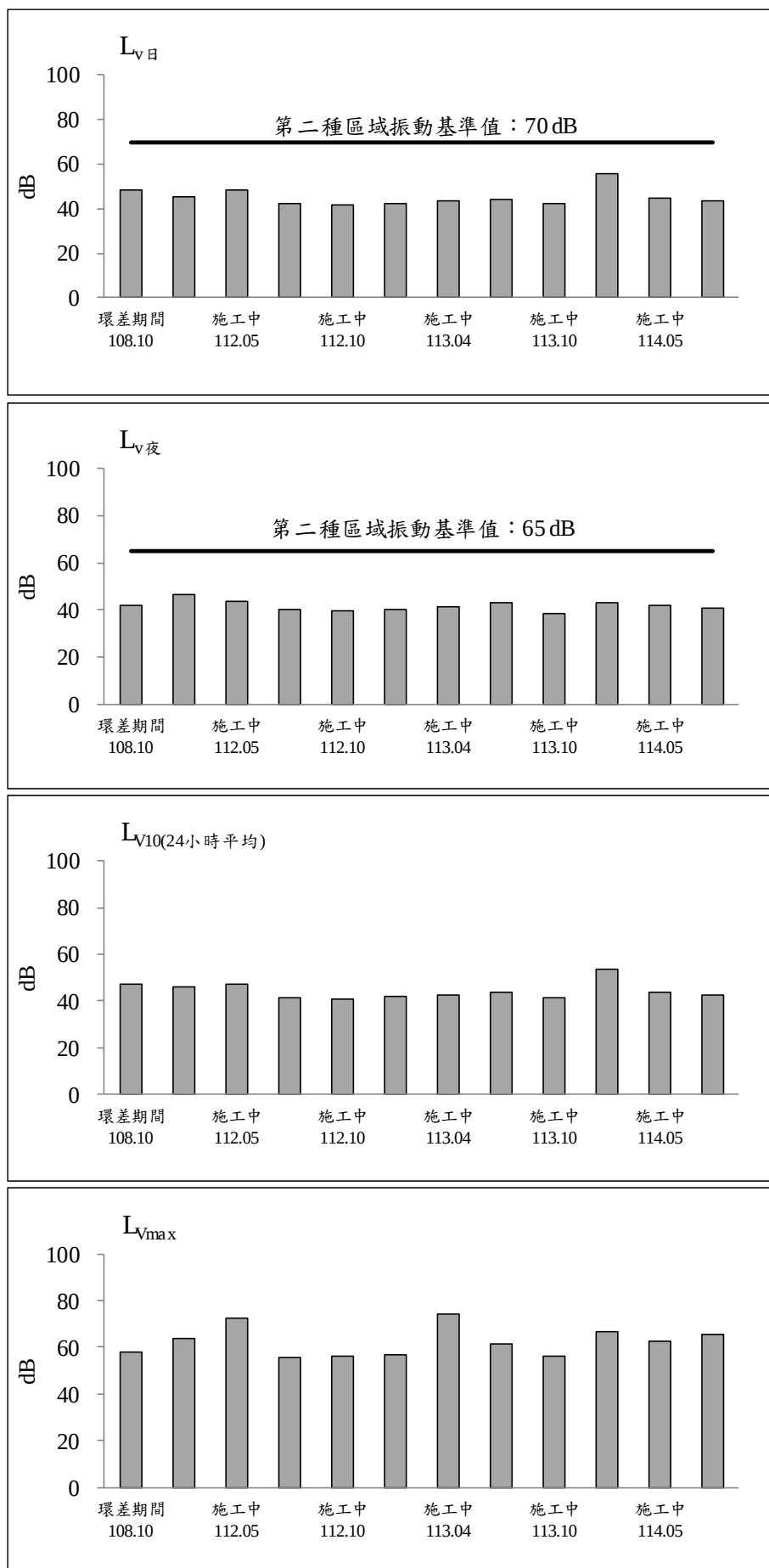
圖 2.2-9 新五路側商家測站歷次振動監測之各項測值變化圖(假日)
