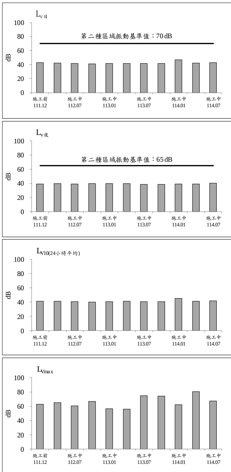
圖 2.2-12 金鑽公寓大廈測站歷次振動監測之各項測值變化圖(平日)
