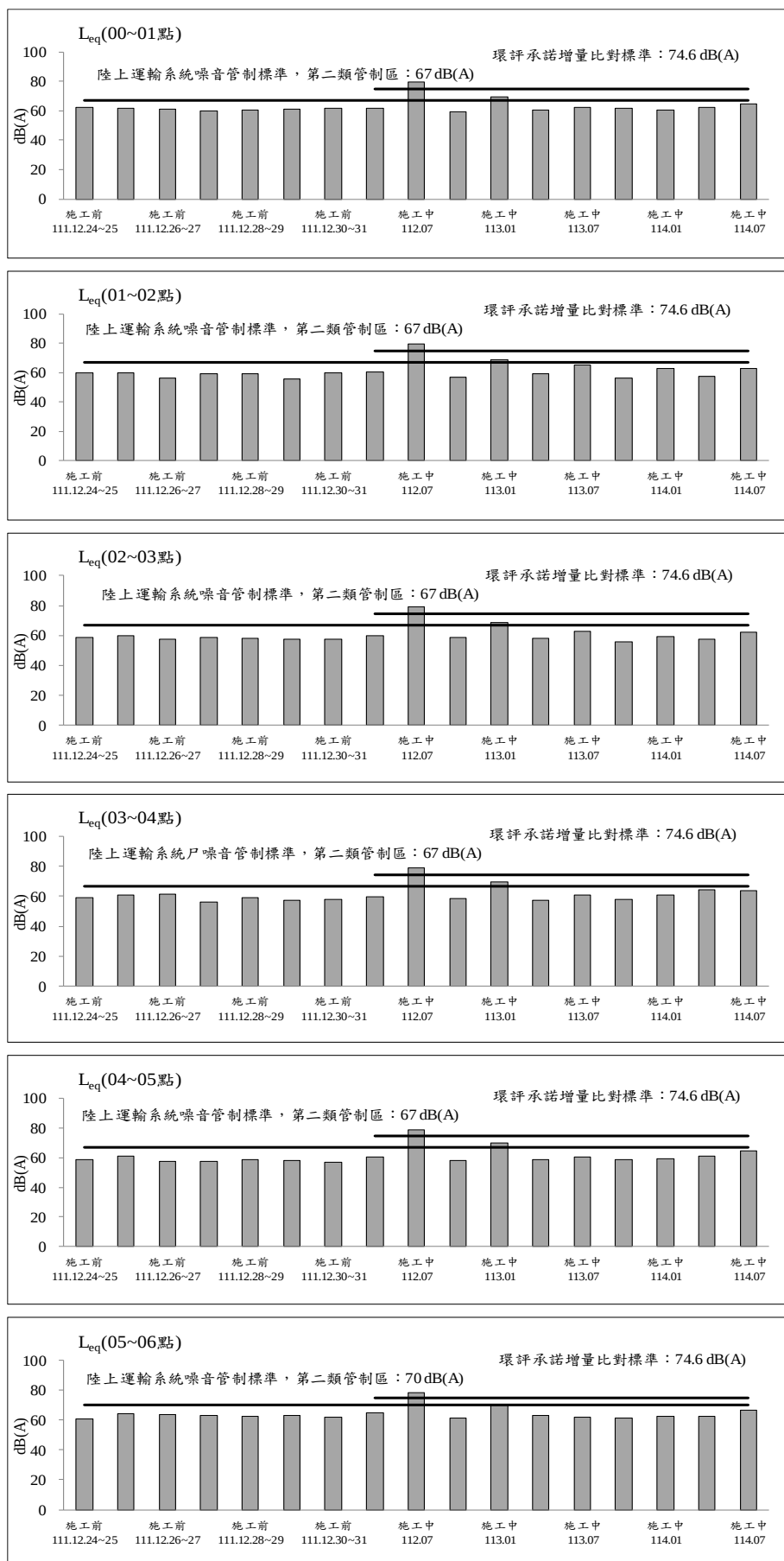
圖 2.2-1 成泰路台北星州社區聚落測站歷次交通噪音監測之各項測值變化圖(假日)
