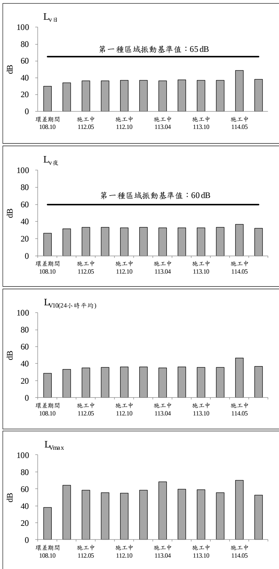
圖 2.2-7 成泰路台北星州社區測站歷次振動監測之各項測值變化圖(假日)
