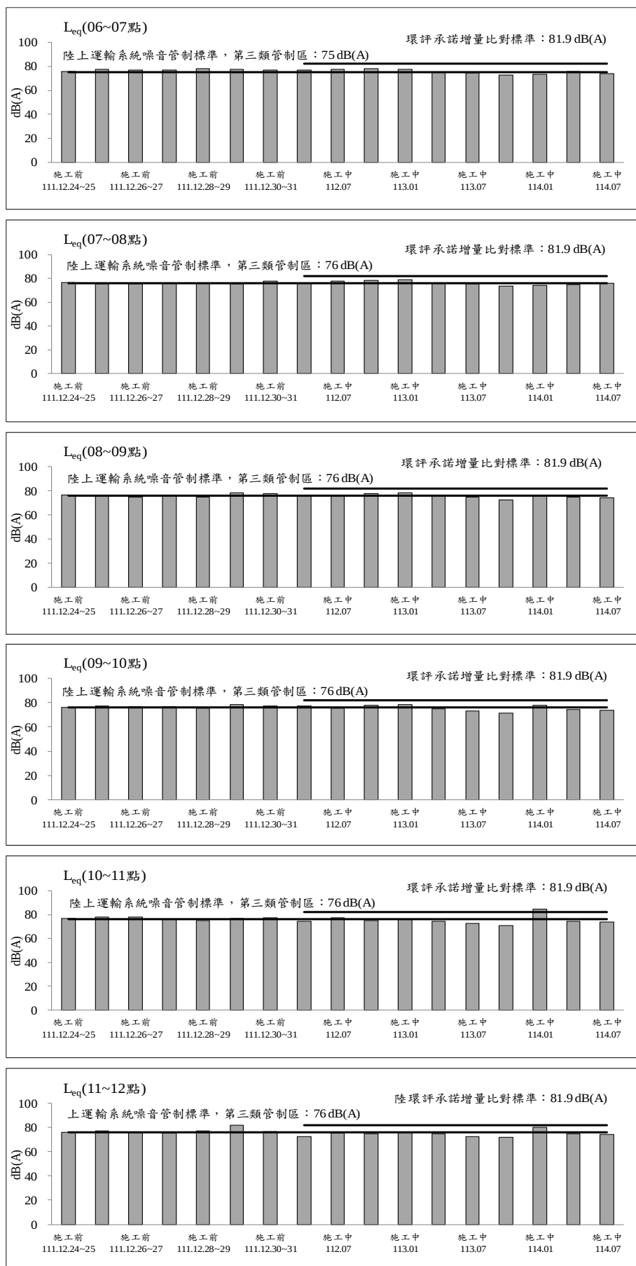
圖 2.2-3 新五路側商家測站歷次交通噪音監測之各項測值變化圖(假日) (續 1)
