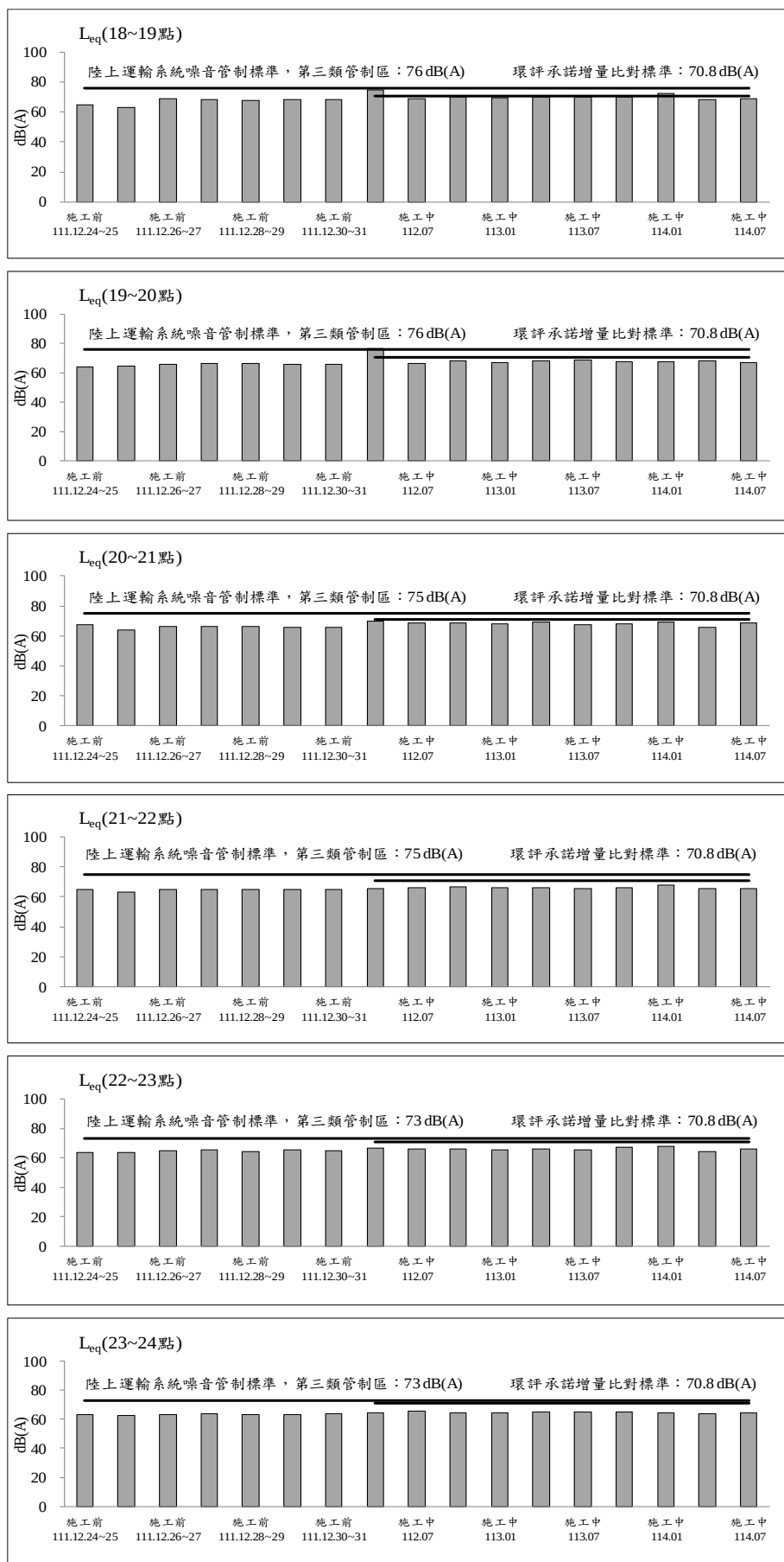
圖 2.2-6 金鑽公寓大廈測站歷次交通噪音監測之各項測值變化圖(平日) (續 3)
