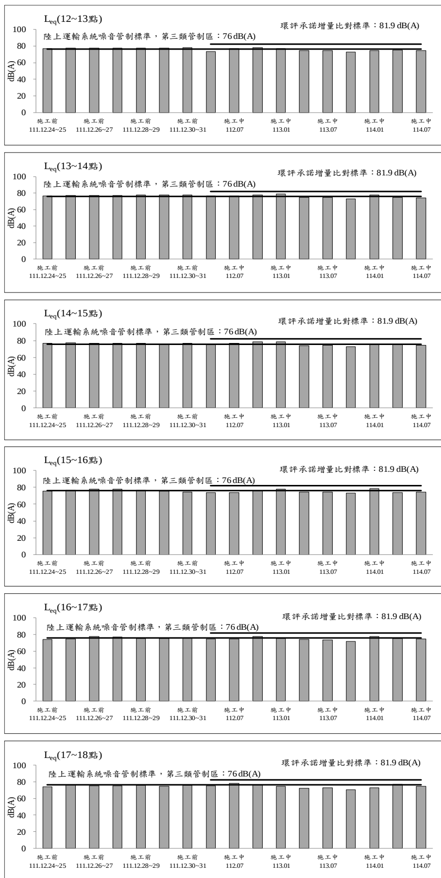
圖 2.2-3 新五路側商家測站歷次交通噪音監測之各項測值變化圖(假日) (續 2)
