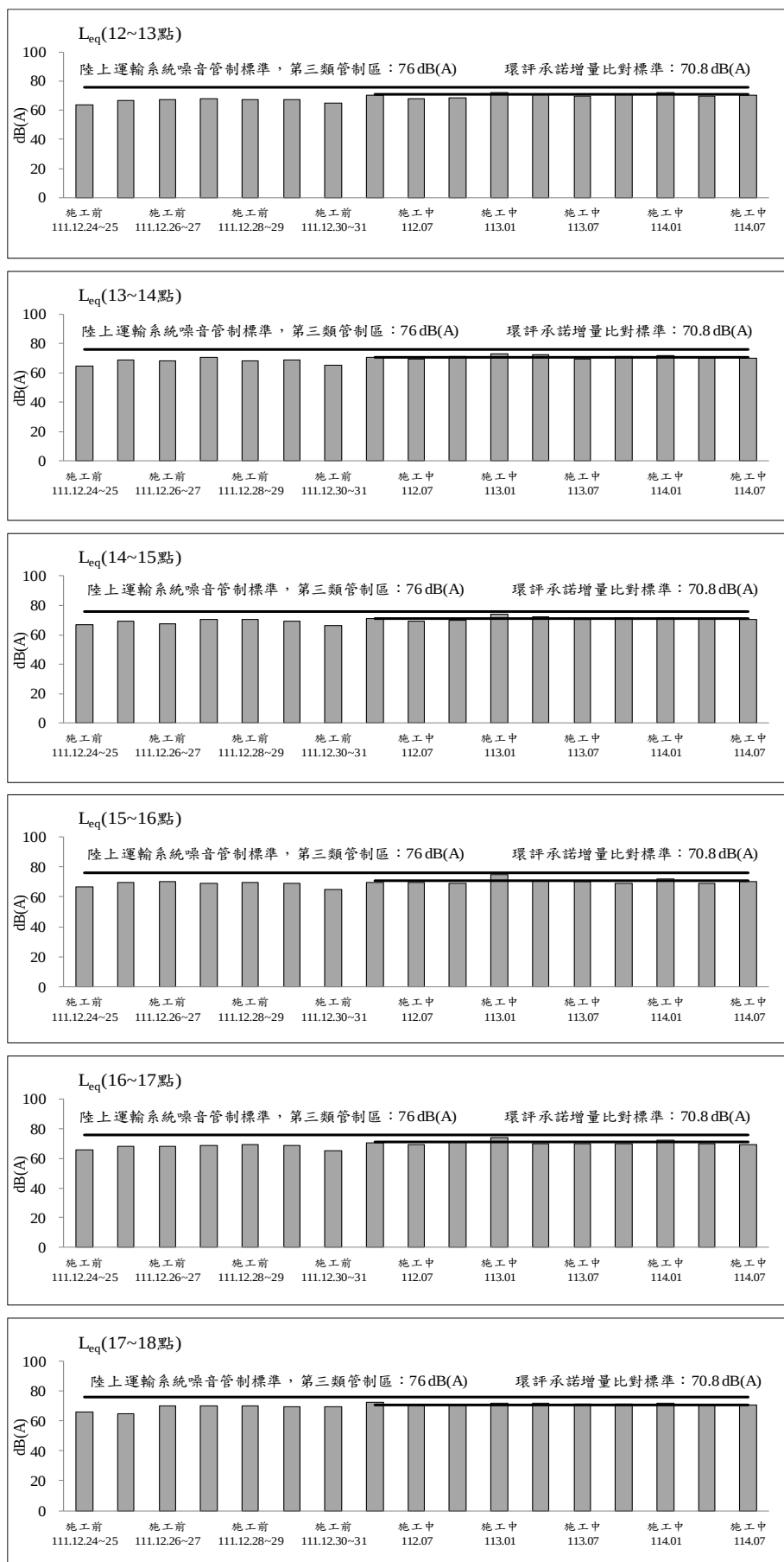
圖 2.2-6 金鑽公寓大廈測站歷次交通噪音監測之各項測值變化圖(平日) (續 2)
