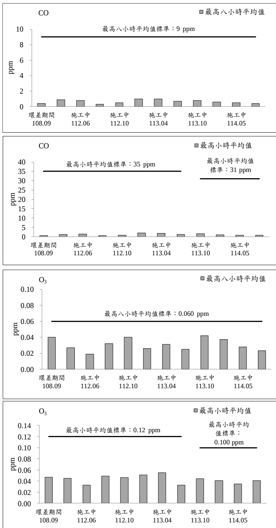
圖 2.1-1 成泰路台北星州社區聚落測站歷次空氣品質監測之各項測值變化圖(續 2)
