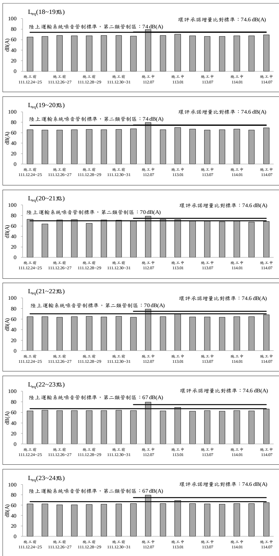
圖 2.2-2 成泰路台北星州社區聚落測站歷次交通噪音監測之各項測值變化圖(平日)(續 3)
