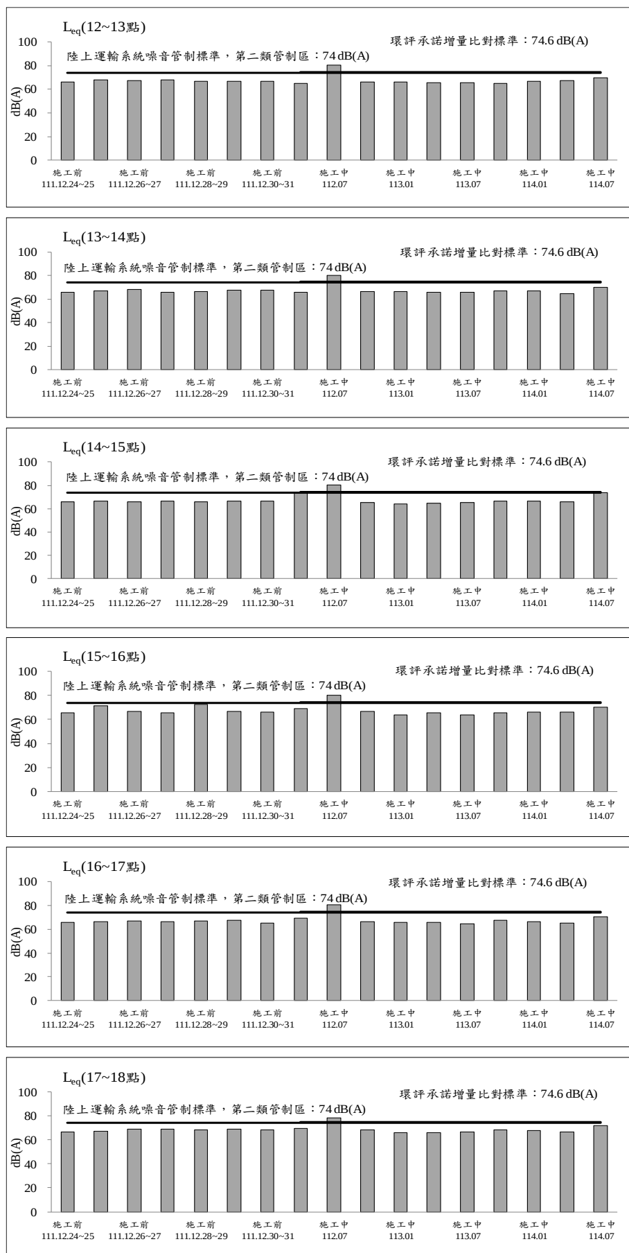
圖 2.2-1 成泰路台北星州社區聚落測站歷次交通噪音監測之各項測值 變化圖(假日)(續 2)
