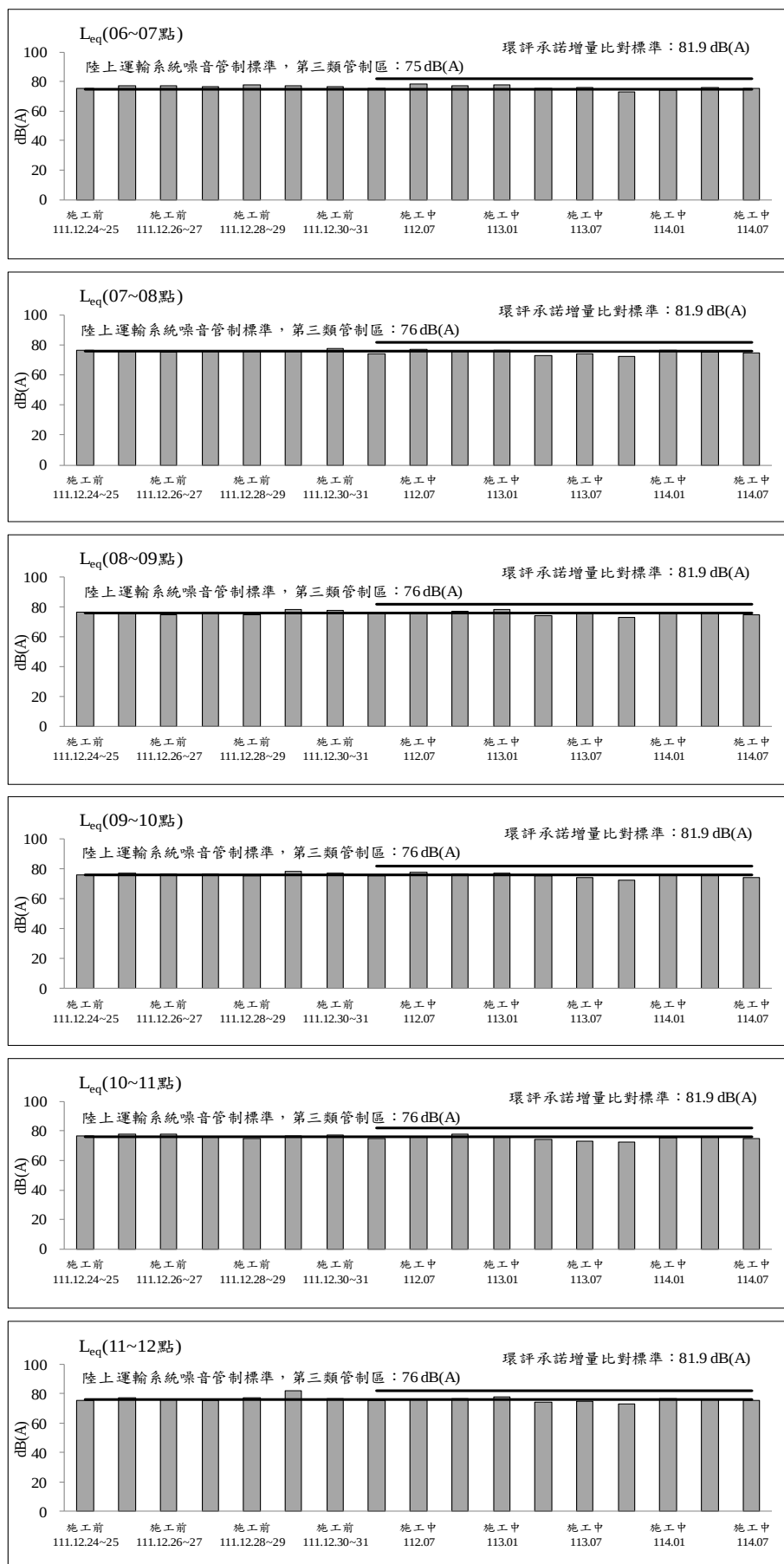
圖 2.2-4 新五路側商家測站歷次交通噪音監測之各項測值變化圖(平日) (續 1)
