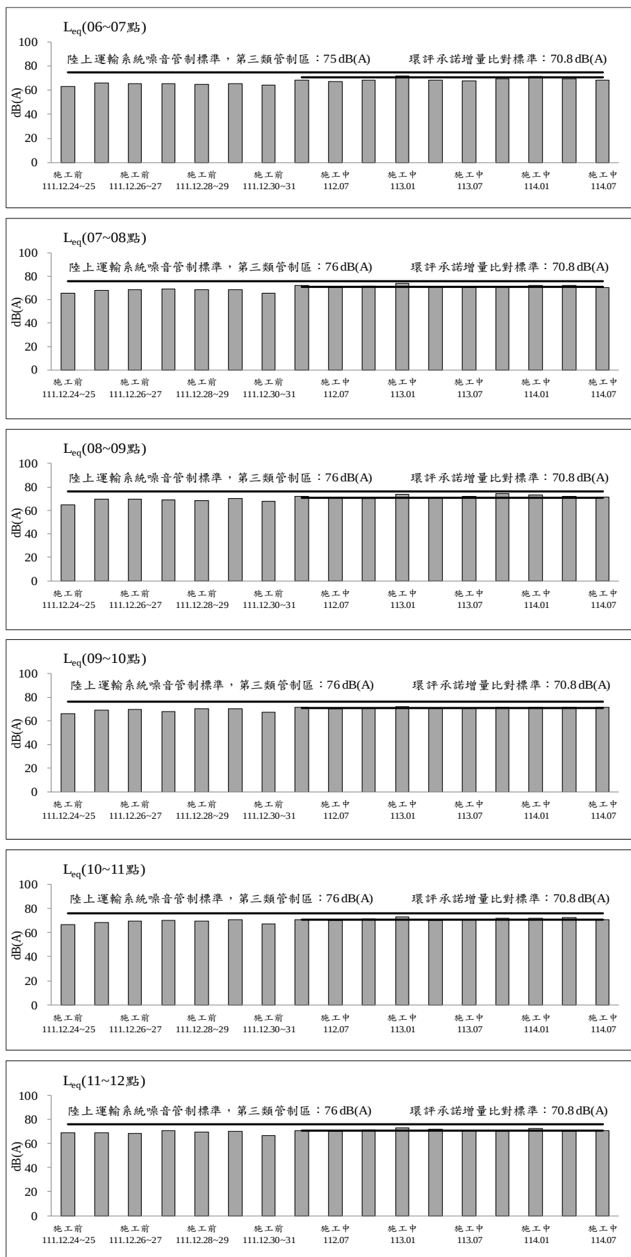
圖 2.2-6 金鑽公寓大廈測站歷次交通噪音監測之各項測值變化圖(平日) (續 1)
