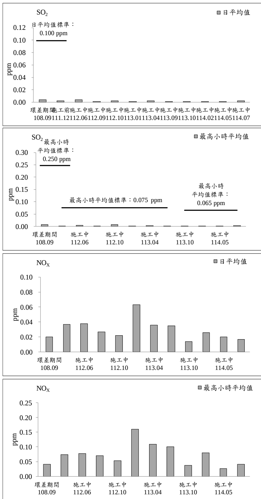
圖 2.1-1 成泰路台北星州社區聚落測站歷次空氣品質監測之各項測值變化圖
