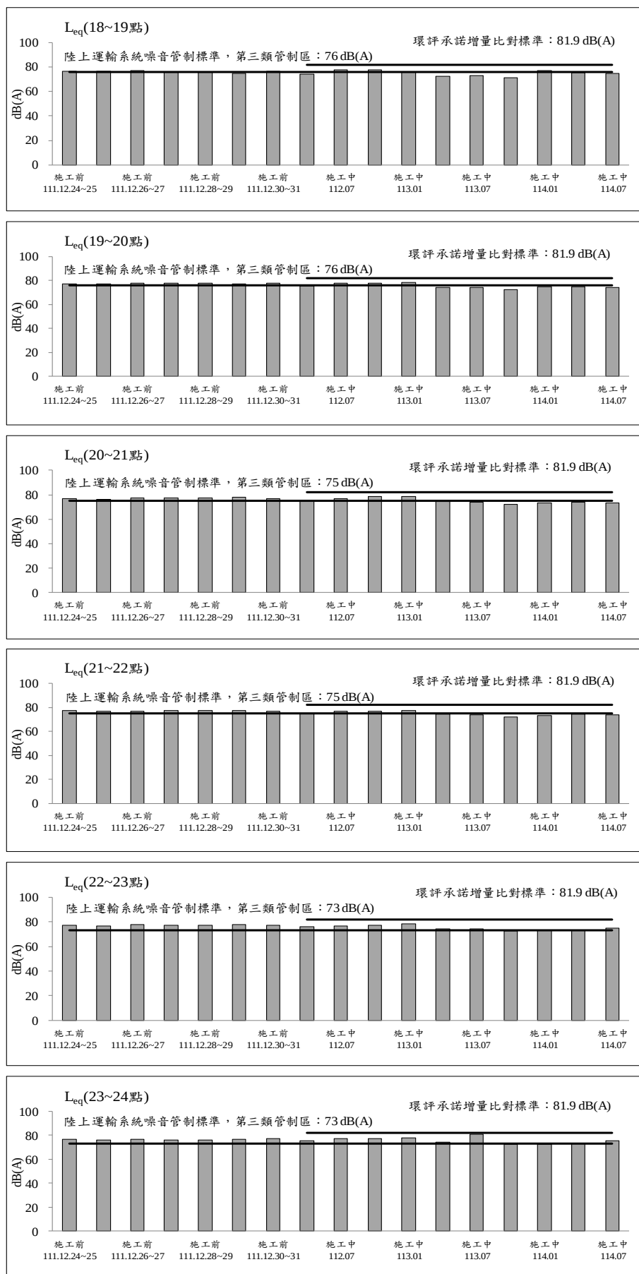
圖 2.2-4 新五路側商家測站歷次交通噪音監測之各項測值變化圖(平日) (續 3)
