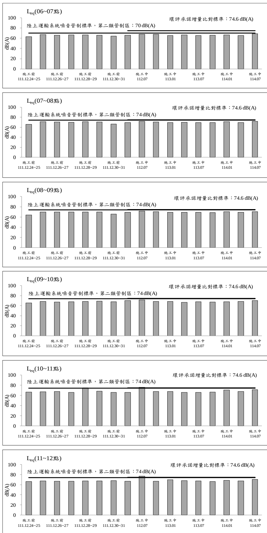
圖 2.2-2 成泰路台北星州社區聚落測站歷次交通噪音監測之各項測值 變化圖(平日)(續 1)
