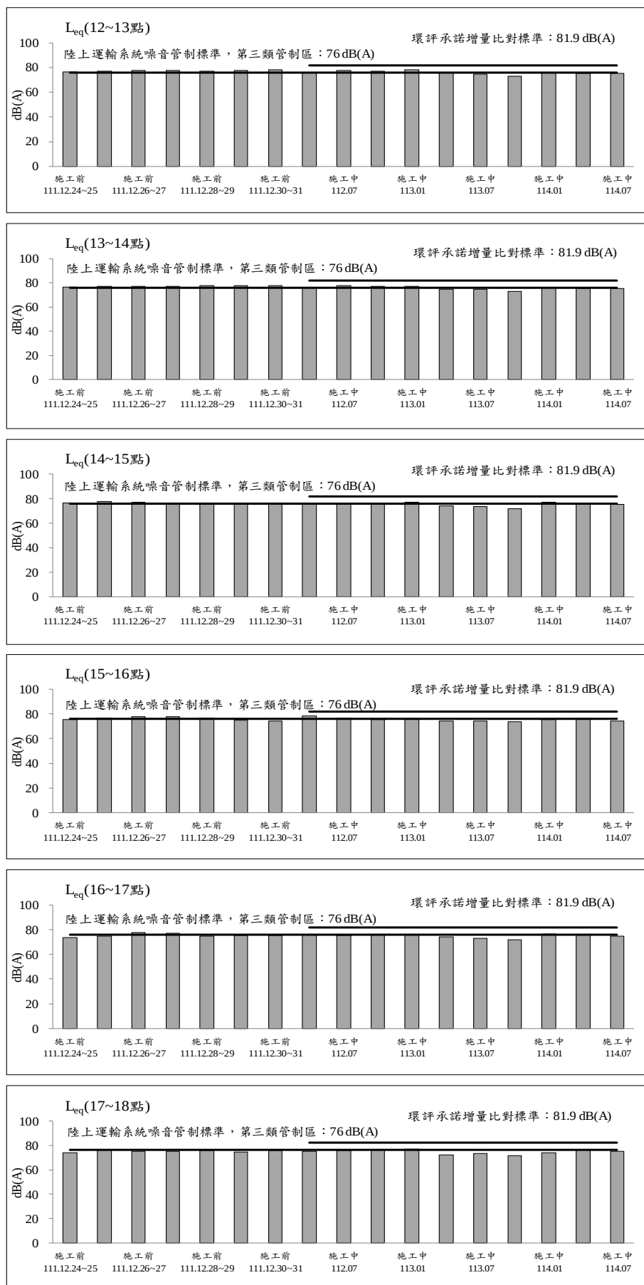
圖 2.2-4 新五路側商家測站歷次交通噪音監測之各項測值變化圖(平日) (續 2)
