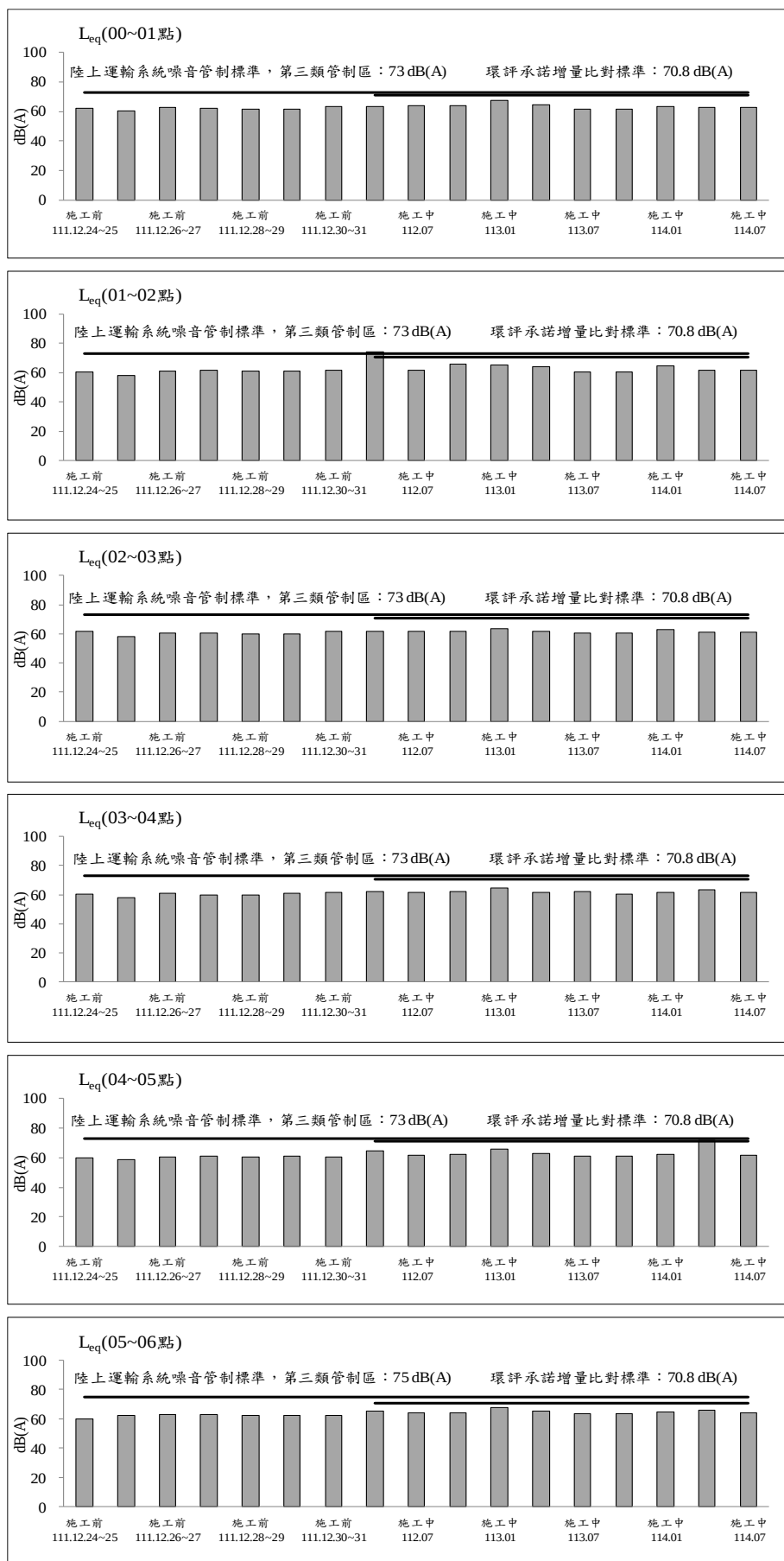
圖 2.2-6 金鑽公寓大廈測站歷次交通噪音監測之各項測值變化圖(平日)
