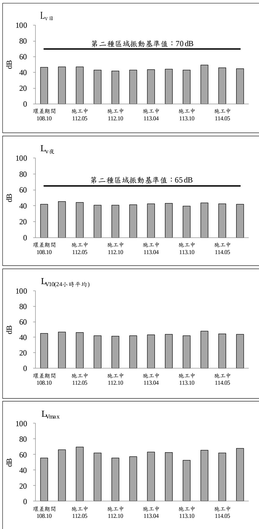
圖 2.2-10 新五路側商家測站歷次振動監測之各項測值變化圖(平日)
