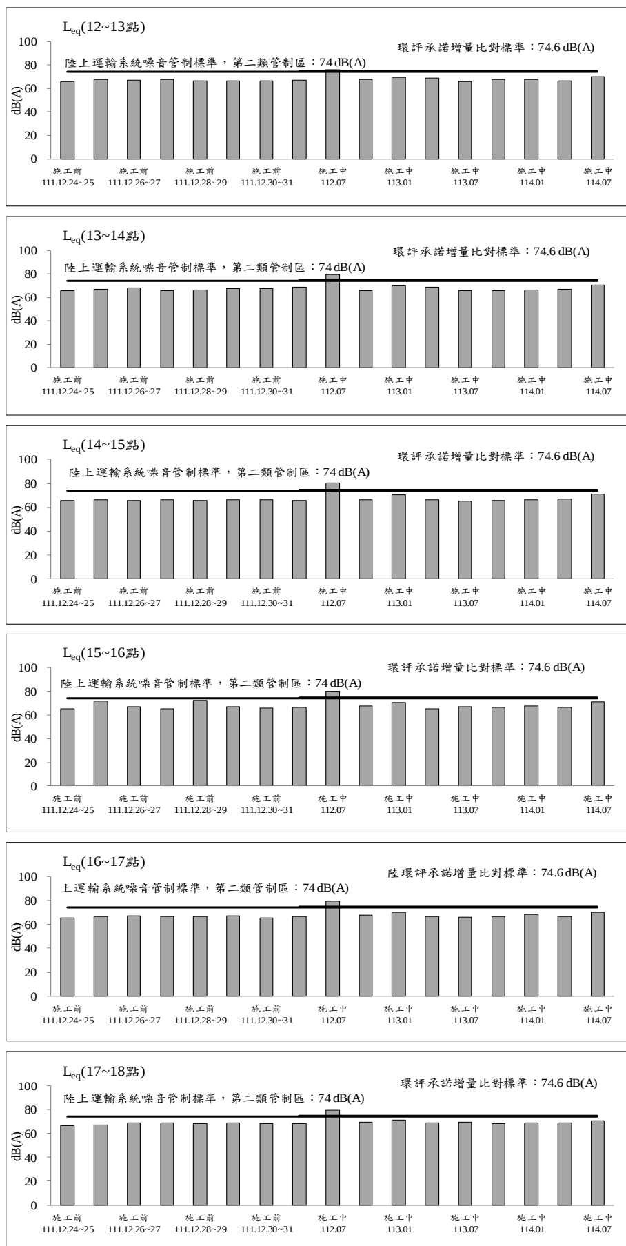
圖 2.2-2 成泰路台北星州社區聚落測站歷次交通噪音監測之各項測值 變化圖(平日)(續 2)
