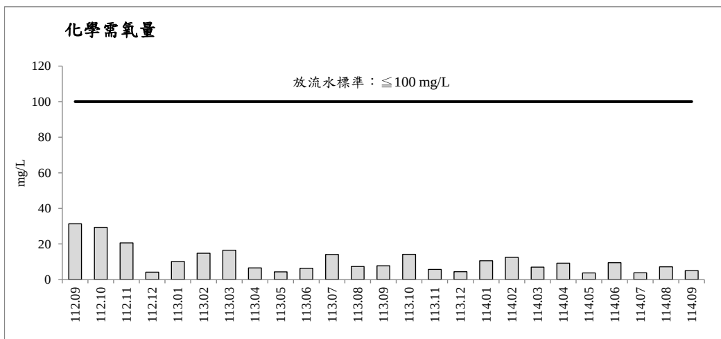
圖 2.5-1 工區放流水監測之各項測值變化圖(續)
