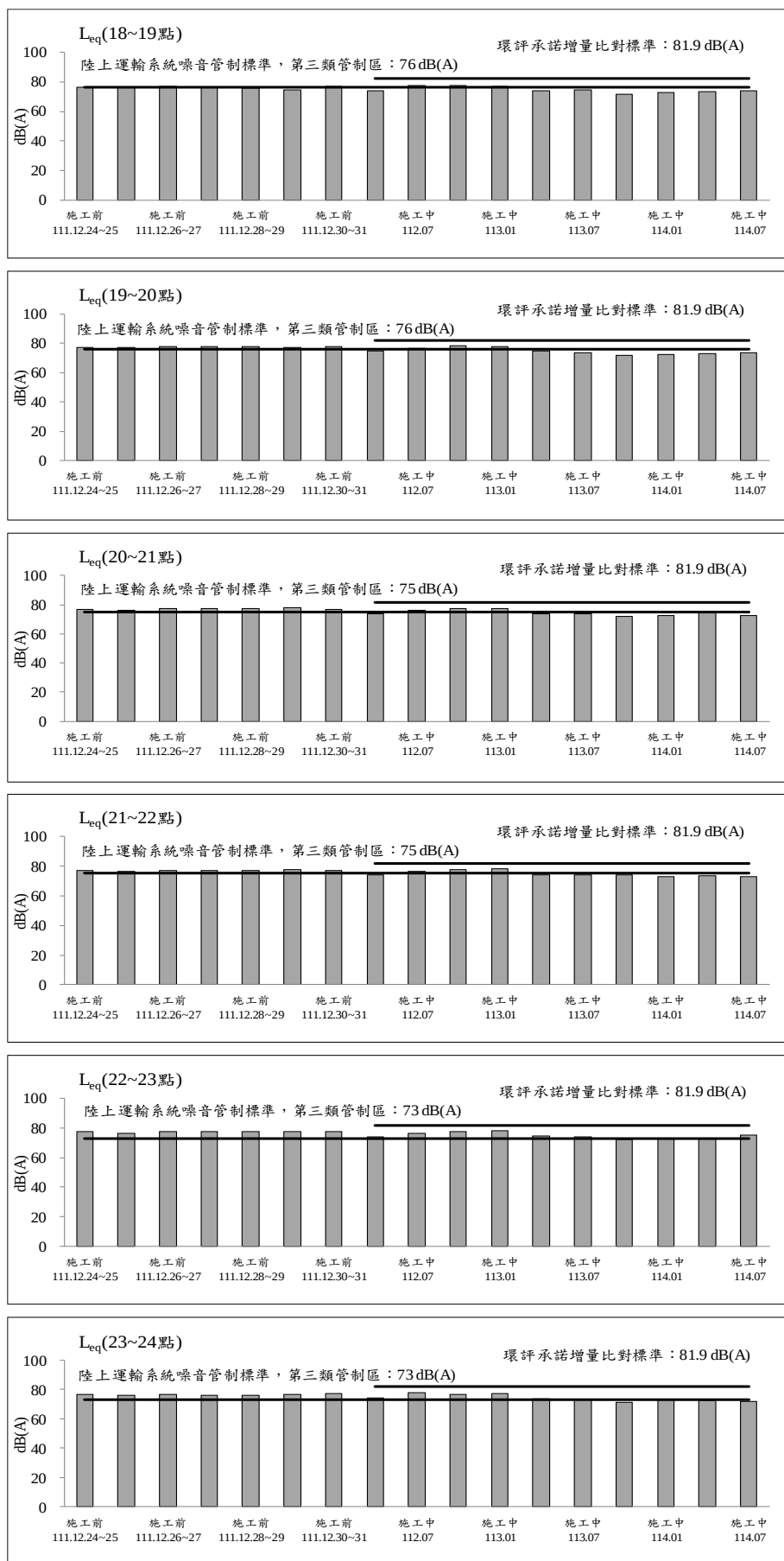
圖 2.2-3 新五路側商家測站歷次交通噪音監測之各項測值變化圖(假日) (續 3)
