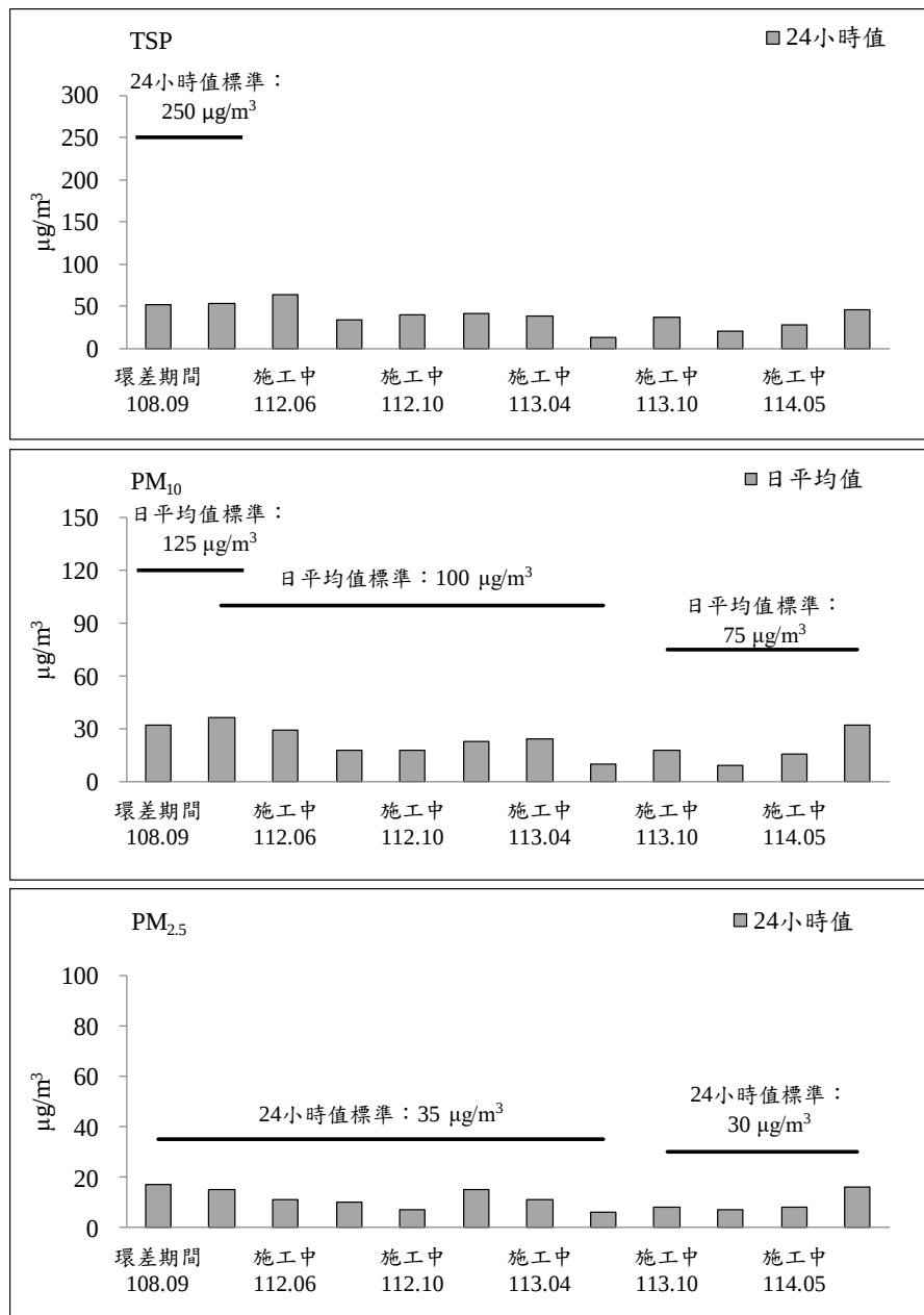
圖 2.1-1 成泰路台北星州社區聚落測站歷次空氣品質監測之各項測值變化圖(續 3)
