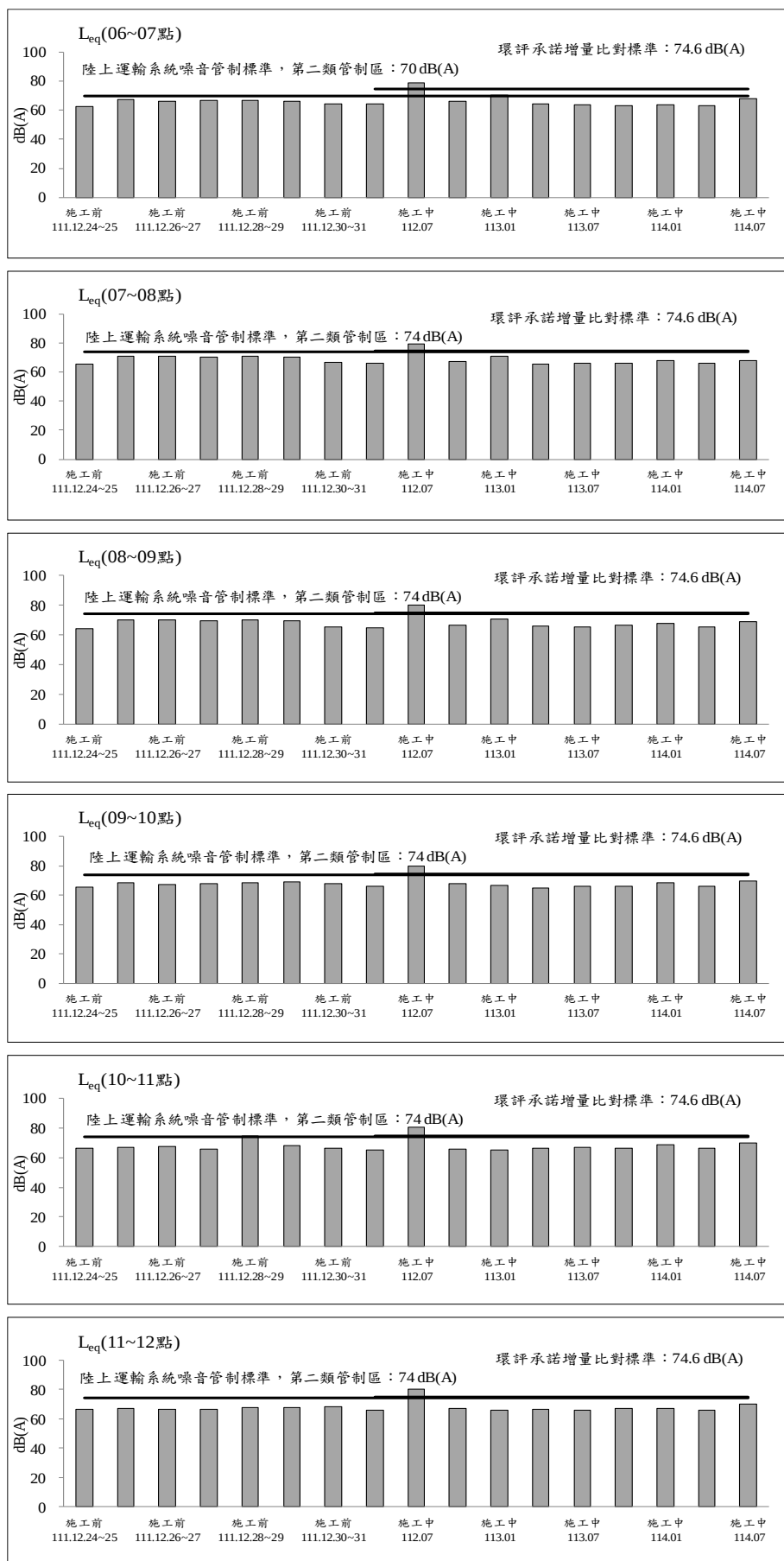
圖 2.2-1 成泰路台北星州社區聚落測站歷次交通噪音監測之各項測值 變化圖(假日)(續 1)
