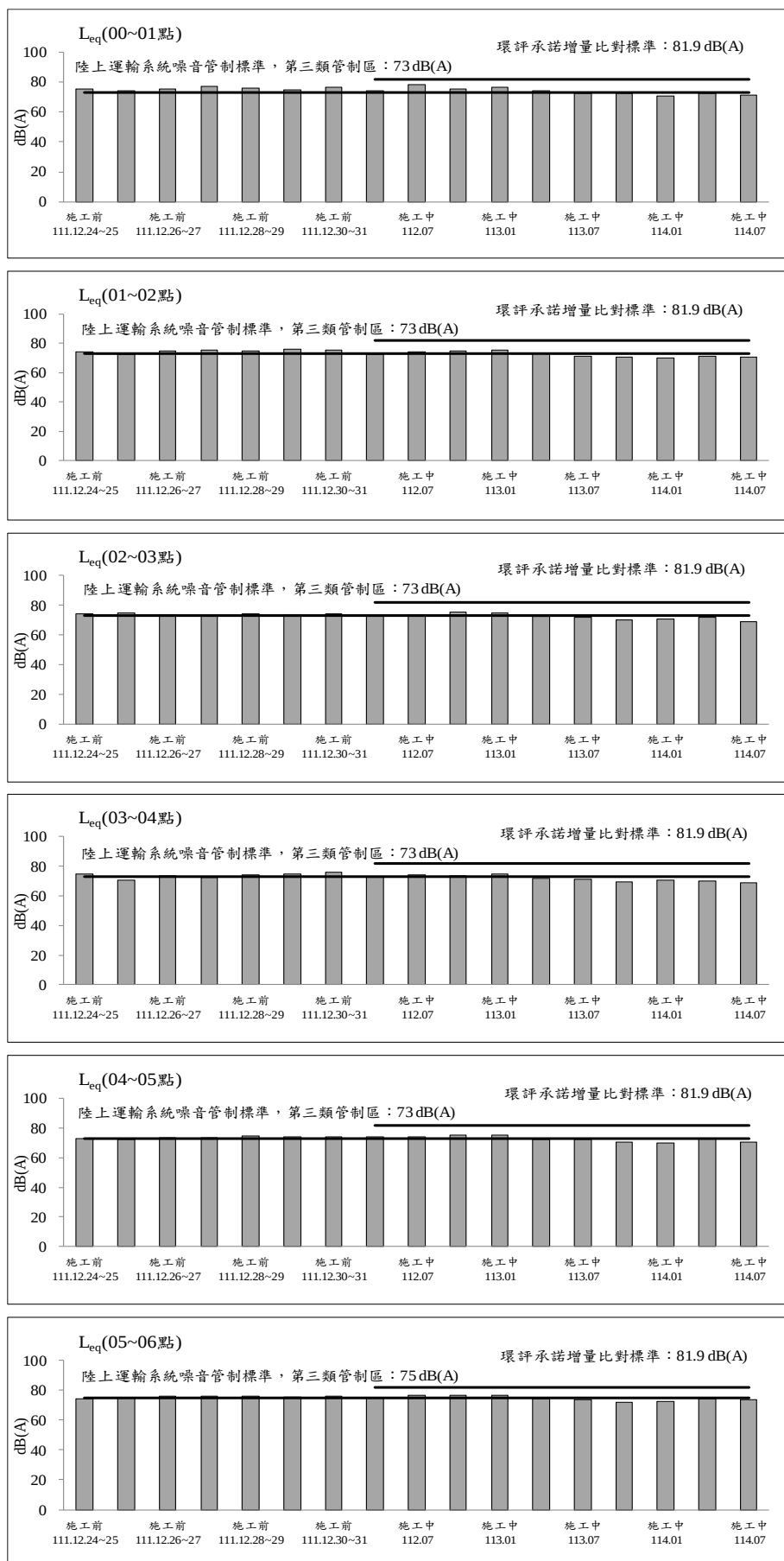
圖 2.2-4 新五路側商家測站歷次交通噪音監測之各項測值變化圖(平日)
