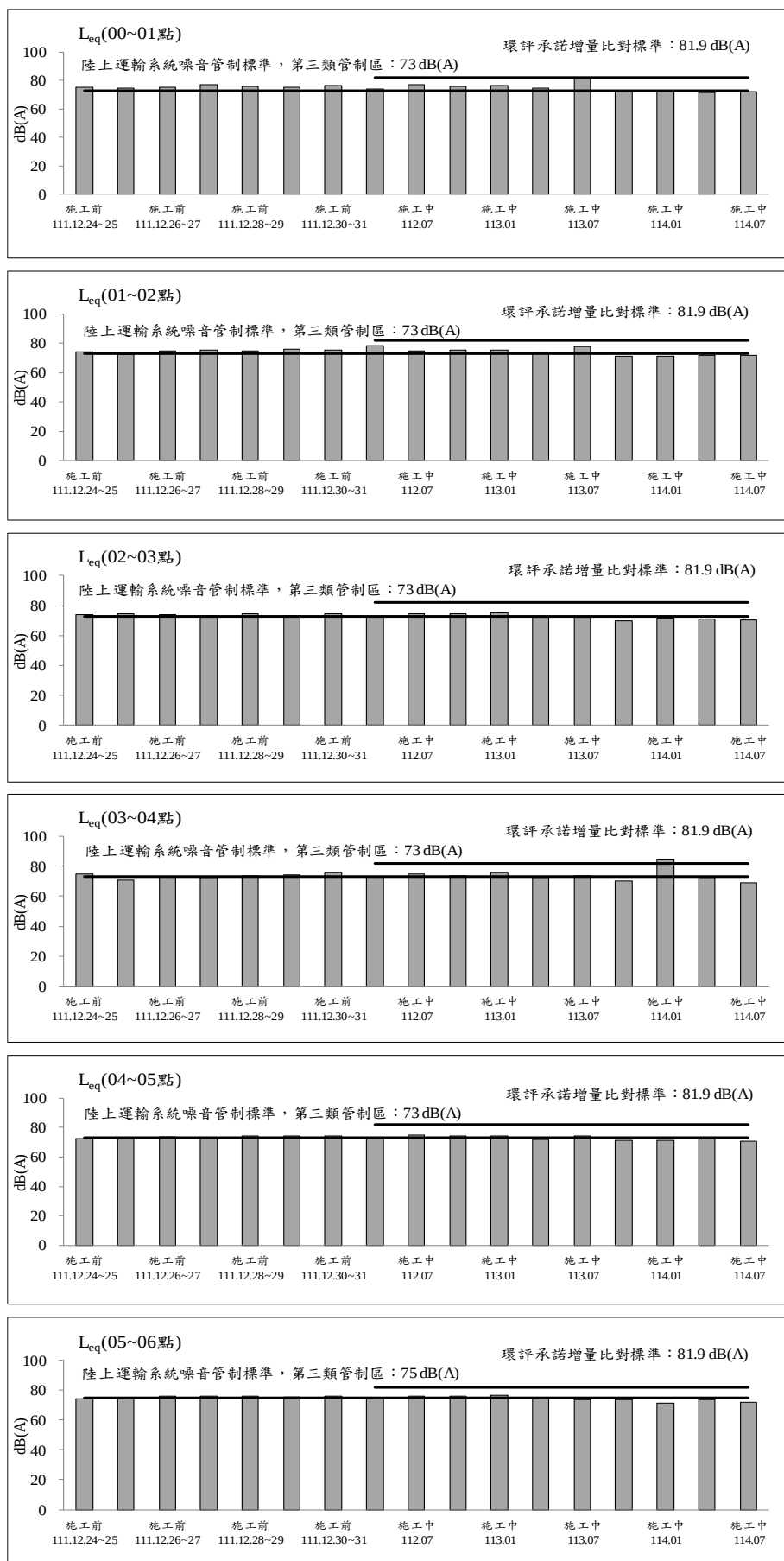
圖 2.2-3 新五路側商家測站歷次交通噪音監測之各項測值變化圖(假日)
