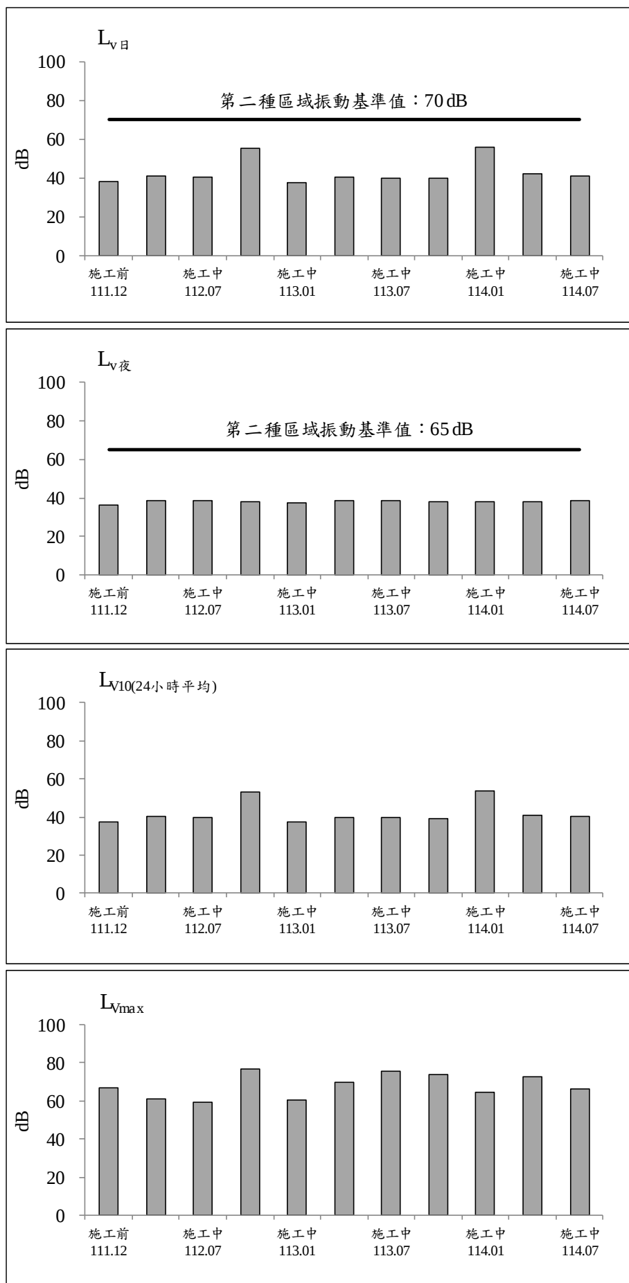
圖 2.2-11 金鑽公寓大廈測站歷次振動監測之各項測值變化圖(假日)
