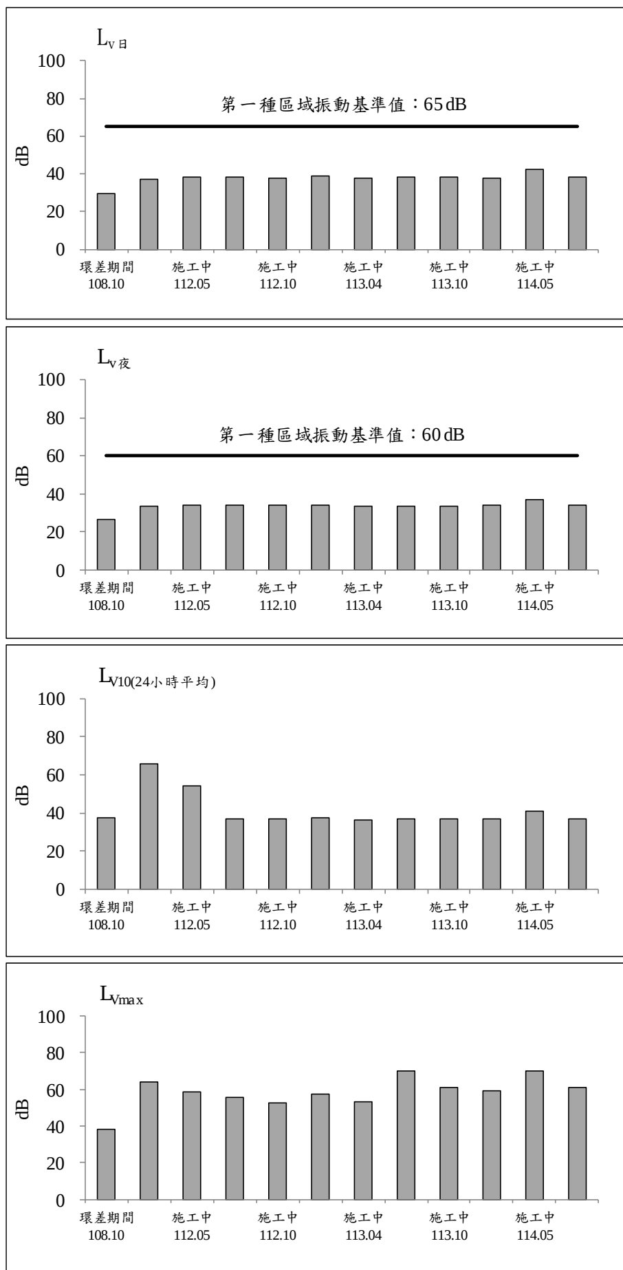
圖 2.2-8 成泰路台北星州社區測站歷次振動監測之各項測值變化圖(平日)
