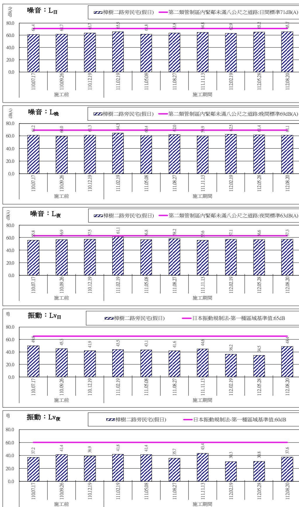
圖 2.2-2 噪音及振動監測結果比較圖-樟樹二路旁民宅(假日)
