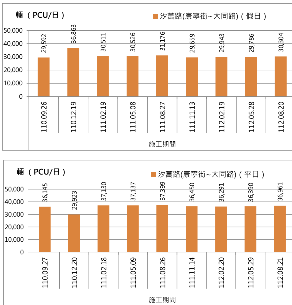
圖 2.4-2 路段交通量統計結果比較圖-汐萬路(康寧街~大同路)
