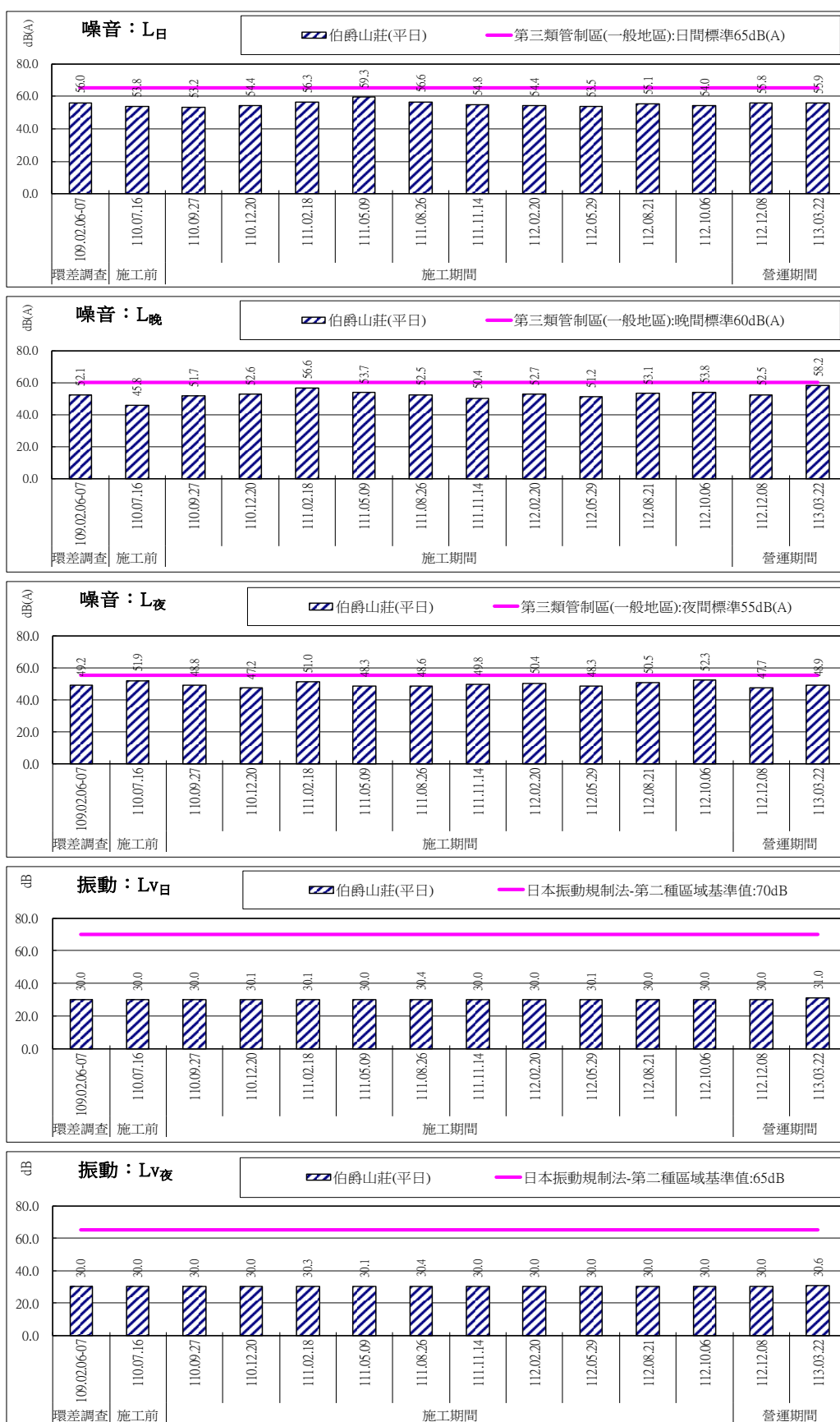
圖 2.1-1 噪音及振動監測結果比較圖-伯爵山莊(平日)
