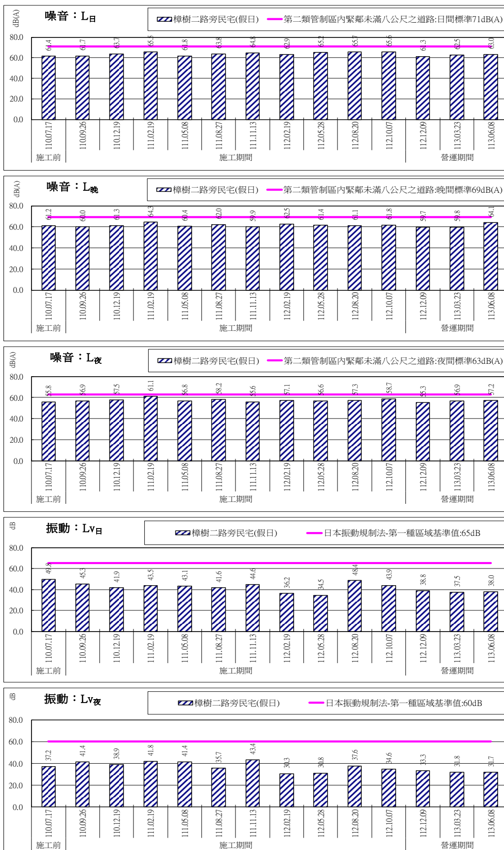
圖 2.1-2 噪音及振動監測結果比較圖-樟樹二路旁民宅(假日)
