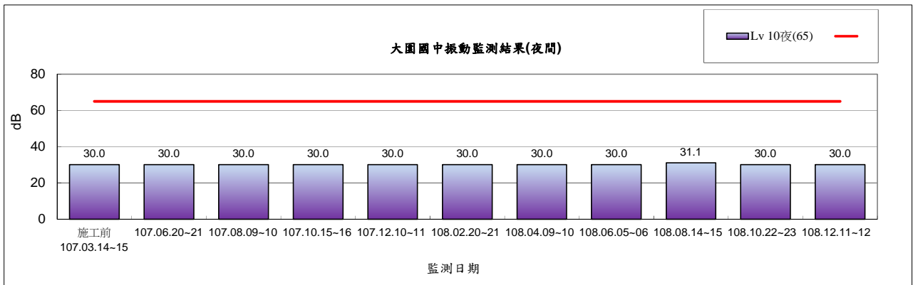
圖 2.2-10 大園國中環境振動監測結果(夜間)
