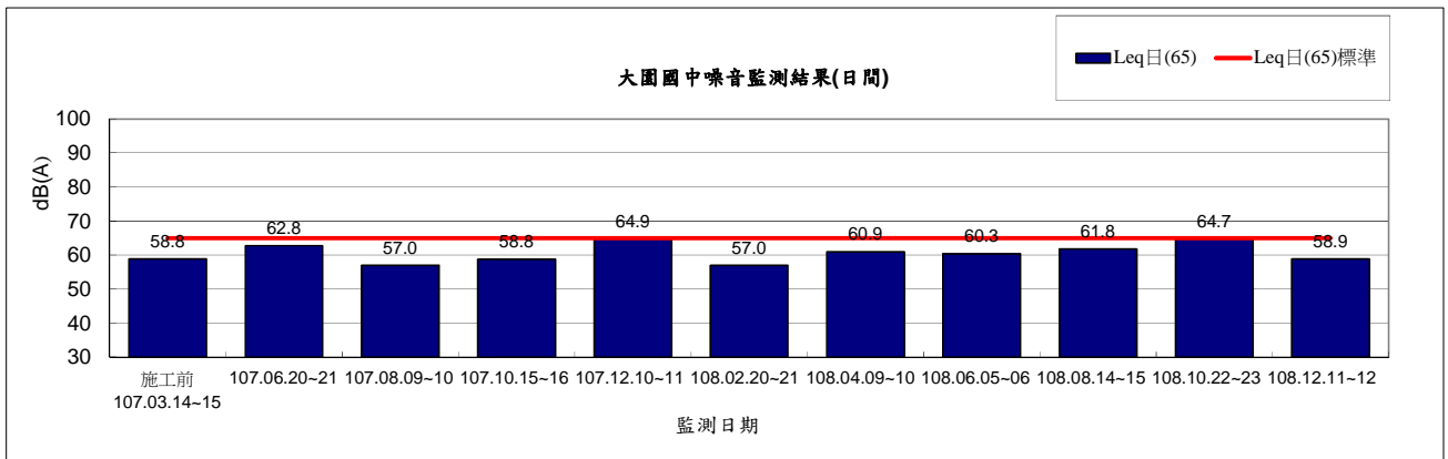
圖 2.2-4 大園國中環境噪音監測結果(日間)
