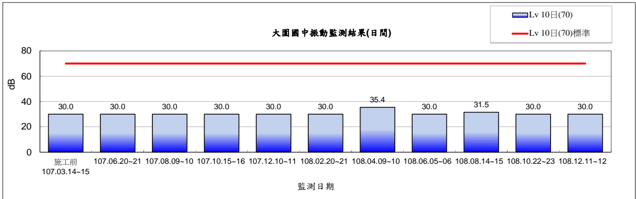
圖 2.2-9 大園國中環境振動監測結果(日間)
