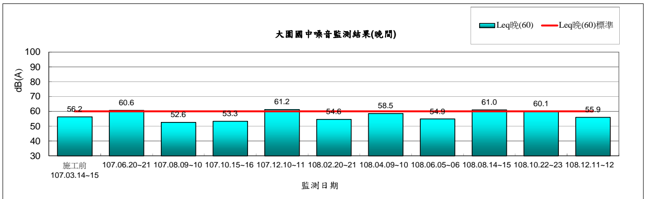
圖 2.2-5 大園國中環境噪音監測結果(晚間)
