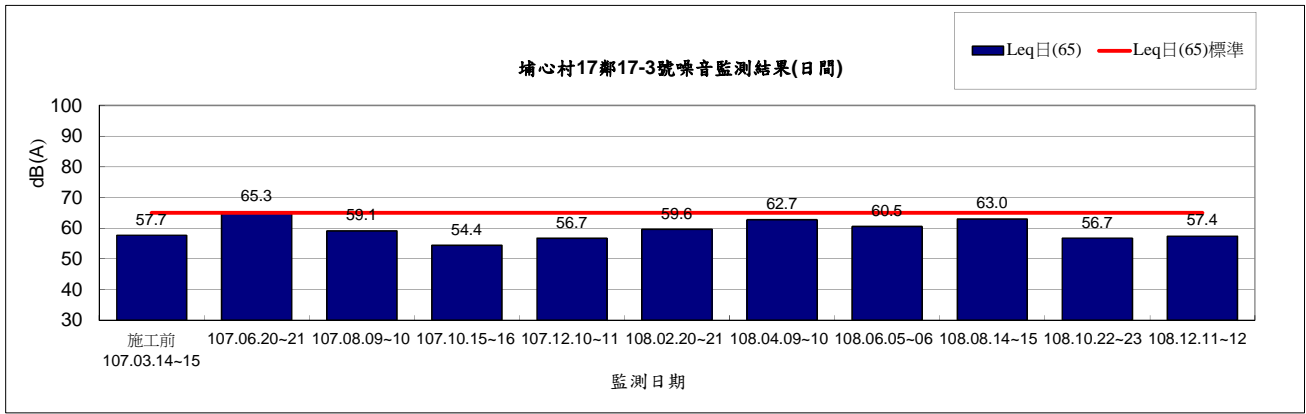
圖 2.2-1 埔心村 17 鄰 17-3 號環境噪音監測結果(日間)
