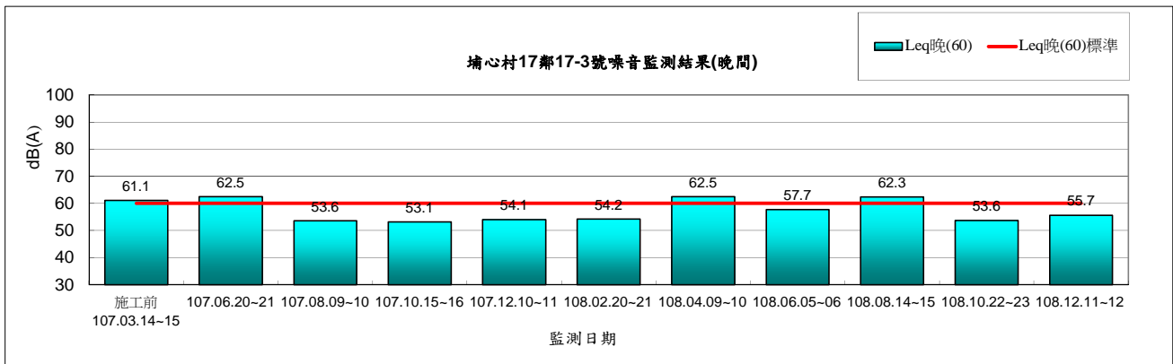
圖 2.2-2 埔心村 17 鄰 17-3 號環境噪音監測結果(晚間)
