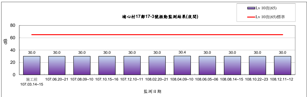
圖 2.2-8 埔心村 17 鄰 17-3 號環境振動監測結果(夜間)
