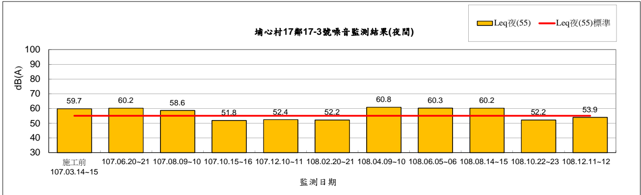
圖 2.2-3 埔心村 17 鄰 17-3 號環境噪音監測結果(夜間)
