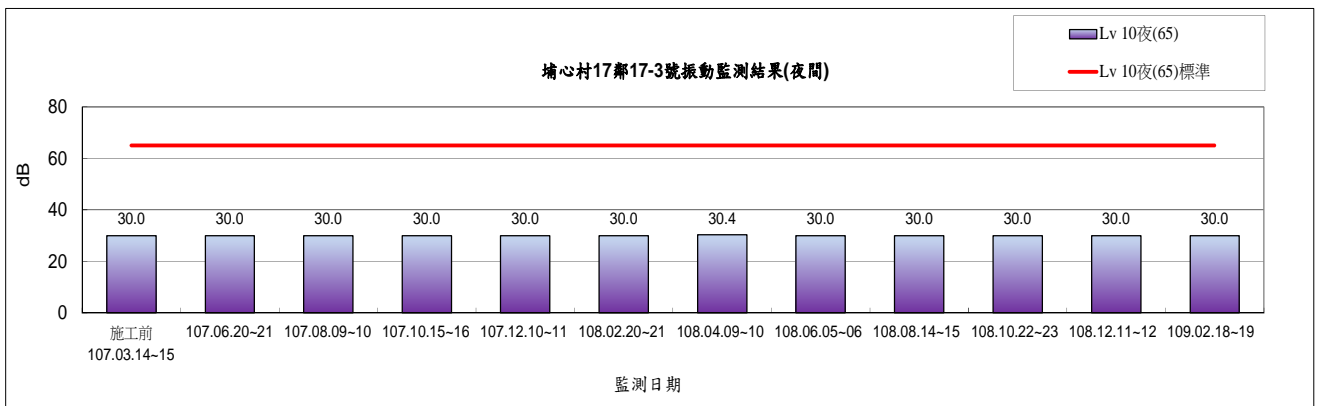
圖 2.2-8 埔心村 17 鄰 17-3 號環境振動監測結果(夜間)
