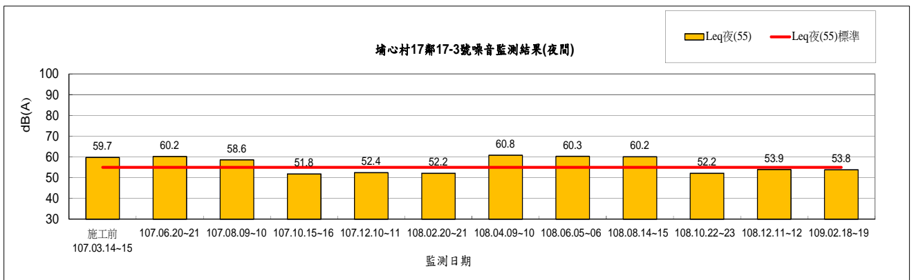
圖 2.2-3 埔心村 17 鄰 17-3 號環境噪音監測結果(夜間)
