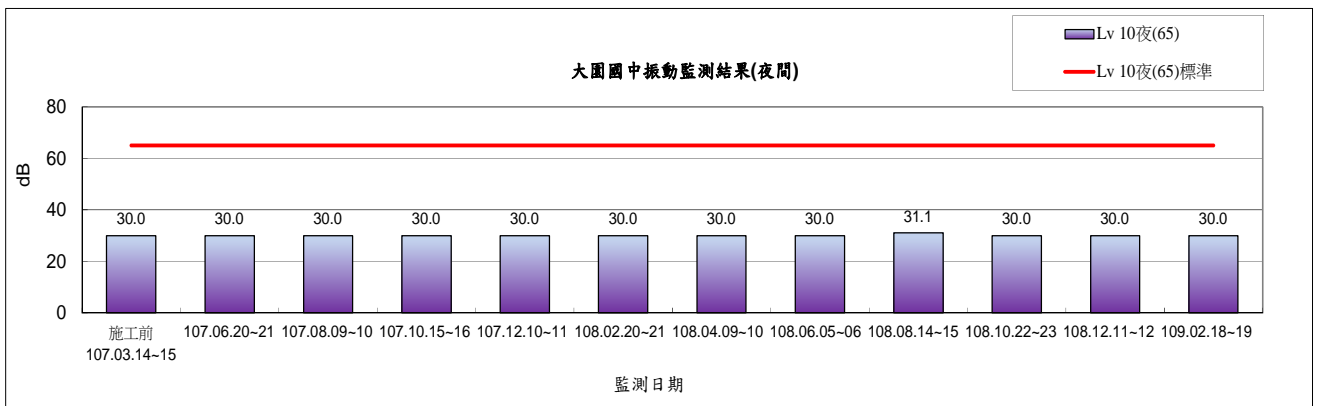
圖 2.2-10 大園國中環境振動監測結果(夜間)
