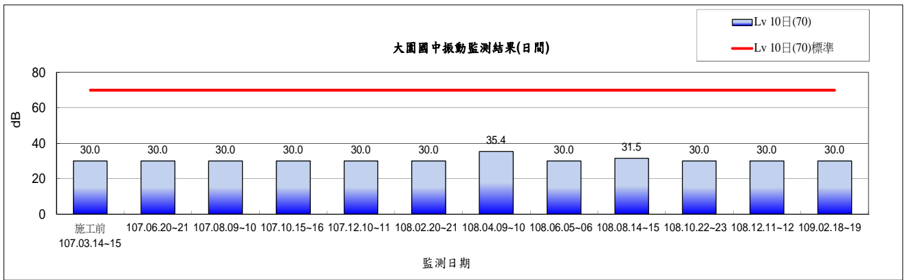
圖 2.2-9 大園國中環境振動監測結果(日間)
