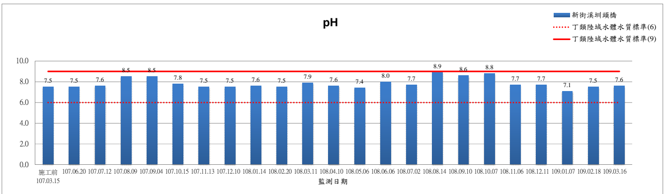
圖 2.3-1 河川水質之 pH 監測結果趨勢圖
