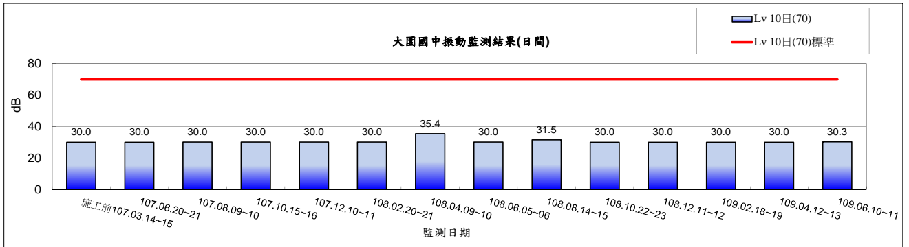
圖 2.2-9 大園國中環境振動監測結果(日間)
