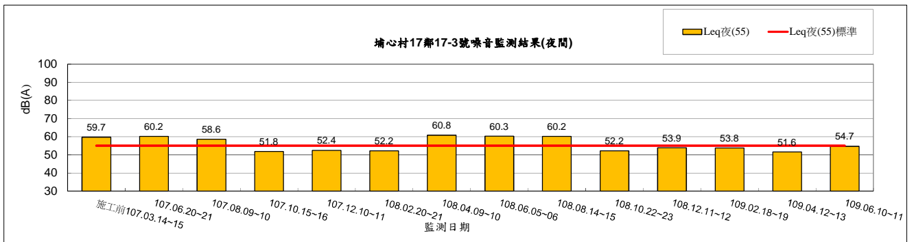
圖 2.2-3 埔心村 17 鄰 17-3 號環境噪音監測結果(夜間)
