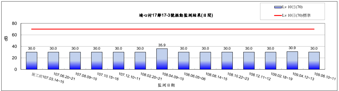
圖 2.2-7 埔心村 17 鄰 17-3 號環境振動監測結果(日間)
