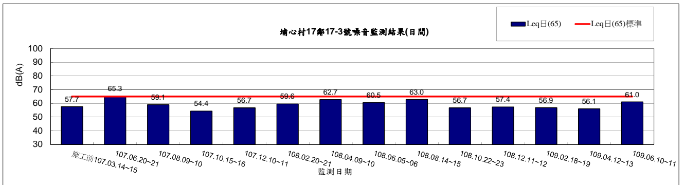
圖 2.2-1 埔心村 17 鄰 17-3 號環境噪音監測結果(日間)
