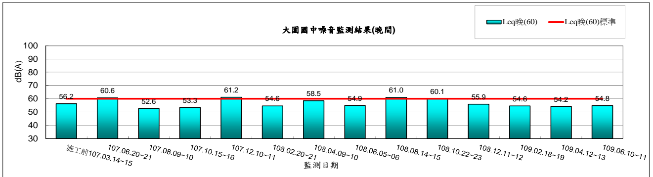
圖 2.2-5 大園國中環境噪音監測結果(晚間)
