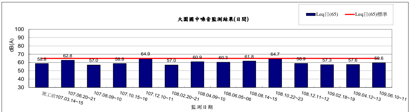
圖 2.2-4 大園國中環境噪音監測結果(日間)
