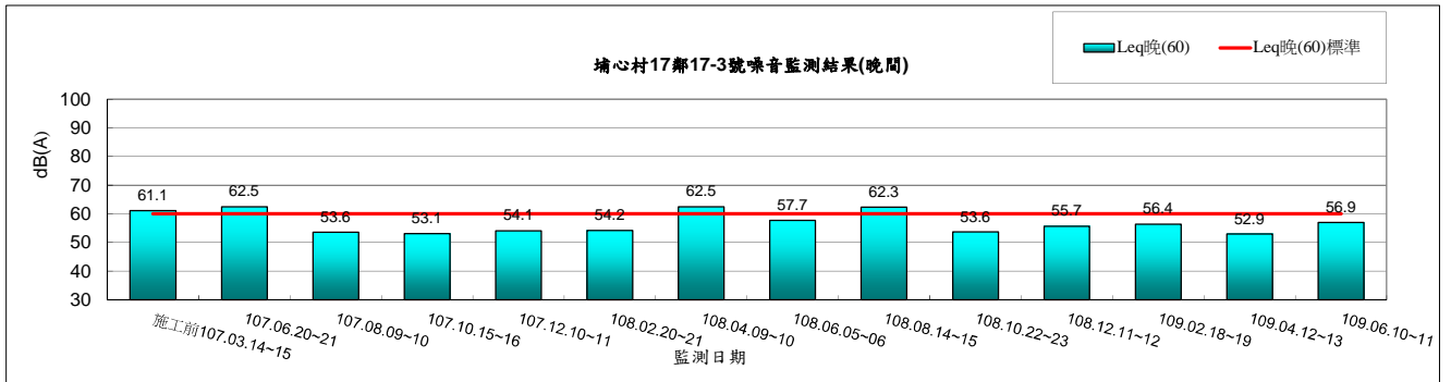
圖 2.2-2 埔心村 17 鄰 17-3 號環境噪音監測結果(晚間)
